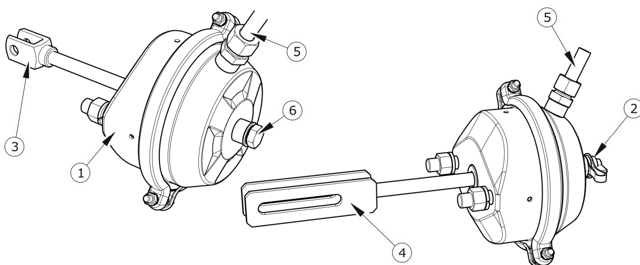
SLIKA 3.7 Pnevmatiski zavorni valji
