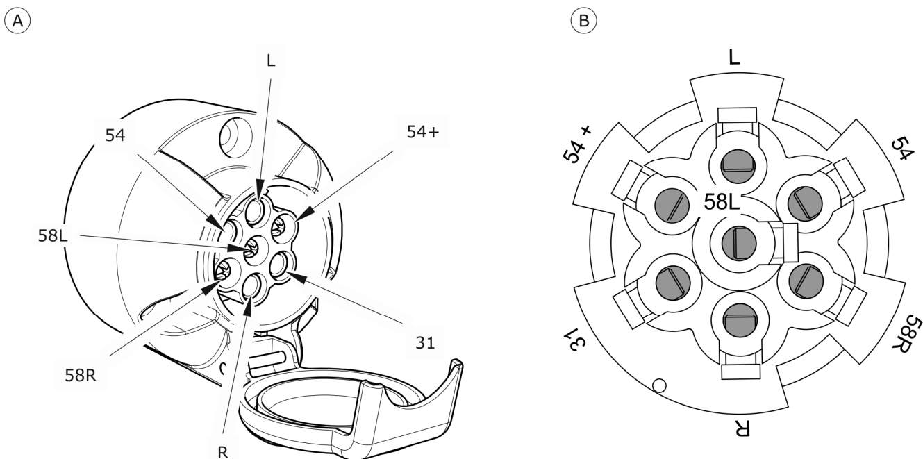
SLIKA 3.11 Priključna vtičnica
