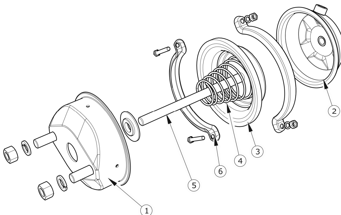
SLIKA 3.8 Konstrukcija pnevmatskega zavornega valja
