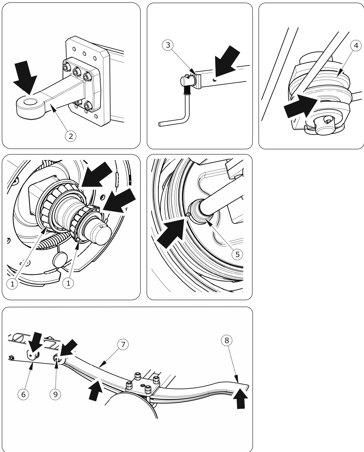
SLIKA 5.12 Mazalne točke na prikolici
