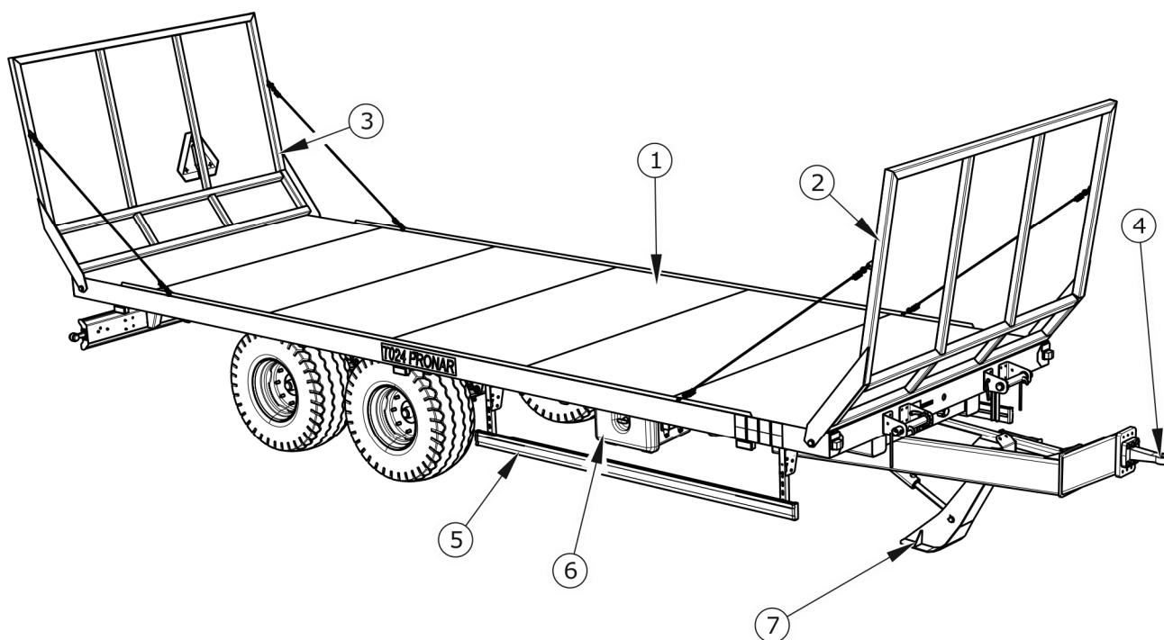
SLIKA 3.1 Konstrukcija prikolice
