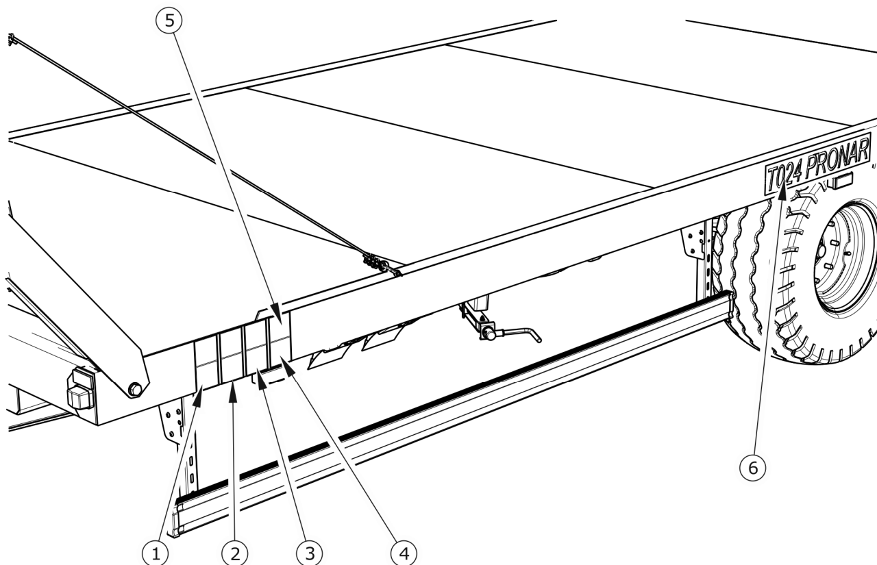
SLIKA 2.2 Razporeditev informativnih in opozorilnih nalepk
