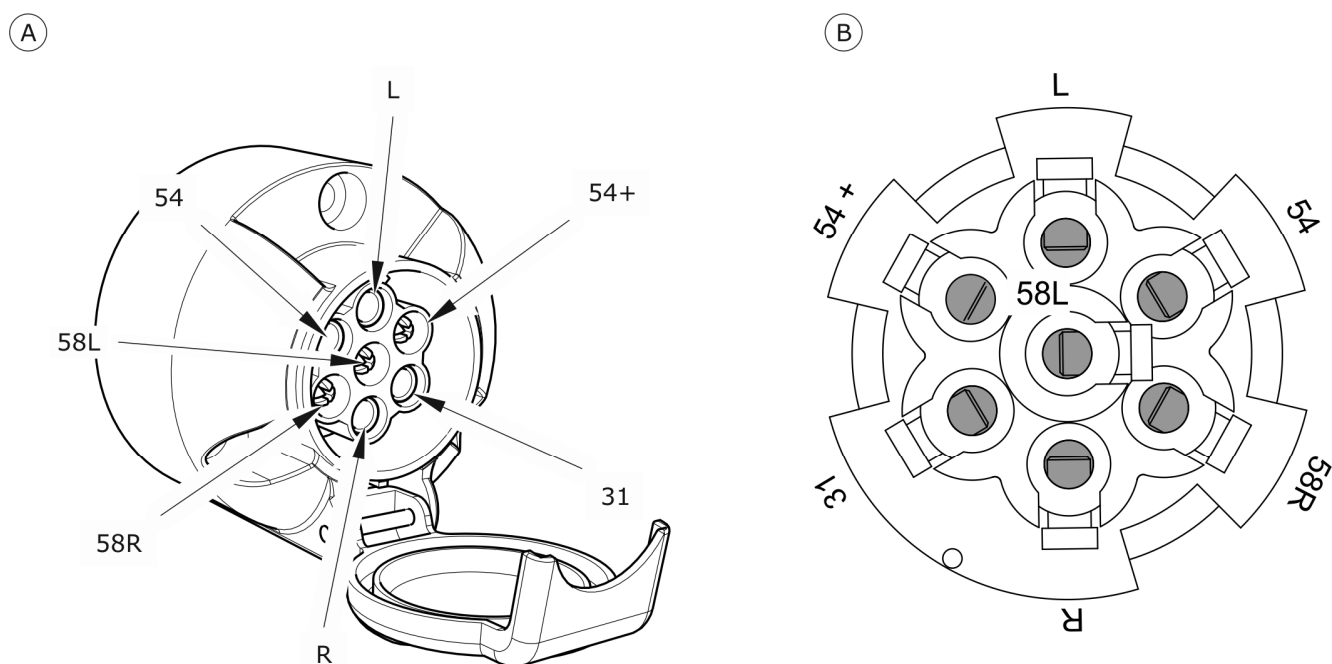
SLIKA 3.11 Priključna vtičnica
