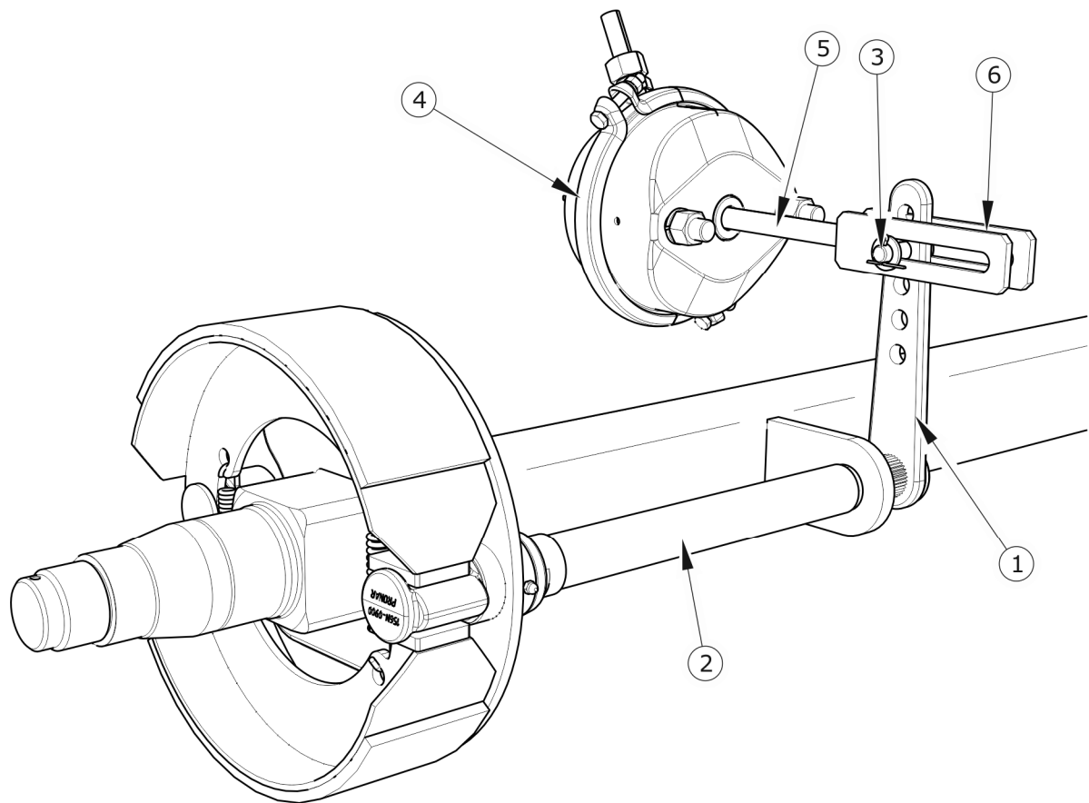
SLIKA 5.7 Konstrukcija zavore pogonske osi
