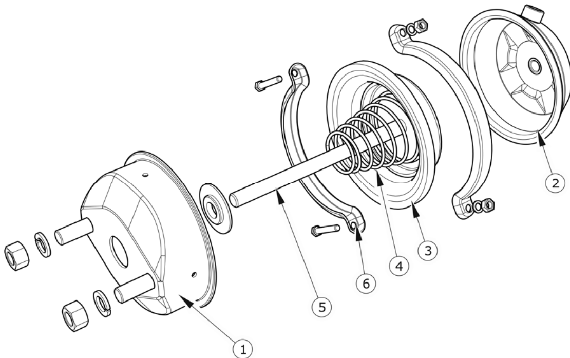
RYSUNEK 3.8 Budowa siłownika pneumatycznego
