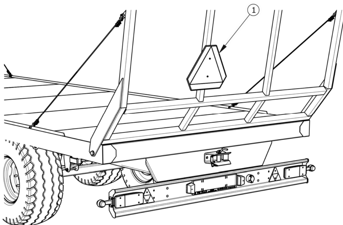
RYSUNEK 2.1 Miejsce montażu tablicy
