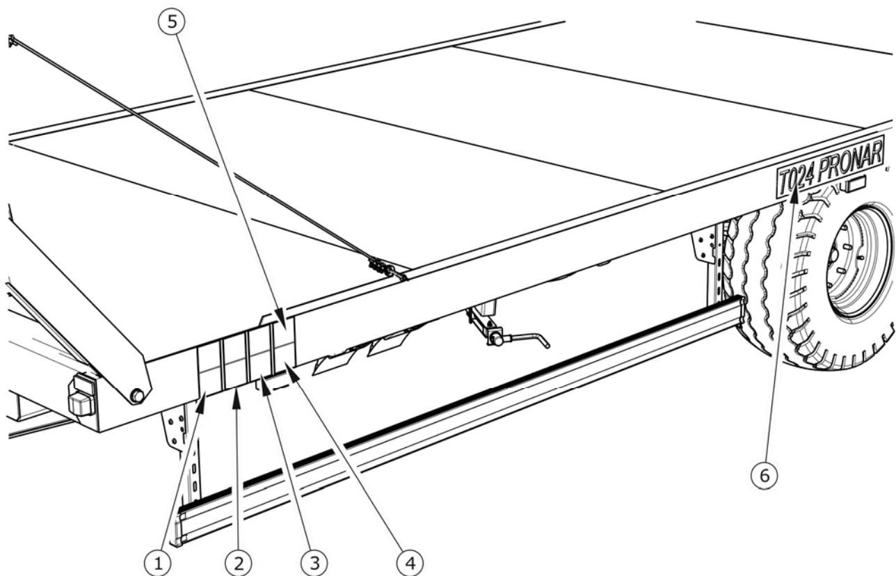
RYСУNEK 2.2 Rozmieszczenie naklejek informacyjnych i ostrzegawczych
