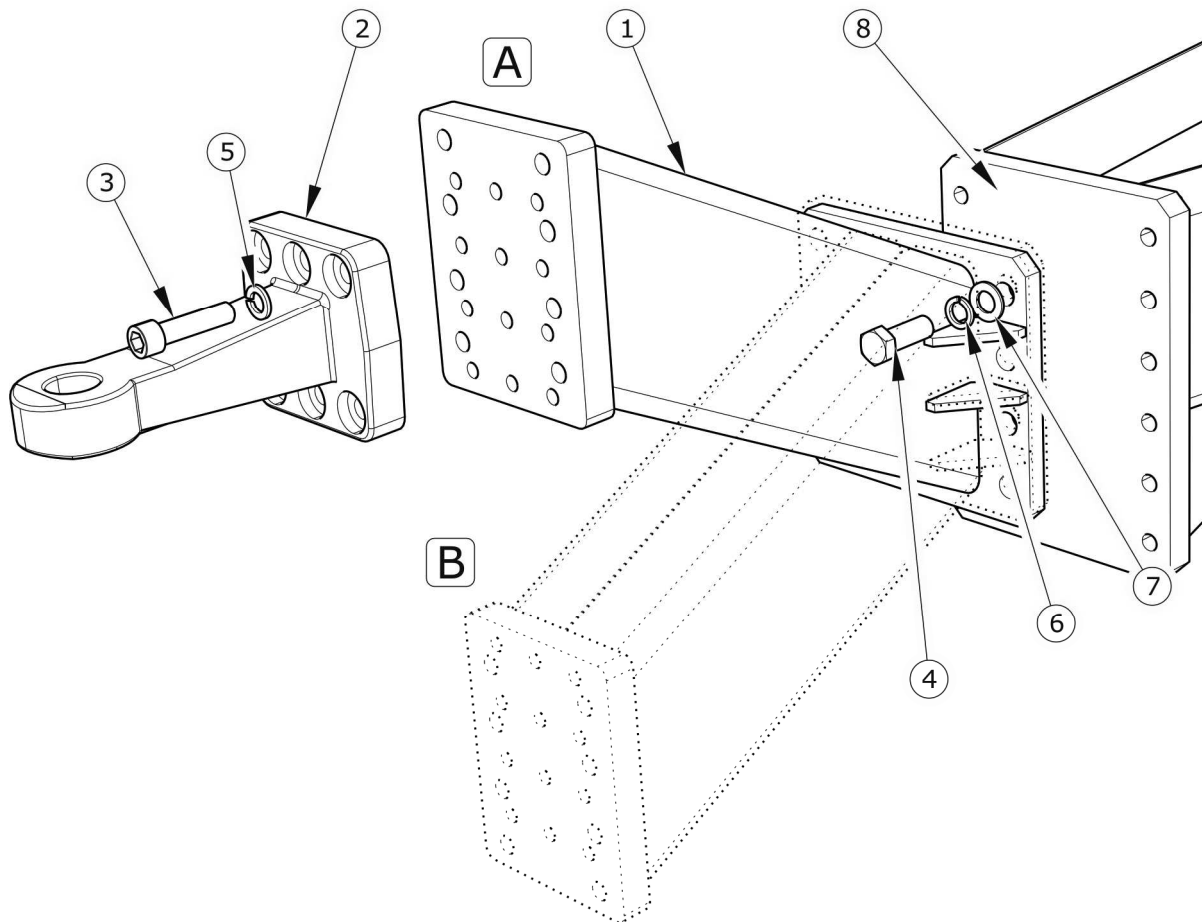
Obrázek 5.14 Regulace polohy oje
