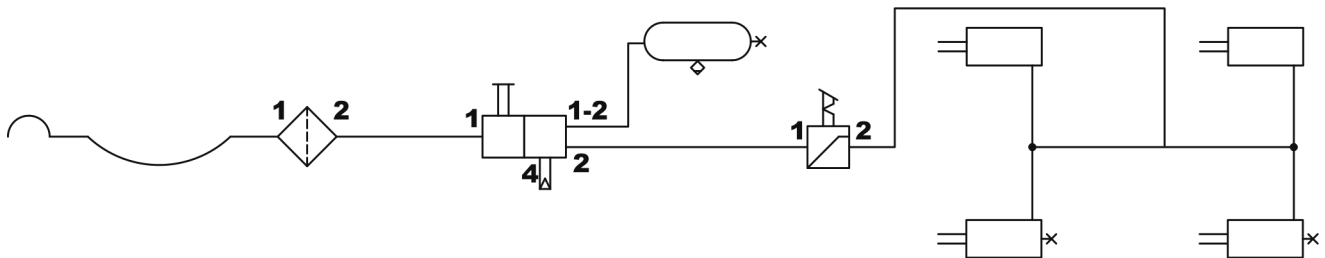
Obrázek 3.5 Schéma vzduchové dvouhadicové instalace s automatickým regulátorem
