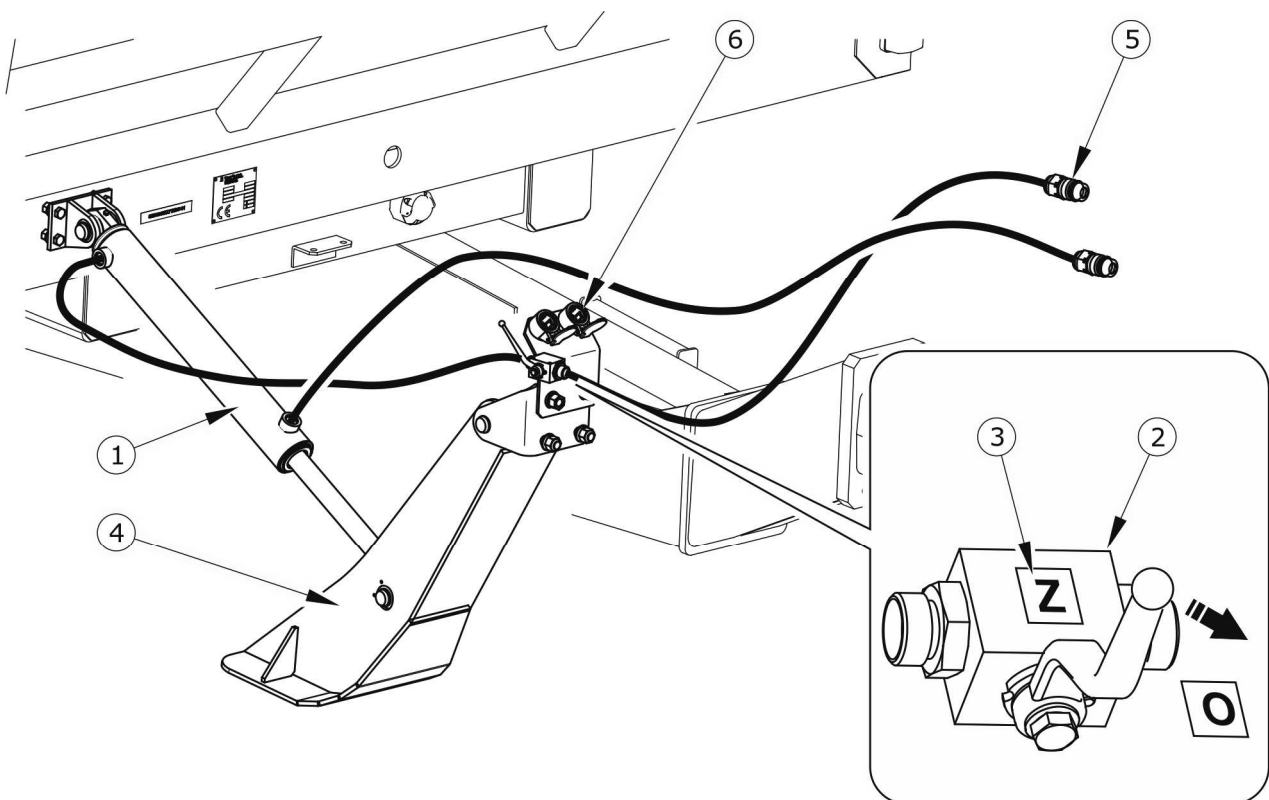
Obrázek 3.12 Konstrukce instalace hydraulické podpěry
