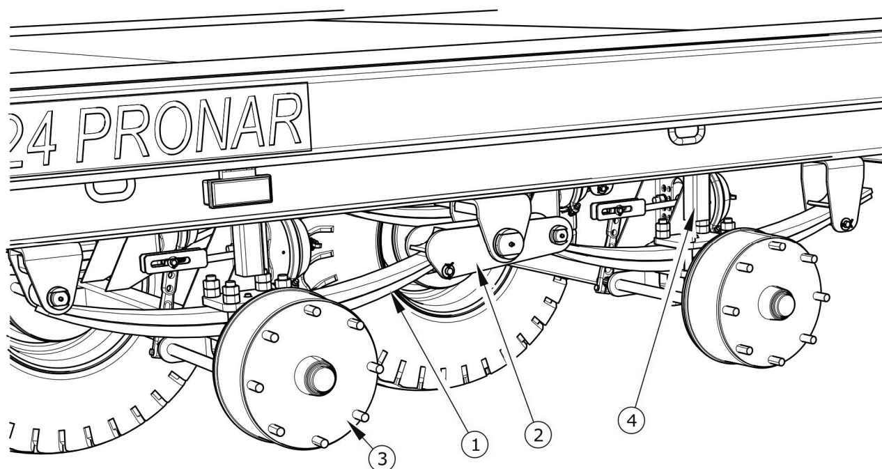
Obrázek 3.2 Zadní pérování
