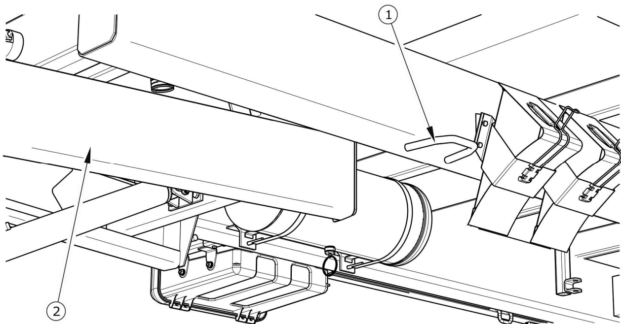
Obrázek 1.3 Přepravní držáky
