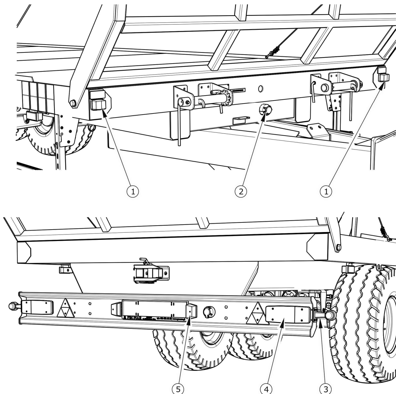
Obrázek 3.10 Rozmístění prvků elektroinstalace
