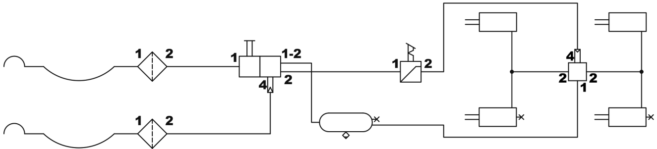
Obrázek 3.4 Schéma vzduchové dvouhadicové instalace s ručním regulátorem
