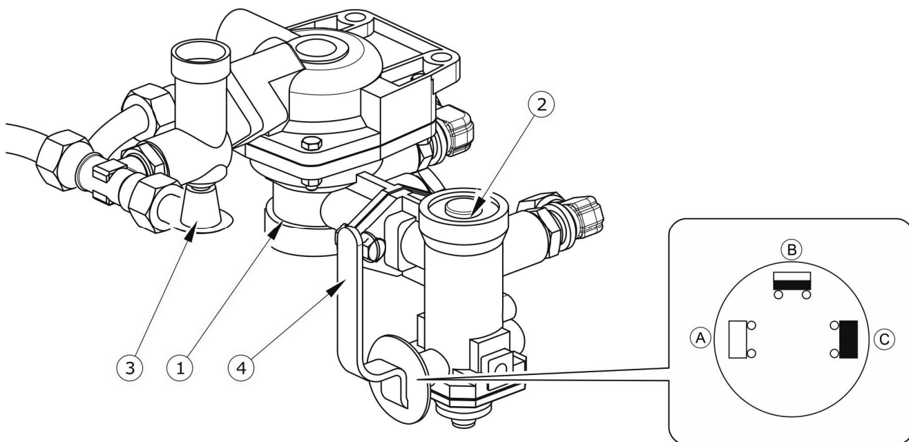
Obrázek 3.9 Ovládací ventil a regulátor brzdné síly
