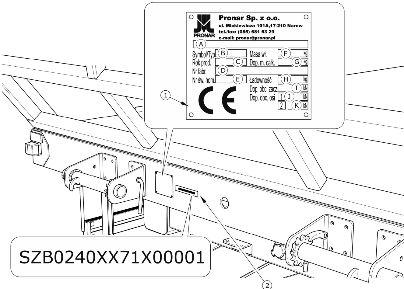
Obrázek 1.1 Místo umístění údajového štítku a vyražení VIN čísla
