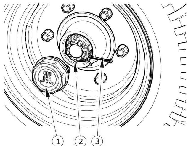
Obrázek 5.3 Seřízení vůle
