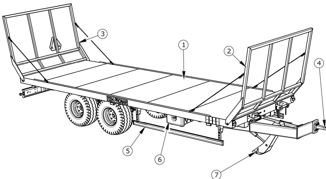
Obrázek 3.1 Konstrukce přívěsu
