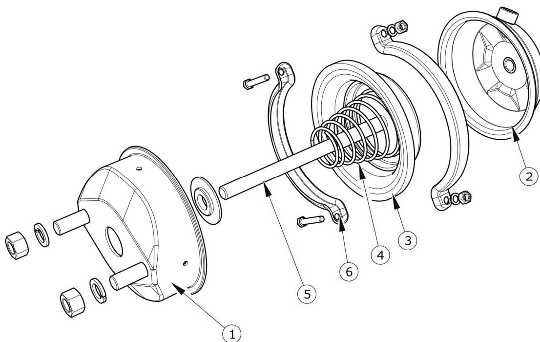
Obrázek 3.8 Konstrukce pneumatického válce
