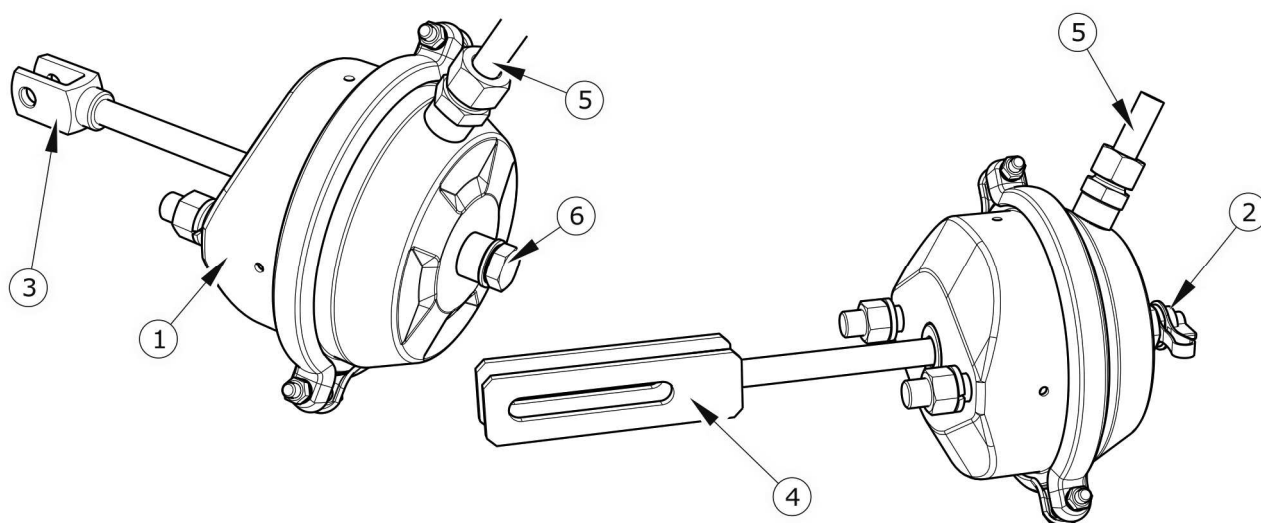
Obrázek 3.7 Brzdové pneumatické válce
