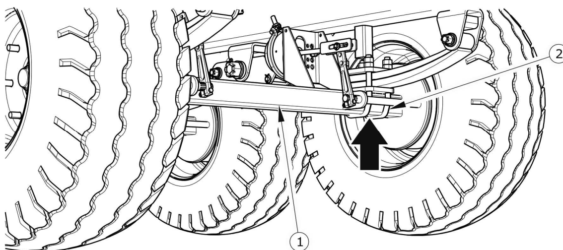
Obrázek 5.1 Podpěrný bod zvedáku
