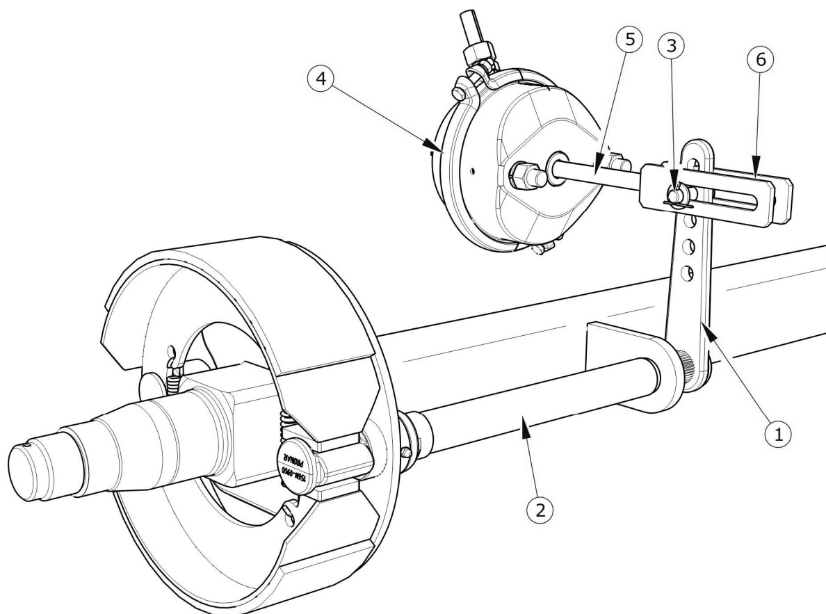
Obrázek 5.7 Stavba brzdý hnací nápravy
