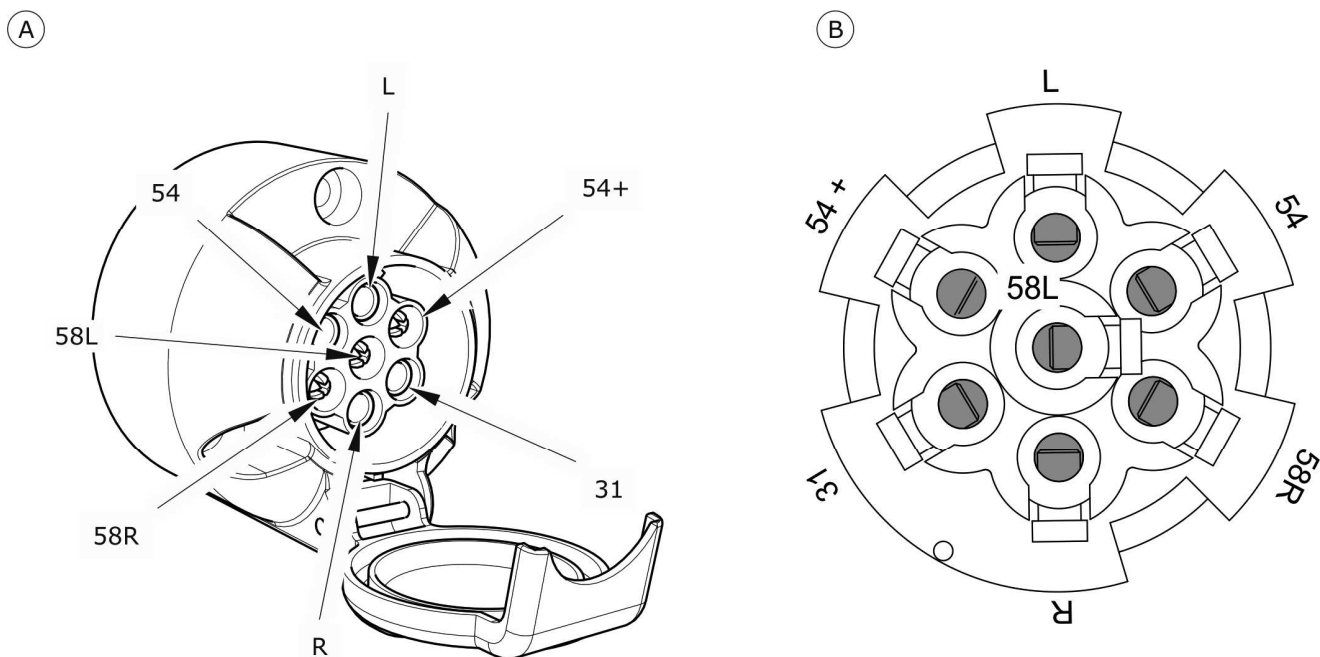
Obrázek 3.11 Připojovací zásuvka
