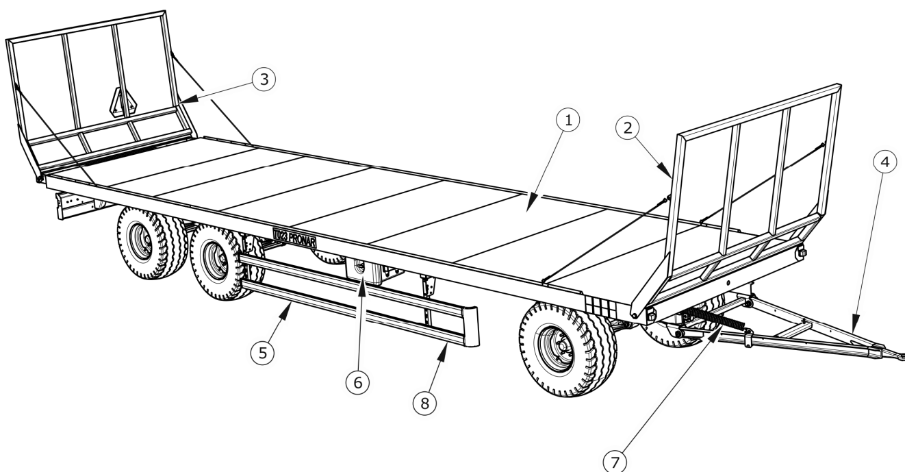
AFB. 3.1 Constructie van de aanhanger
