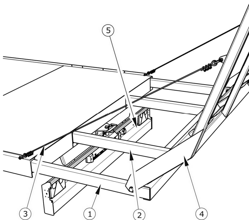
Obrázek 3.2 Výsuvný rám
