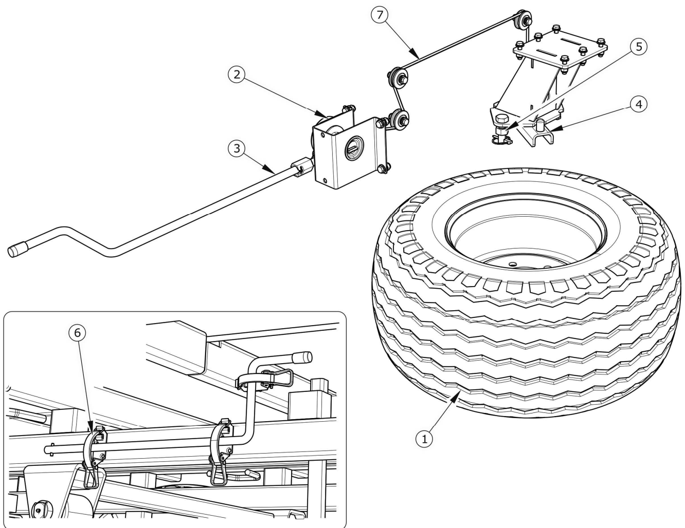
Obrázek 3.16 Konstrukce navijáku náhradního kola
