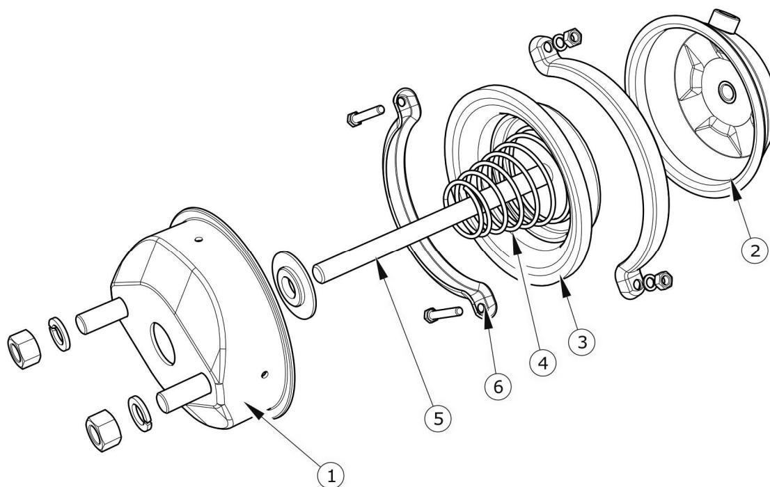
Obrázek 3.12 Konstrukce membranového válce
