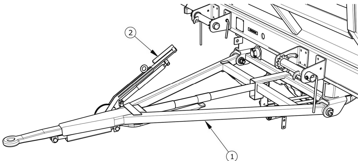
Obrázek 3.5 Nájezdová oj
