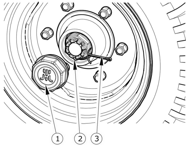
Obrázek 5.3 Seřízení vůle
