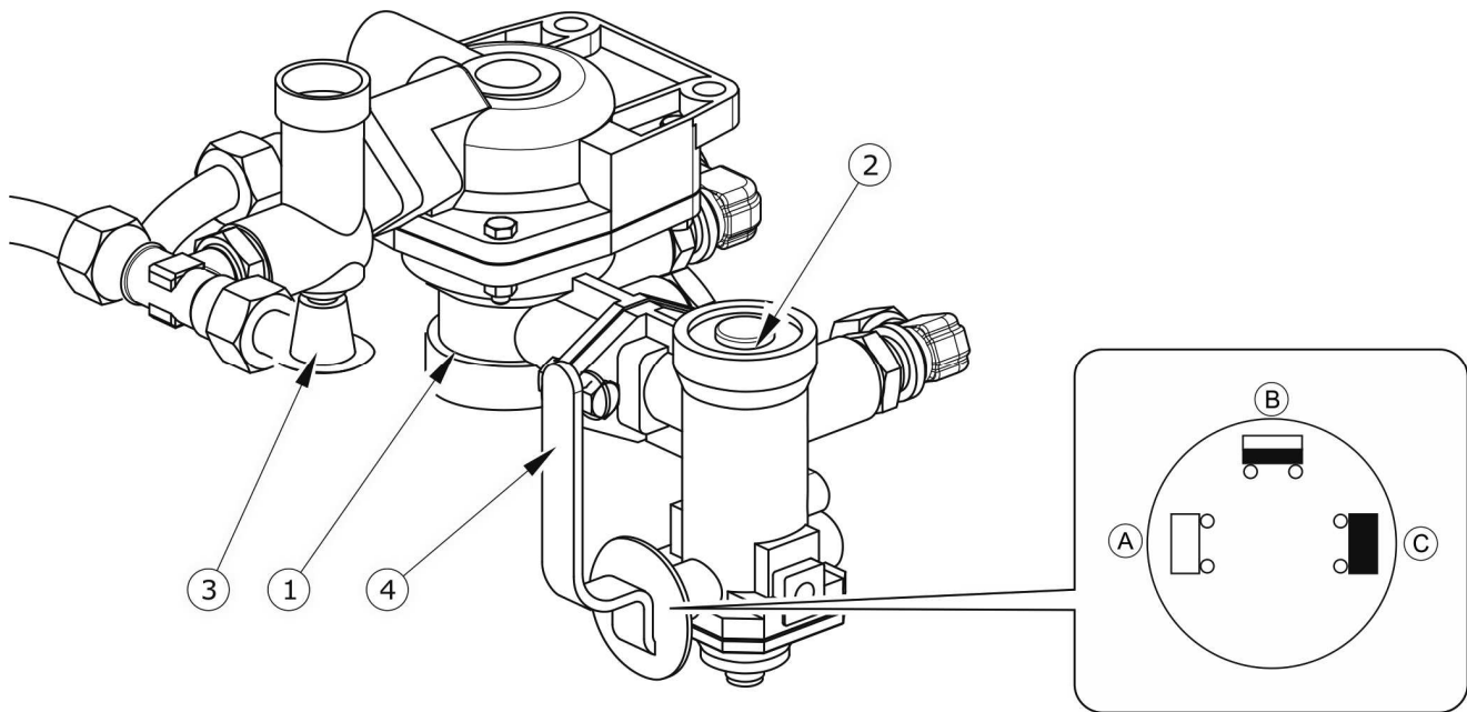
Obrázek 3.13 Ovládací ventil a regulátor brzdné síly
