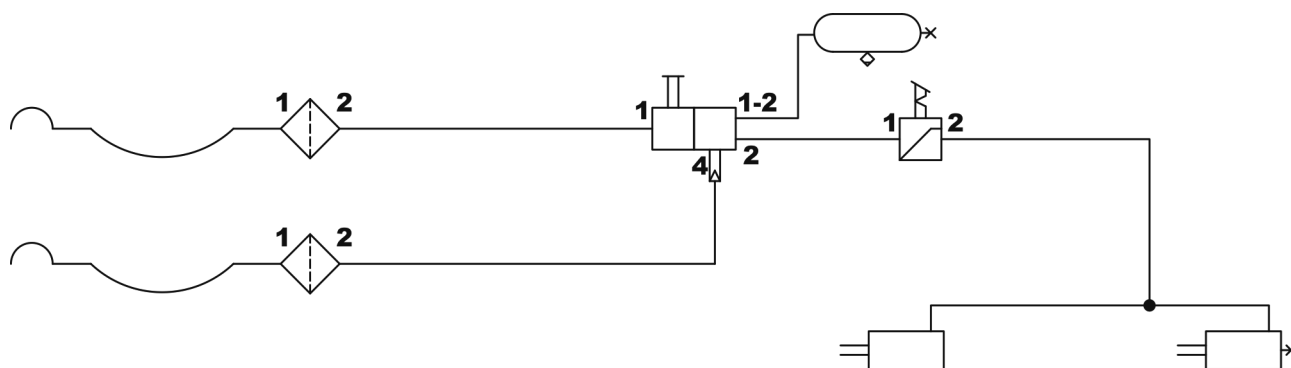
Obrázek 3.7 Schéma vzduchové dvouhadicové instalace s ručním regulátorem
