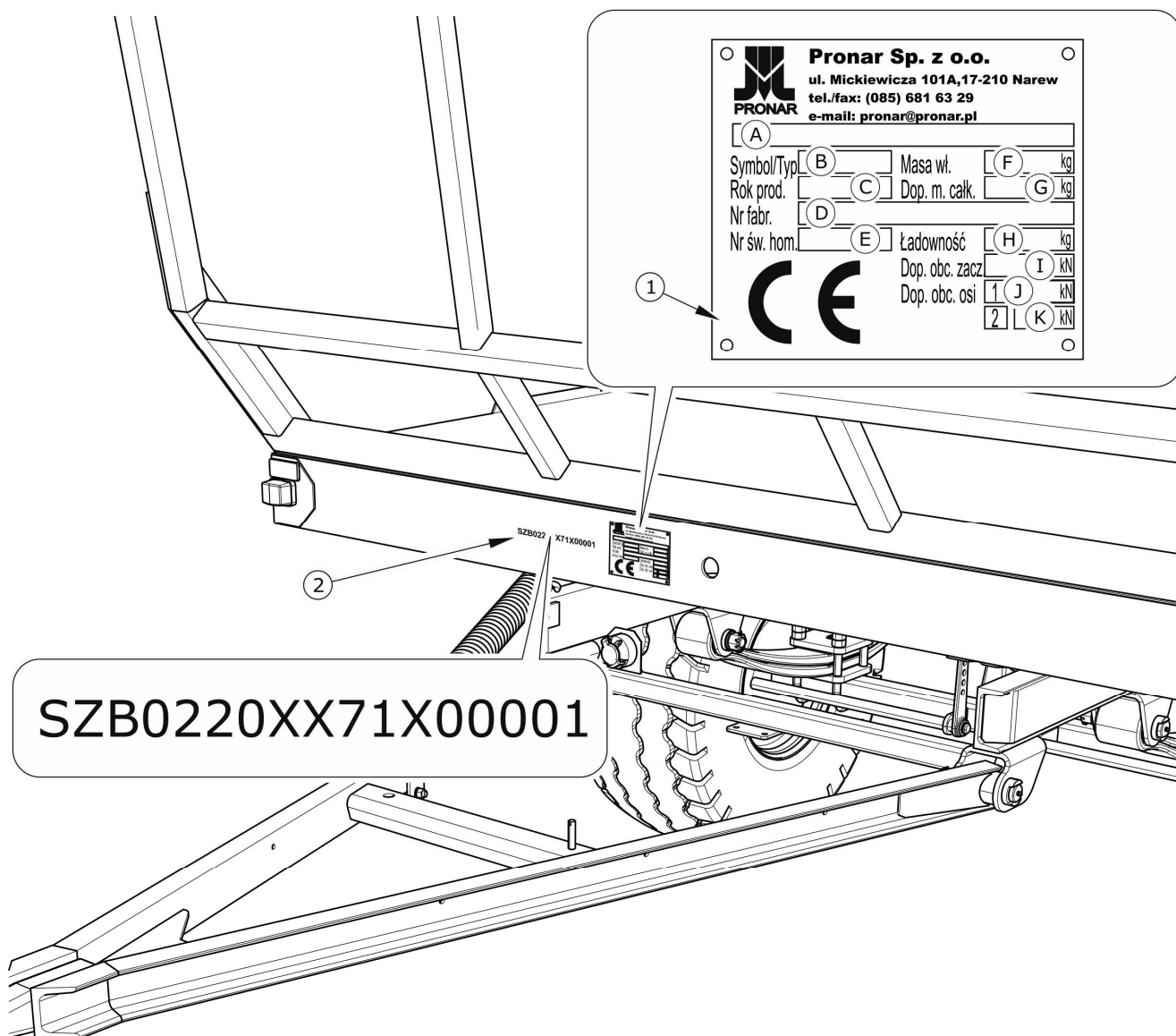
Obrázek 1.1 Místo umístění údajového štítku a vyznačení VIN čísla
