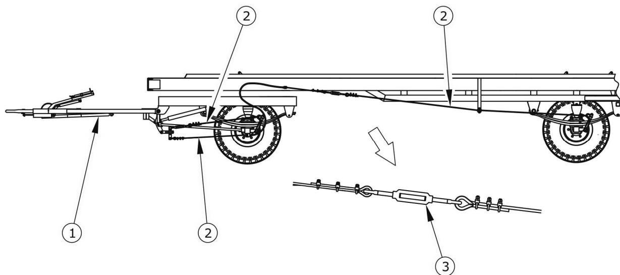
Obrázek 5.10 Regulace nájezdové brzdy
