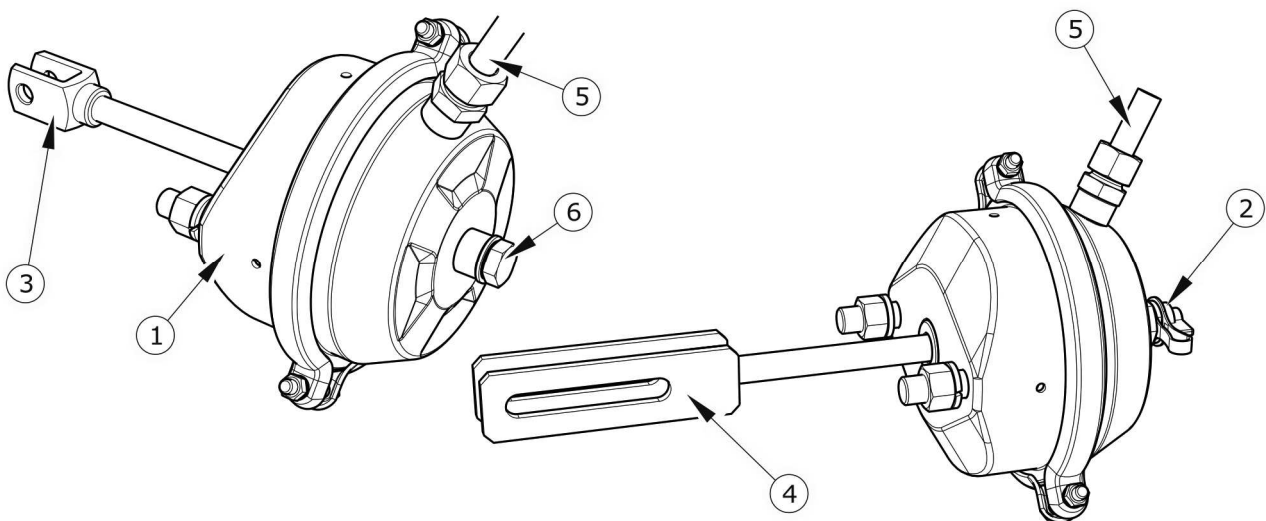
Obrázek 3.11 Brzdové pneumatické válce
