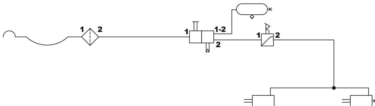
Obrázek 3.9 Schéma vzduchové jednohadicové instalace s ručním regulátorem
