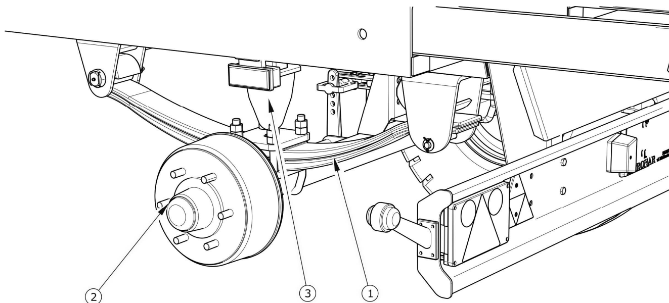
Obrázek 3.3 Zadní pérování
