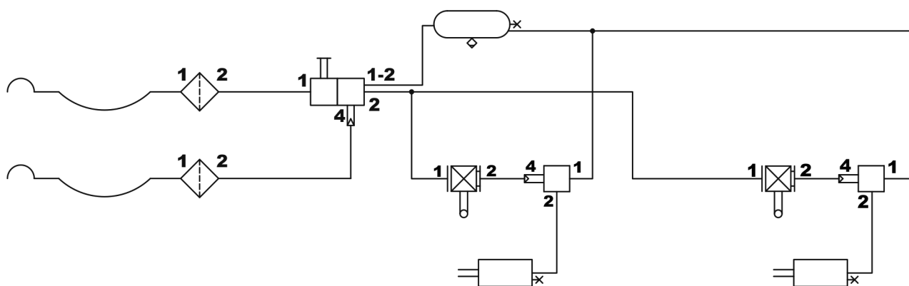
Obrázek 3.8 Schéma vzduchové dvouhadicové instalace s automatickým regulátorem
