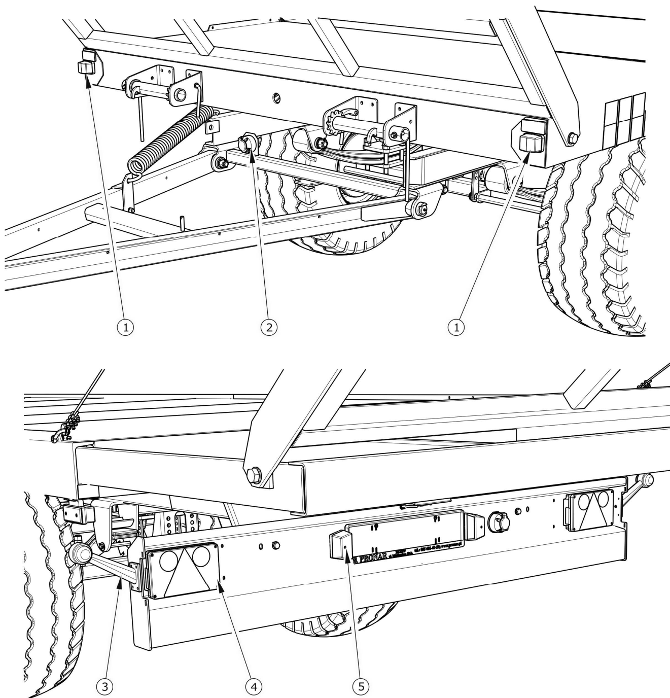
Obrázek 3.14 Rozmístění prvků elektroinstalace
