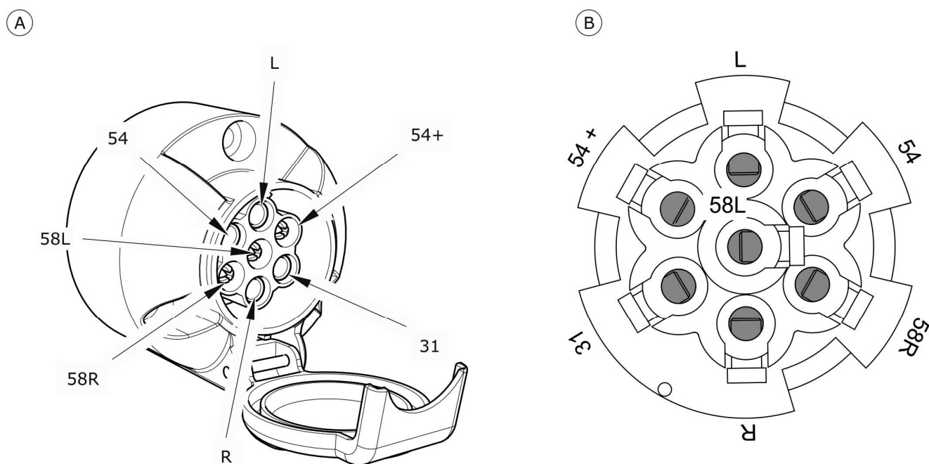
Obrázek 3.15 Připojovací zásuvka
