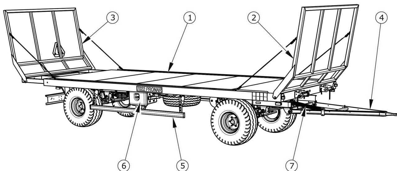
Obrázek 3.1 Konstrukce přívěsu
