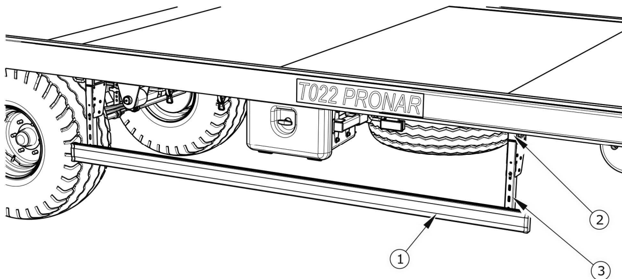
Obrázek 3.6 Boční nájezdové zábrany
