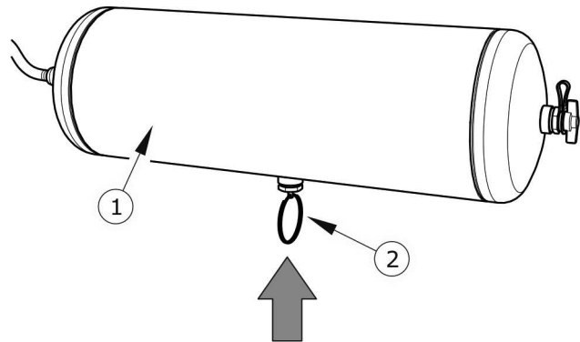
Obrázek 5.12 Odvodňování vzdušníku
