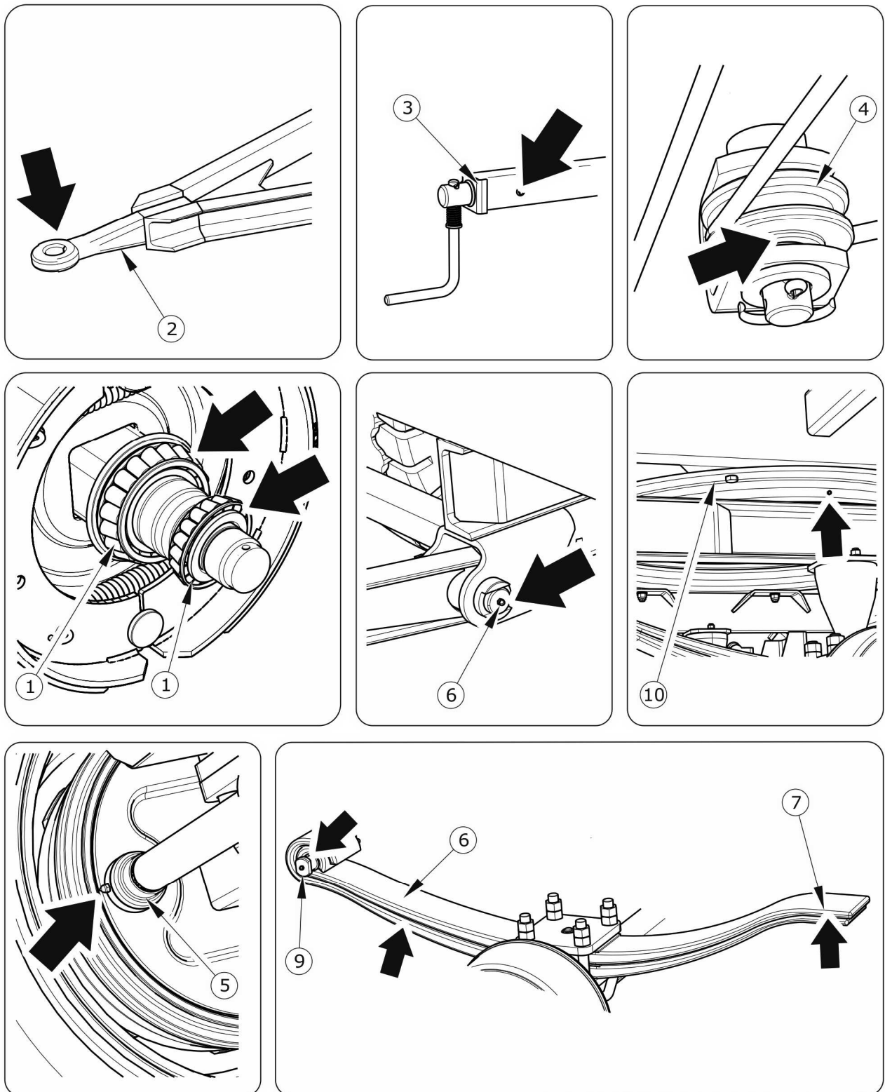
Obrázek 5.13 Mazací místa přívěsu
