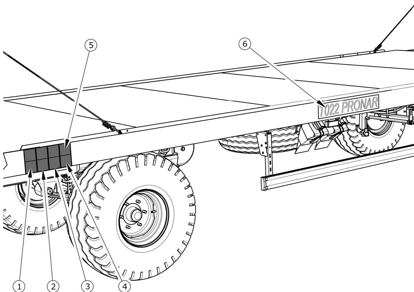
RYSUNEK 2.1 Rozmístění informačních a výstražných nálepek
