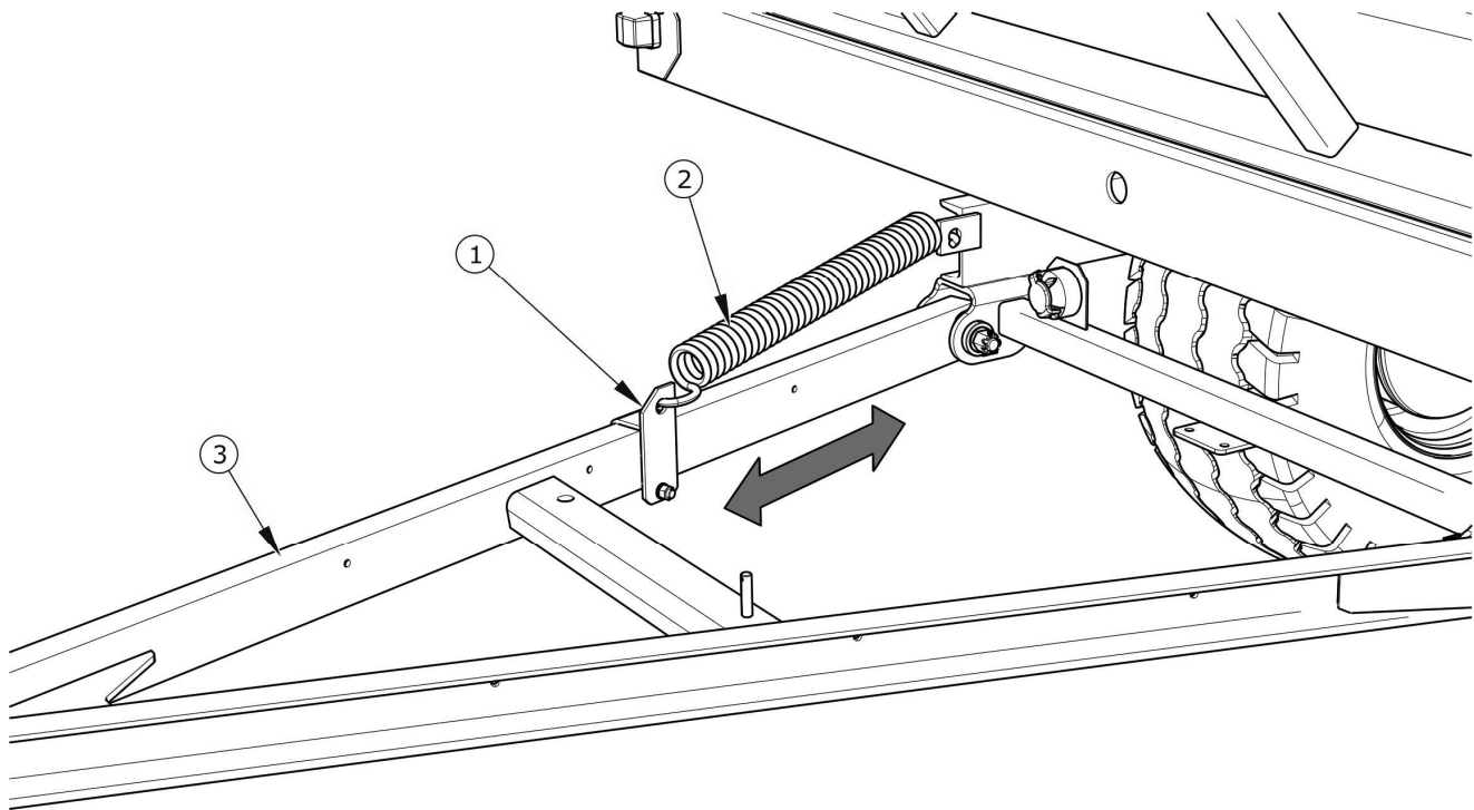
Obrázek 5.15 Regulace polohy oje
