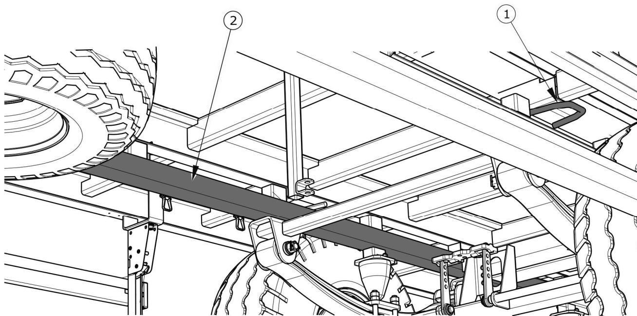
Obrázek 1.3 Převravní držáky
