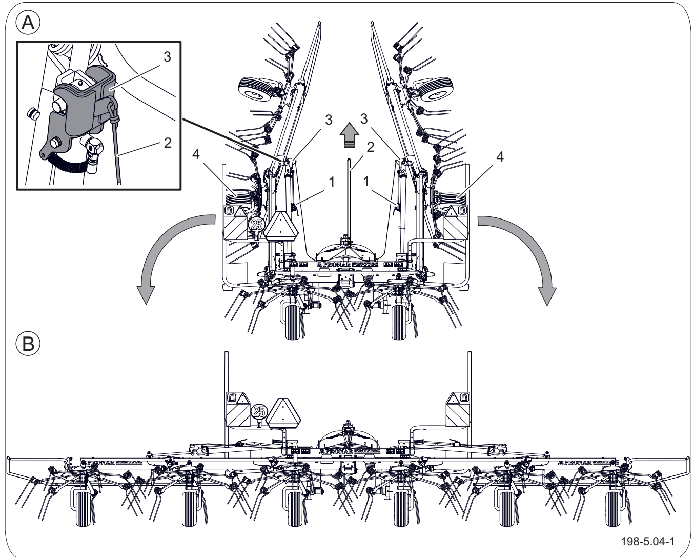
Rysunek 5.8 Pzycje przetrząsacza
