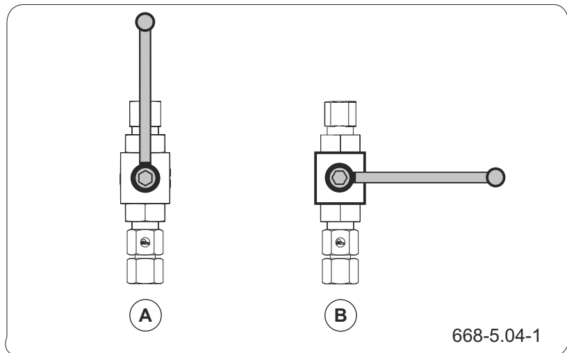
Rysunek 5.17 Zawór kulowy
