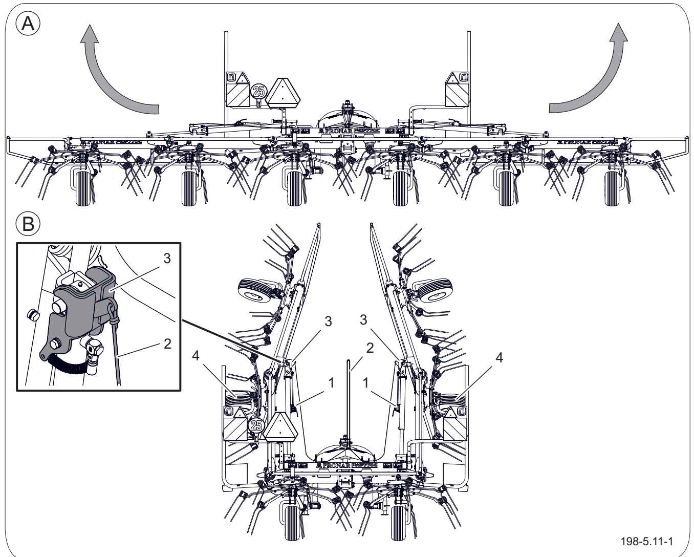
Rysunek 5.15 Pozycje przetrząsacza
