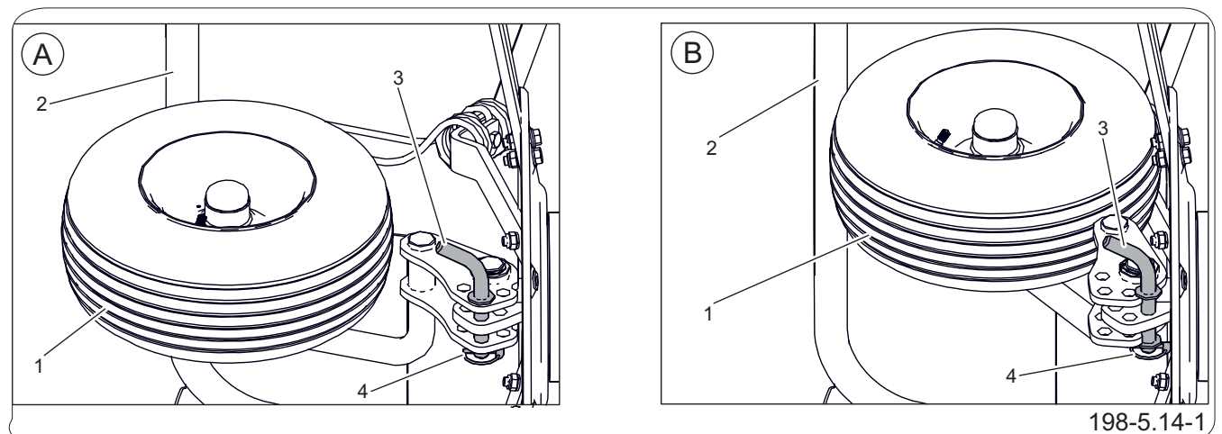
Rysunek 5.16 Ustawienie kół jezdnych
