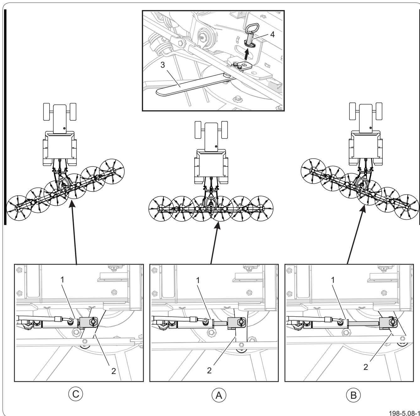
Rysunek 5.14 Przetrzęsanie graniczne - sterowanie hydrauliczne (wyposażenie opcjonalne) (1) siłownik hydrauliczny (2) dźwignia regulacji hydraulicznej (3) dźwignia regulacji mechanicznej (4) sworzeń blokujący z zawleczką (A) przetrzęsanie na środek (B) przetrzęsanie prawą stroną (C) przetrzęsanie lewą stroną
