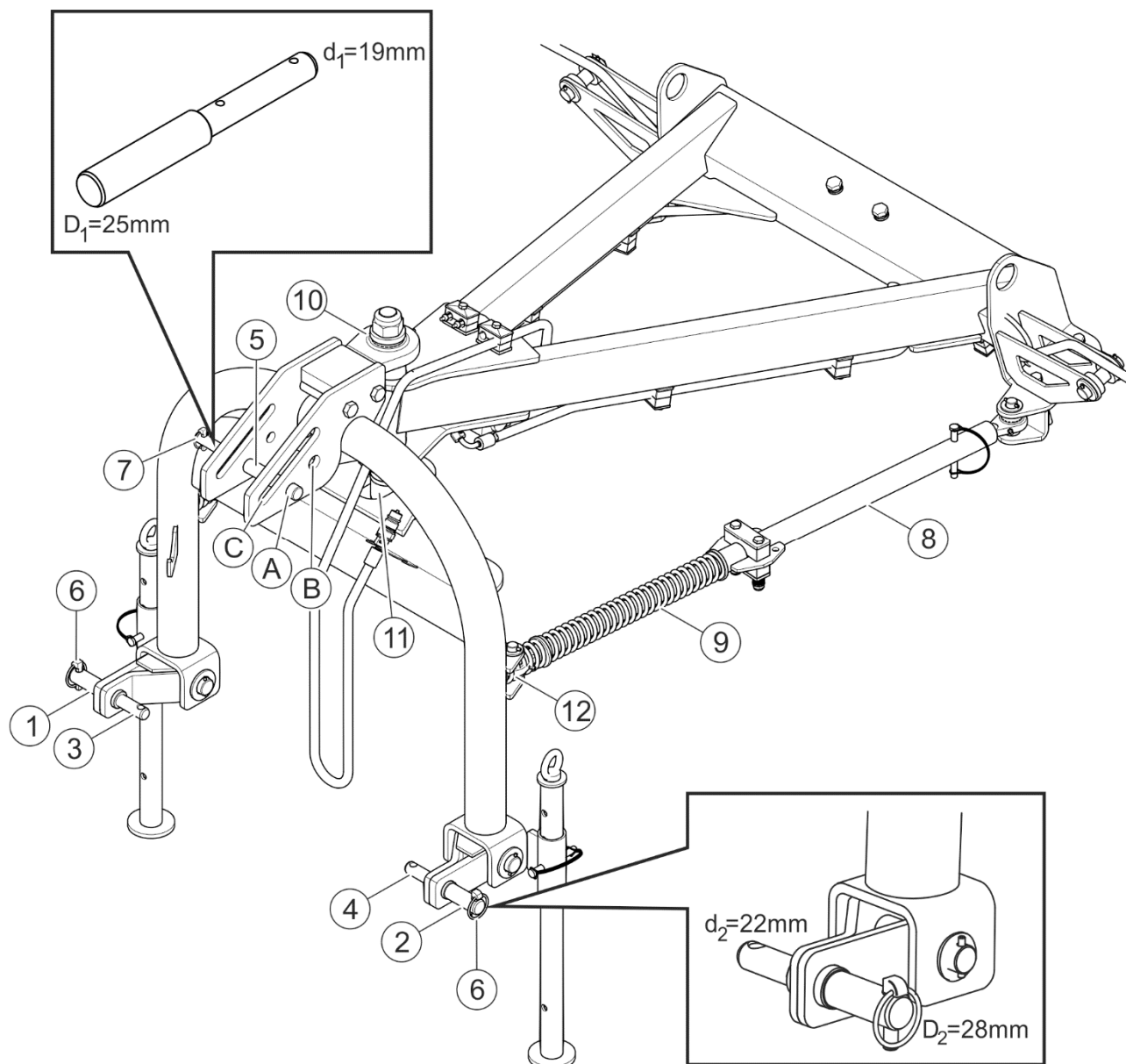
РИСУНОК 3.2 Система навески
