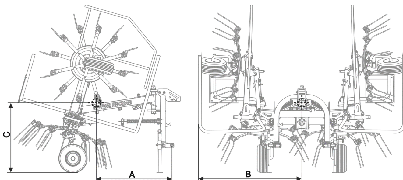
РИСУНОК 1.3 Расположение центра тяжести ворошилки карусельного типа в транспортном положении.
