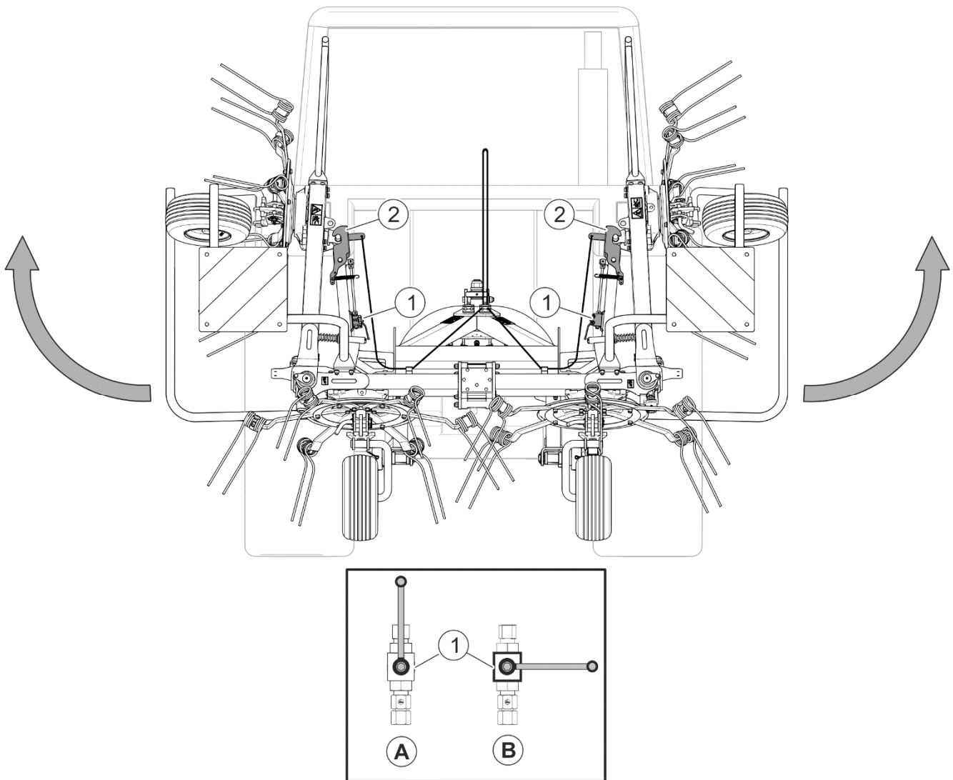
РИСУНОК 4.4 Установка ворошилки в транспортное положение.
