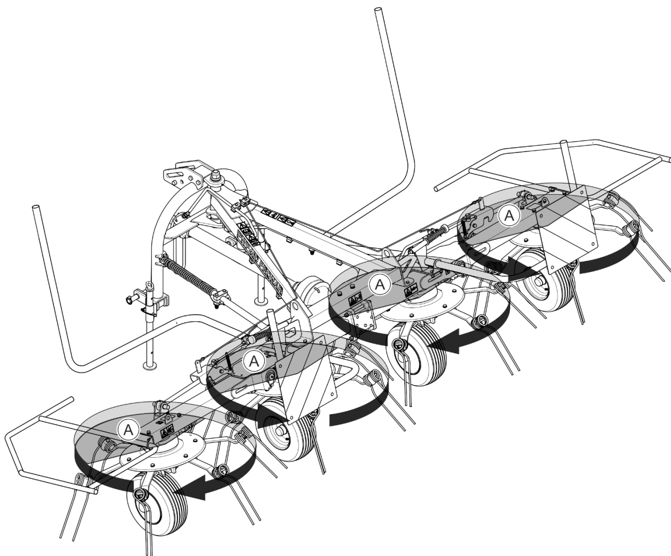
РИСУНОК 3.3 Принцип действия ворошилки
