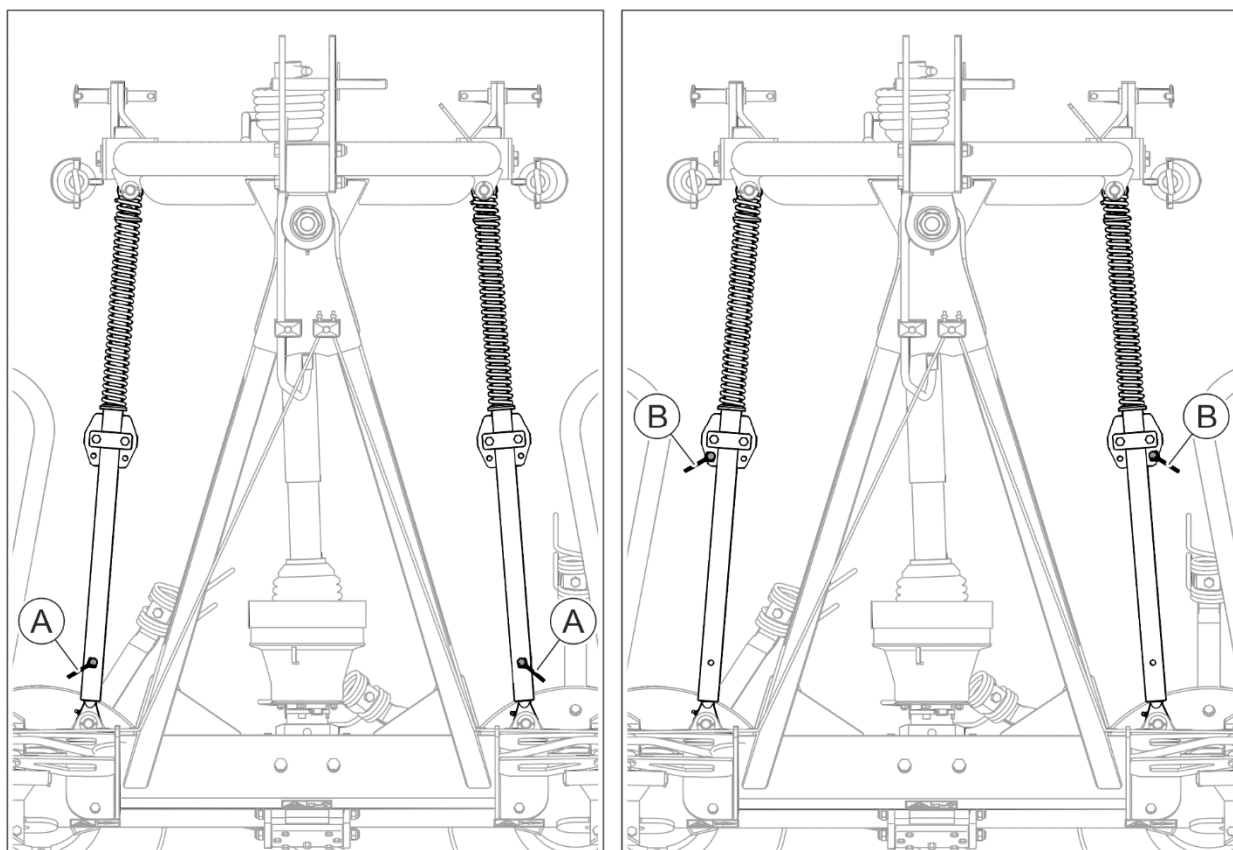
РИСУНОК 4.7 Установка амортизатора в рабочее положение.
