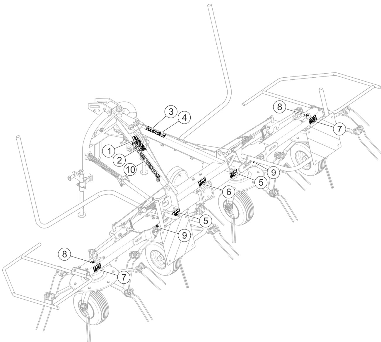
РИСУНОК 2.1 Размещение информационных и предупреждающих наклеек. Описание значений символов (ТАБЛИЦА 2.1)
