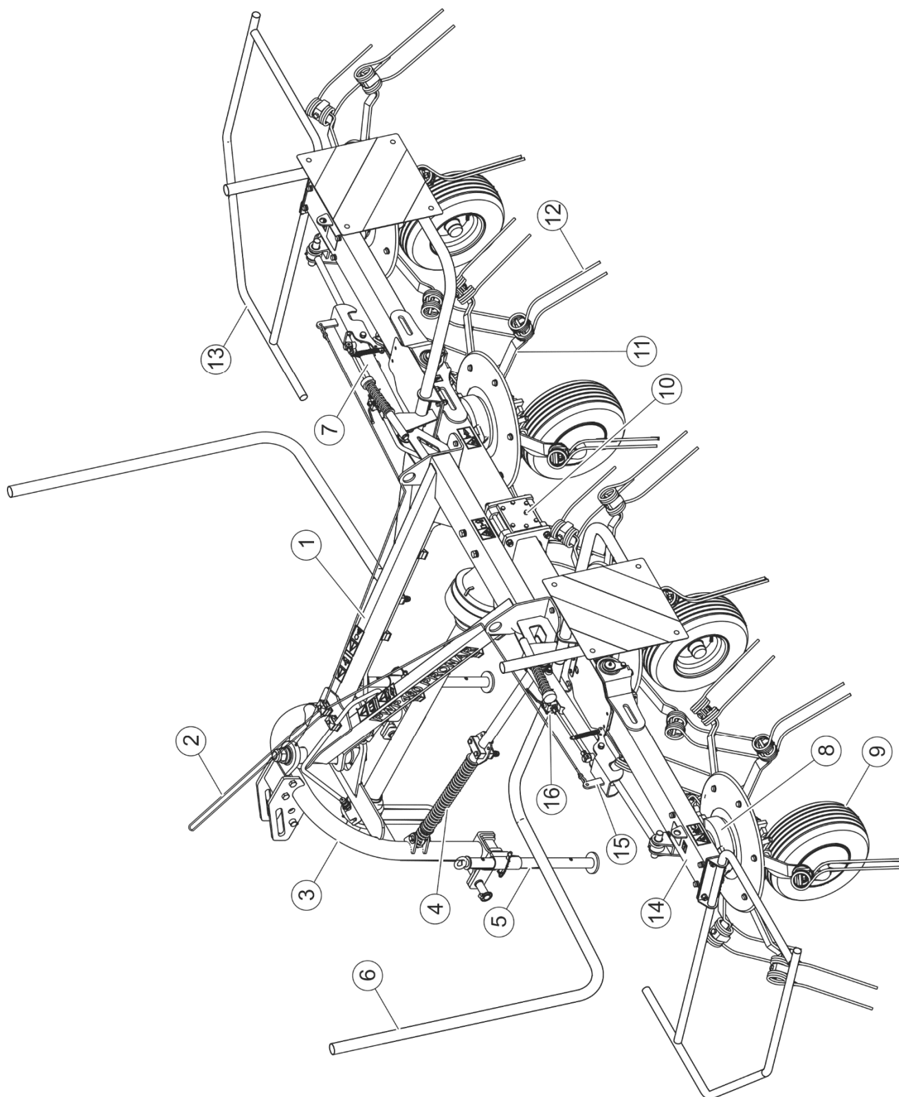
РИСУНОК 3.1 Общее устройство
