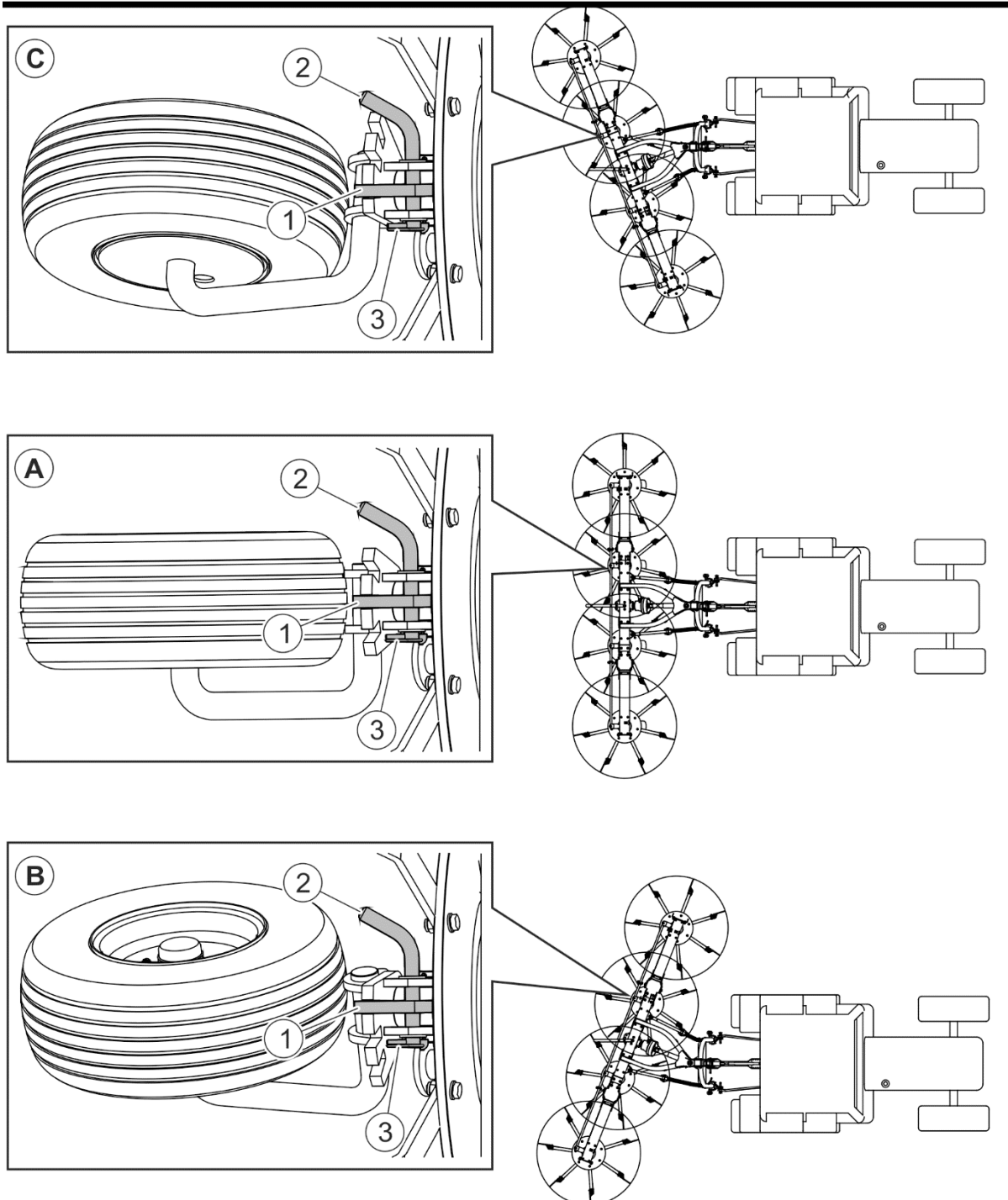
РИСУНОК 4.9 Работа ворошилкой – ворошение вдоль края поля
