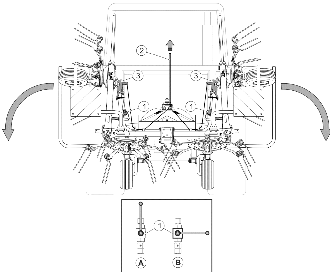
РИСУНОК 4.6 Установка ворошилки-вспушителя в рабочее положение
