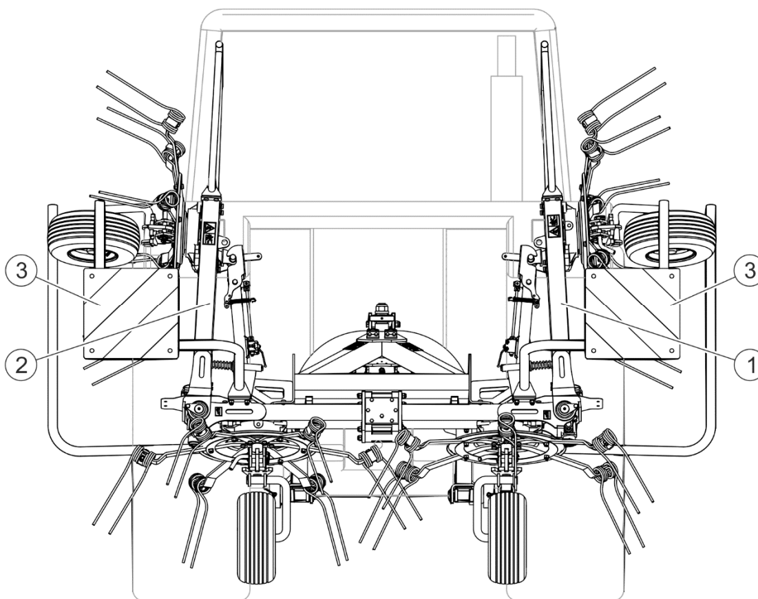
РИСУНОК 4.3 Транспортное положение ворошилки.
