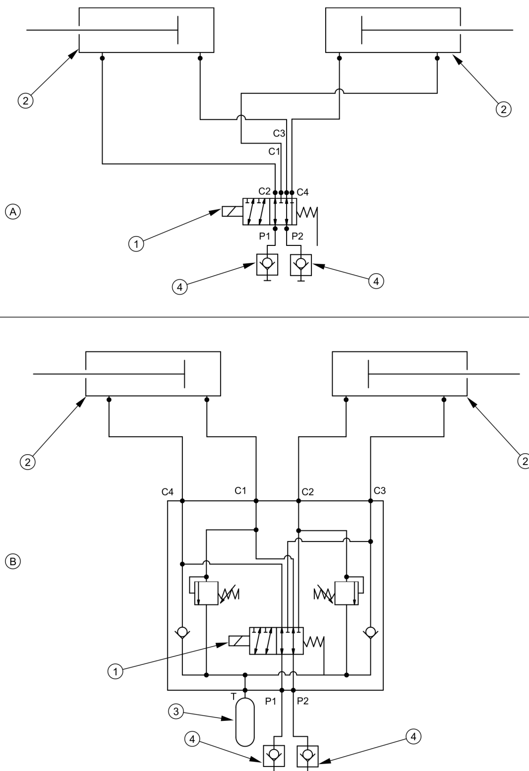
РИСУНОК 3.4 Принципиальная схема гидравлической системы
