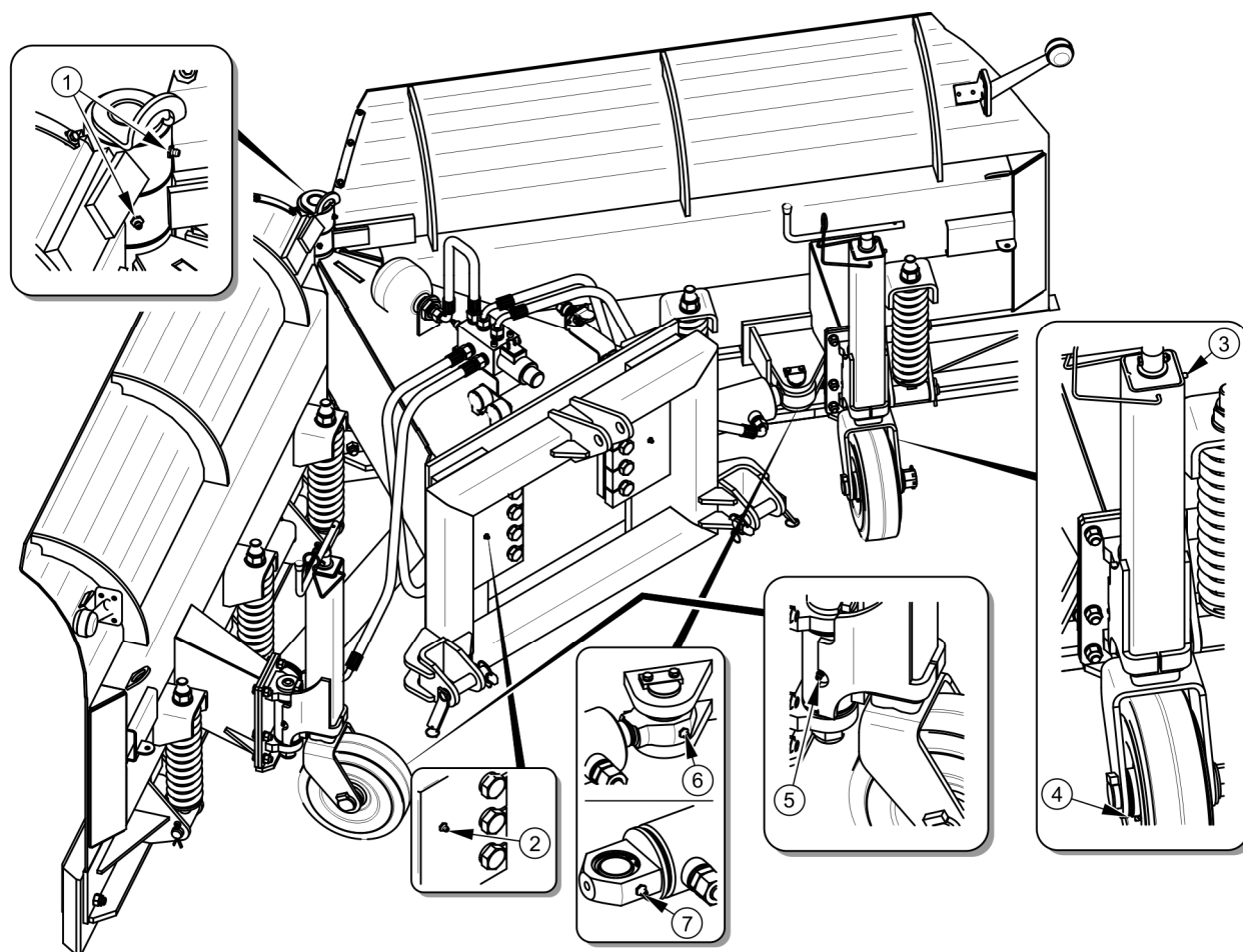
РИСУНОК 5.3 Точки смазки
