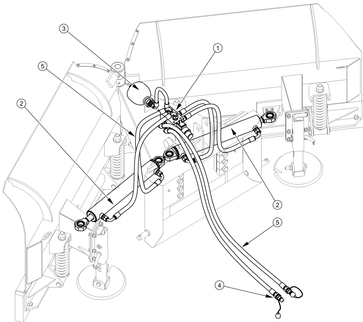
РИСУНОК 3.3 Элементы снегоотвала
