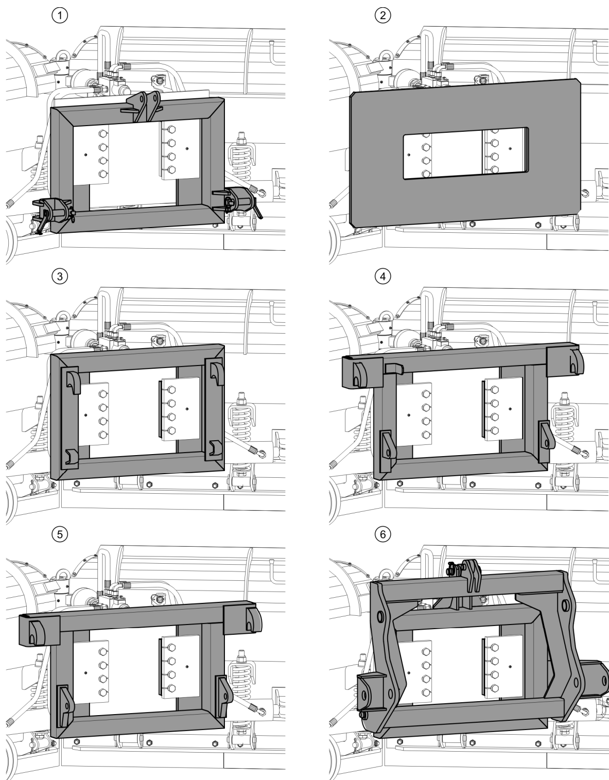
РИСУНОК 4.1 Типы навесных систем
