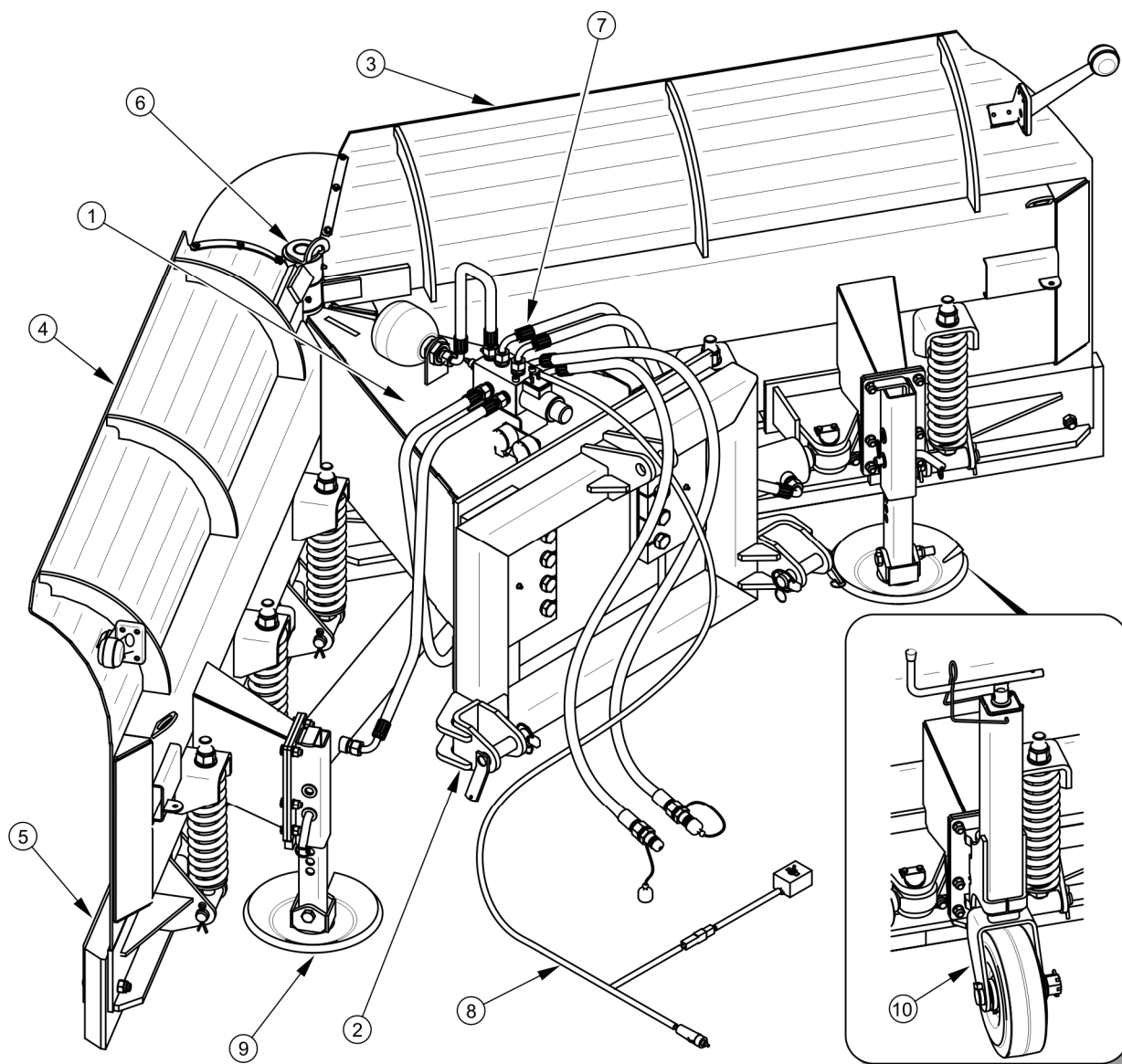
РИСУНОК 3.2 Элементы снегоотвала
