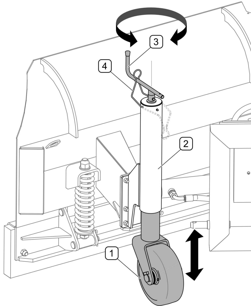
RYСУNEK 4.9 Regulacja wysokości pracy w pługach wyposażonych w kółka jezdne (1)- kółko; (2)- korpus; (3)- pokrętło; (4)- blokada pokrętła
