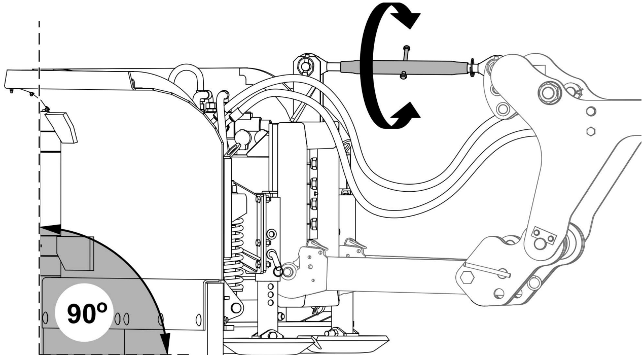
RYSUNEK 4.5 Poziomowanie korpusu pługa
