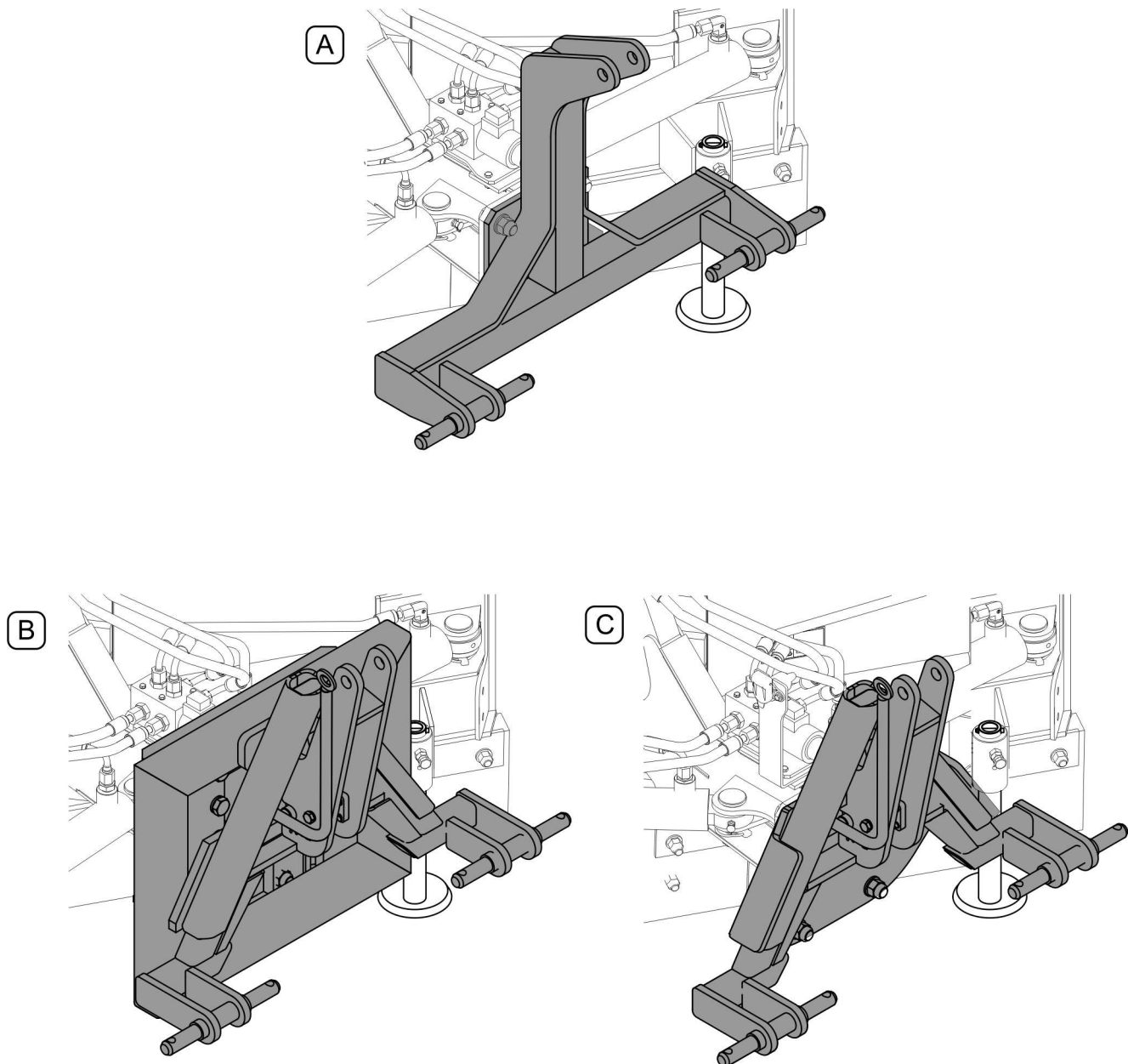
RYSUNEK 4.1 Rodzaje układów zawieszenia
