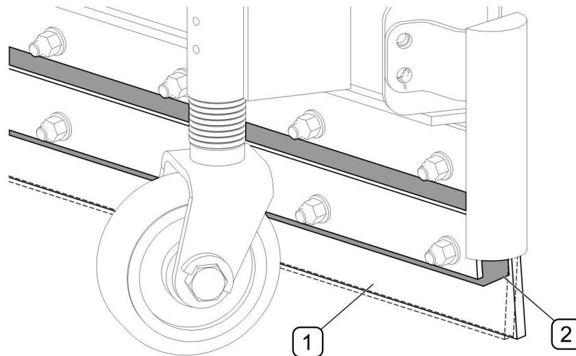
RYSUNEK 4.7 Amortyzacja listew zgarniających stalowych
