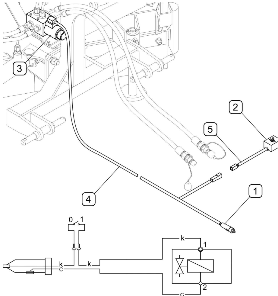
RYSUNEK 3.4 Budowa instalacji elektrycznej
