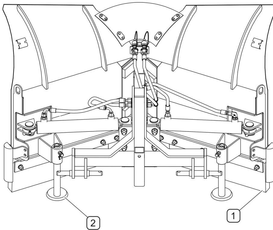
RYSUNEK 4.8 Pozycja pług po odłączeniu od nośnika
