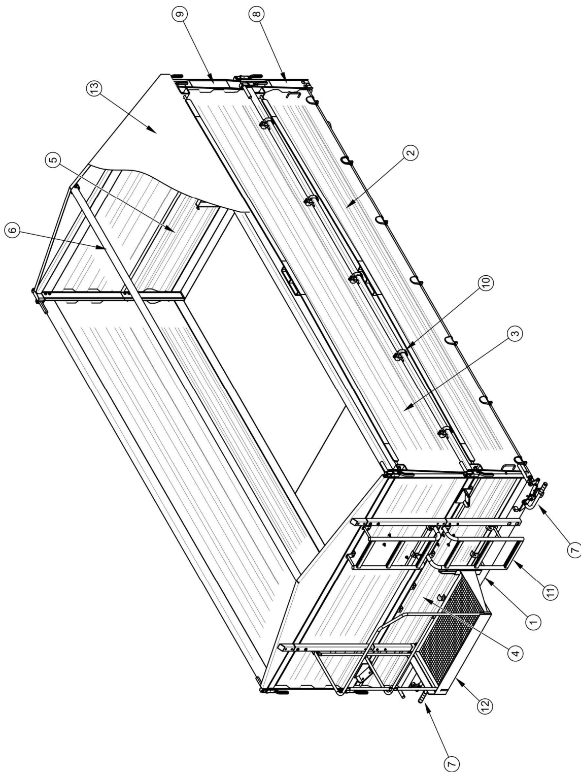
Obrázek 3.2 Korba
