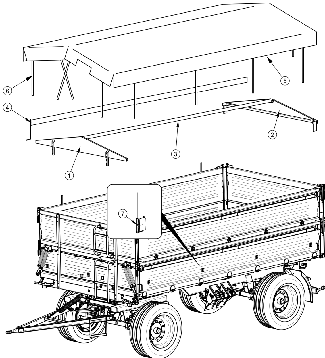
Obrázek 5.14 Podpěrná konstrukce s plachtou
