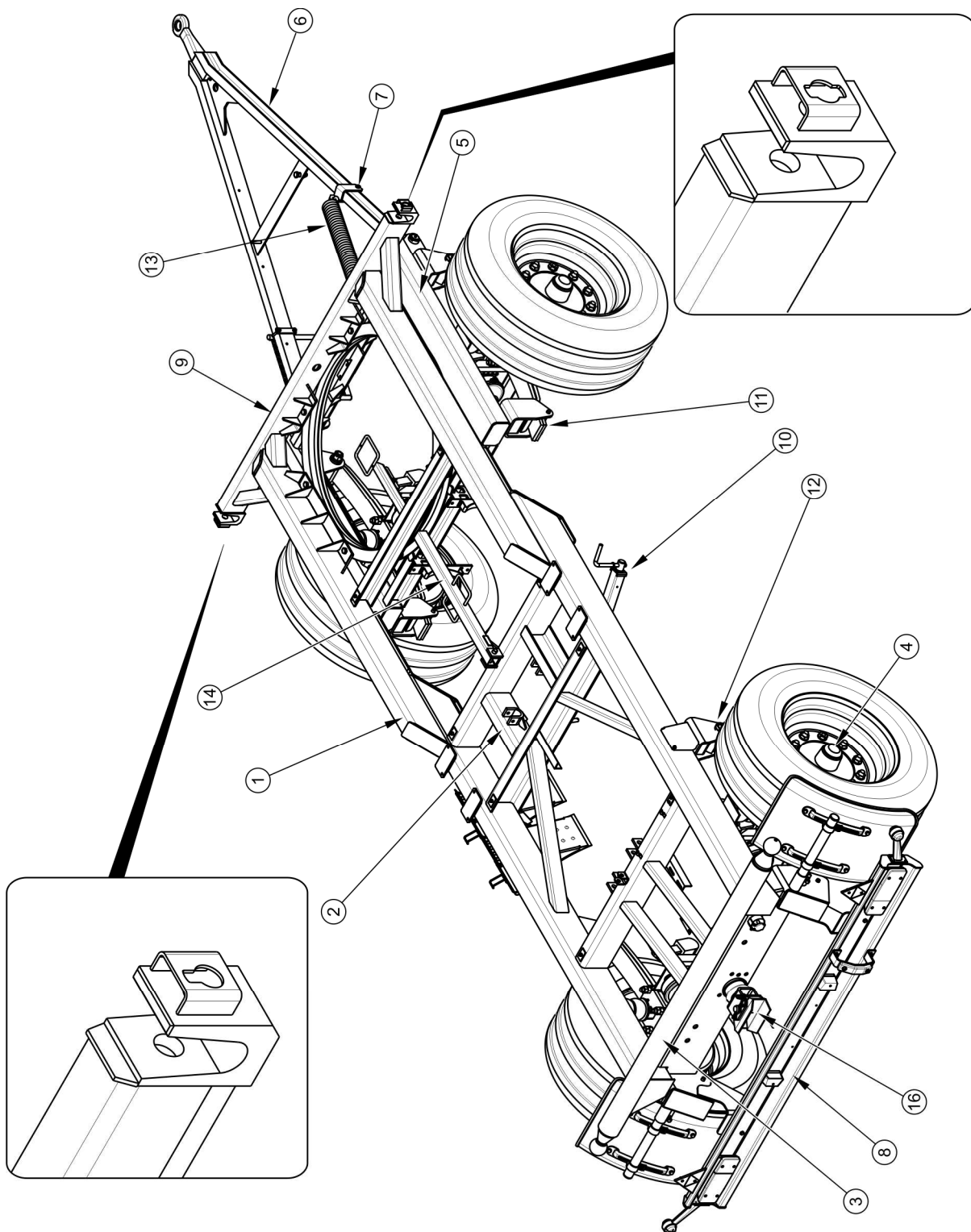
Obrázek 3.1 Podvozek přívěsu
