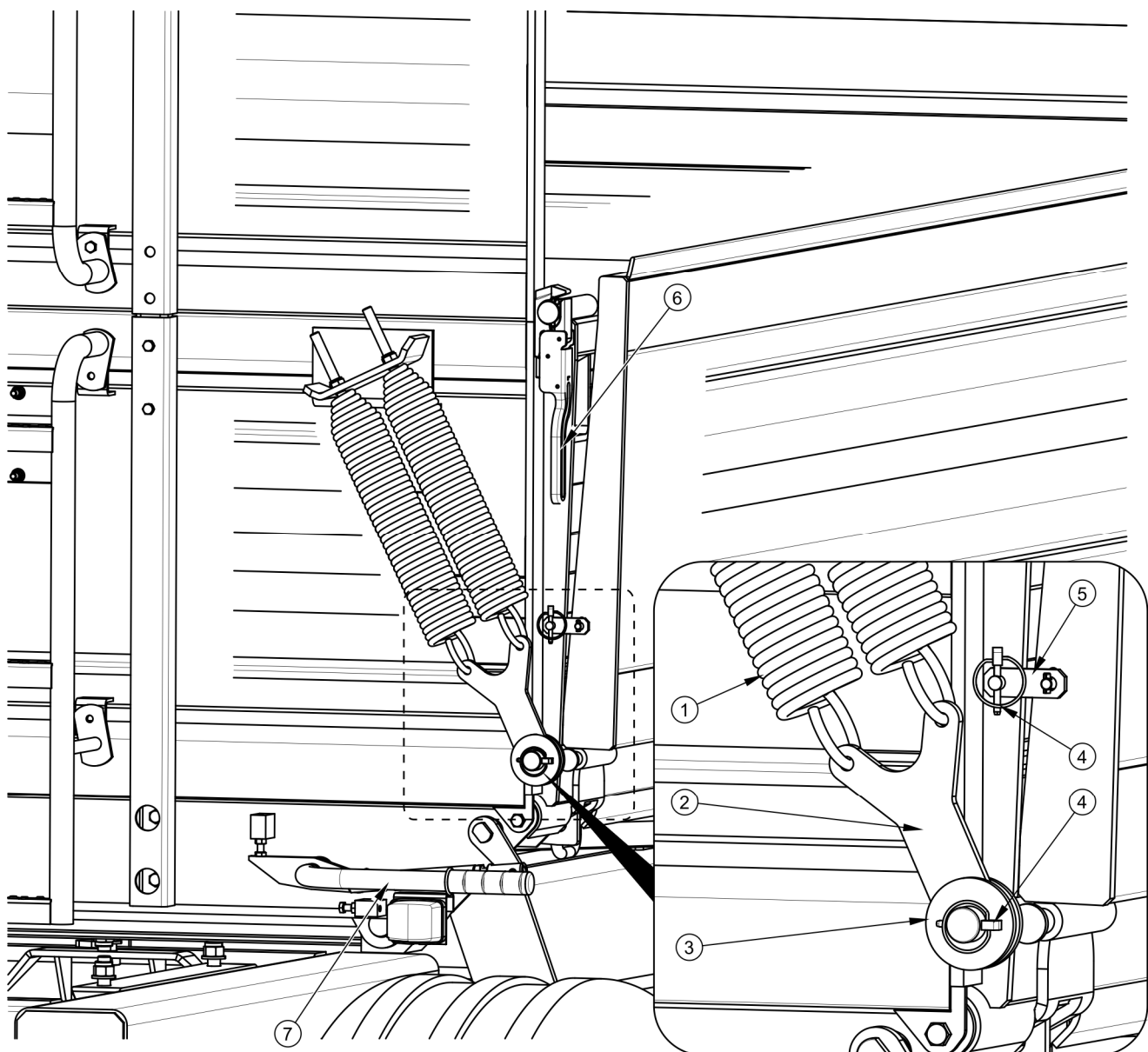
Obrázek 4.5 Kotevní mechanismus
