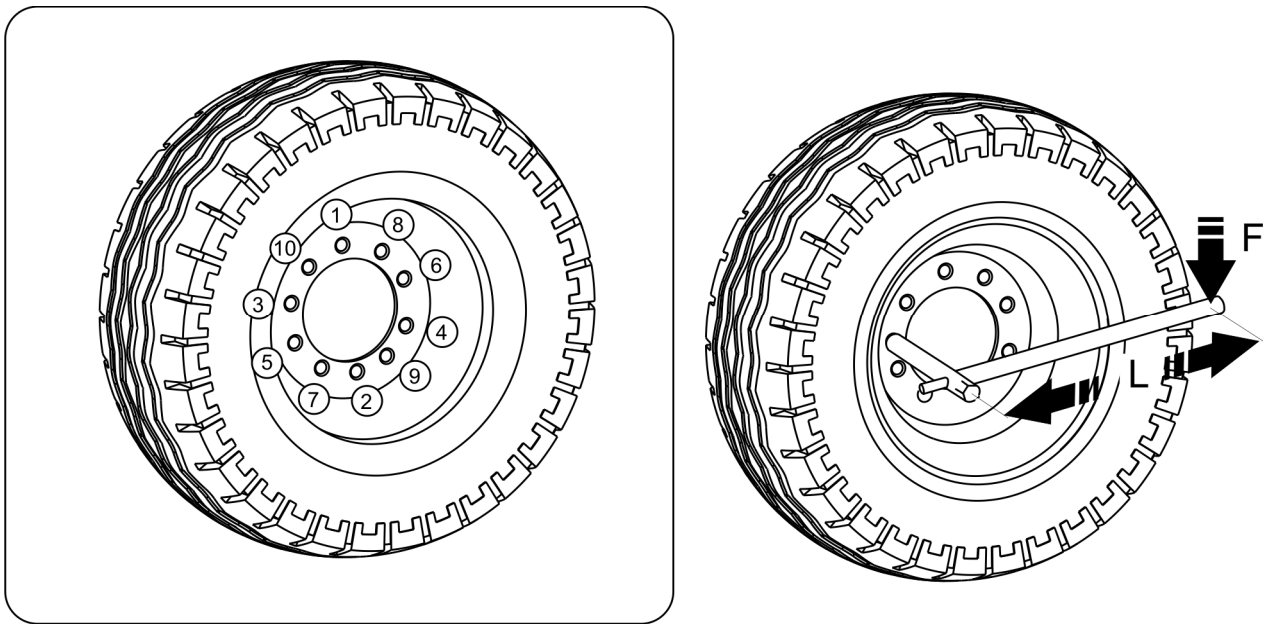
Obrázek 5.4 Pořadí dotahování matic
