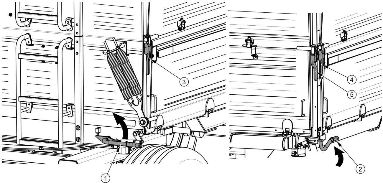
Obrázek 4.3 Otevírání bočnic
