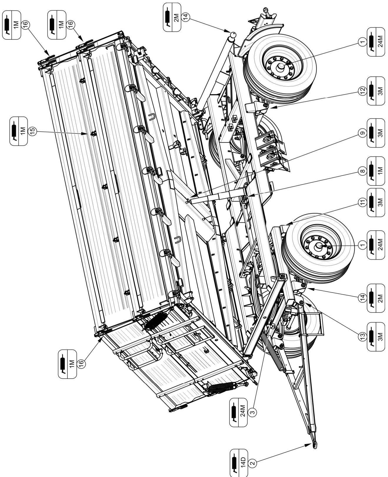
Obrázek 5.11 Mazací místa přívěsu, část 1
