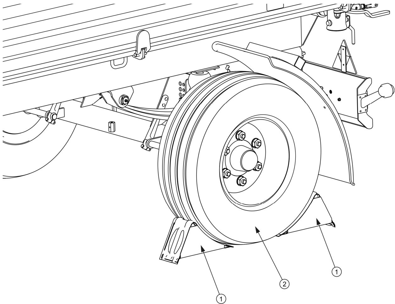
Obrázek 2.1 Způsob podložení klínů
