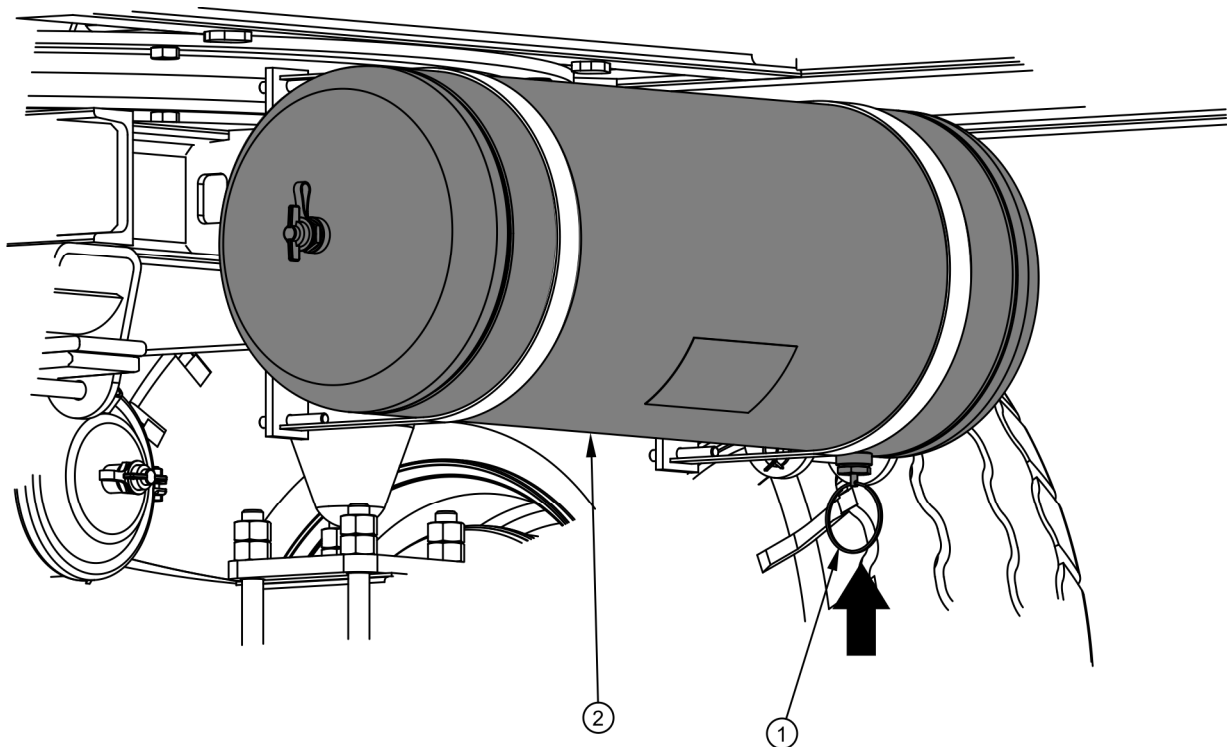
Obrázek 5.9 Odvodňování vzdušníku
