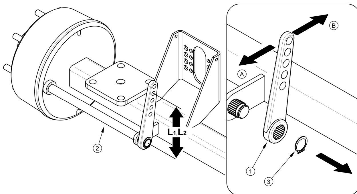
Obrázek 5.5 Seřízení mechanických brzd pojzdových náprav
