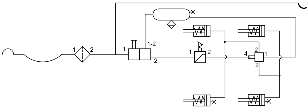
RYSUNEK 3.6 Budowa i schemat instalacji hamulcowej pneumatycznej jedнопrzewodowej
