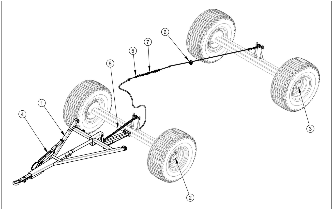
RYSUNEK 3.8 Hamulec najazdowy
