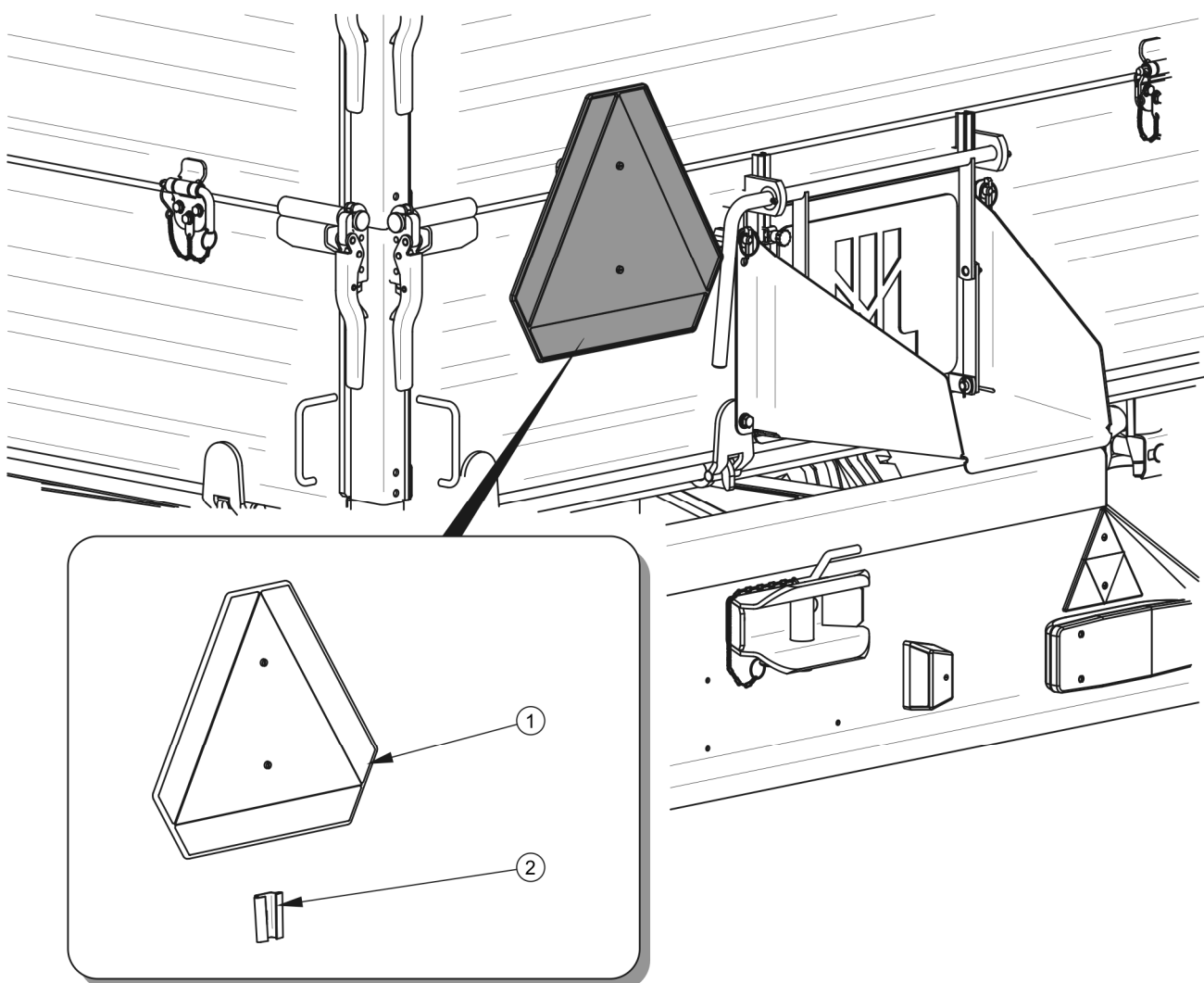
Obrázek K 2.2 Místo montáže tabulky označující pomalá vozidla
