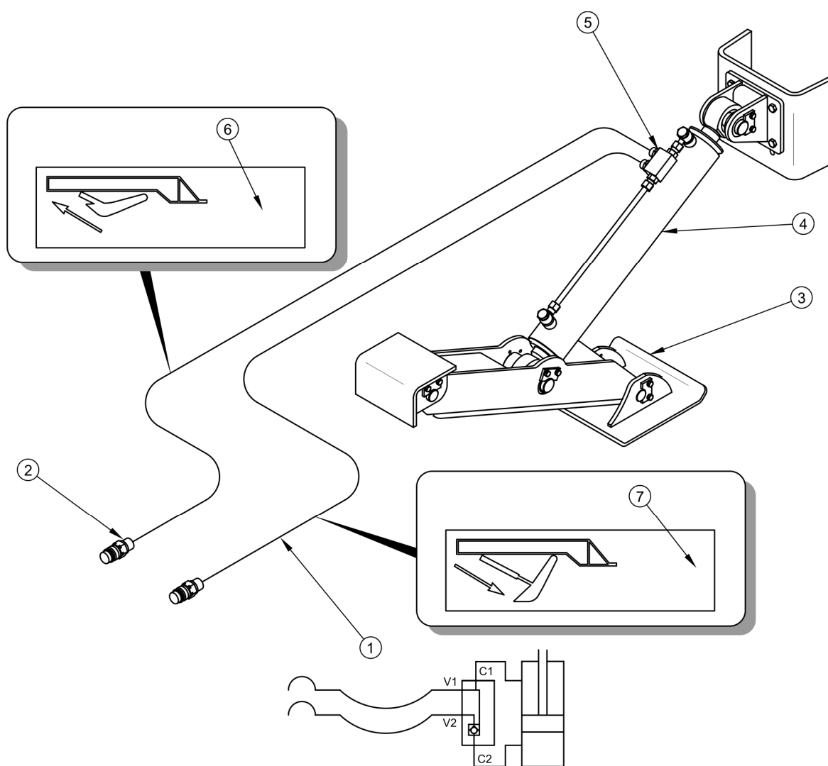
Obrázek 3.12 Konstrukce a schéma hydraulické instalace nůžkové podpěry
