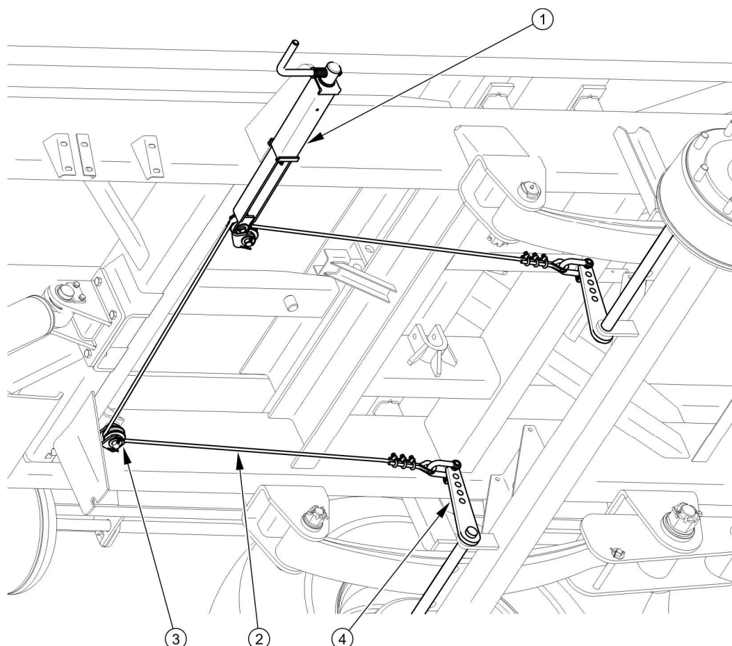
Obrázek 3.13 Konstrukce parkovací brzdy
