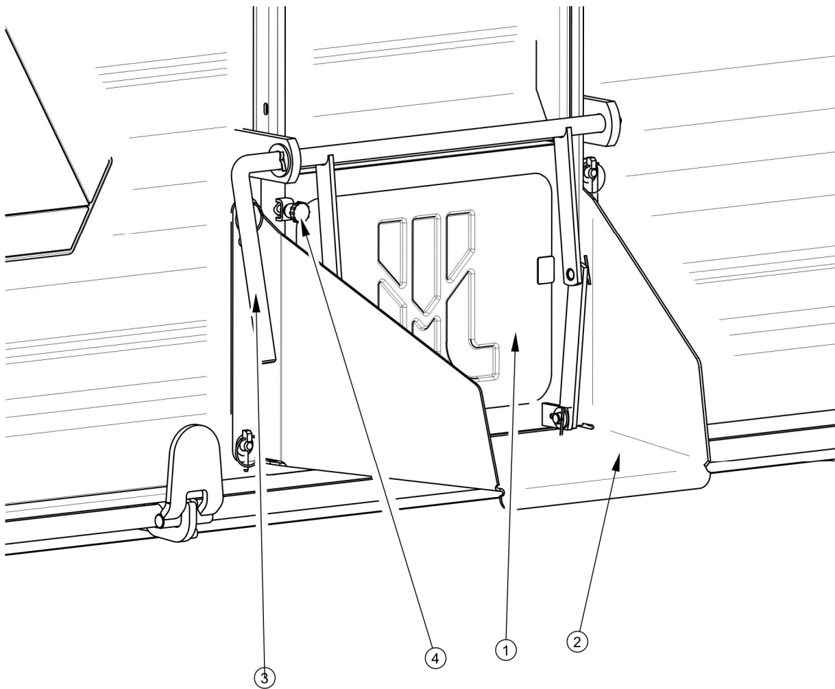
Obrázek 4.6 Skluz
