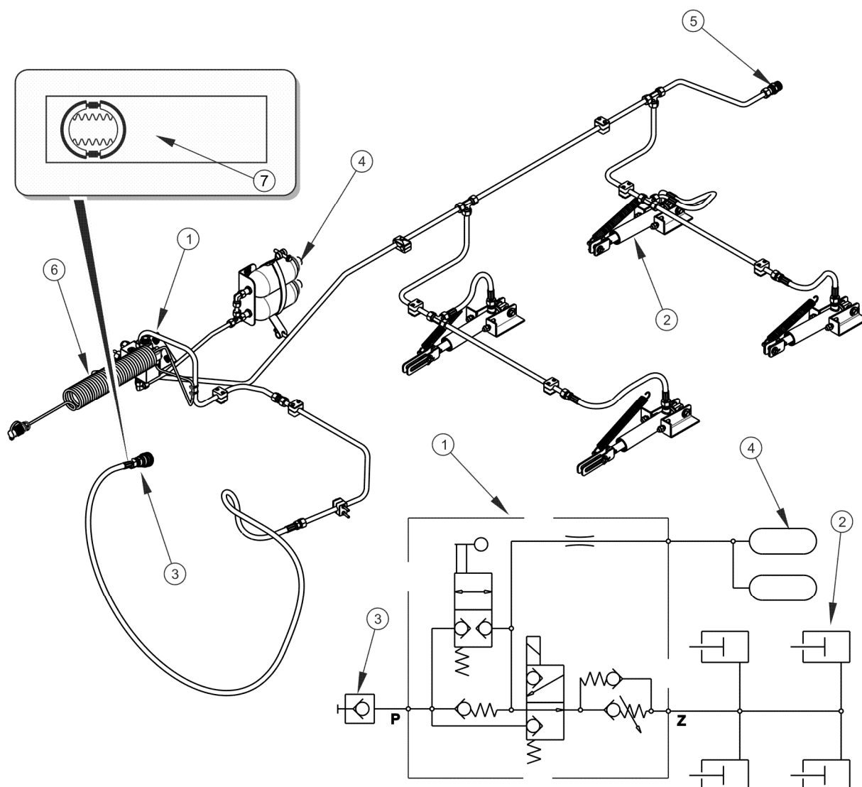
Obrázek 3.9 Konstrukce a schéma hydraulické brzdové instalace
