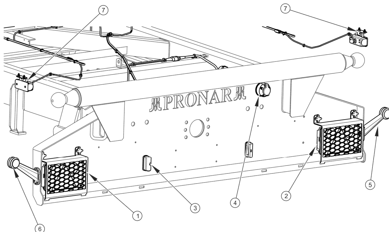
Obrázek 3.15 Rozmístění prvků elektroinstalace a odrazových skel – pohled zezadu
