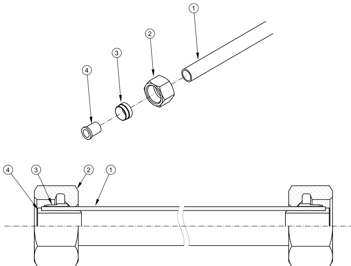
Obrázek 5.9 Konstrukce vzduchové hadice.
