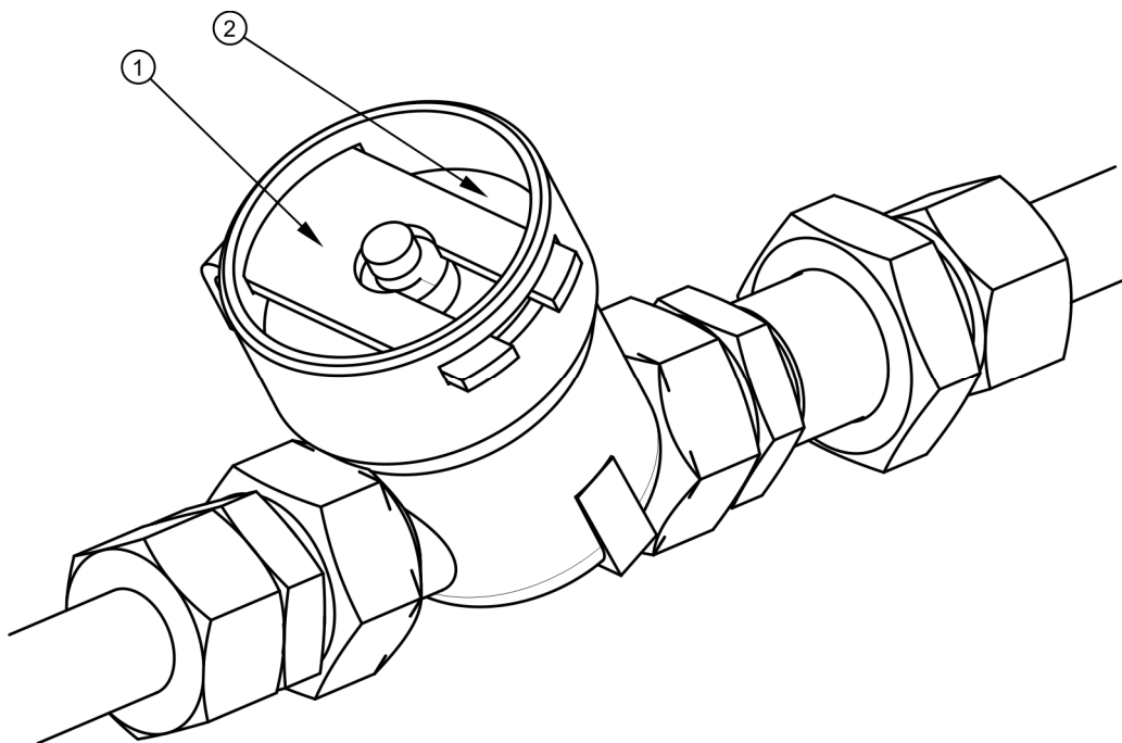
Obrázek 5.7 Vzduchový filtr
