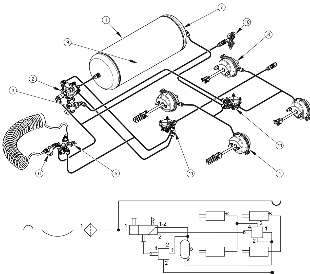
Obrázek 3.5 Konstrukce a schéma vzduchové jednohadicové brzdové instalace
