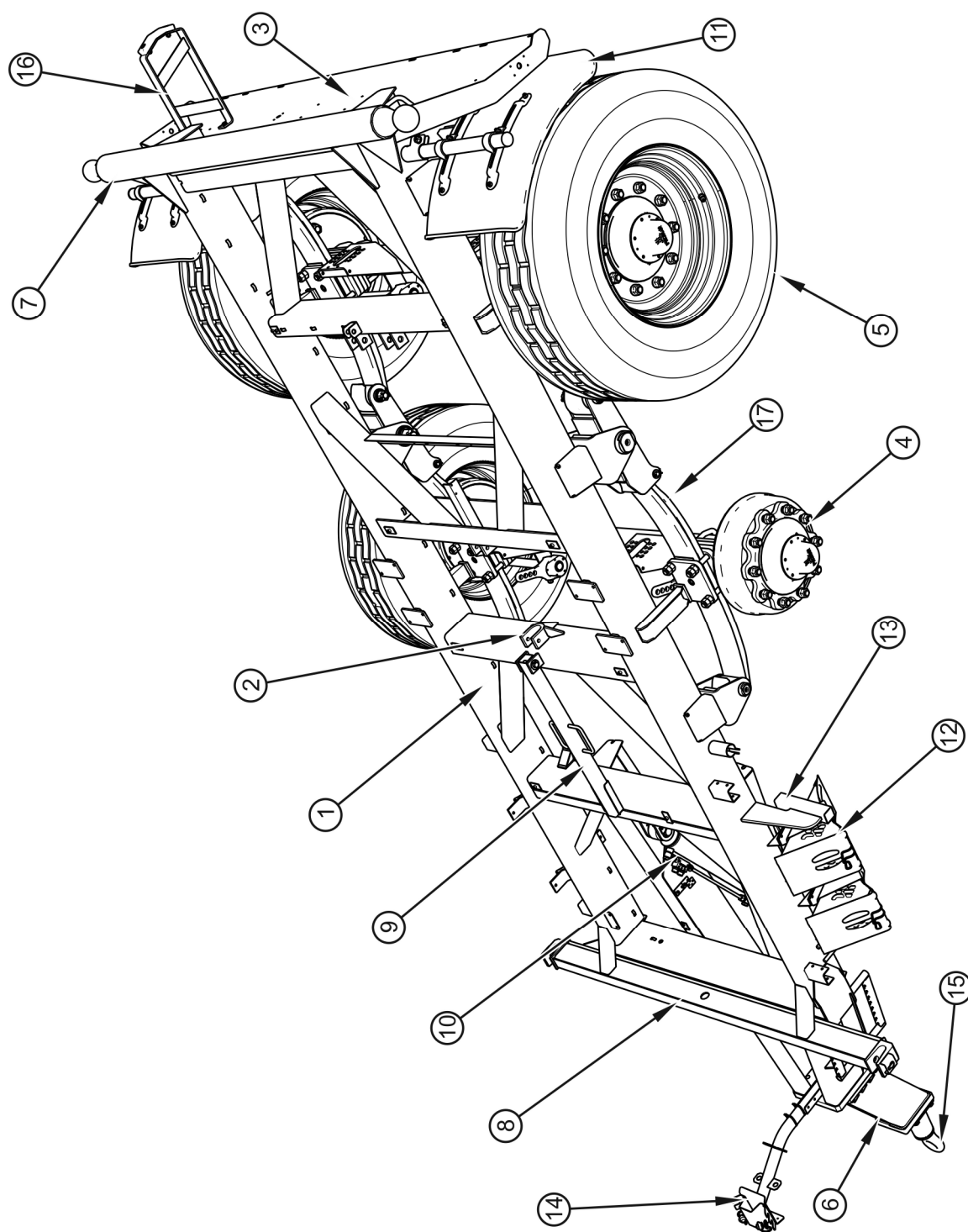
Obrázek 3.1 Podvozek přívěsu
