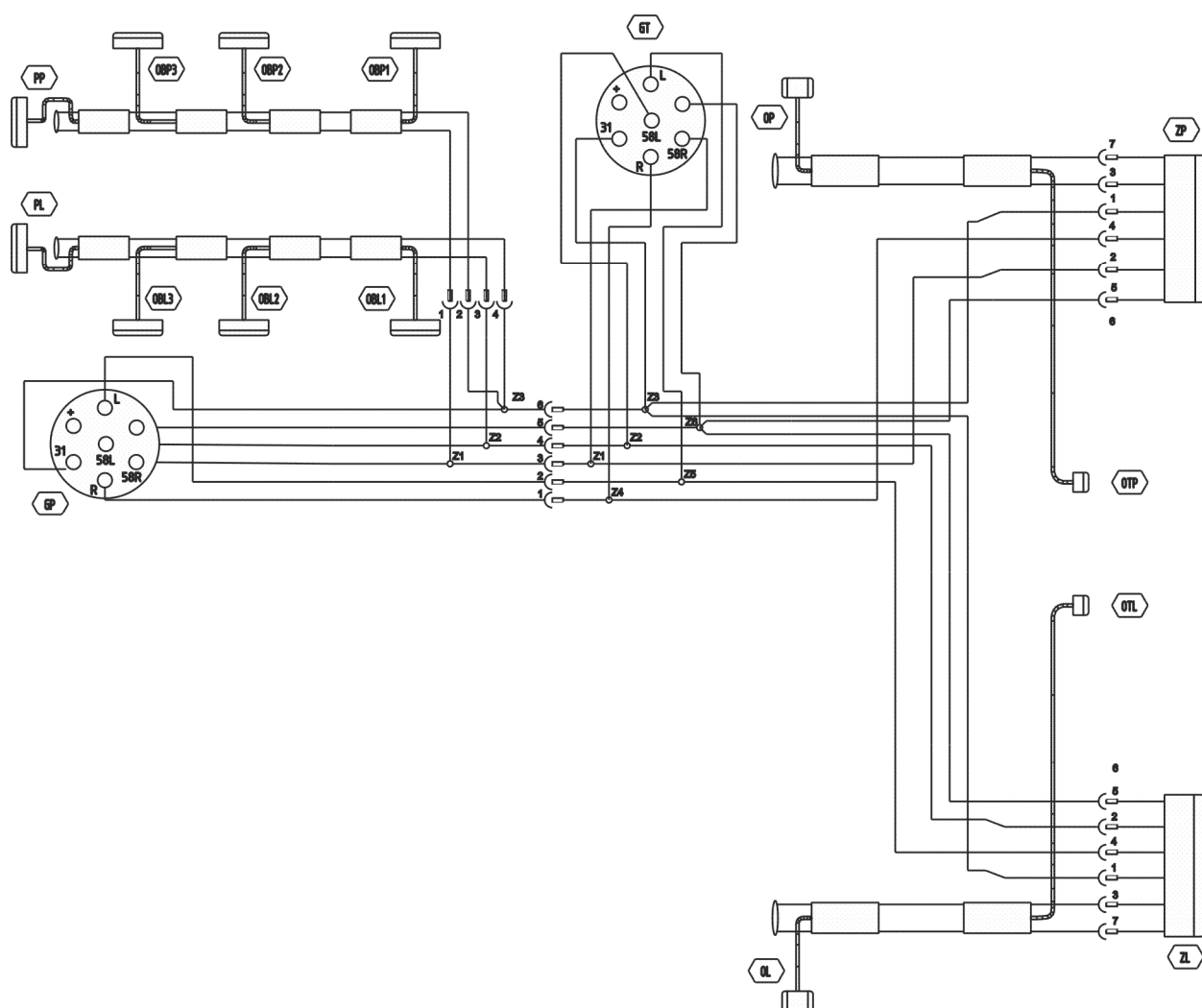
Obrázek 3.14 Ideové schéma elektroinstalace
