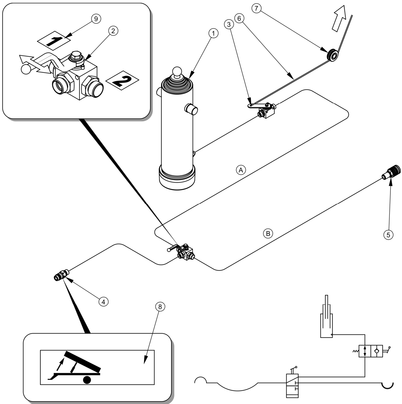
Obrázek 3.11 Konstrukce a schéma hydraulické instalace sklápění
