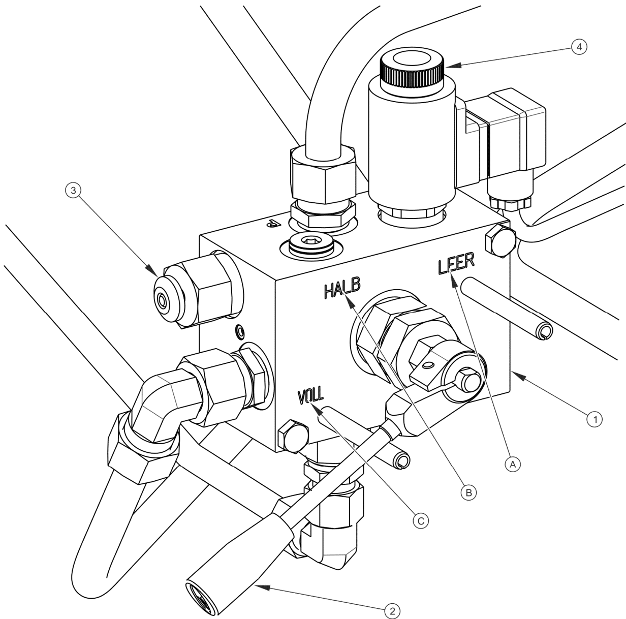
Obrázek 3.10 Elektrohydraulický brzdový ventil
