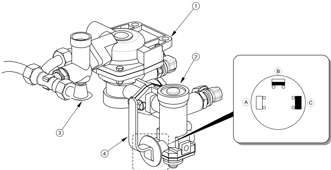
Obrázek 3.8 Ovládací ventil a regulátor brzdné síly
