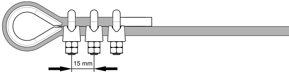
Obrázek 5.6 Montáž svorek brzdového lanka
