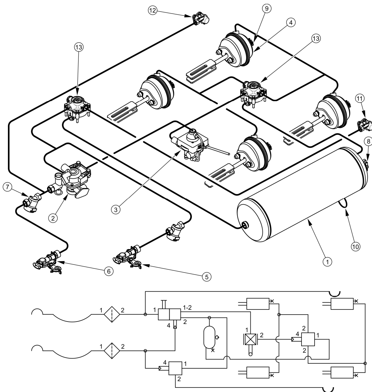
Obrázek 3.7 Konstrukce a schéma vzduchové brzdové dvouhadicové instalace s automatickým regulátorem brzdné síly
