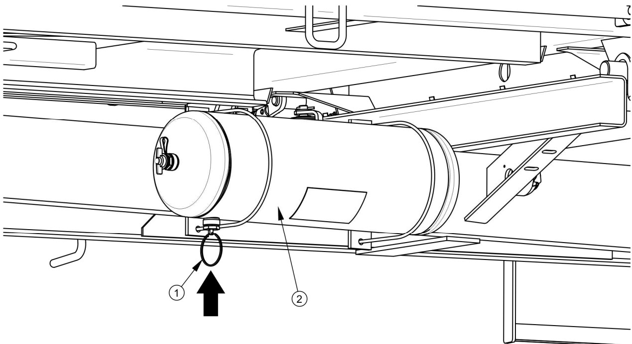
Obrázek 5.8 Odvodňování vzdušníku
