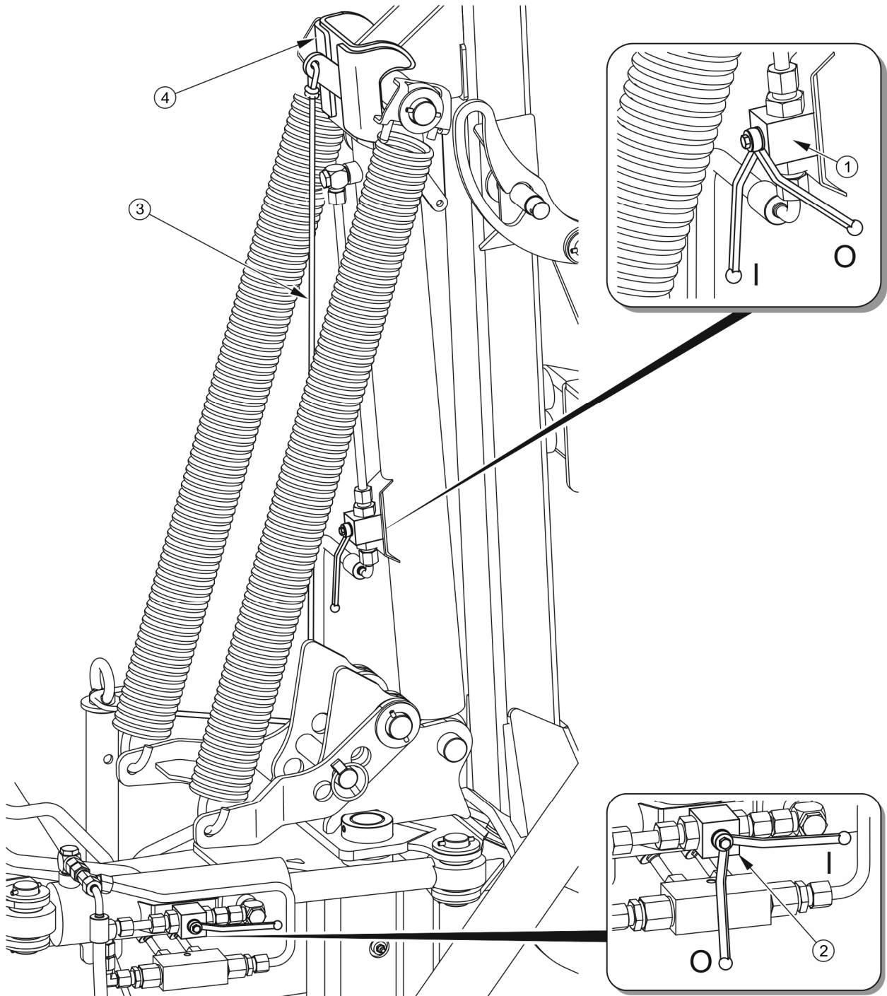
RYSunEK 4.6 Ustawienie kosiarki w pozycji roboczej
