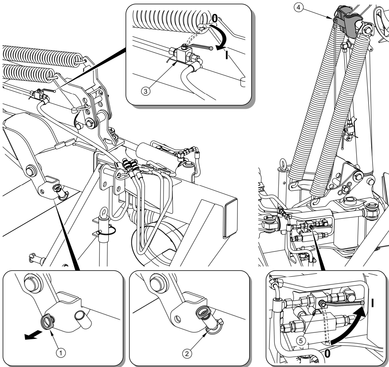
RYSUNEK 4.4 Ustawienie pozycji transportowej
