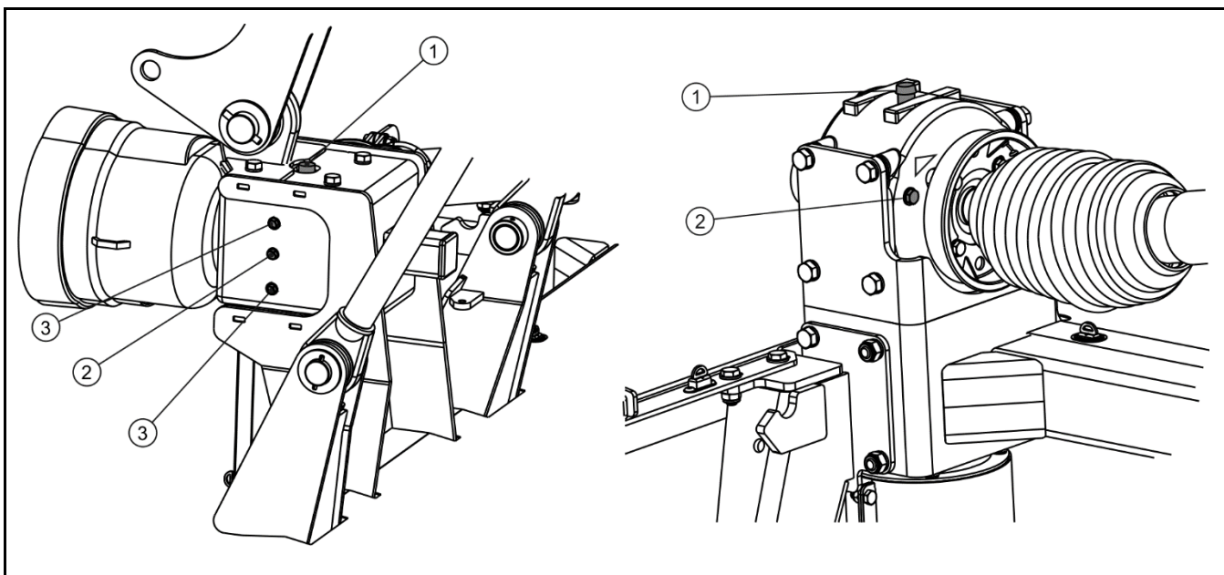
РИСУНОК 5.4 Контрольные точки передач
