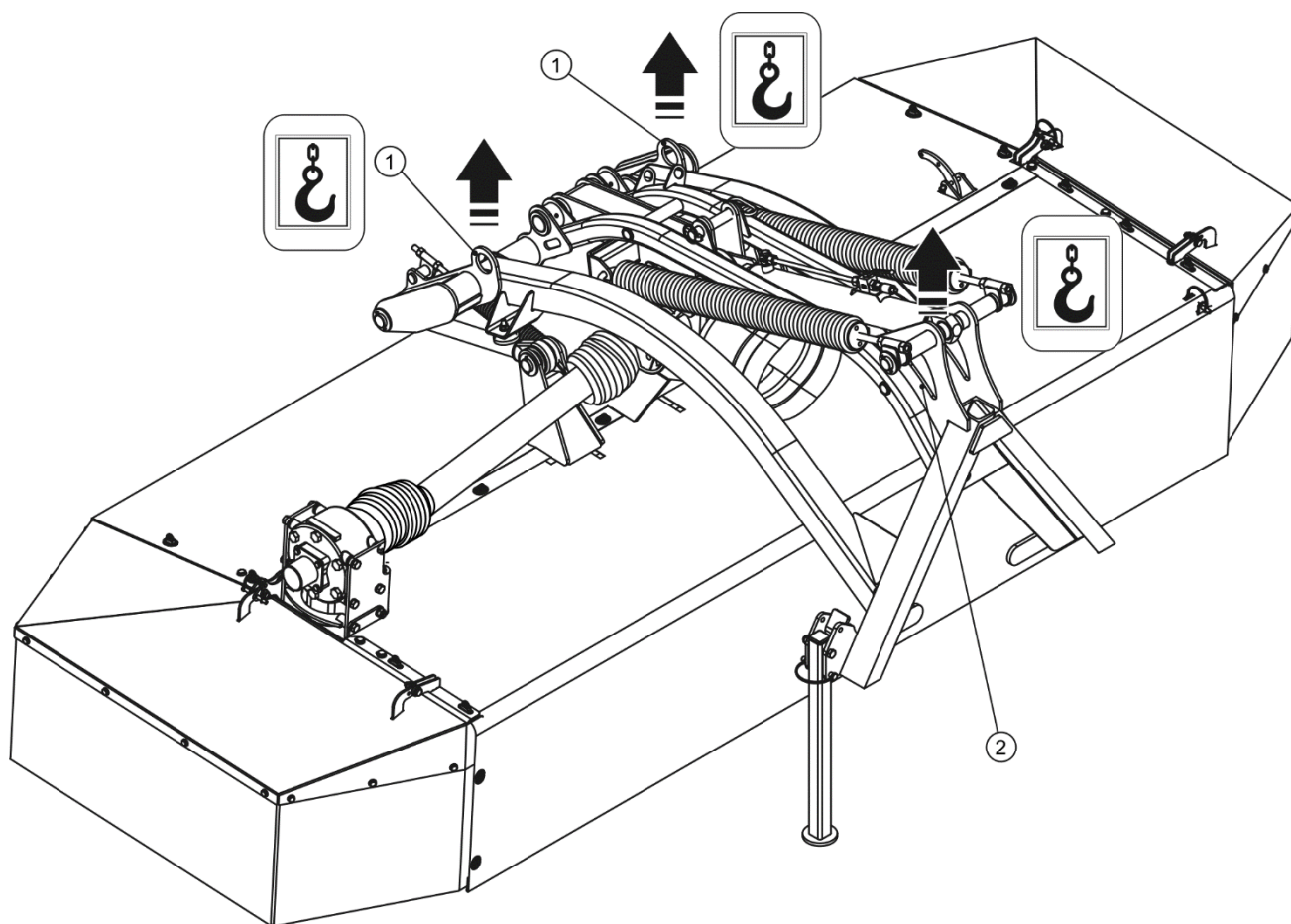
РИСУНОК 1.2 Транспортные захваты.
