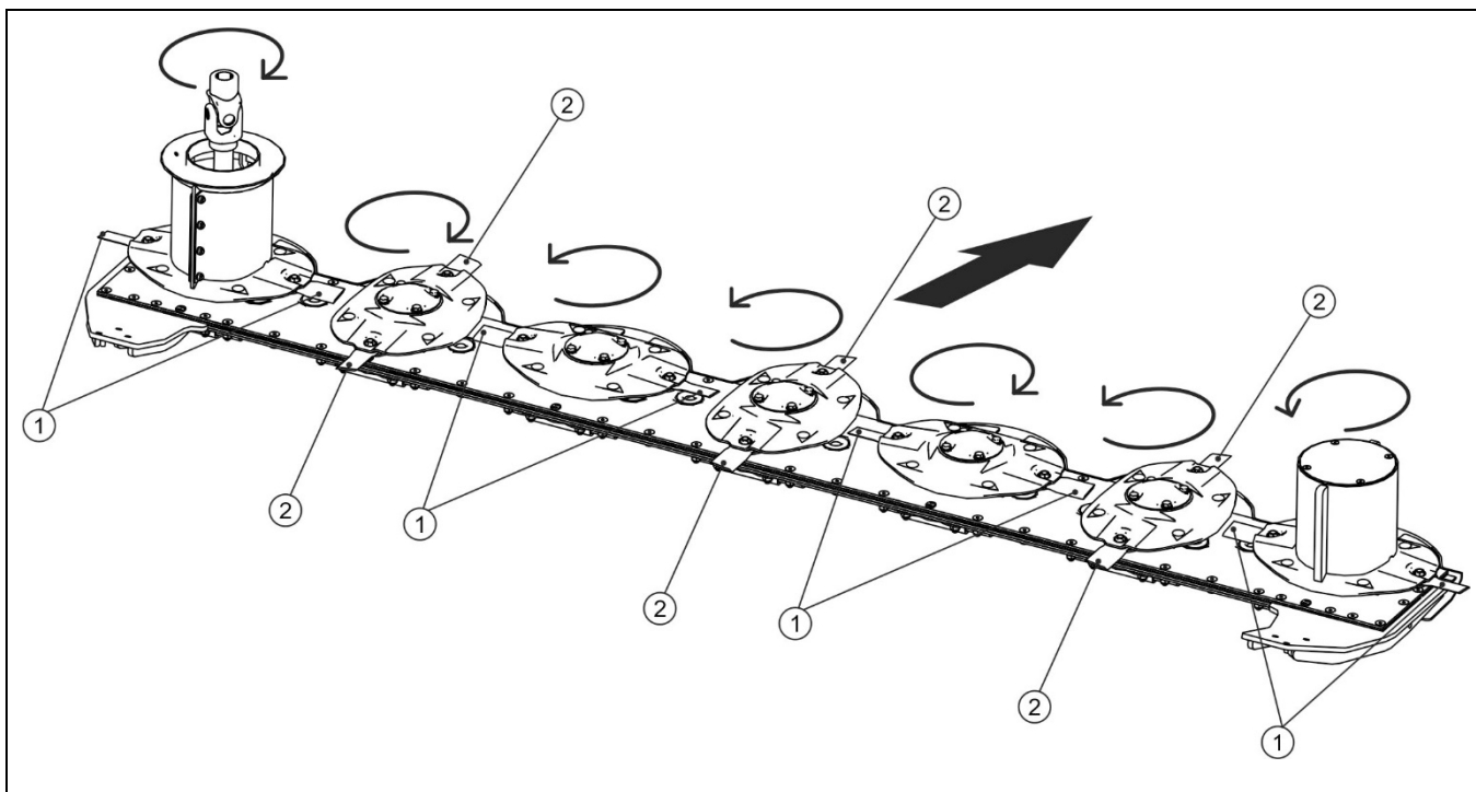
РИСУНОК 5.2 Направление вращения режущих дисков
