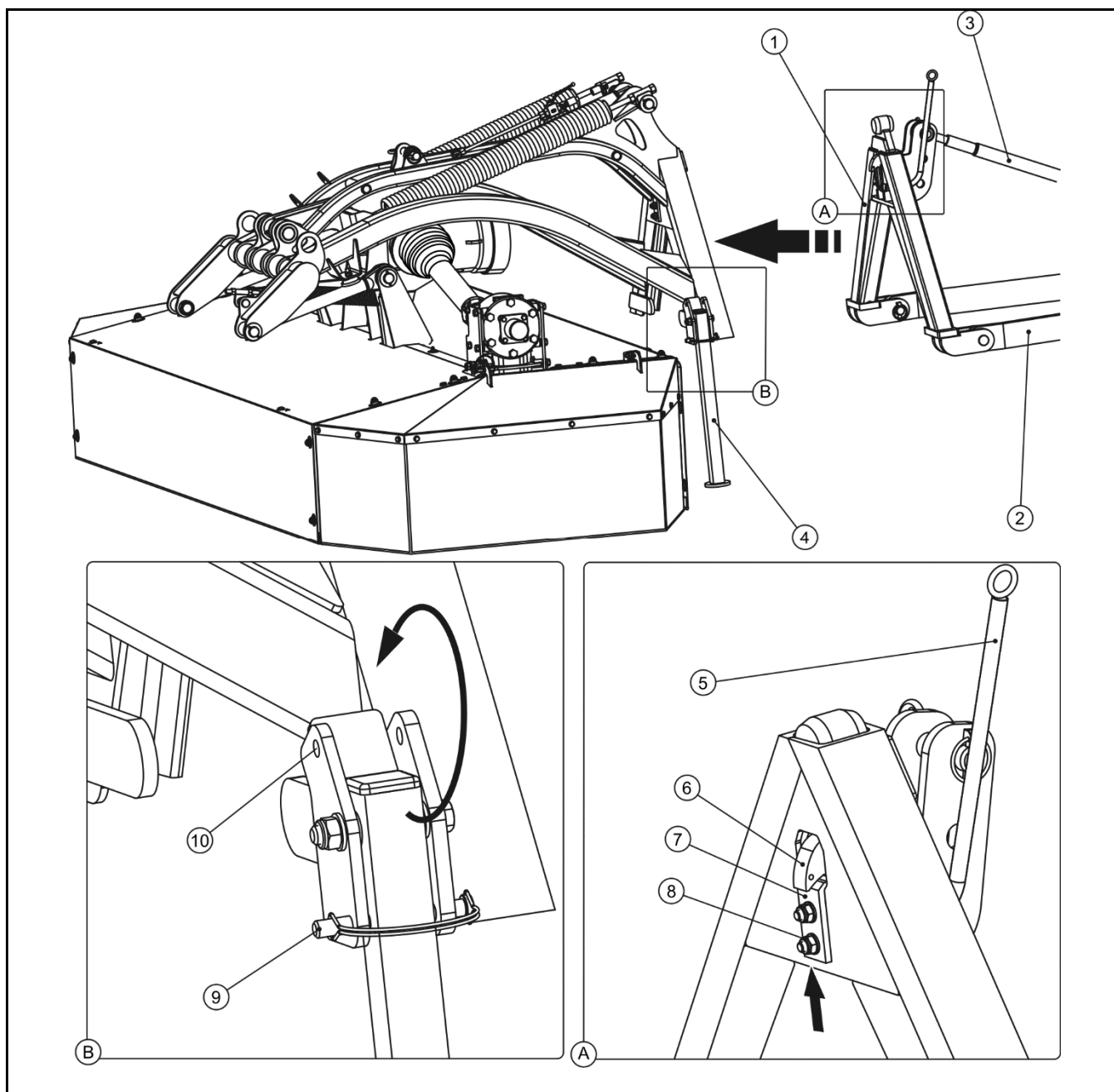
РИСУНОК 4.2 Подсоединение к трактору
