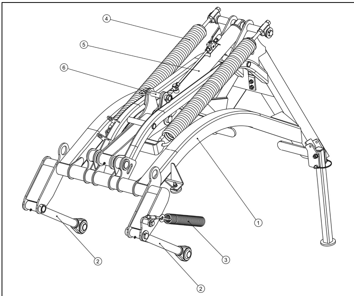
РИСУНОК 3.2 Устройство системы навески
