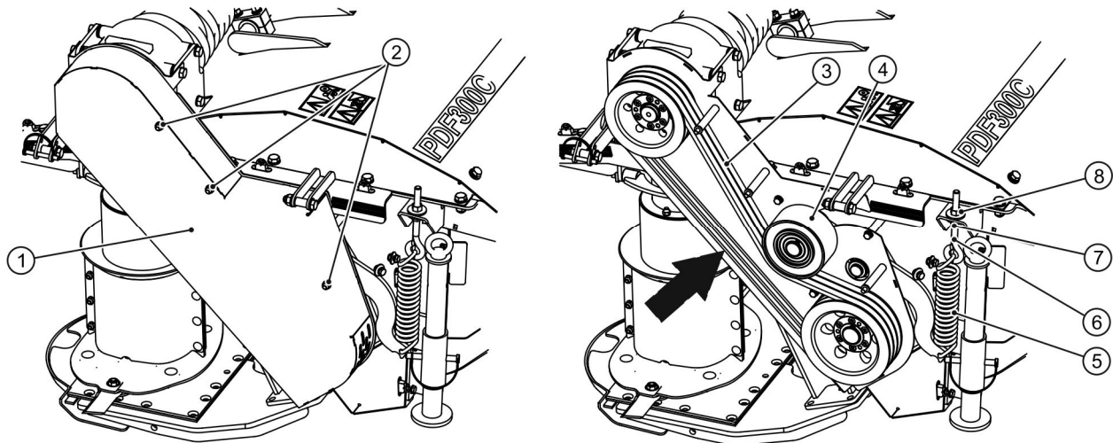
РИСУНОК 5.6 Регулирование натяжения ременной передачи PDF300C
