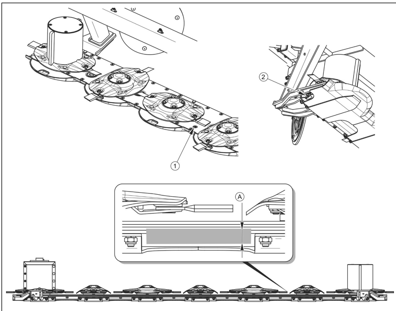
РИСУНОК 5.7 Проверка уровня масла в режущем бруске
