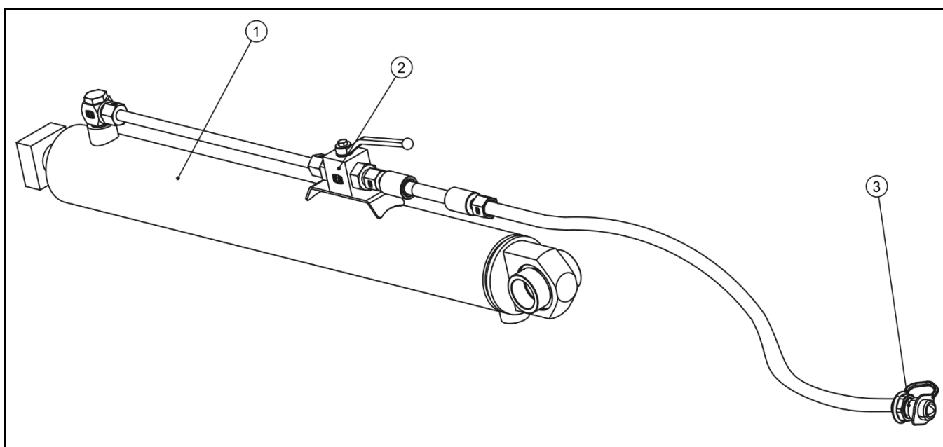
РИСУНОК 3.5 Устройство гидравлической системы
