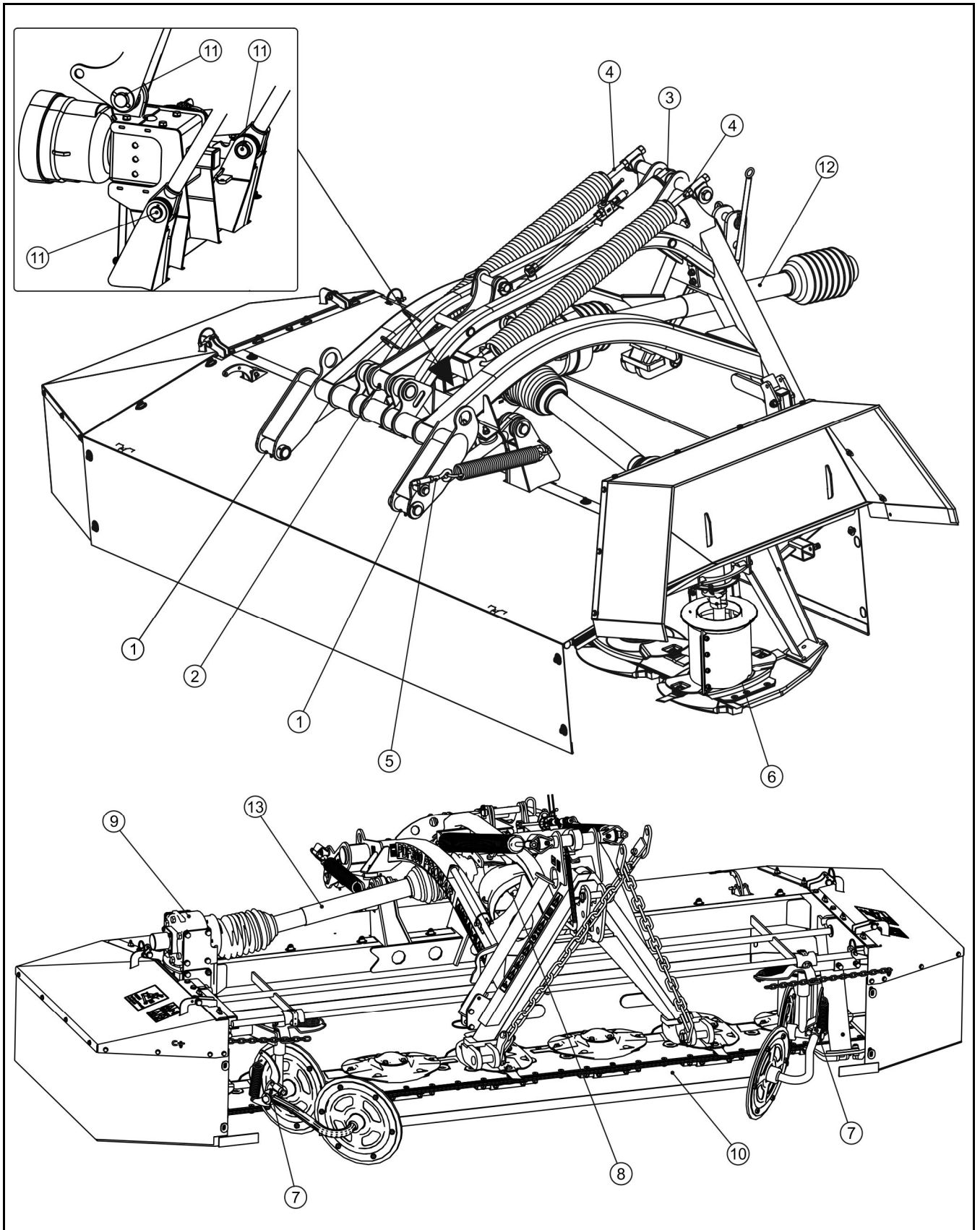
РИСУНОК 5.9 Точки смазки косилки PDF300 / PDF300C
