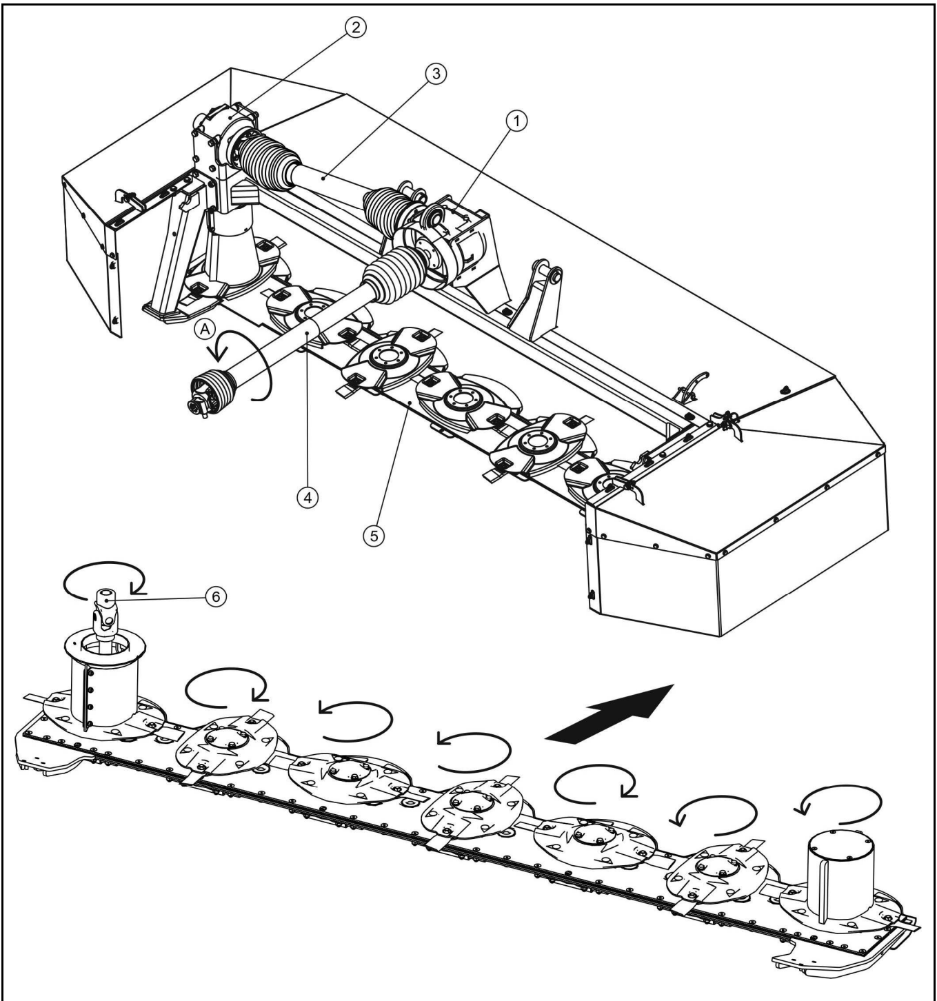
РИСУНОК 3.4 Механизм передачи привода
