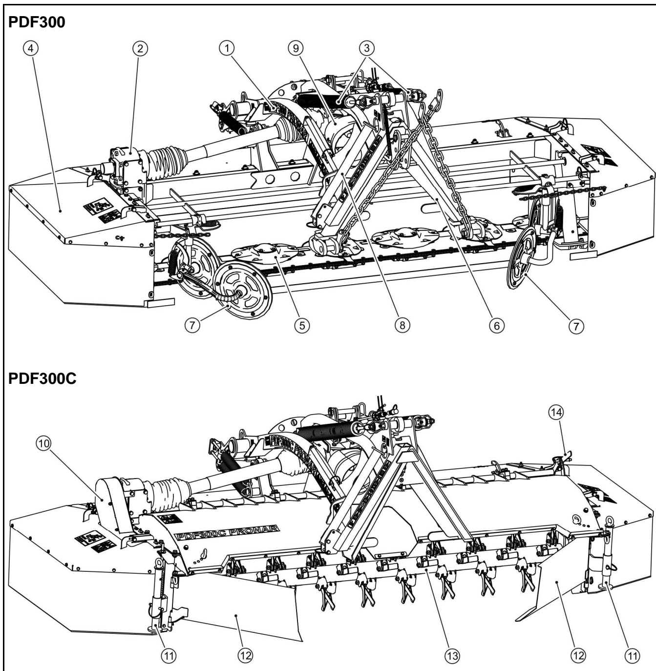
РИСУНОК 3.1 Общее устройство
