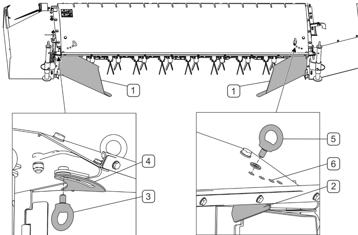
РИСУНОК 4.9 Регулировка подборщиков покоса PDF300C.
