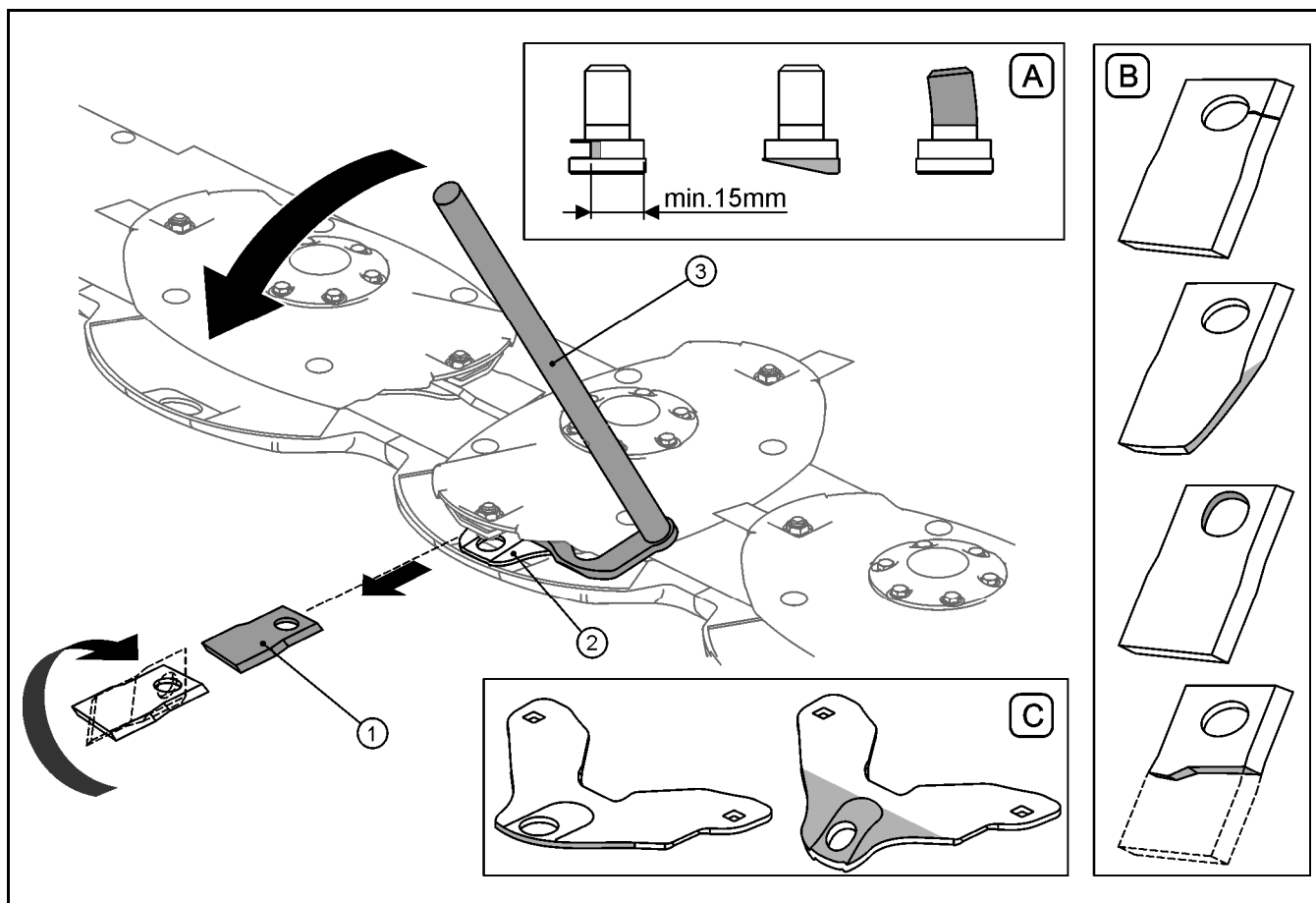
РИСУНОК 5.1 Замена ножей на режущем брус
