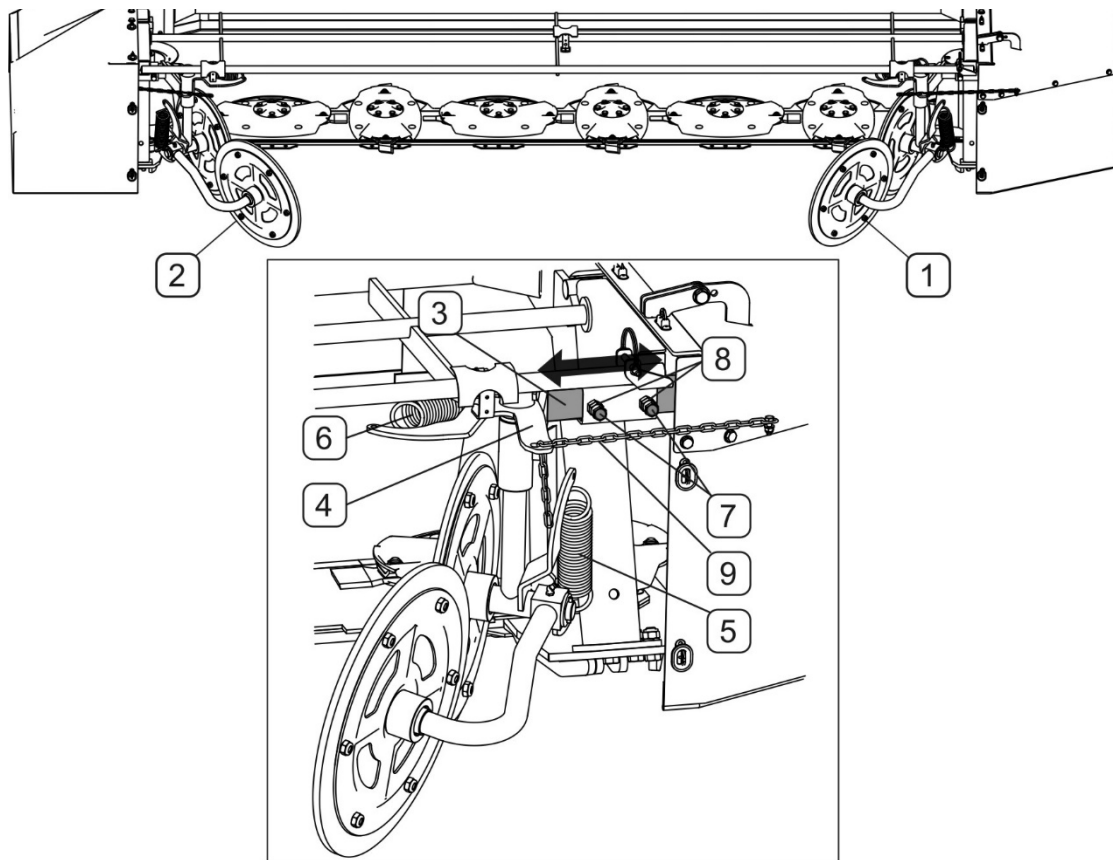
РИСУНОК 4.8 Регулировка подборщиков покоса PDF300
