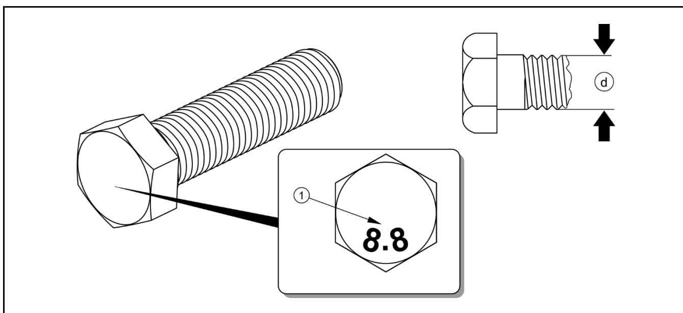
РИСУНОК 5.11 Болт с метрической резьбой
