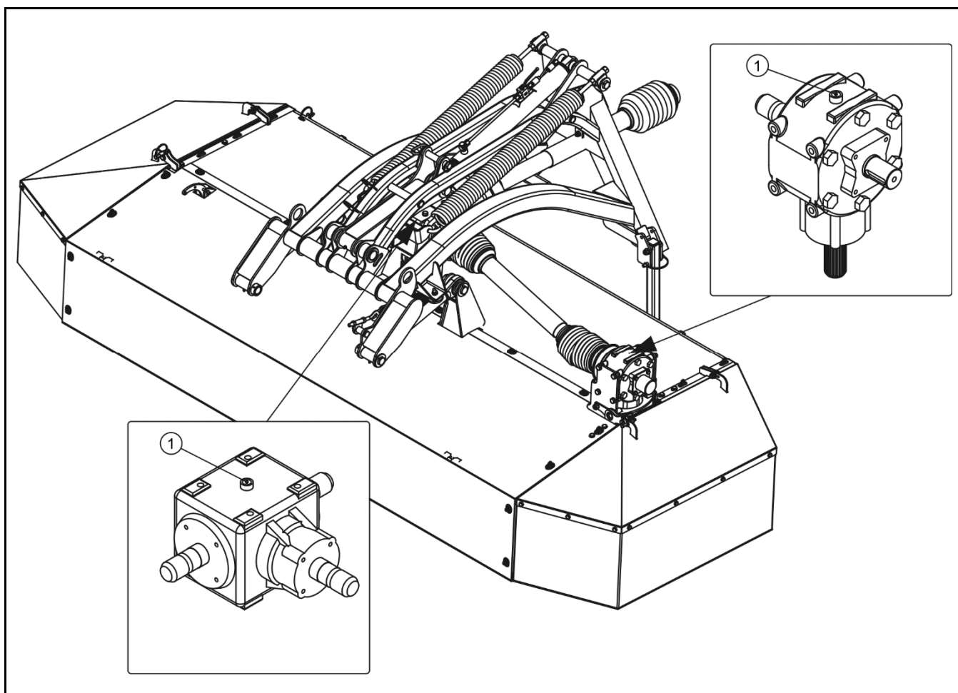
РИСУНОК 5.5 Размещение угловых передач
