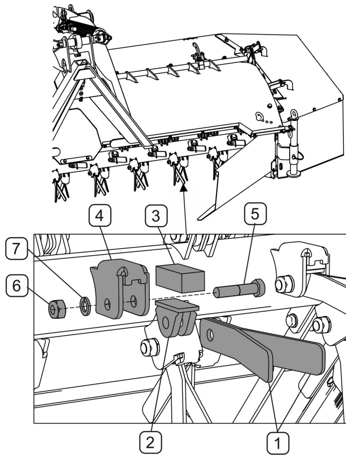
РИСУНОК 5.3 Замена ударных ножей вспушвателя покоса (PDF300C).
