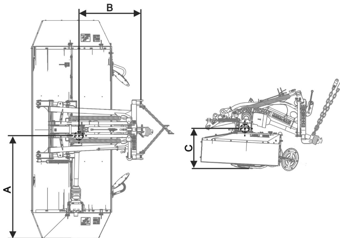
РИСУНОК 1.3 Расположение центра тяжести косилки PDF300 / PDF300C.
