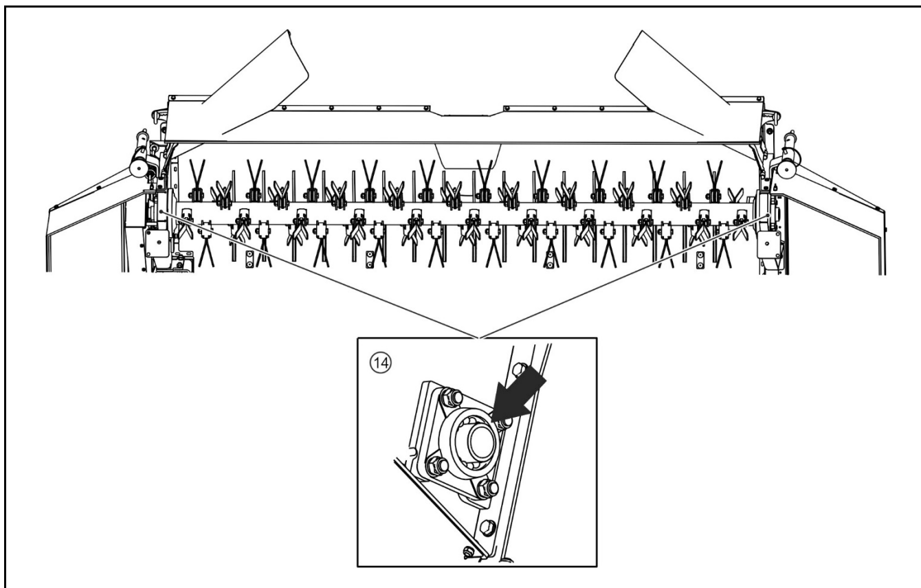
РИСУНОК 5.10 Точки смазки косилки PDF300C
