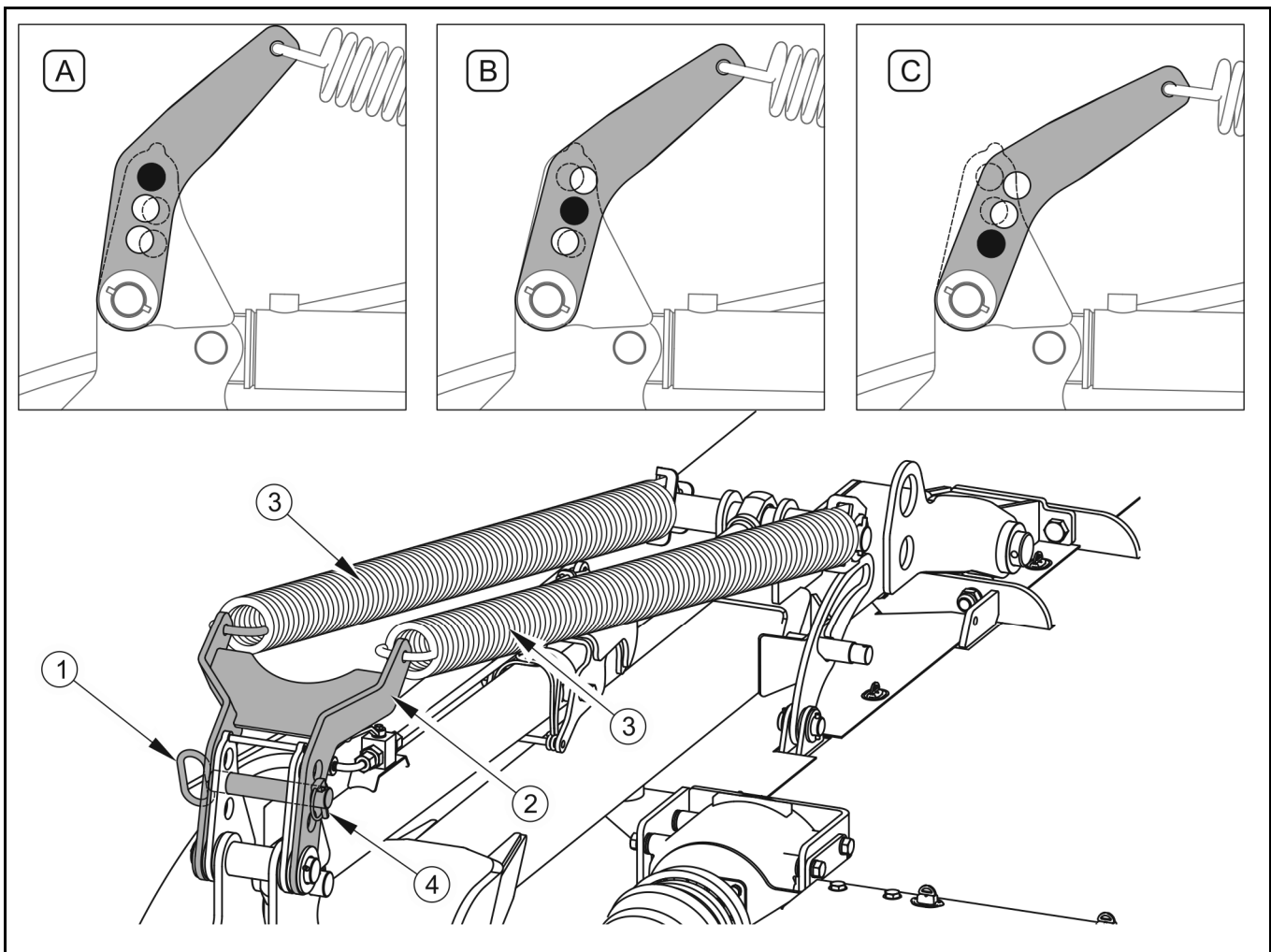
RYСУNEK 4.8 Regulacja nacisku listwy tnącej
