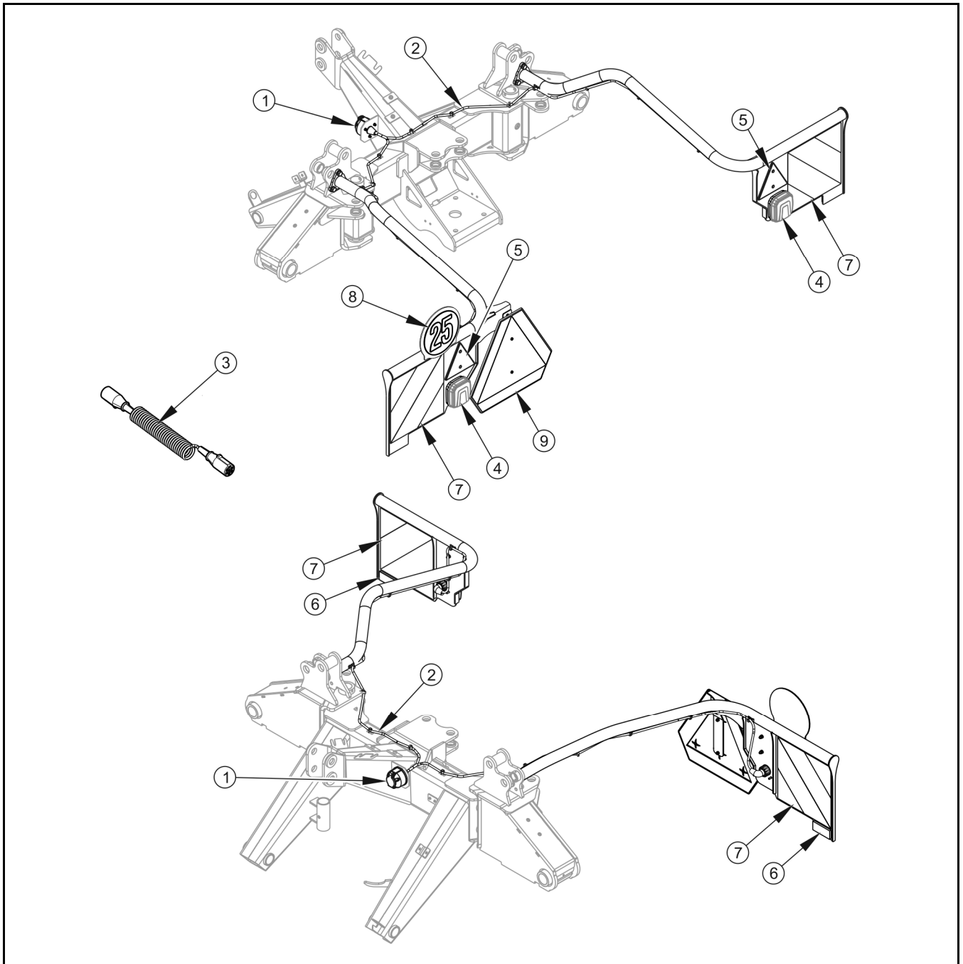
RYSUNEK 4.14 Instalacja oświetleniowa i dodatkowe oznakowanie
