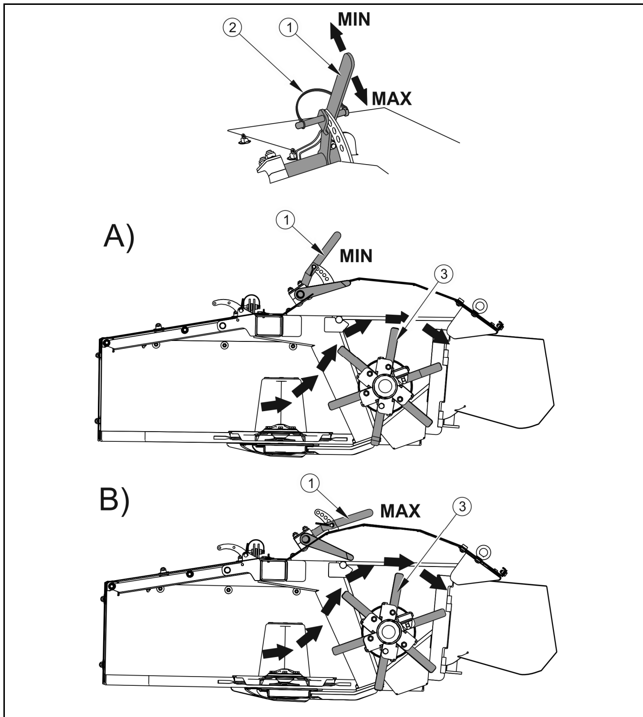
RYСУNEK 4.12 Ustawienie szerokości pokosu PDD830C
