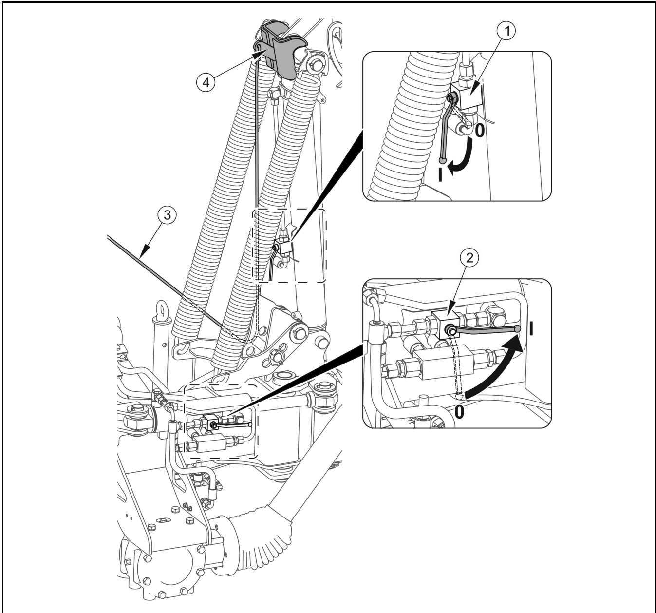
RYSUNEK 4.6 Ustawienie kosiarki do pozycji roboczej
