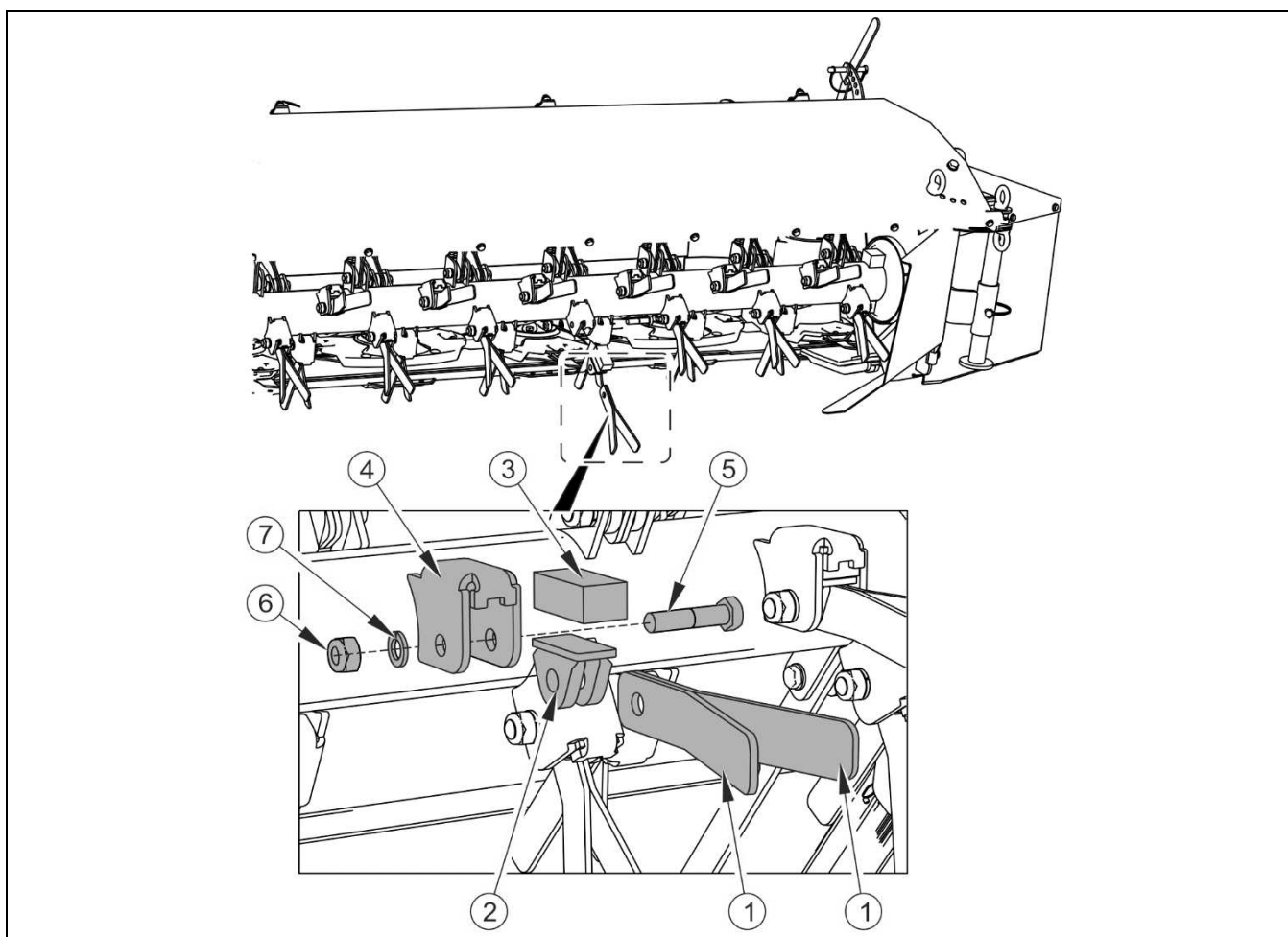
РИСУНОК 5.2 Замена ударных ножей вспушивателя покоса (PDD830C)
