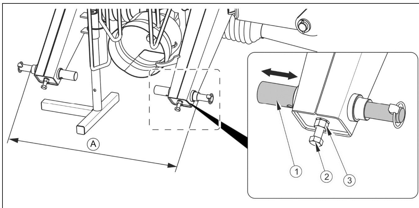
РИСУНОК 4.2 Регулировка нижних сцепных шкворней навесной системы косилки
