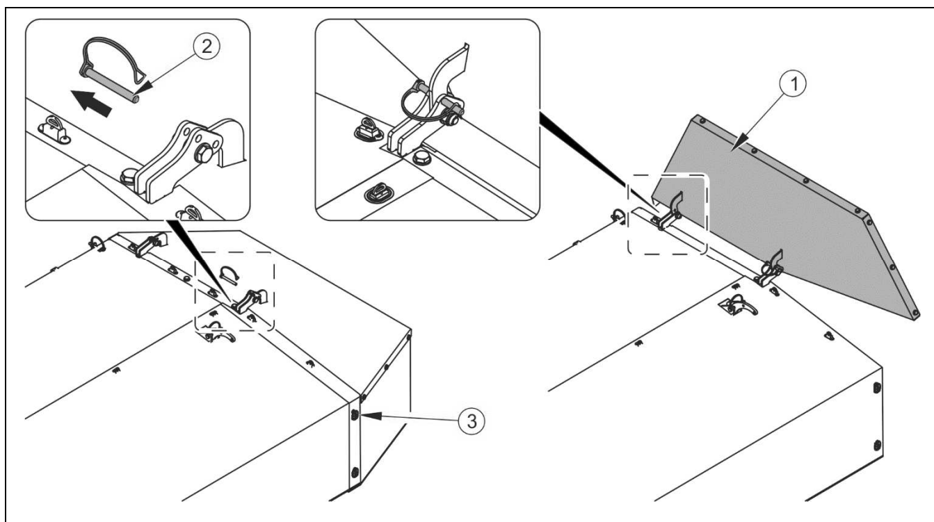
РИСУНОК 4.5 Подъем кожухов на время транспорта
