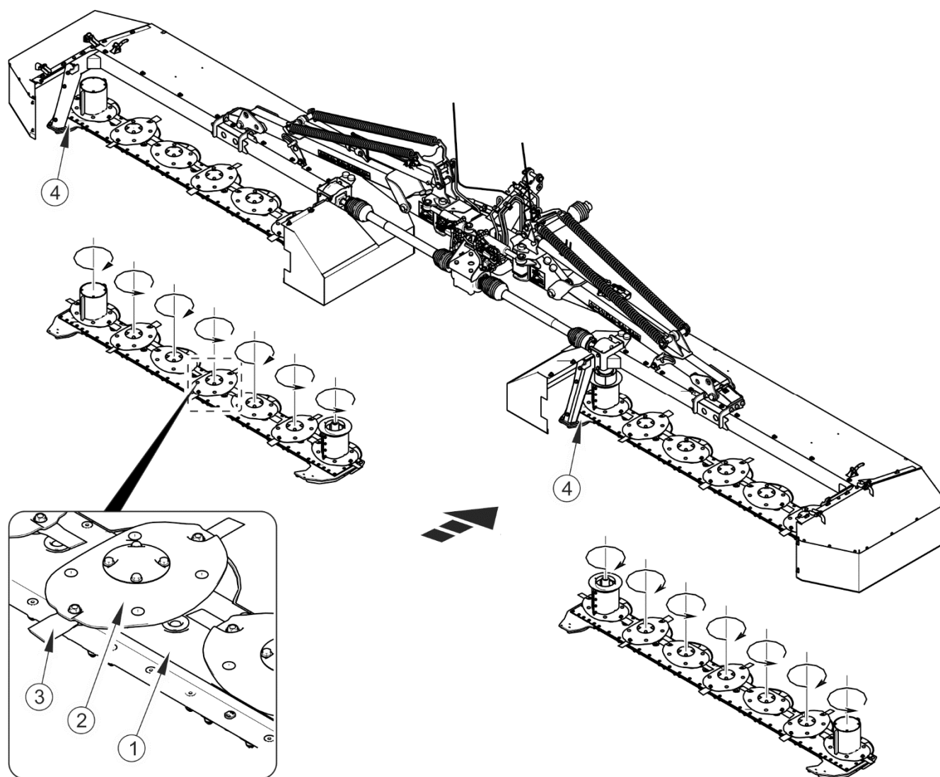
РИСУНОК 3.4 Режущий аппарат
