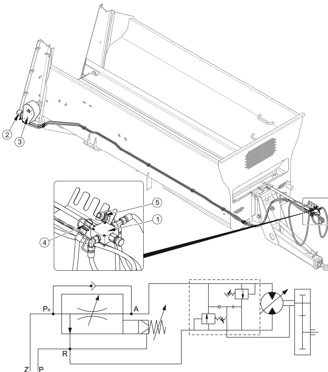
DISEGNO 3.4 Costruzione e schema dell'impianto idraulico del meccanismo di alimentazione
