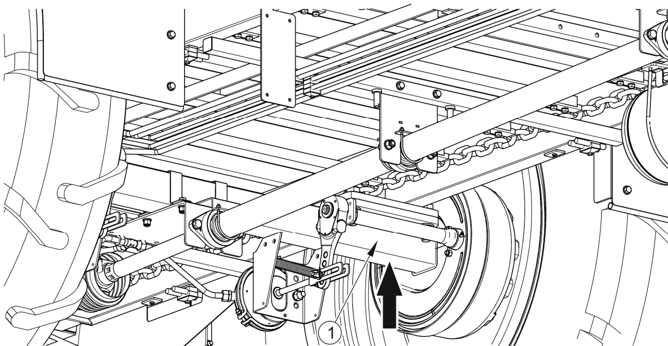
DISEGNO 5.2 Punto di appoggio sollevatore
