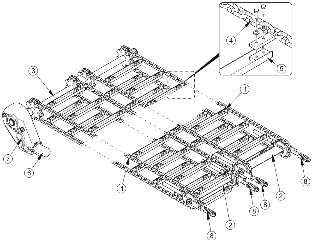
DISEGNO 3.3 Meccanismo di alimentazione NV161/4, NV161/5
