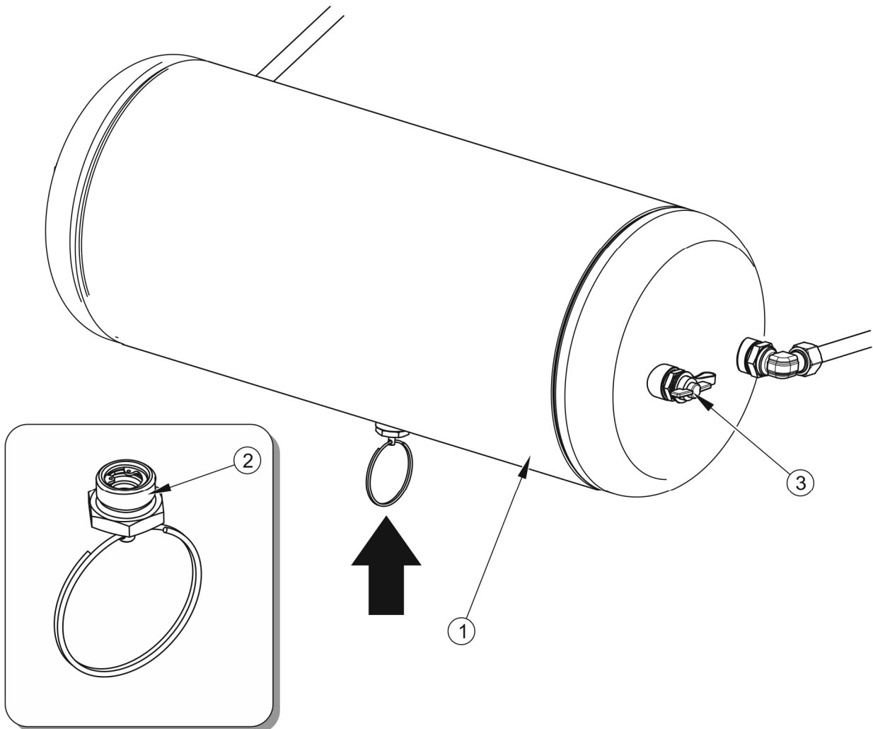
DISEGNO 5.10 Drenaggio serbatoio aria
