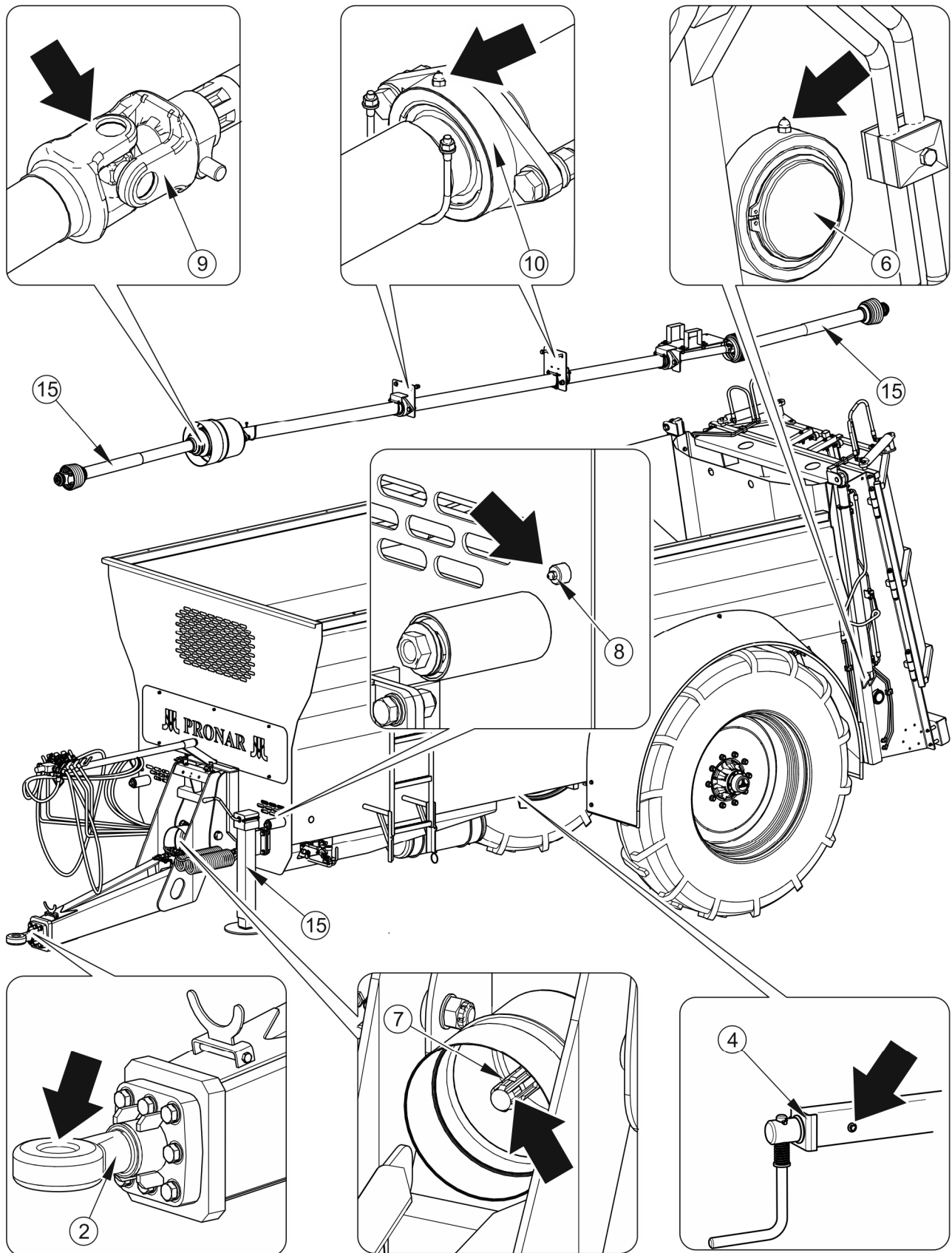
RYSUNEK 5.15 Punkty smarne rozrzutnika
