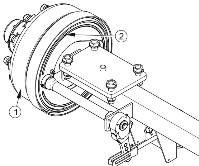
RYSUNEK 5.1 Kontrola okładzin hamulcowych
