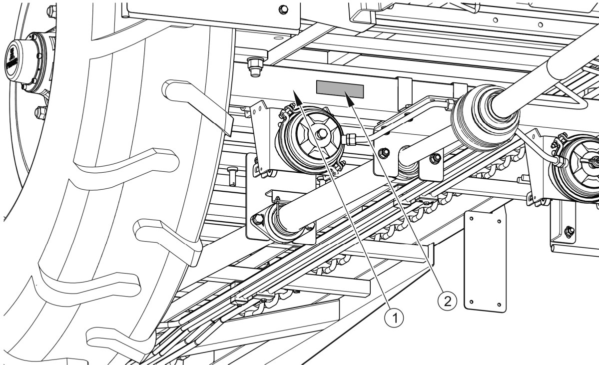
RYSUNEK 1.2 Miejsce umieszczenia tabliczki znamionowej osi jezdnej
