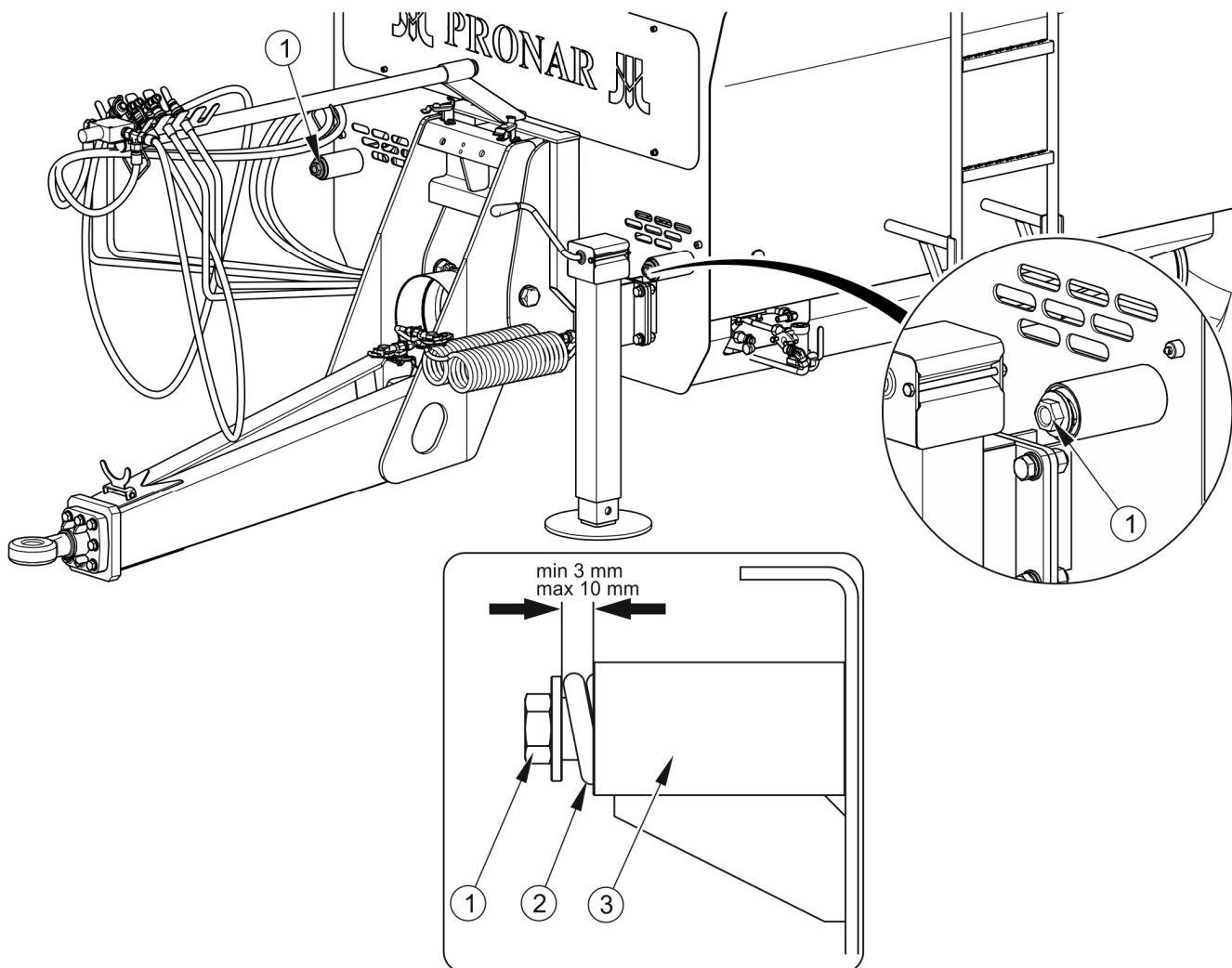
RYSUNEK 5.16 Regulacja napięcia przenośnika podłogowego
