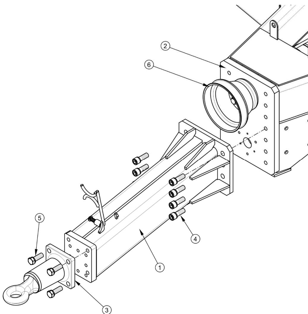
РИСУНОК 5.15 Монтаж нижнего дышла
