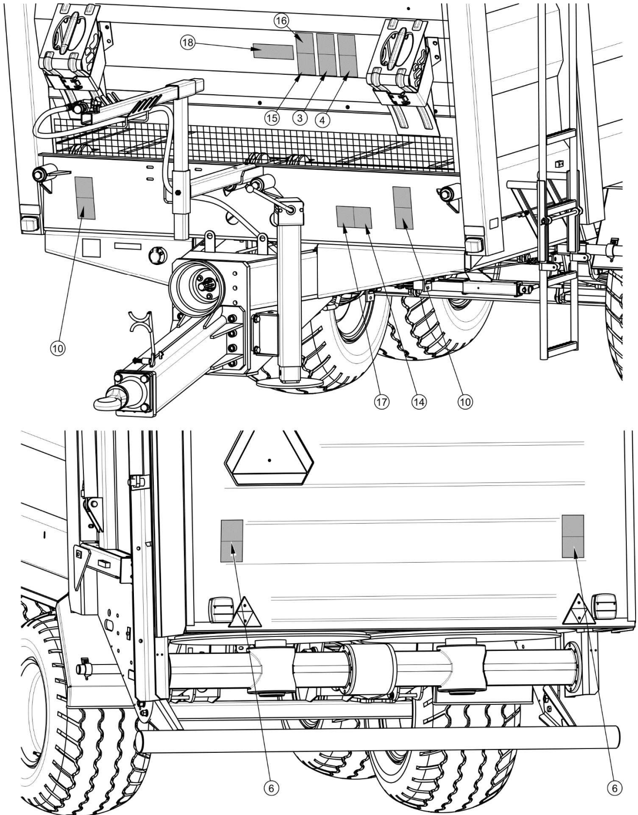
РИСУНОК 2.3 Размещение информационных и предупреждающих наклеек
