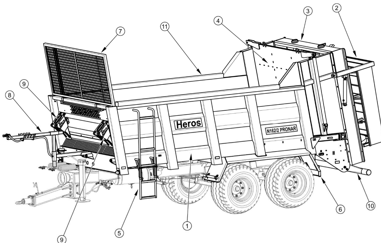
РИСУНОК 3.2 Грузовая платформа
