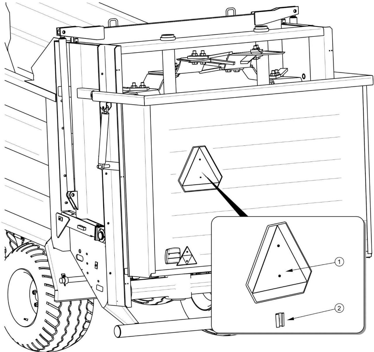
РИСУНОК 2.2 Размещение предупреждающего знака
