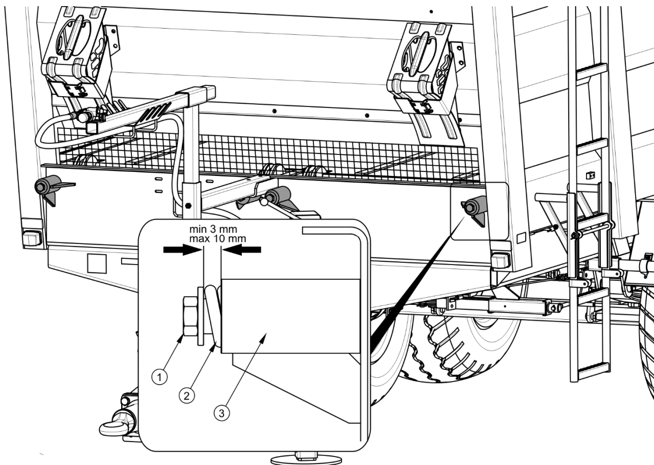
РИСУНОК 5.14 Регулирование натяжения цепи напольного транспортера
