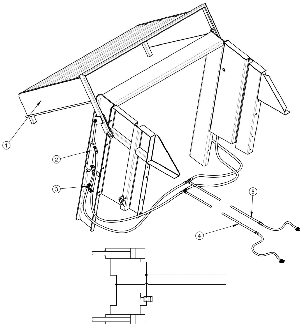
РИСУНОК 3.8 Устройство и схема гидравлической системы заднего борта
