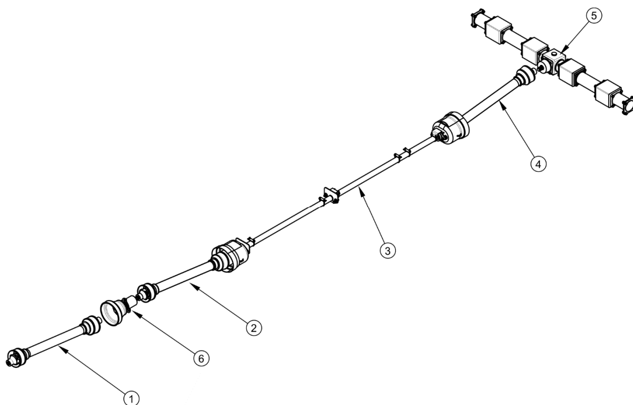
РИСУНОК 3.7 Система передачи привода
