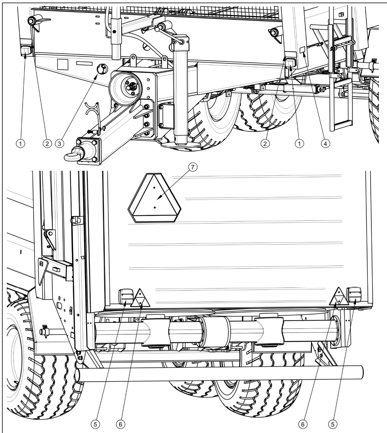
РИСУНОК 3.14 Размещение элементов электрической системы и световой сигнализации
