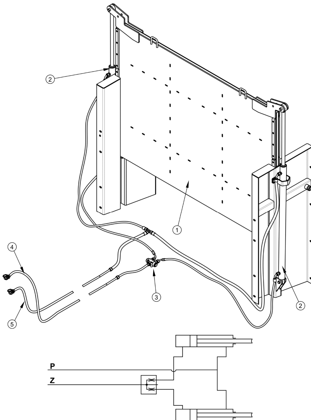
РИСУНОК 3.9 Устройство и схема гидравлической системы заслонки
