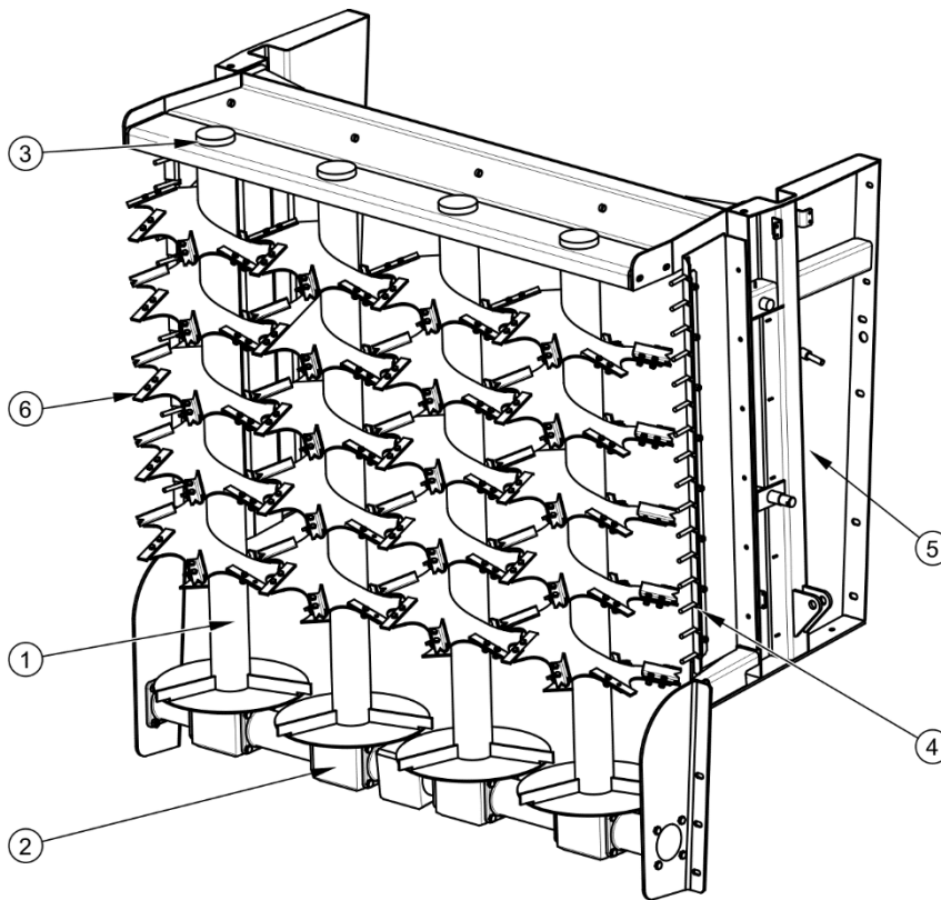
РИСУНОК 3.6 Четырехвальцовый измельчающий адаптер
