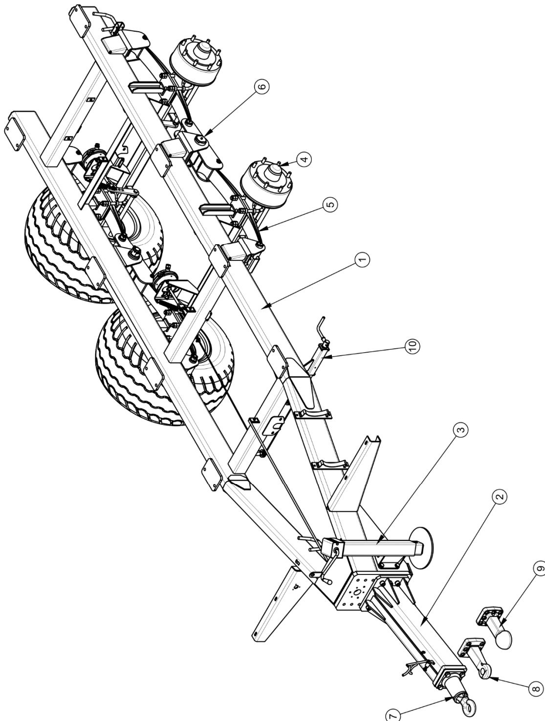
РИСУНОК 3.1 Шасси разбрасывателя
