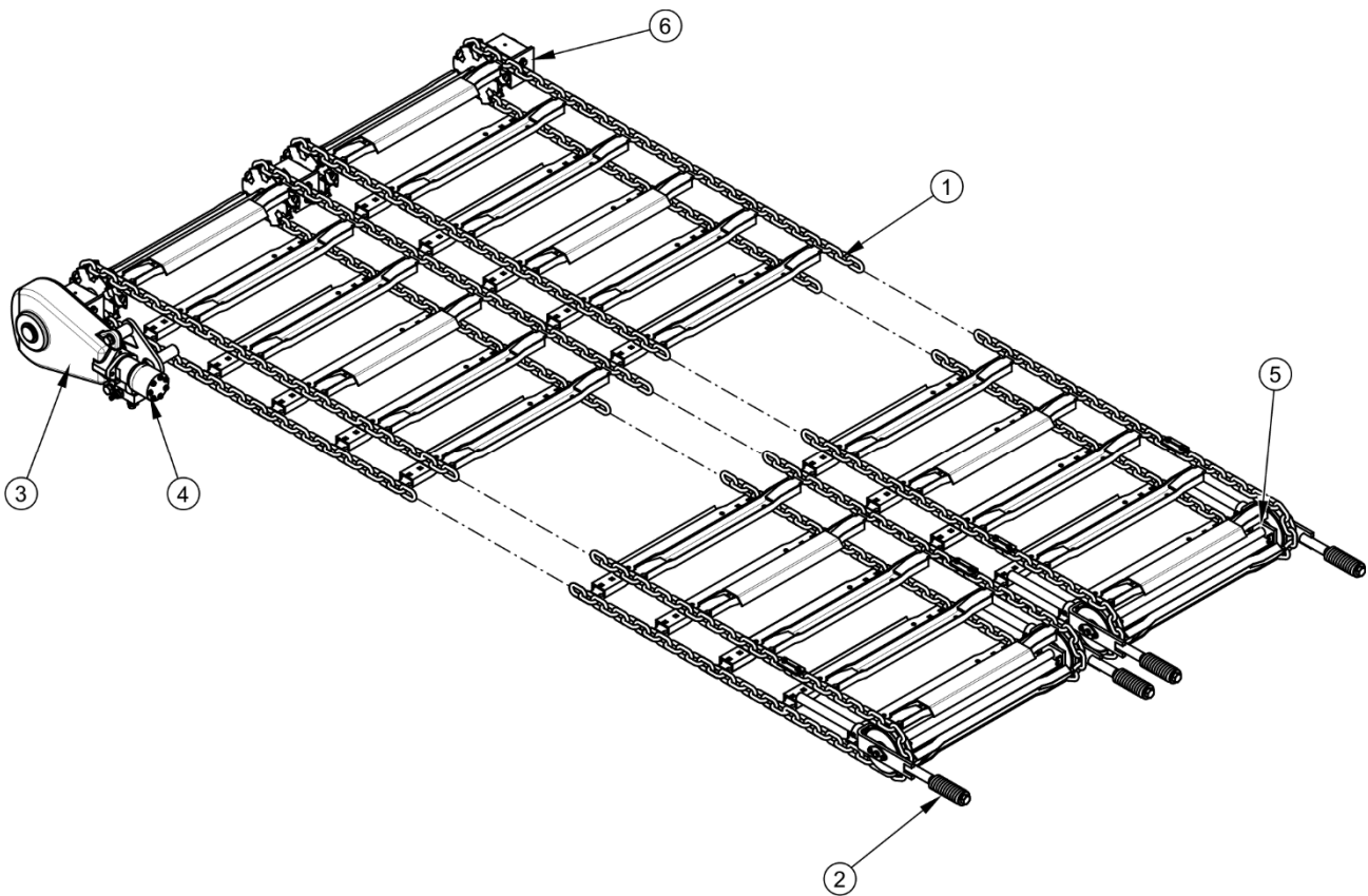
РИСУНОК 3.3 Подающий механизм
