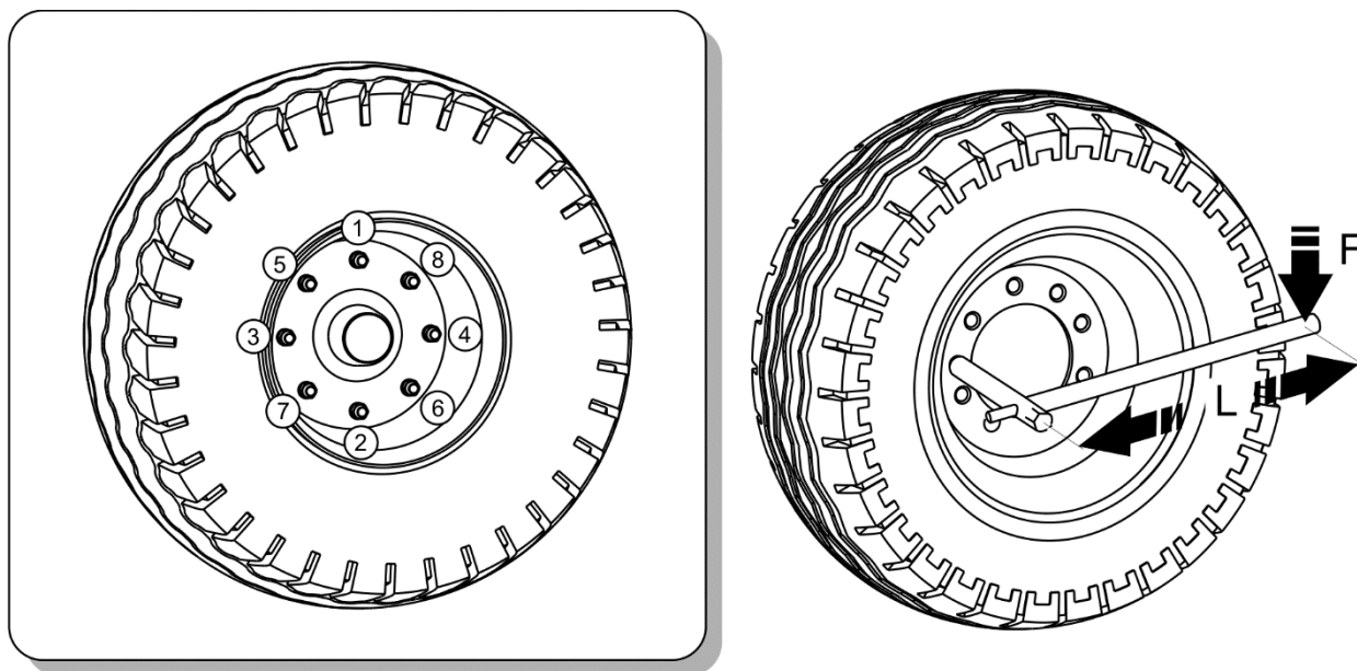
РИСУНОК 5.4 Очередность затяжки гаек, оси с 8 шпильками M22x1.5
