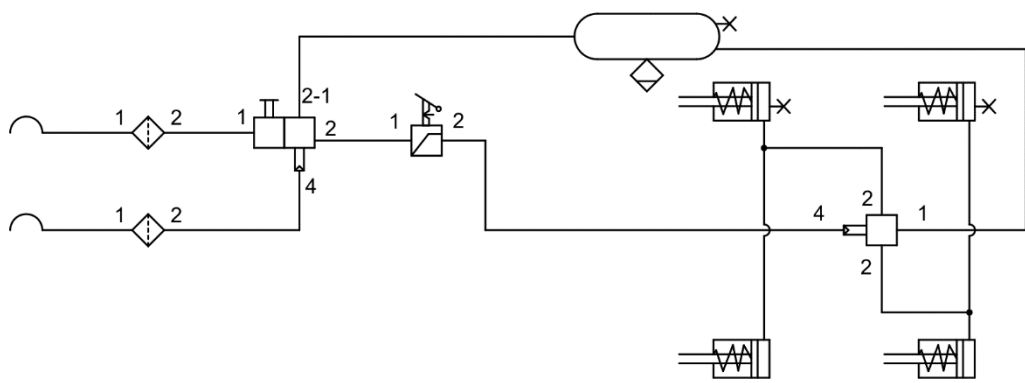
РИСУНОК 3.11 Двухпроводная пневматическая система
