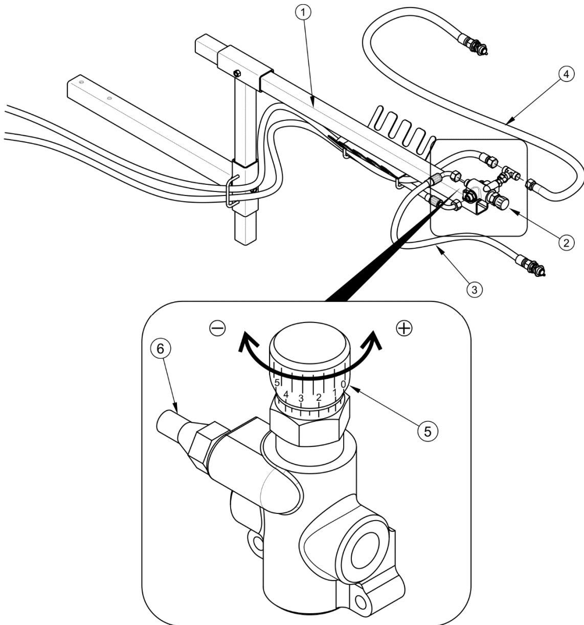
РИСУНОК 4.2 Размещение регулятора протекания
