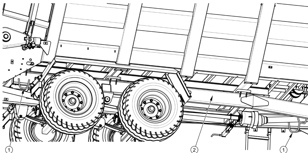
РИСУНОК 1.3 Расположение транспортных захватов
