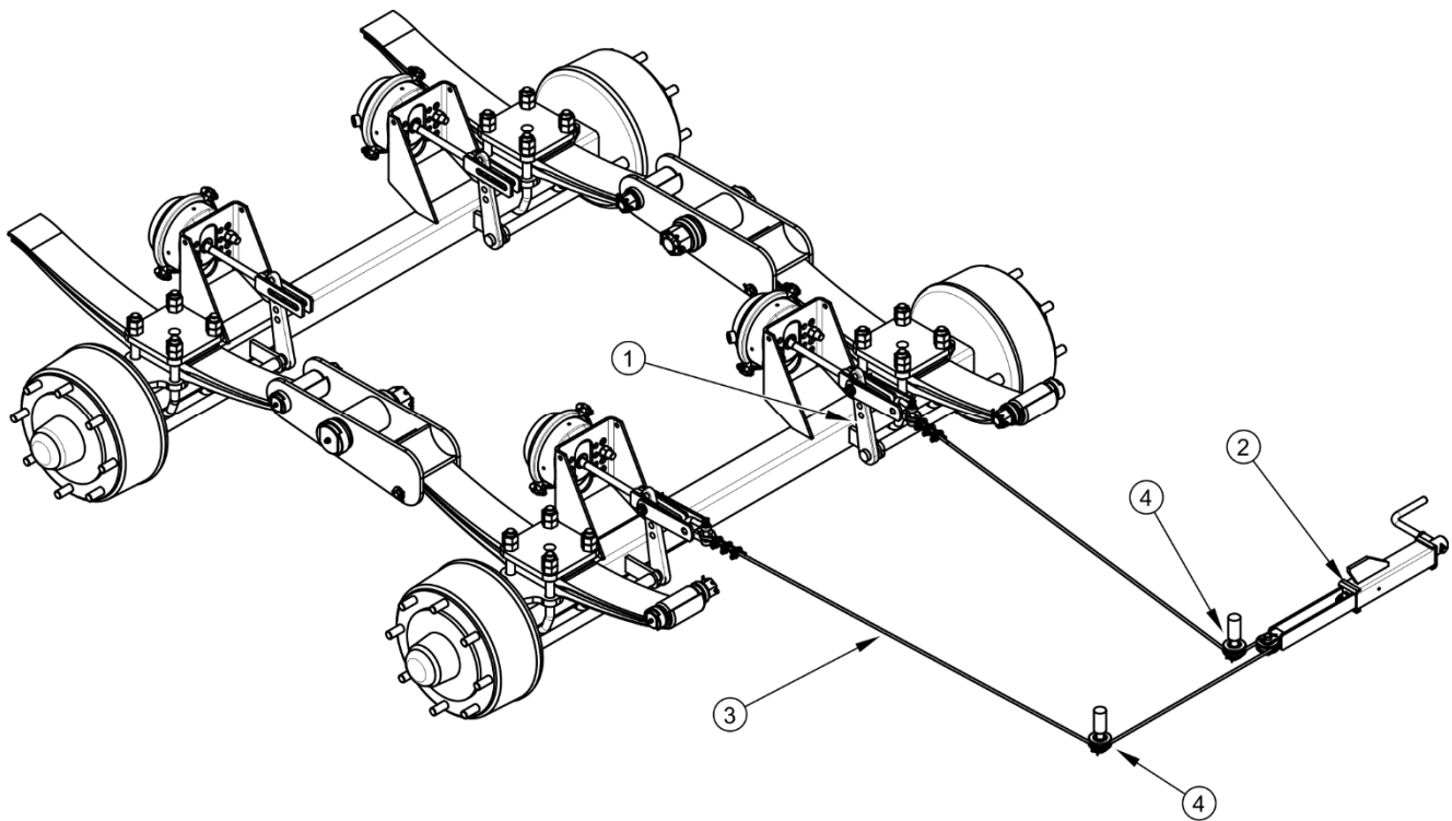
РИСУНОК 3.13 Стояночный тормоз
