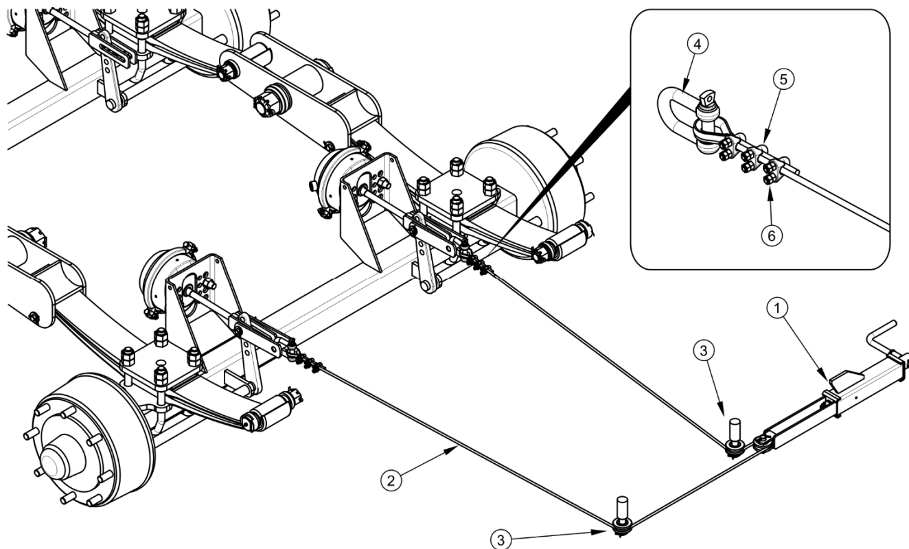
РИСУНОК 5.6 Регулирование натяжения троса стояночного тормоза
