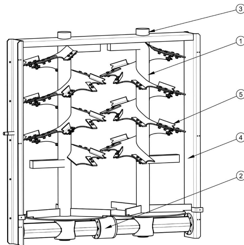
РИСУНОК 3.5 Двухвальный измельчающий адаптер
