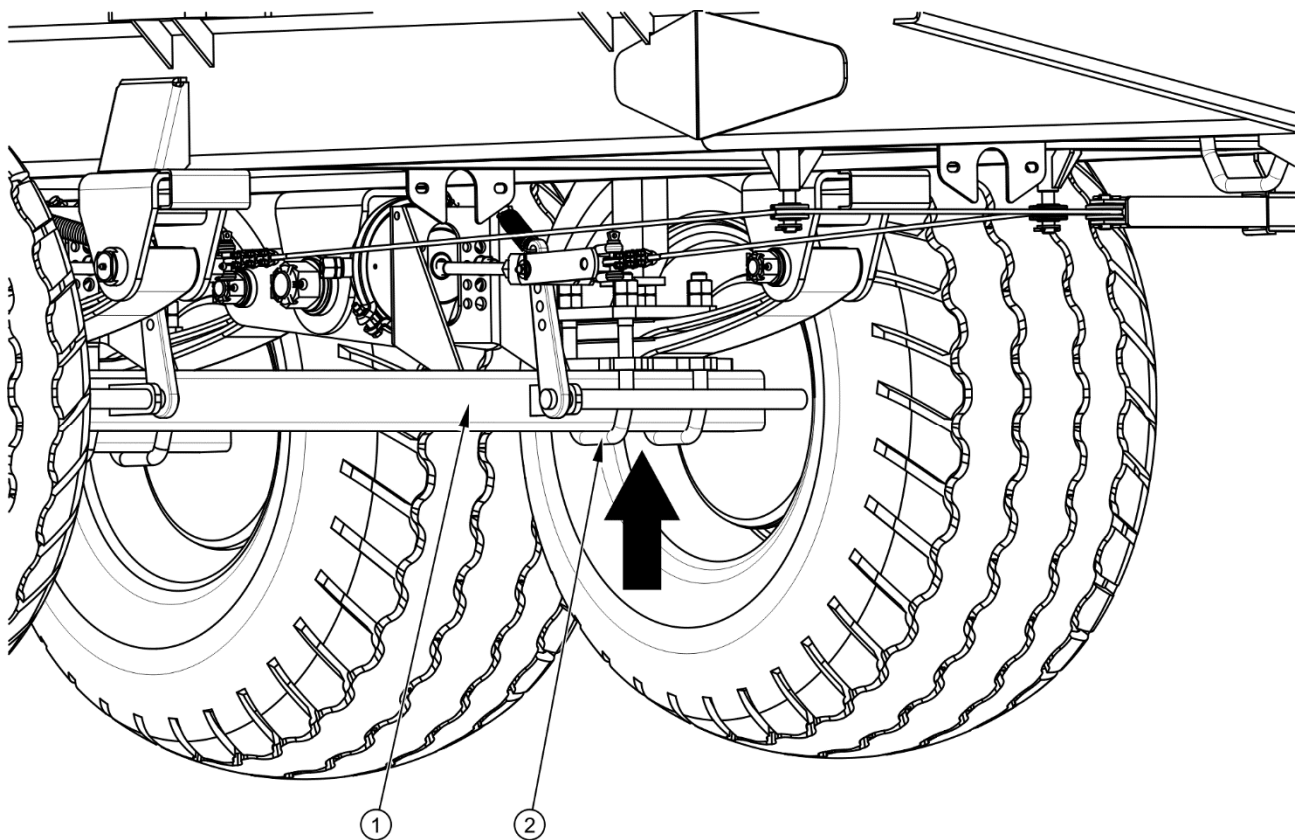
РИСУНОК 5.2 Точка поддомкрачивания
