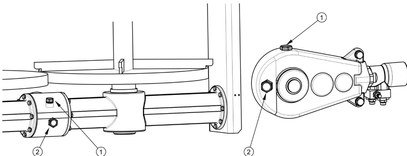
РИСУНОК 5.11 Контрольные точки и места заливки масла в редукторных передачах
