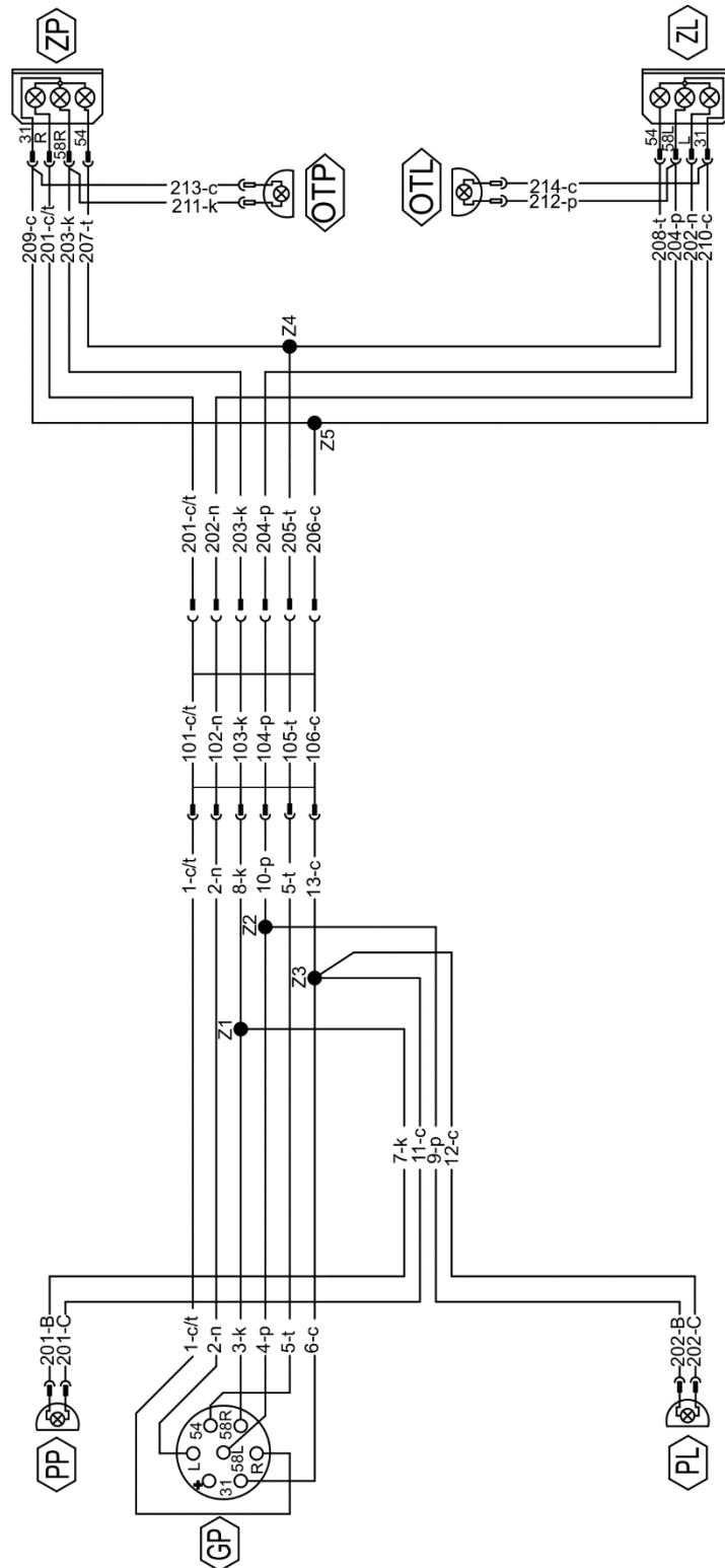
РИСУНОК 3.15 Схема электрической системы
