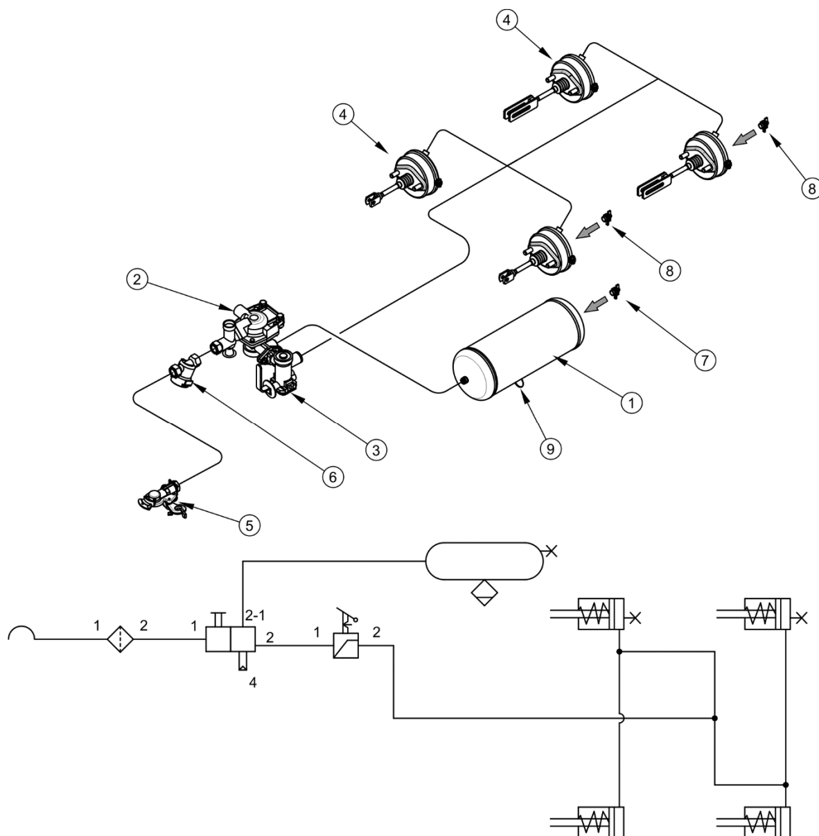
РИСУНОК 3.10 Однопроводная пневматическая система
