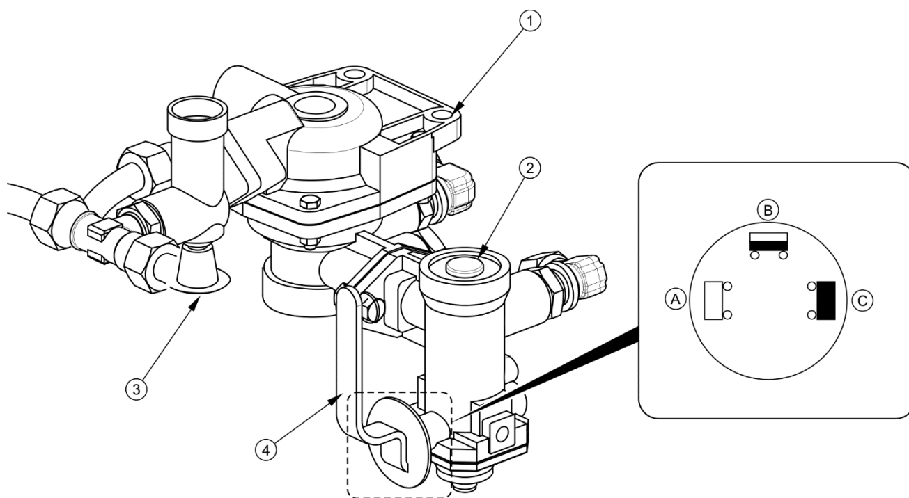
РИСУНОК 3.12 Управляющий клапан и регулятор силы торможения
