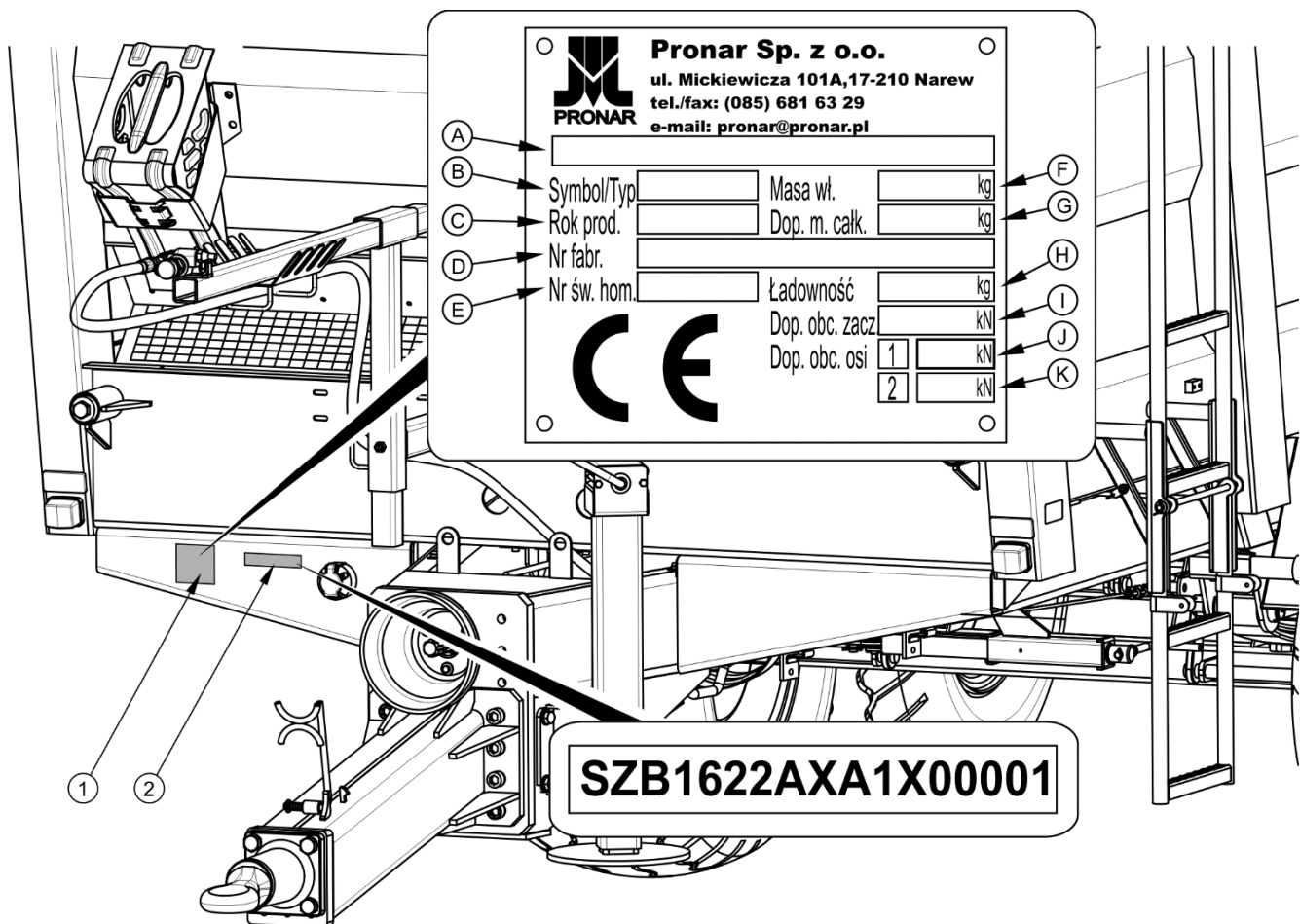
РИСУНОК 1.1 Идентификация разбрасывателя навоза
