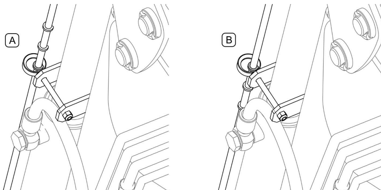
РИСУНОК 4.13 Датчик высоты подъема рабочего органа
