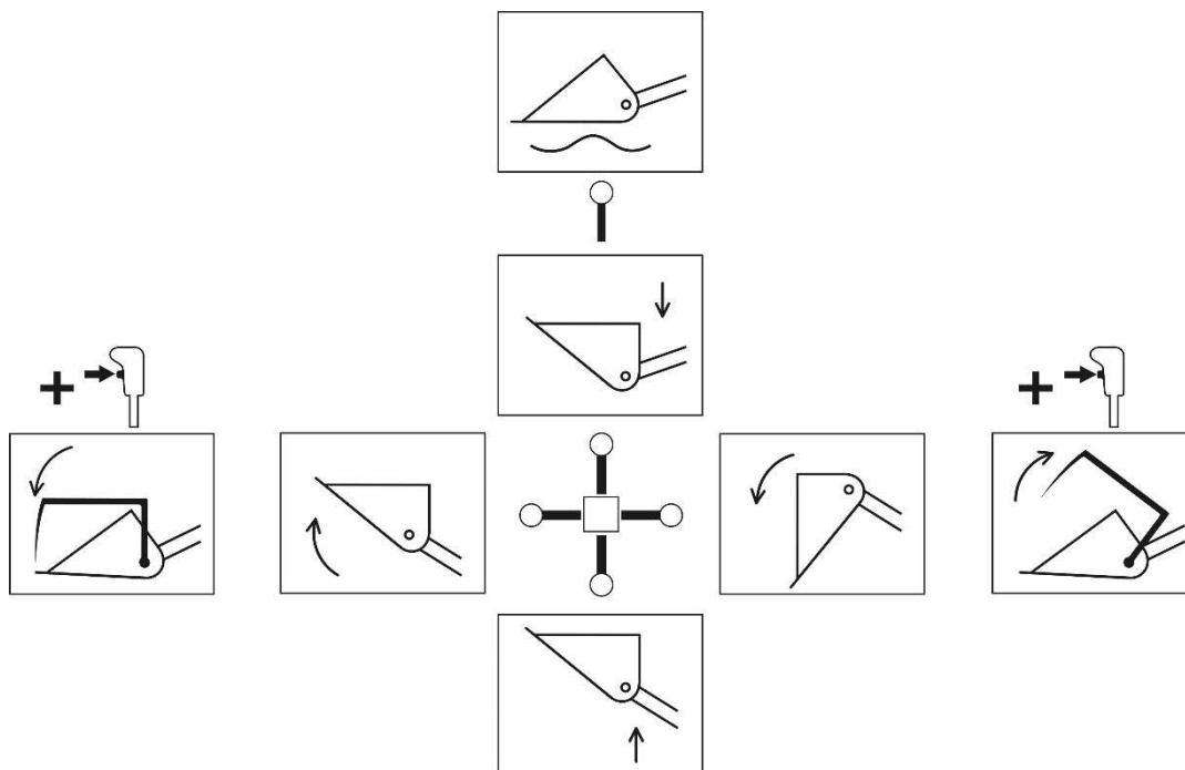
РИСУНОК 4.11 Схема управления погрузчиком
