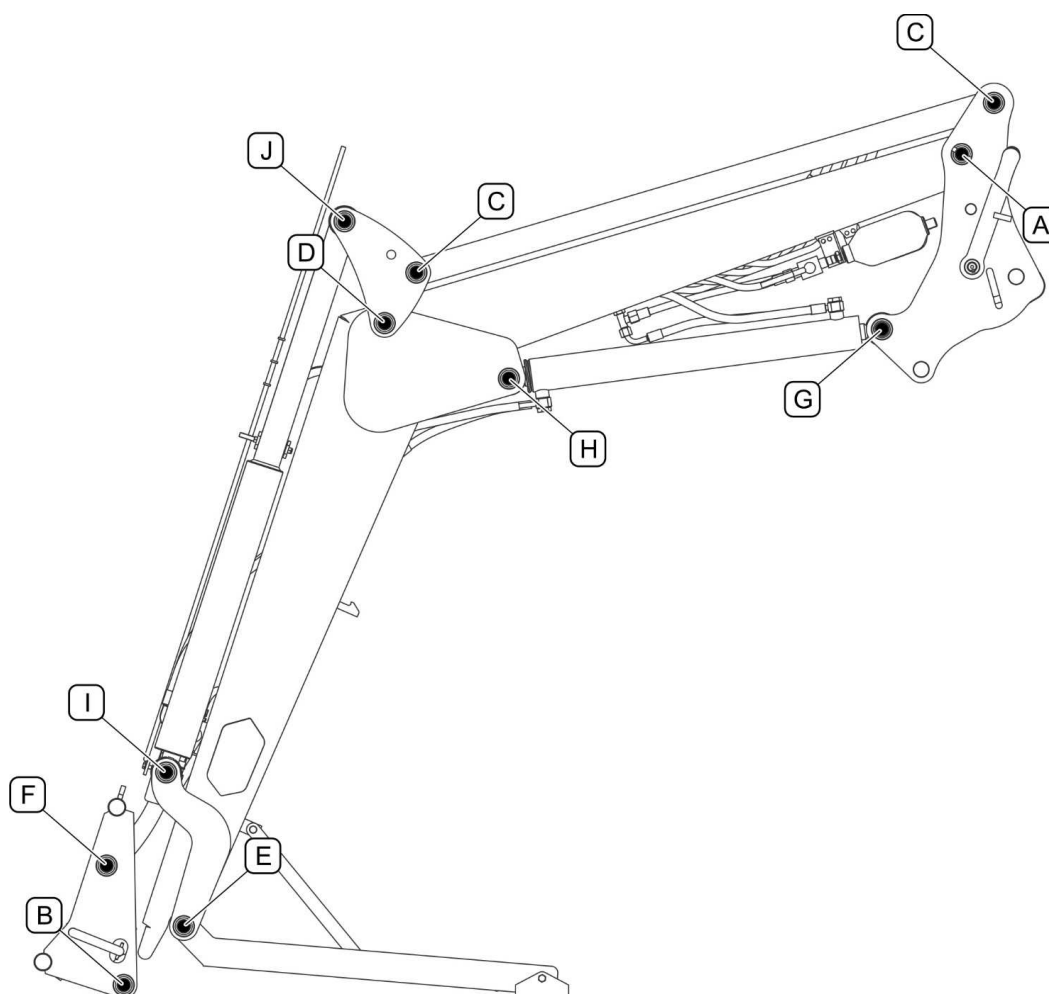
РИСУНОК 5.3 Точки смазки
