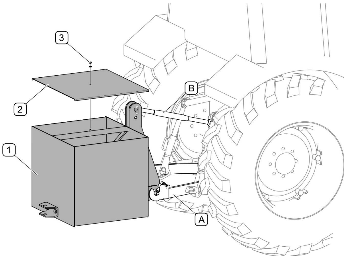
РИСУНОК 4.18 Противовес (опция)
