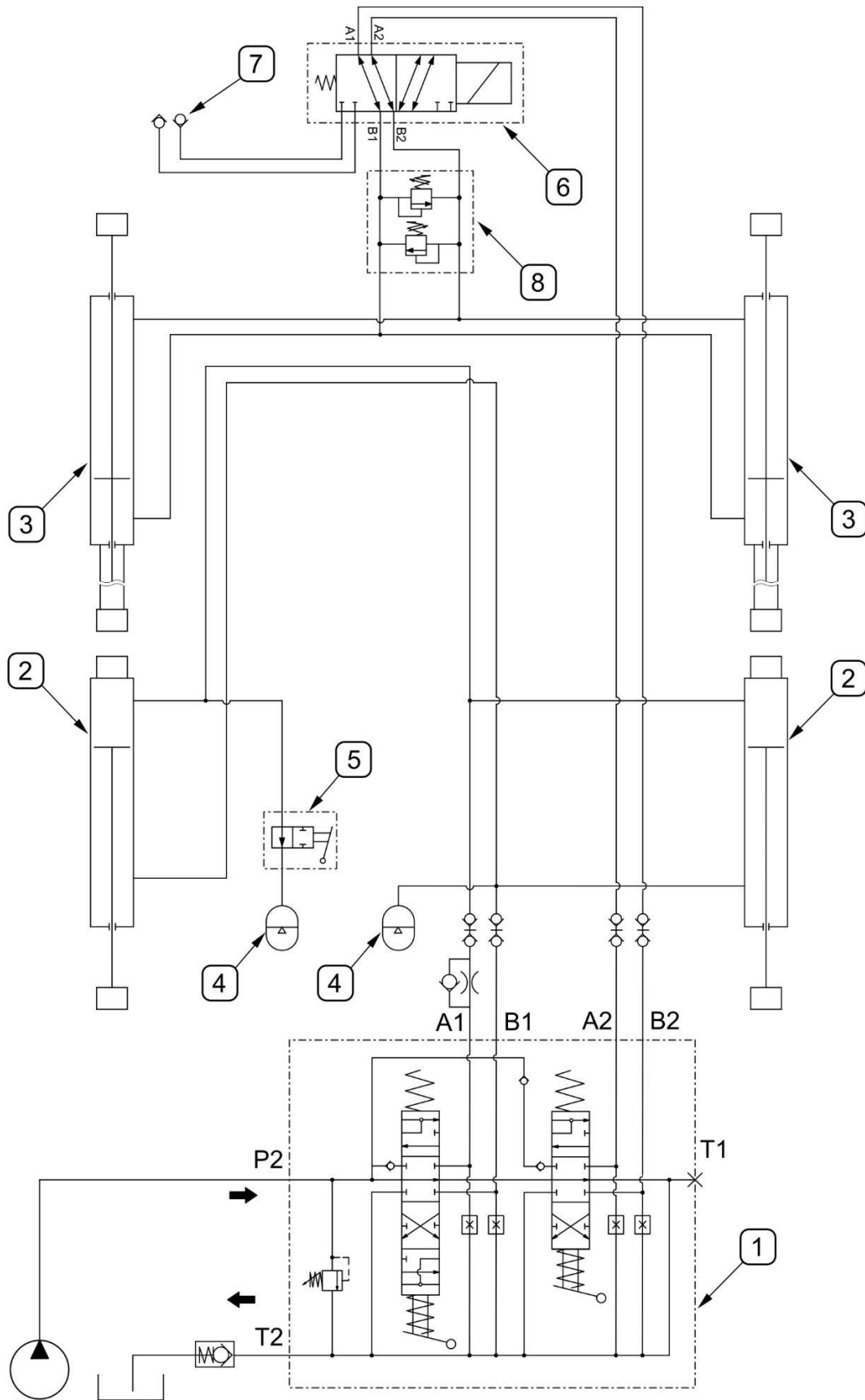
РИСУНОК 3.4 Принципиальная гидравлическая схема погрузчика LC5
