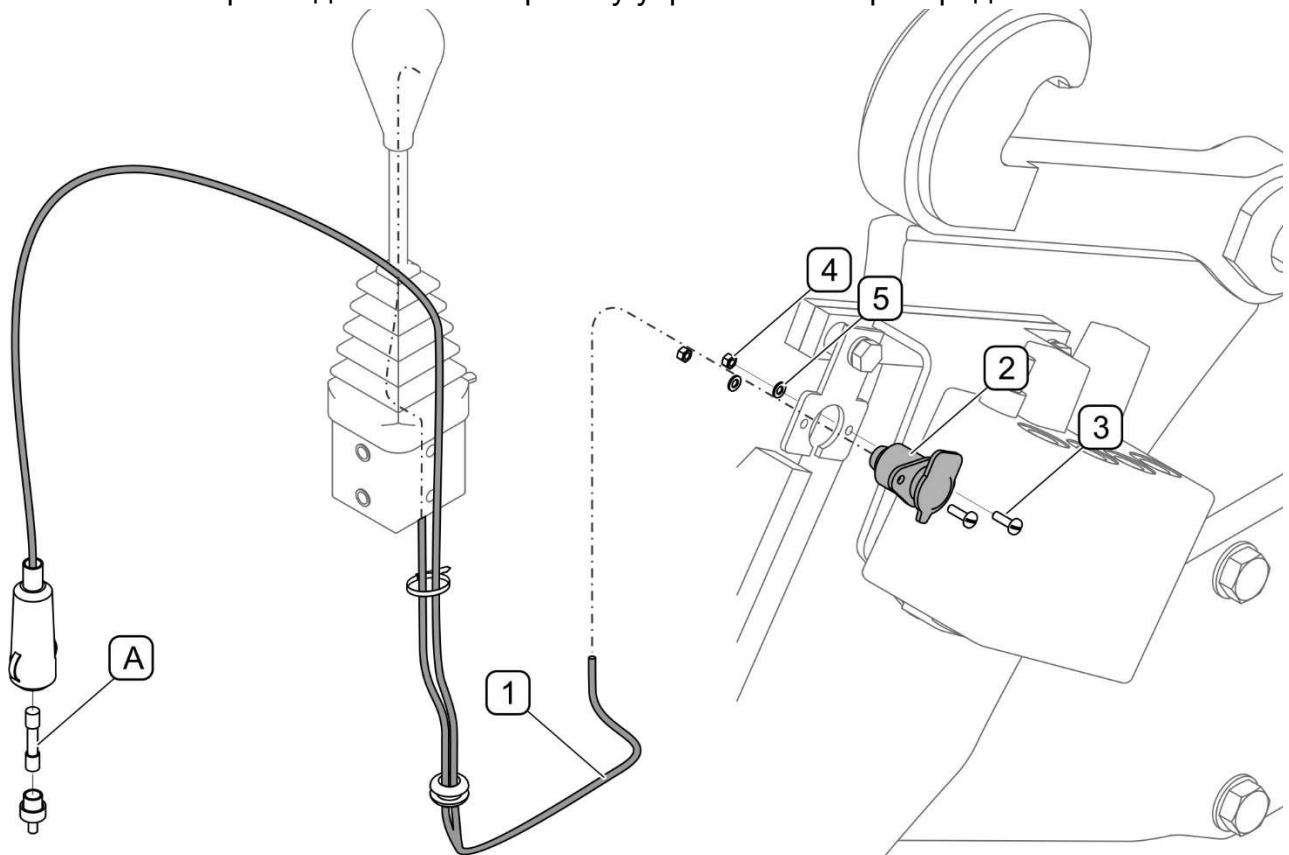
РИСУНОК 4.9 Подсоединение электропитания
