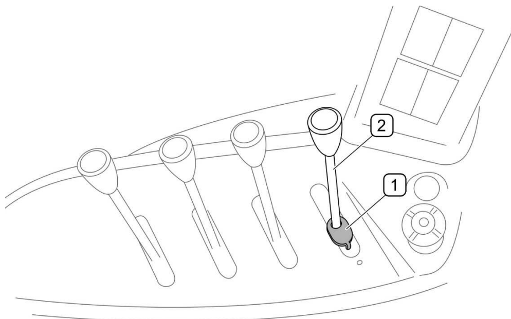
РИСУНОК 4.6 Модификация рычага управления внешней гидравликой трактора (PRONAR 6170)
