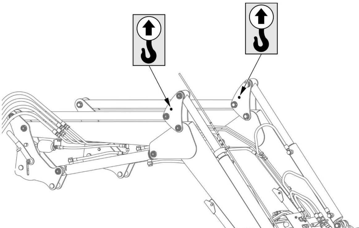
РИСУНОК 1.2 Транспортные захваты
