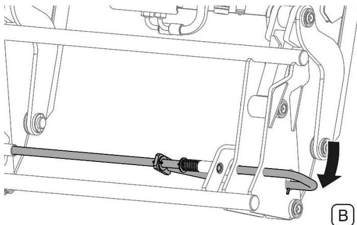
РИСУНОК 4.19 Принцип действия механизма быстрого крепежа
