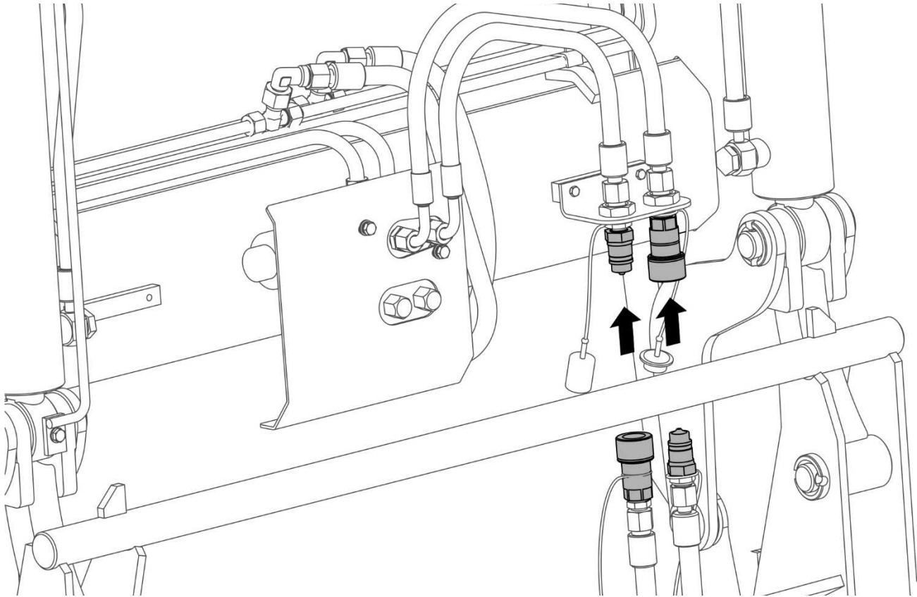
РИСУНОК 4.21 Присоединение гидравлической системы рабочего органа
