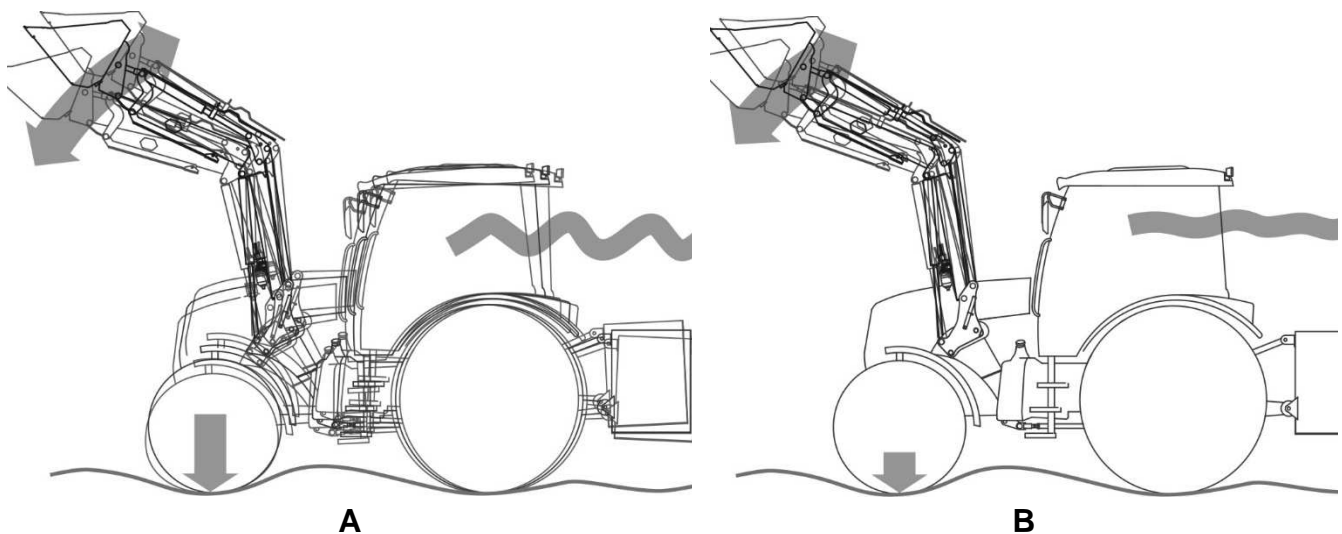
РИСУНОК 4.15 Работа с гидравлическим амортизатором
