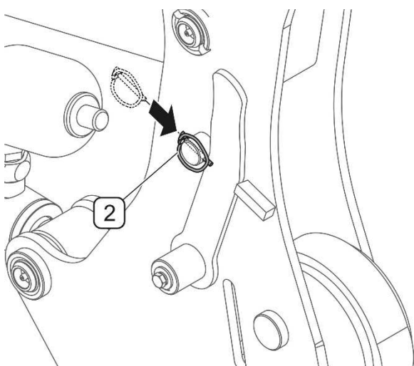
РИСУНОК 4.16 Соединение стрелы с несущей рамой
