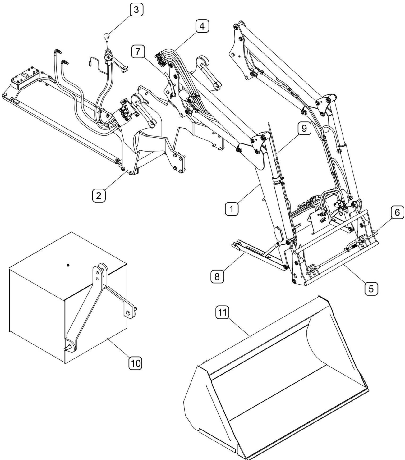
РИСУНОК 3.2 Общее устройство фронтального погрузчика PRONAR LC5
