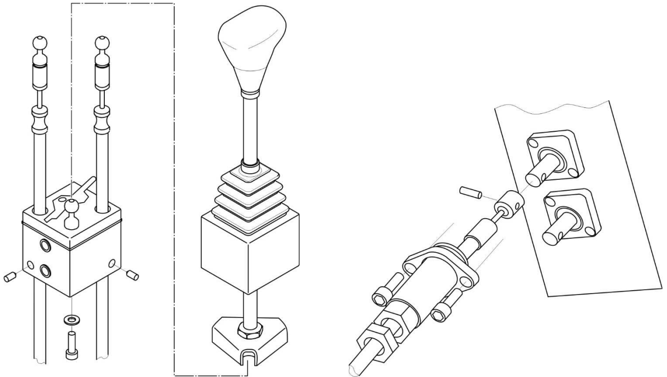
РИСУНОК 4.8 Присоединение тяг к рычагу управления и к распределителю
