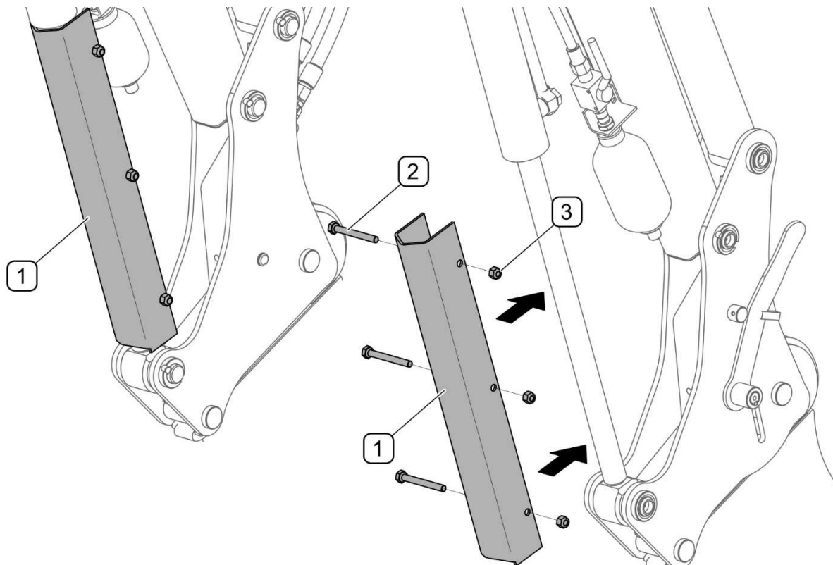
РИСУНОК 5.1 Сервисные блокировки
