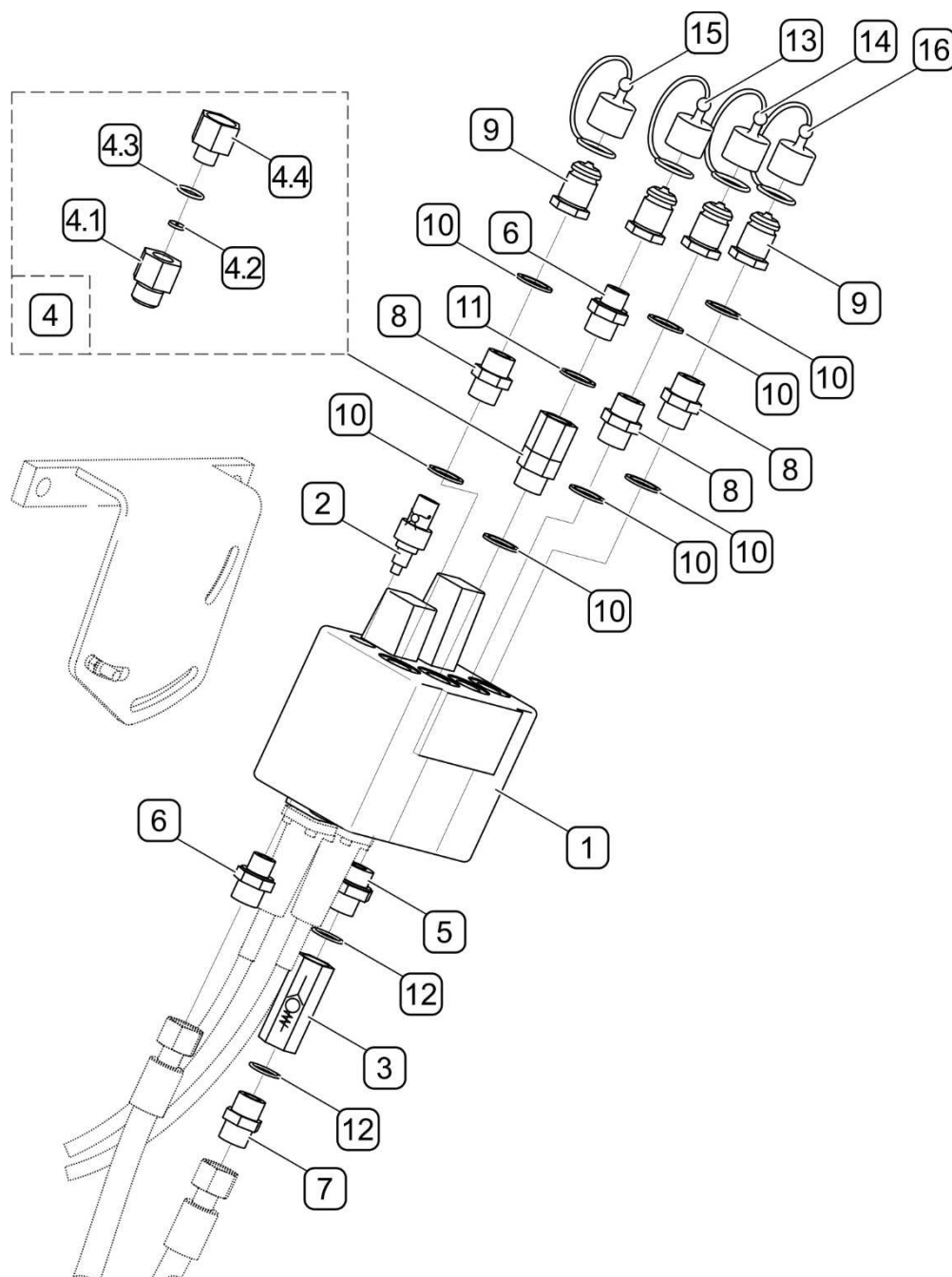
РИСУНОК 4.4 Монтаж распределителя
