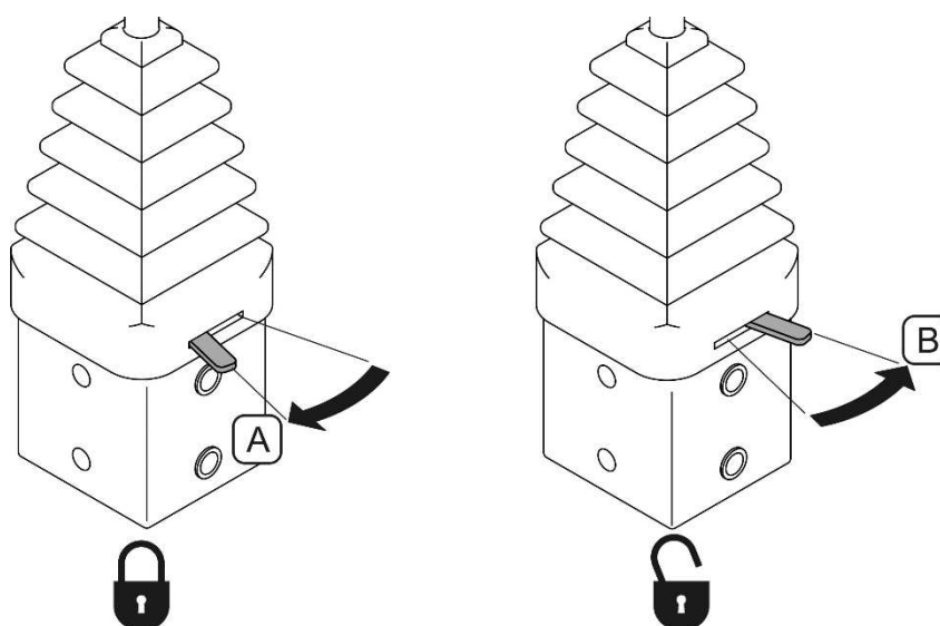
РИСУНОК 4.12 Блокировка рычага управления
