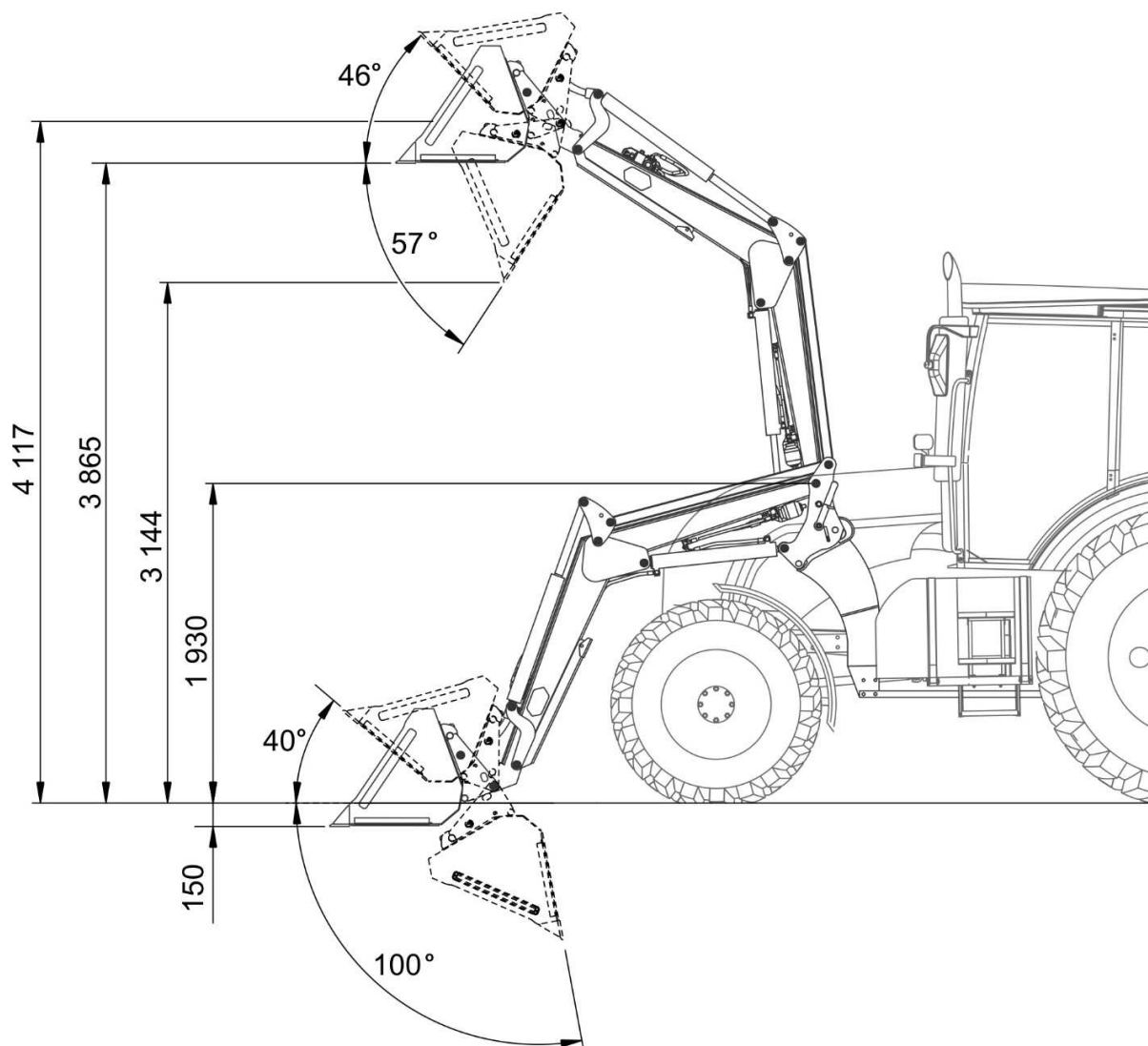
РИСУНОК 3.1 Рабочие положения погрузчика
