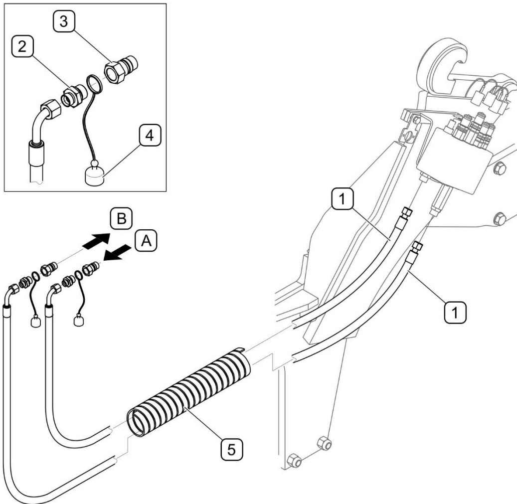
РИСУНОК 4.5 Присоединение распределителя к гидравлической системе трактора (A) - подача масла с задних быстрых разъемов трактора; (B) - возврат масла в систему трактора; (1) - гидропровод 210N-05020200; (2) - корпус муфты GE15LREDOMDCF; (3) - быстроразъемное соединение NV 12 GAS M; (4) - колпачок быстрого разъема; (5) - спиральный шланг SGX-50 L=1500 мм
