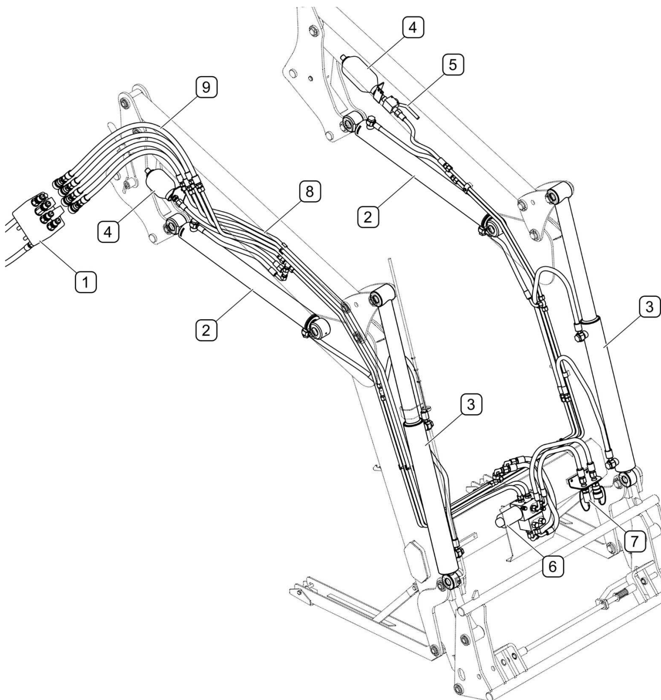
РИСУНОК 3.3 Устройство гидравлической системы фронтального погрузчика LC5
