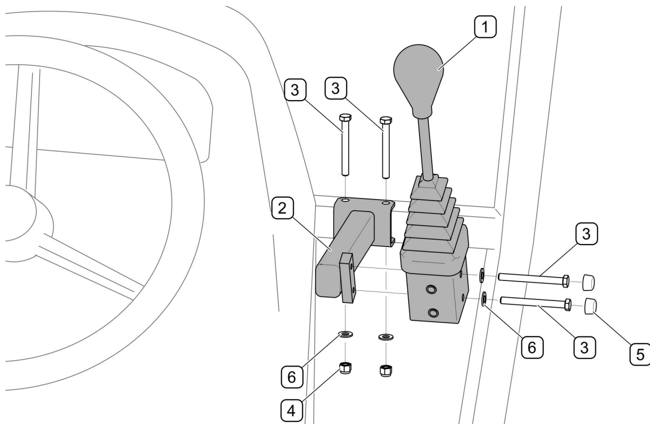
RYSUNEK 4.7 Montaż dźwigni sterowania w kabinie ciągnika (PRONAR 6170)
