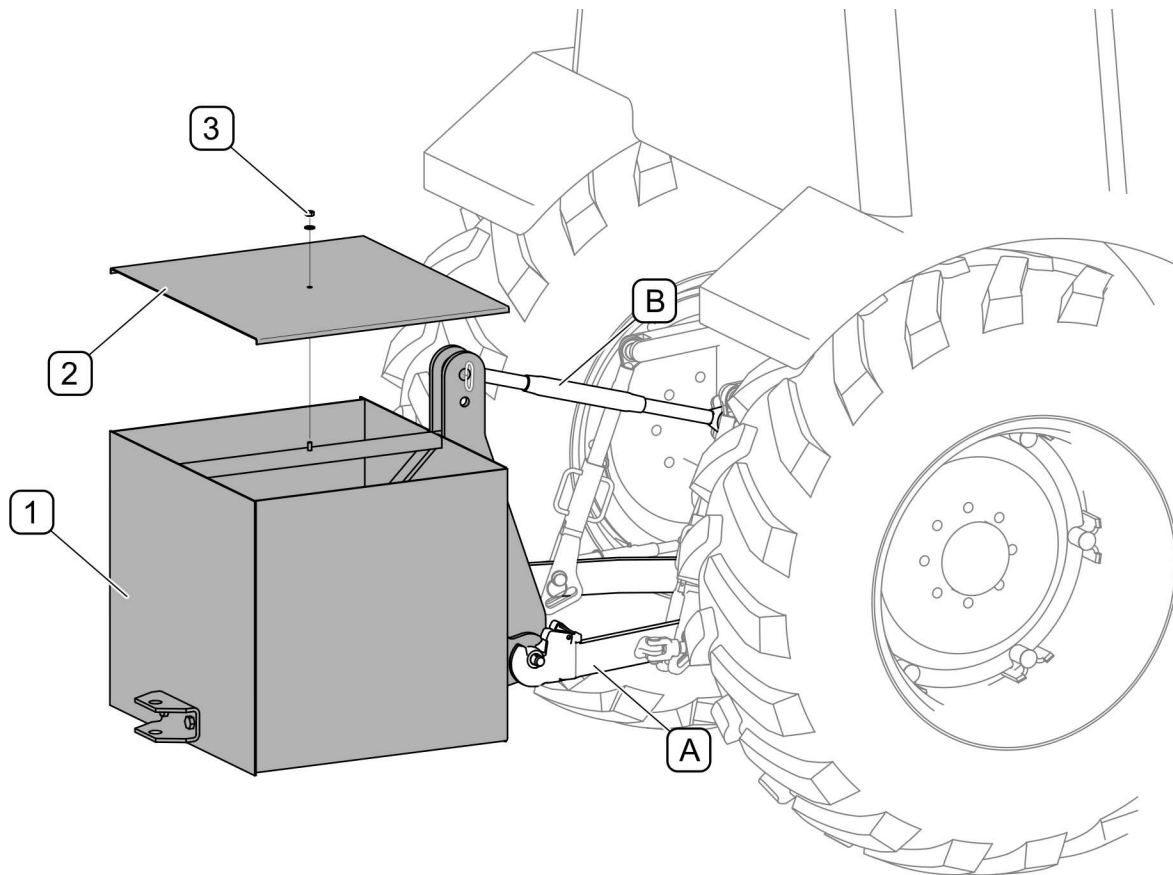
RYSUNEK 4.18 Przeciwcieżar (opcja)
