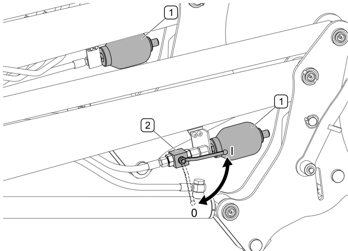
RYСУNEK 4.14 Włączanie amortyzacji hydraulicznej
