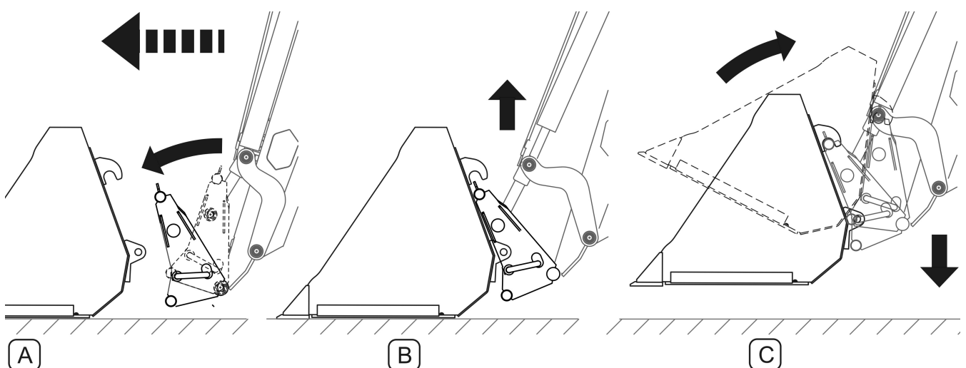
RYСУNEK 4.20 Montaż osprzętu roboczego
