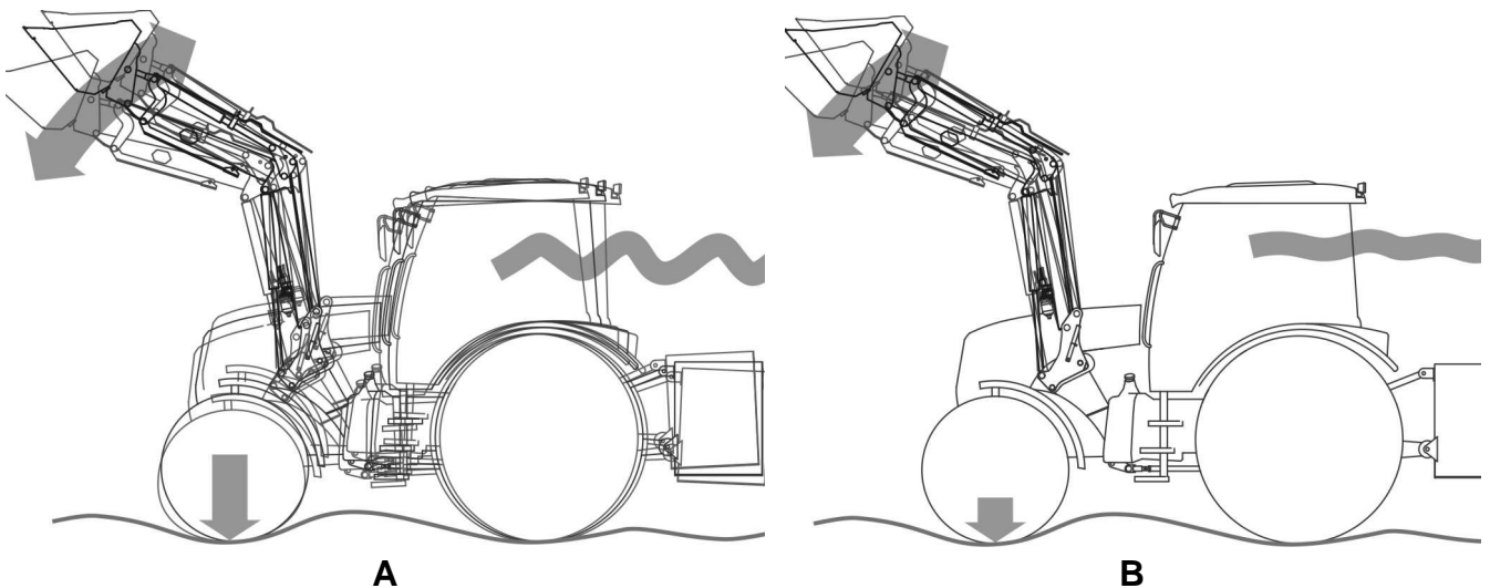
RYСУNEK 4.15 Praca z amortyzatorem hydraulicznym
