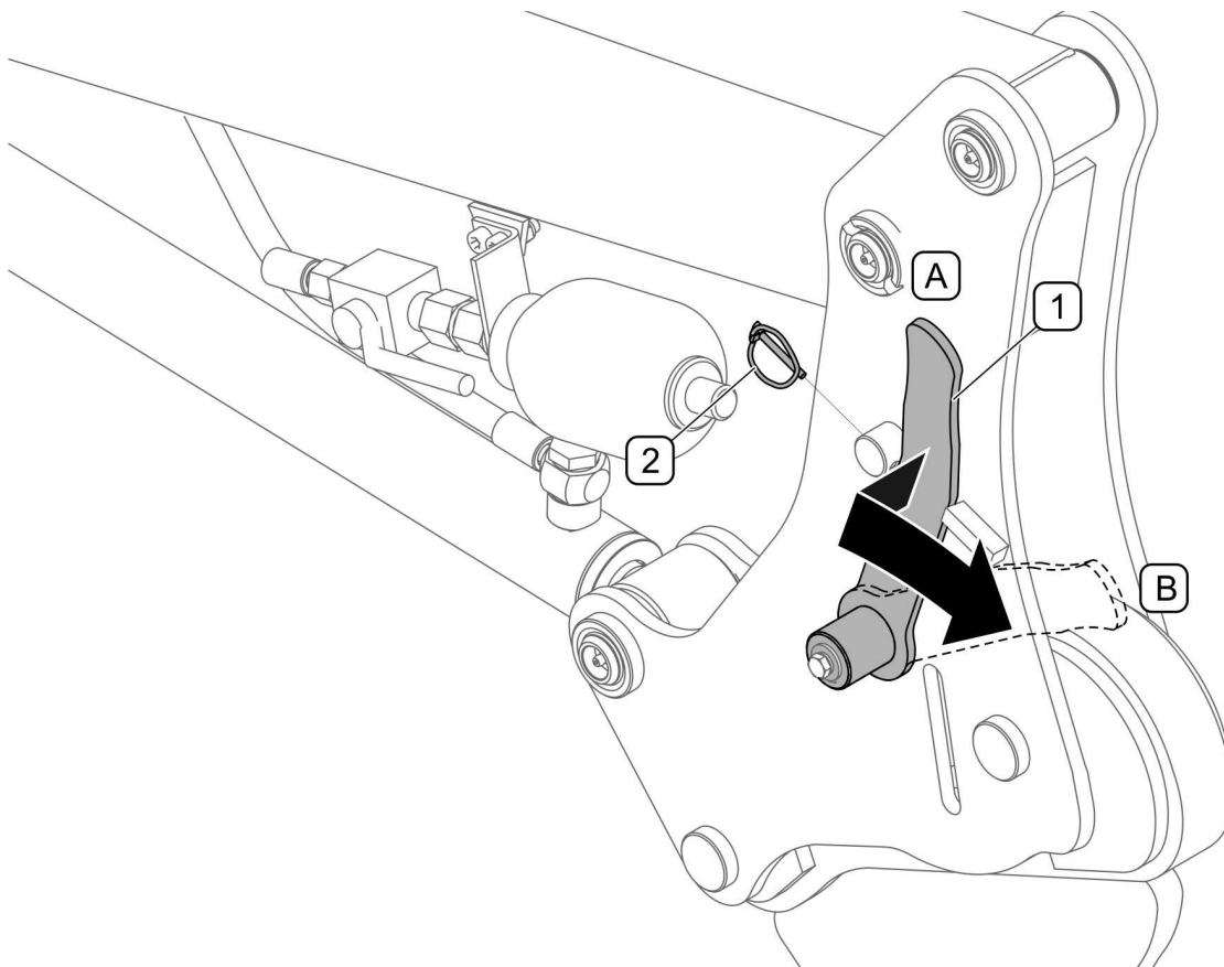
RYSUNEK 4.23 Odłączanie wysięgnika od ramy nośnej
