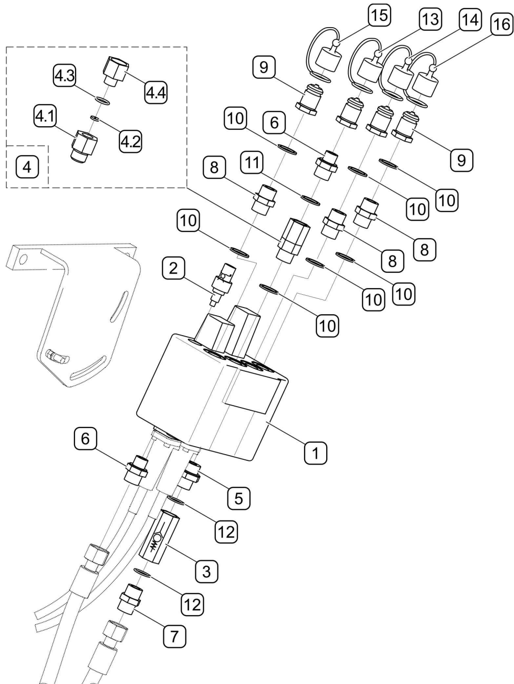
RYSUNEK 4.4 Montaż rozdzielacza
