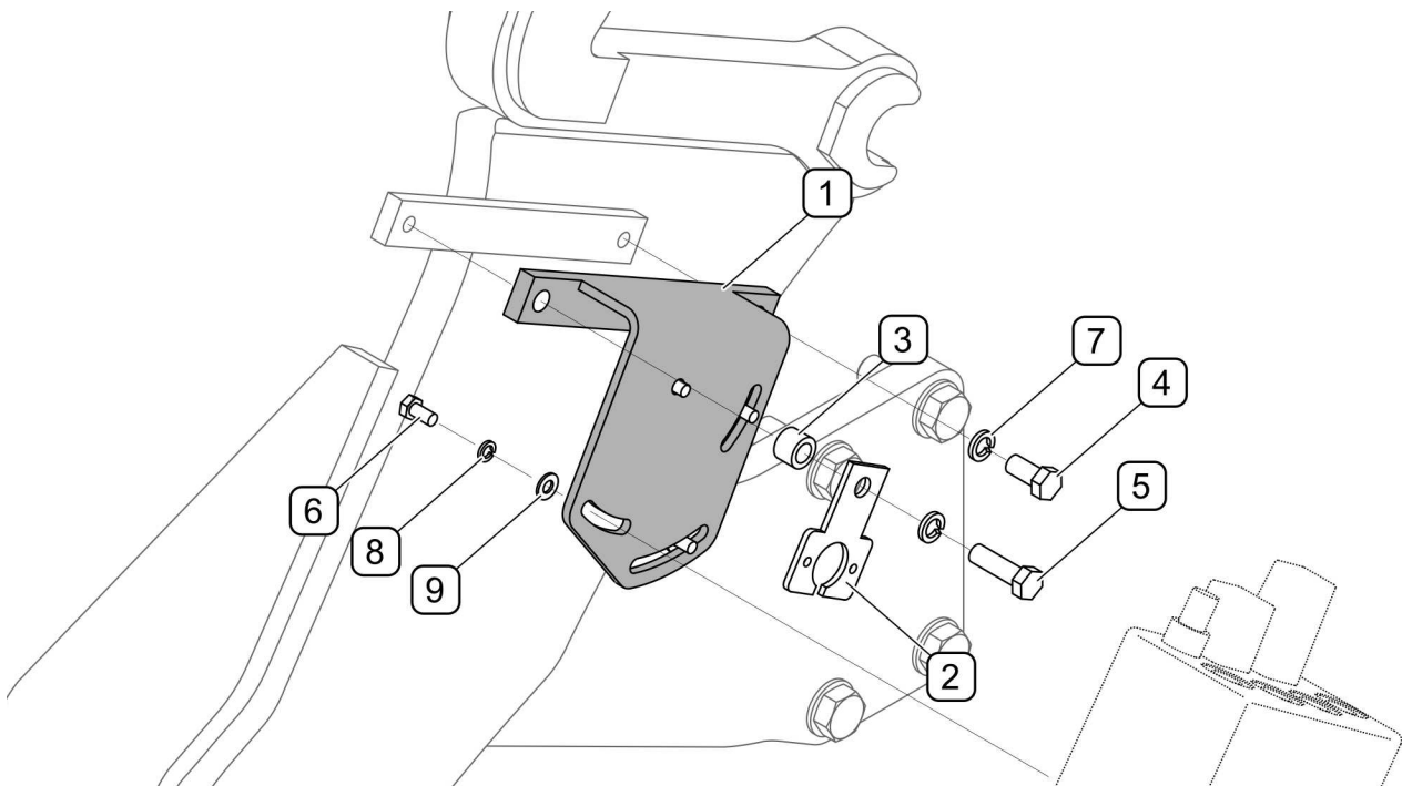
RYSunEK 4.3 Montaż wspornika rozdzielacza do ramy nośnej
