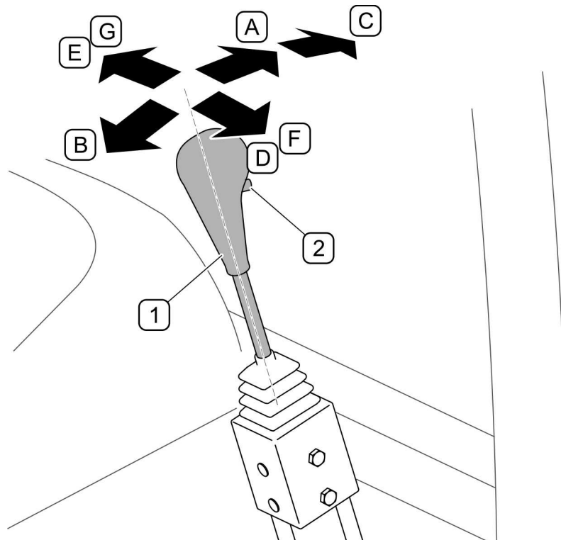
RYSUNEK 4.10 Dźwignia sterowania ładowaczem
