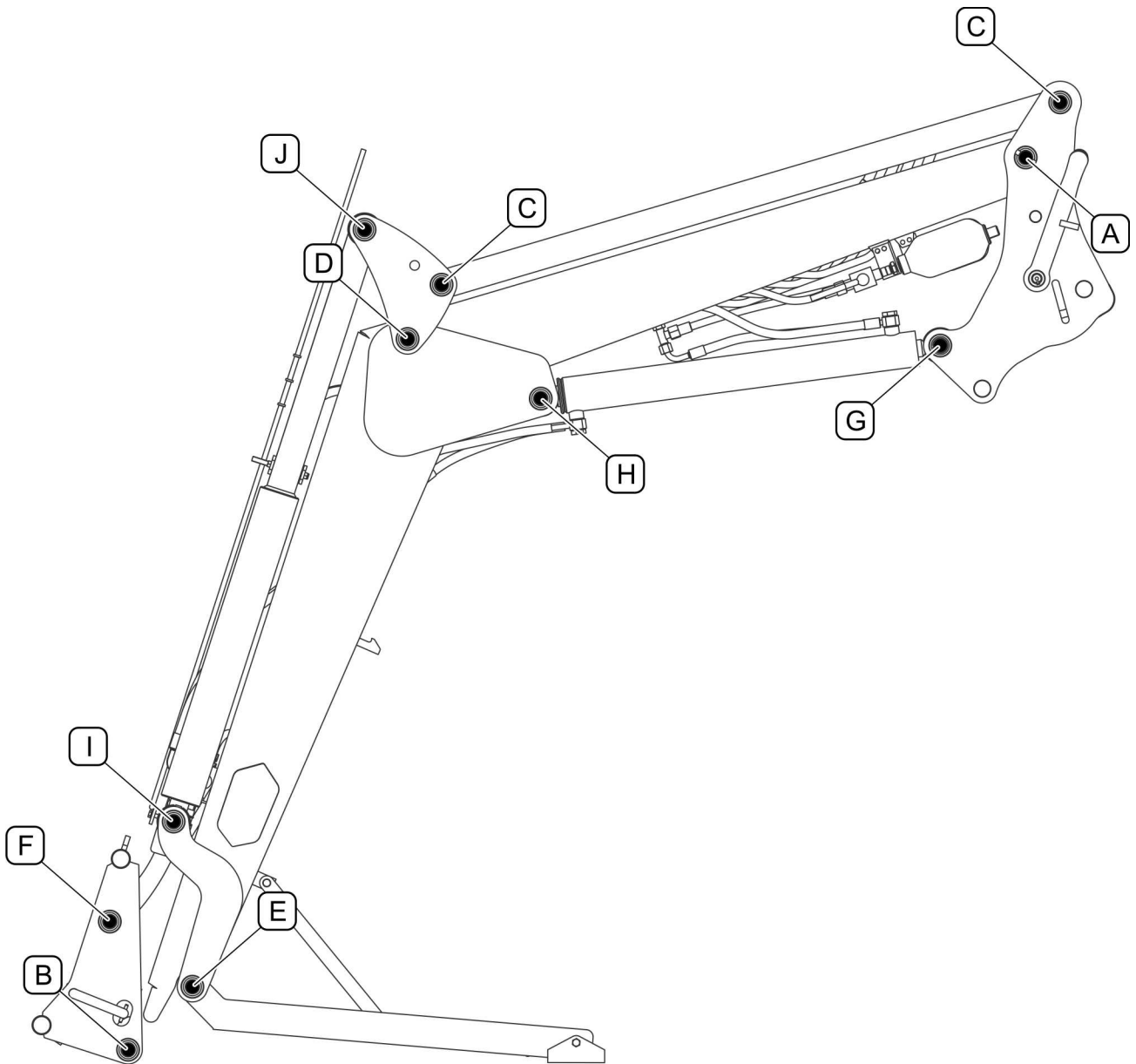
RYSunEK 5.3 Punkty smarowania
