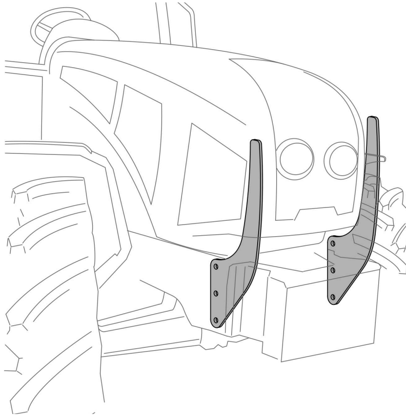
RYSUNEK 4.24 Zderzaki – opcja (PRONAR 6170)
