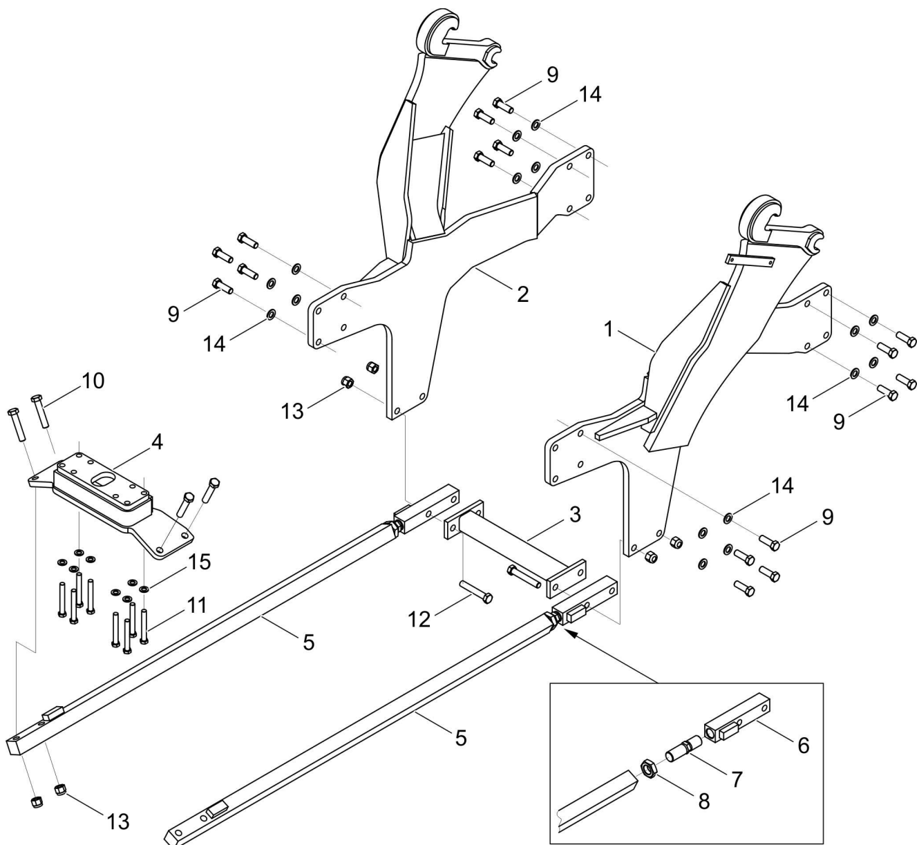
RYSUNEK 4.1 Montaż ramy nośnej (PRONAR 6170)
