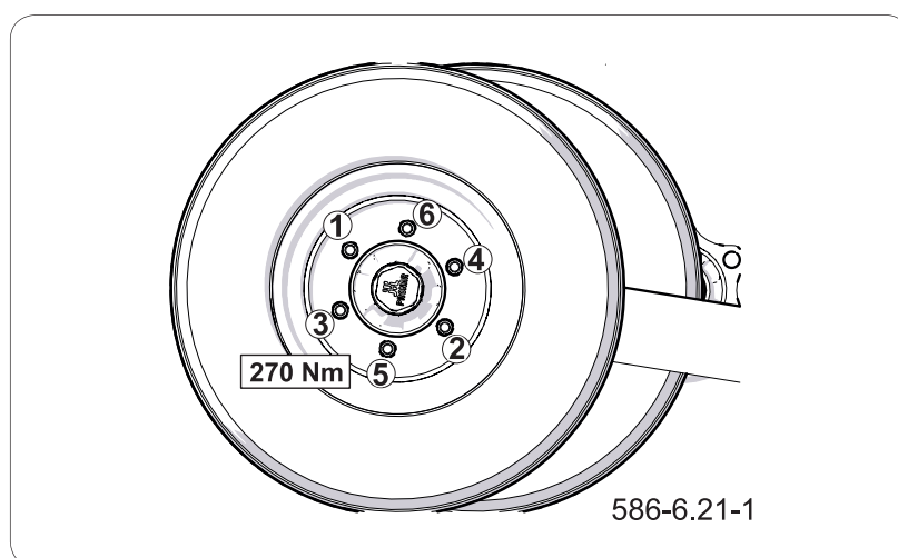
Рисунок 6.4 Очередность затяжки гаек
