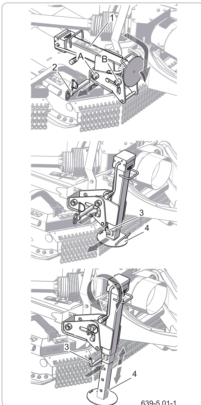
Рисунок 5.4 Механическая опора
