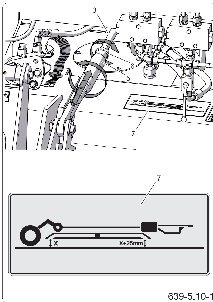
Рисунок 5.3 Регулировка наклона косилки
