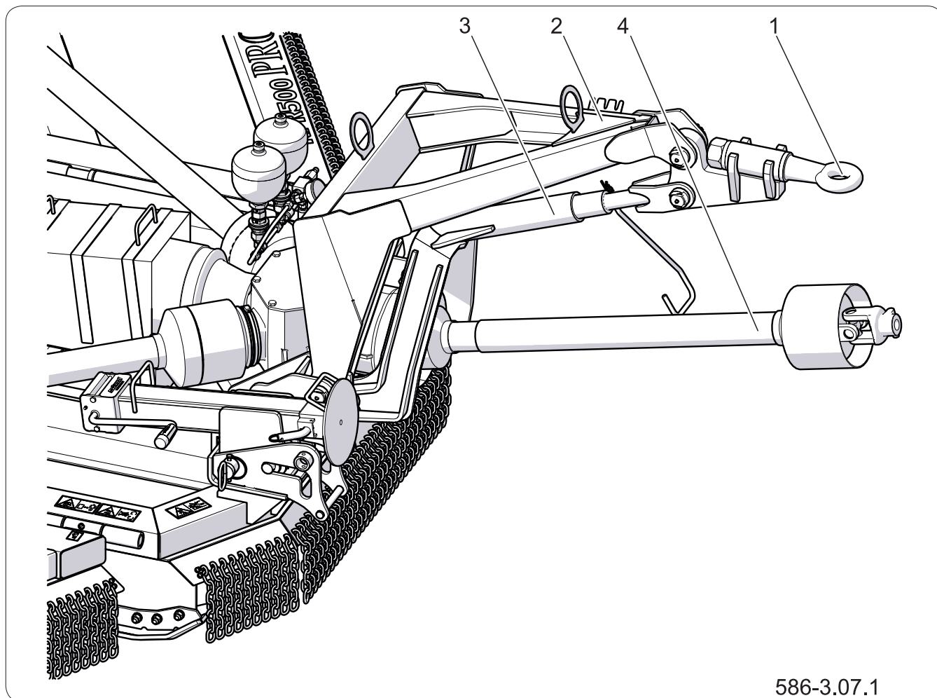
Рисунок 4.5 Верхнее тягово-сцепное устройство
