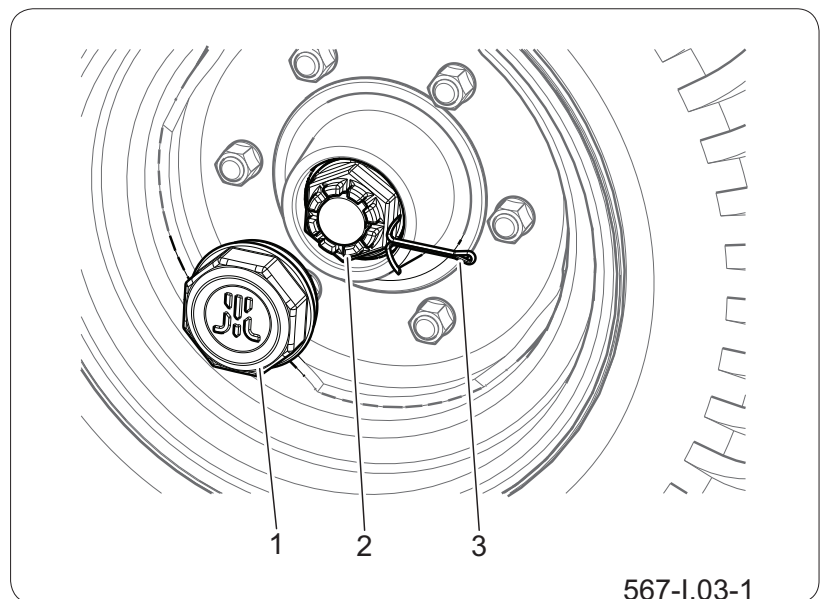
Рисунок 6.7 Регулирование люфта в ходовой оси
