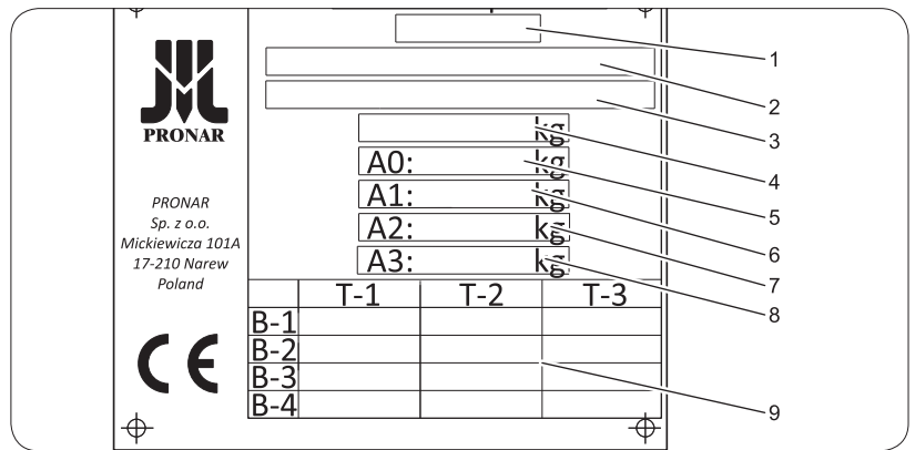
Рисунок 2.2 Заводская табличка ЕС
