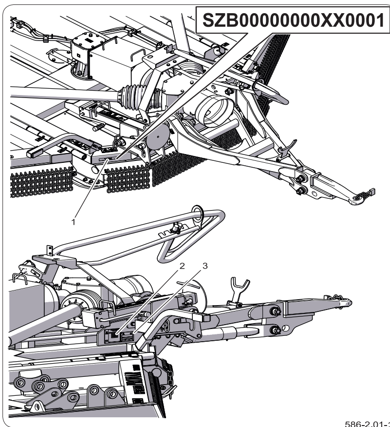
Рисунок 2.1 Идентификация машины
