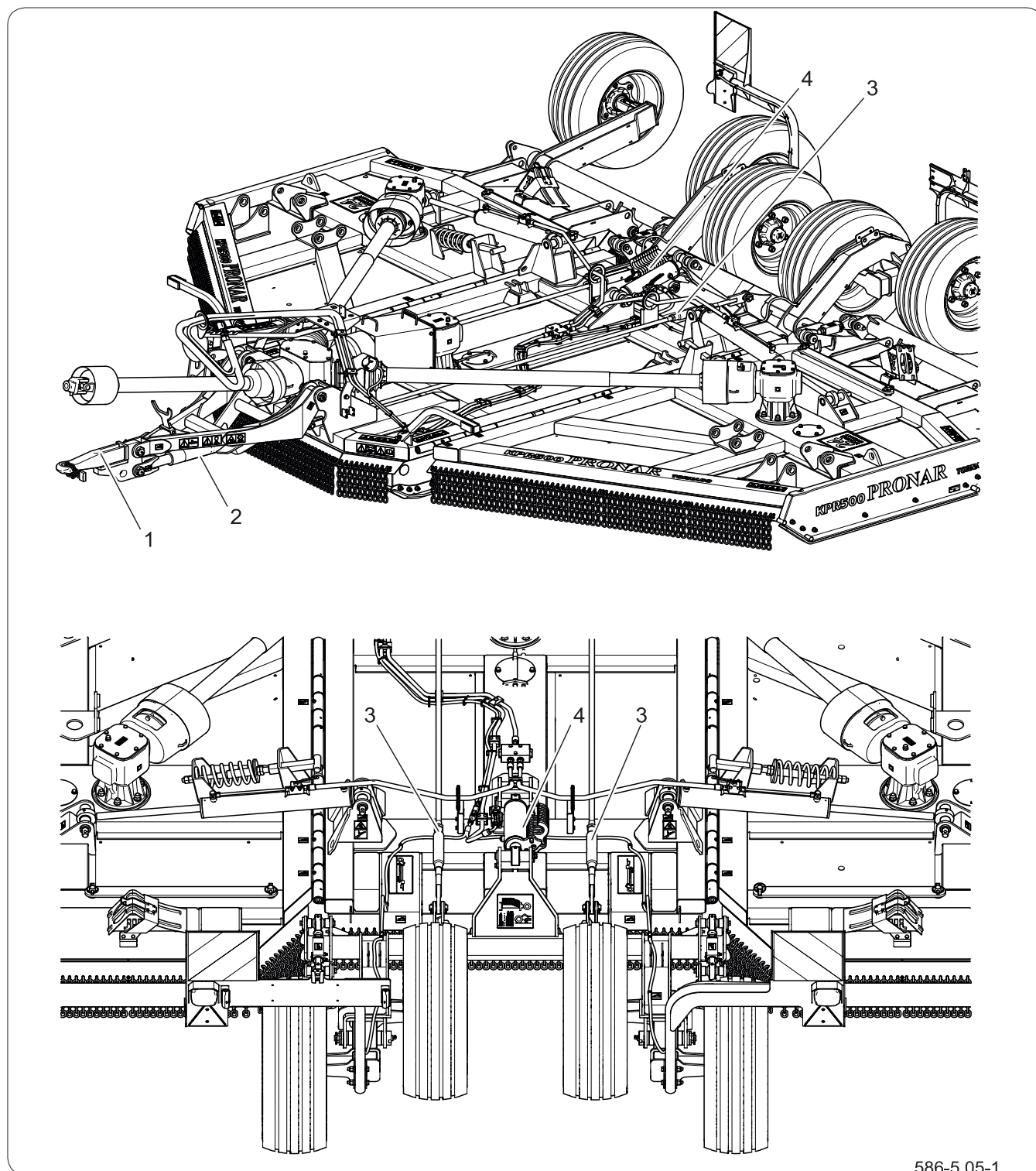
Рисунок 5.1 Регулировка положения машины
