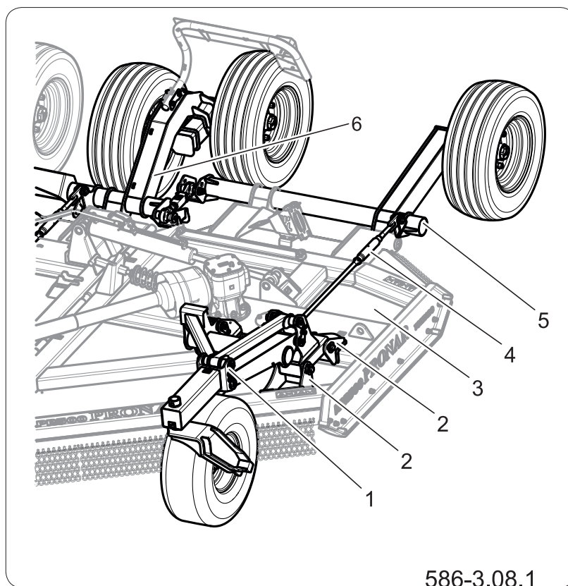
Рисунок 4.6 Передние копирующие колеса
