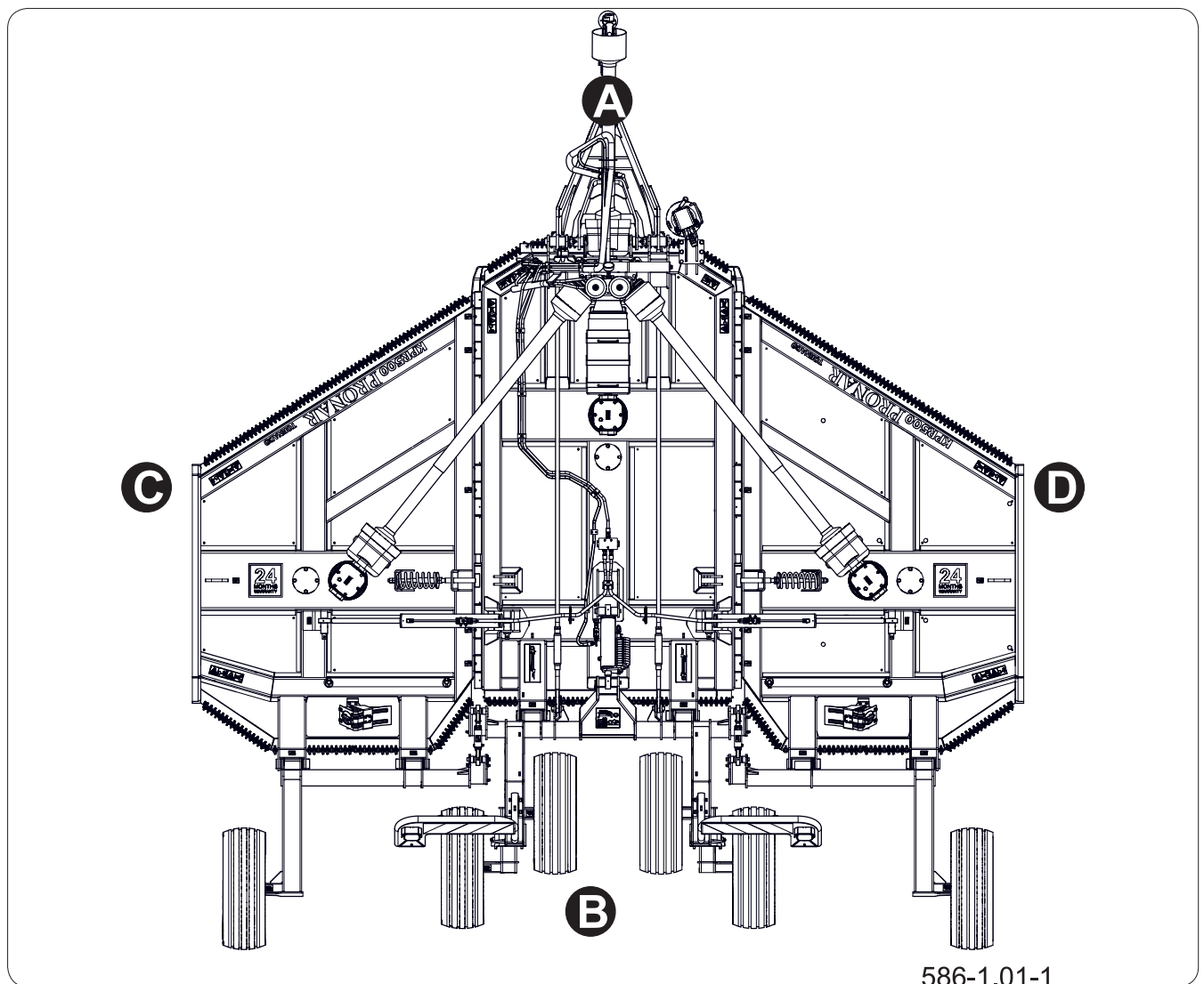
Рисунок 1.1 Определение сторон косилки
