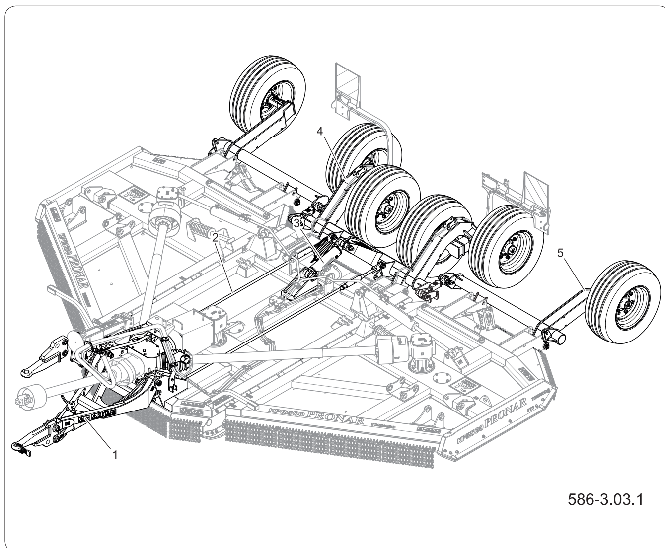
Рисунок 4.1 Устройство системы подвески
