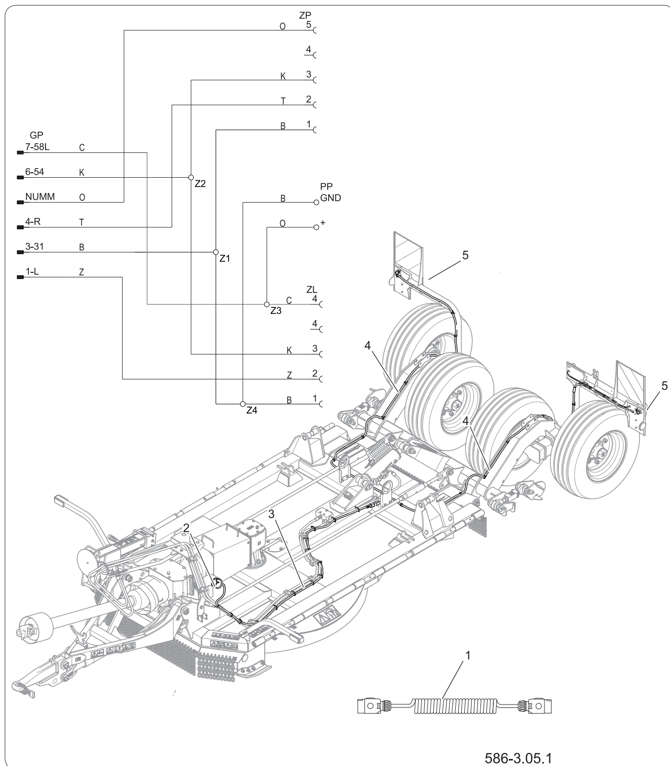
Рисунок 4.3 Конструкция электрической системы косилки KPR500 (1) спиральный кабель, 7-контактная электрическая вилка 12 В, (2) 7-контактная электрическая вилка (3) центральный жгут (4) освещение номерного знака (5) задние фонари
