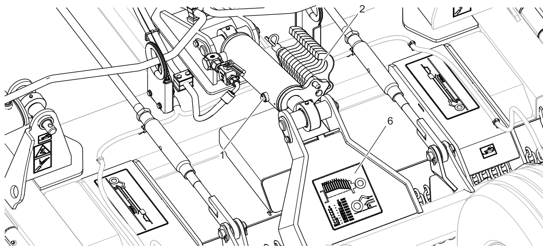
Рисунок 5.6 Транспортная блокировка
