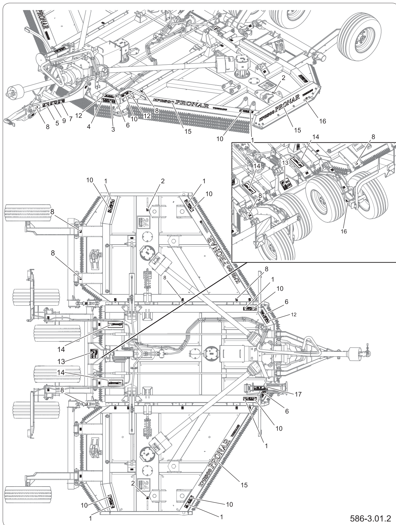
Рисunek 3.1 Расположение информационных и предупреждающих наклеек
