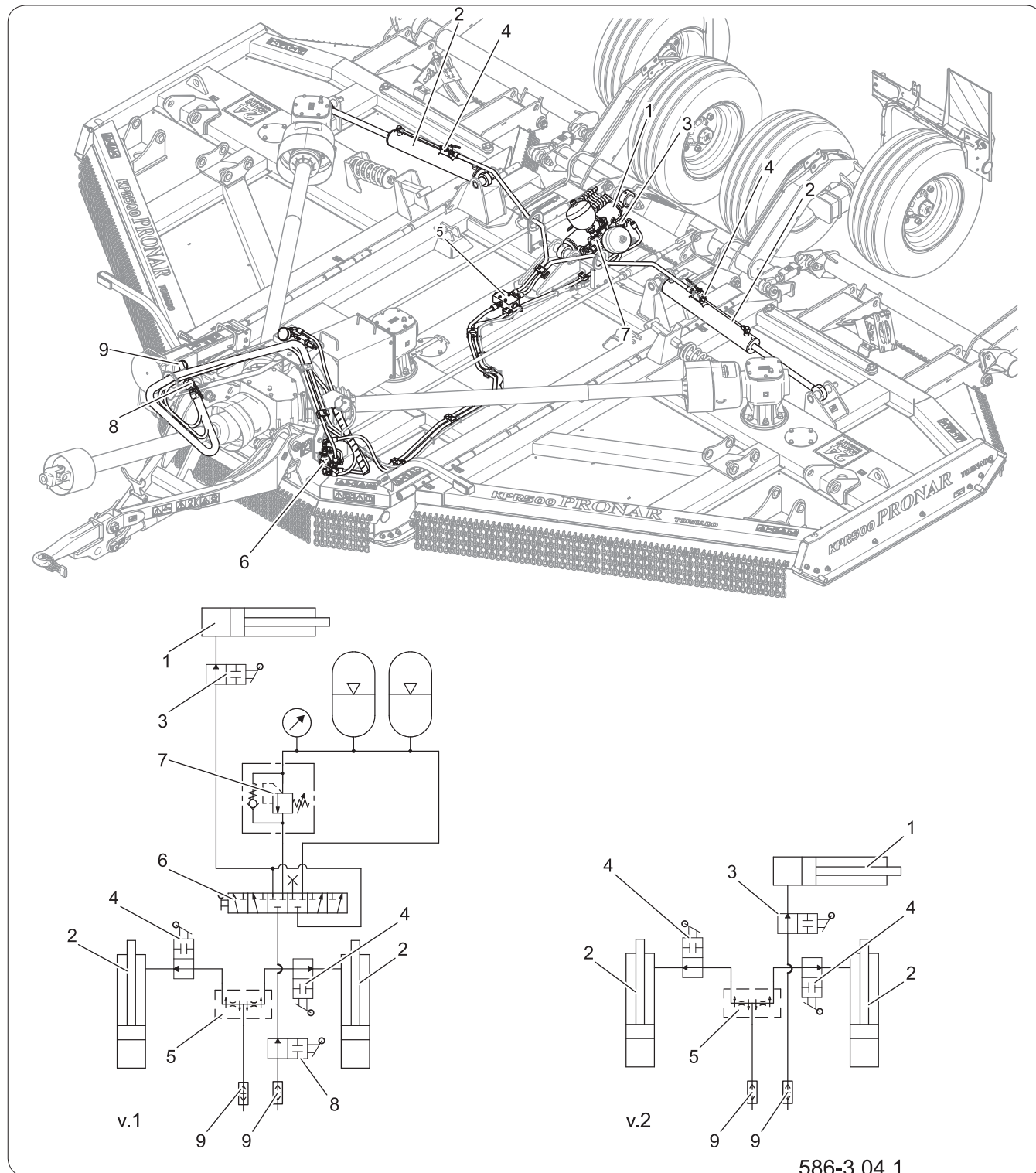
Рисунок 4.2 Устройство гидравлической системы
