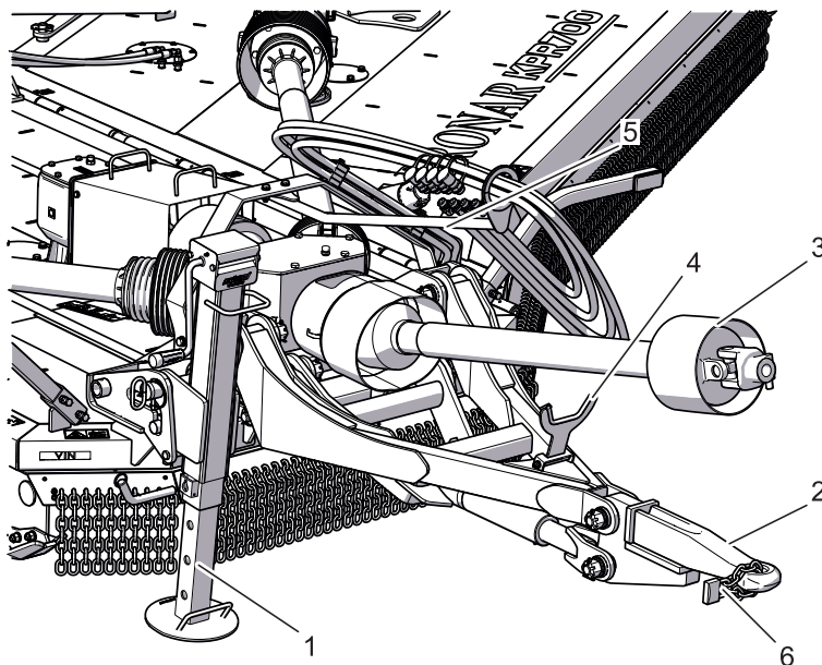
Рисунок 5.5 Подсоединение косилки к носителю
