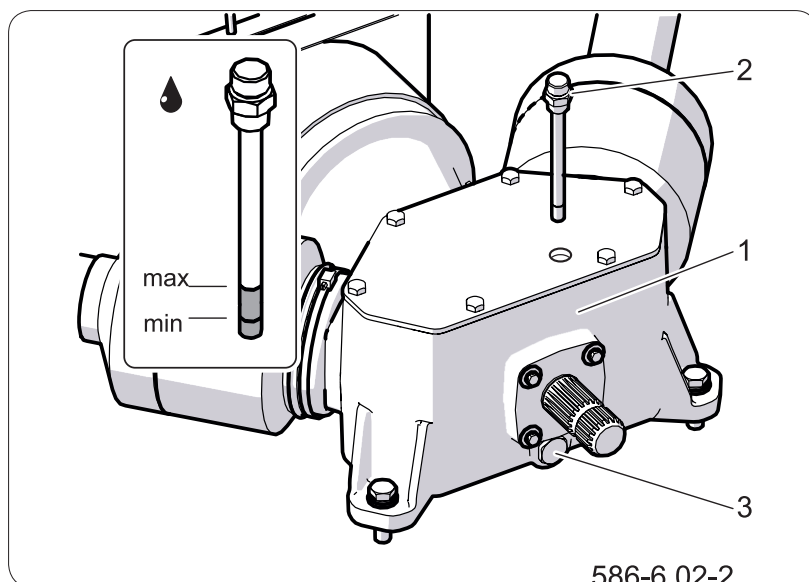
Рисунок 6.9 Проверка и замена масла в коробке передач (1) - корпус коробки (2) - пробка с измерительным щупом (3) - отверстие для слива масла
