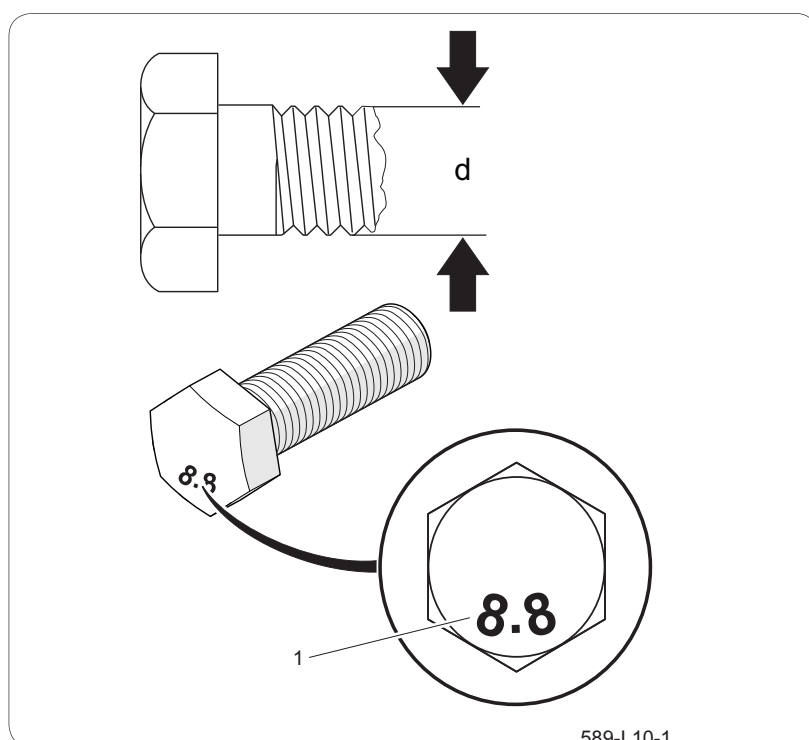
Рисунок 6.3 Винт с метрической резьбой (1) Класс прочности (d) диаметр резьбы
