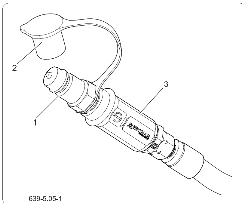
Рисунок 5.9 Подключение к гидравлической системе
