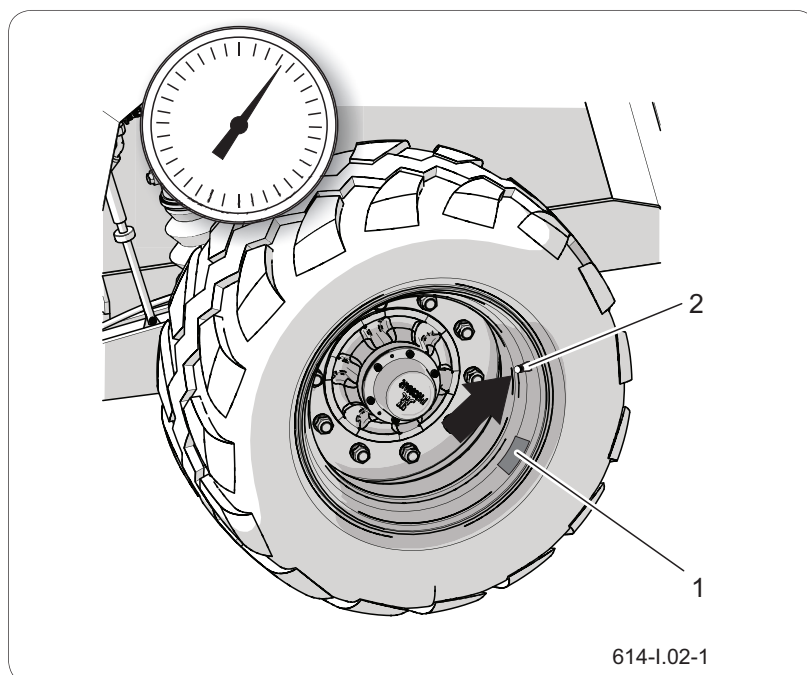
Рисунок 6.2 Колесо машины (1) наклейка (2) клапан
