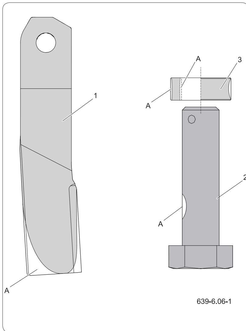
Рисунок 6.12 Возможные места износа элементов головки (1) - нож, (2) - винтовое крепление ножа; (3)- втулка ножа, (A) - места износа, полостей.
