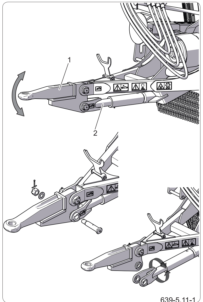
Рисунок 5.2 Настройка наклона дышла (1) тяга дышла (2) винт тяги
