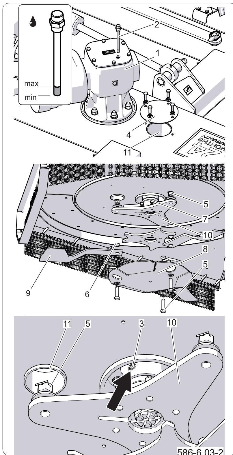
Рисунок 6.10 Проверка и замена масла в угловых передачах
