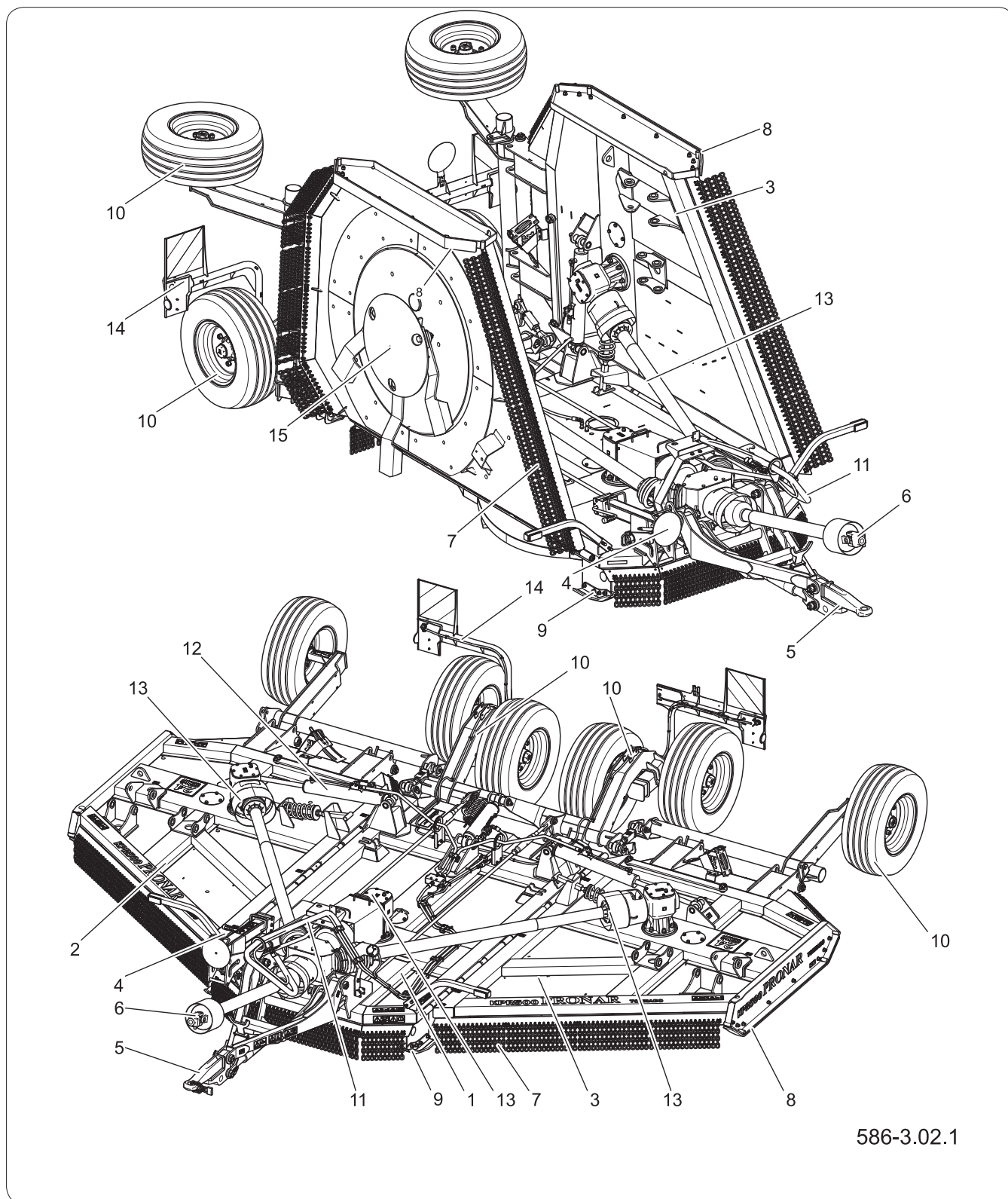
Рисунок 4.1 Устройство косилки-измельчителя KPR500
