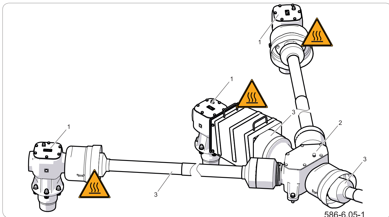
Рисунок 6.8 Проверка и замена масла в системе передачи привода
