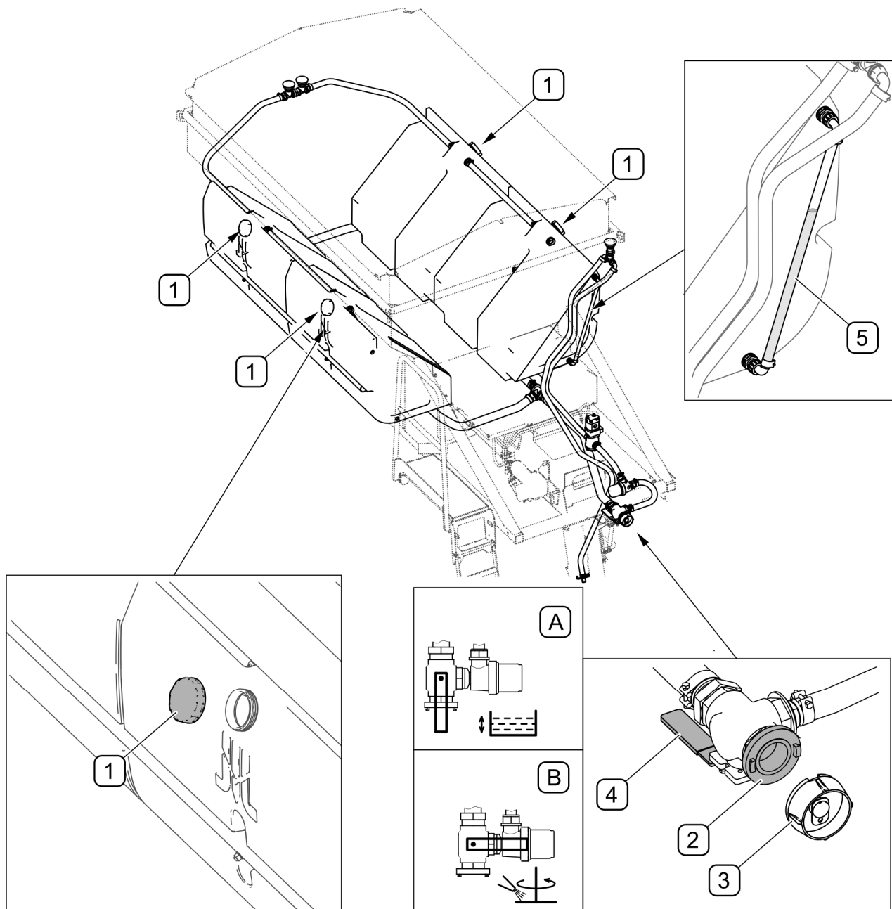
RYSUNEK 4.16 Napełnianie zbiorników solanką
