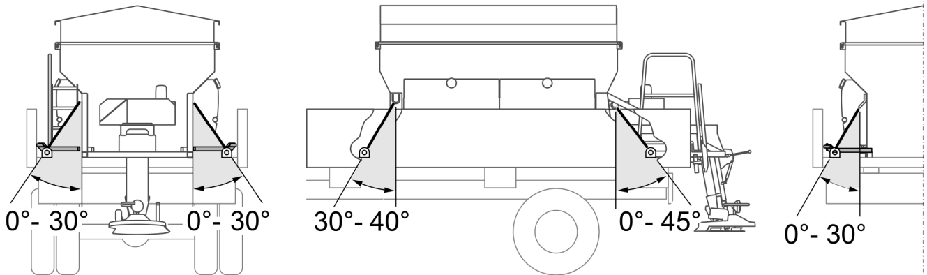
RYSUNEK 4.8 Mocowanie 4
