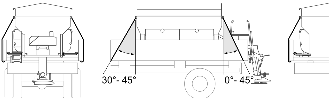
RYSUNEK 4.7 Mocowanie 3
