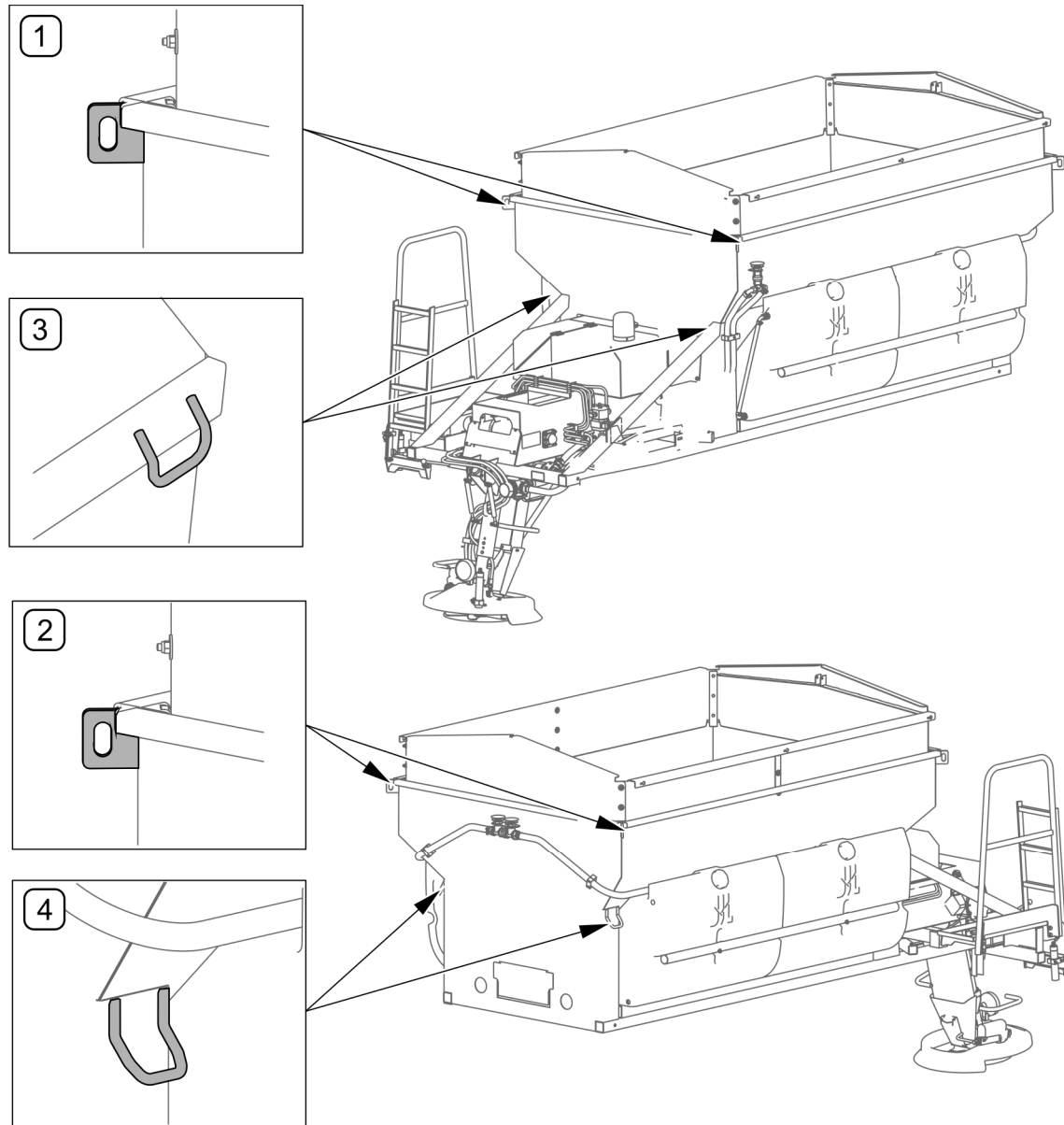
RYSUNEK 4.4 Punkty mocowania pasów
