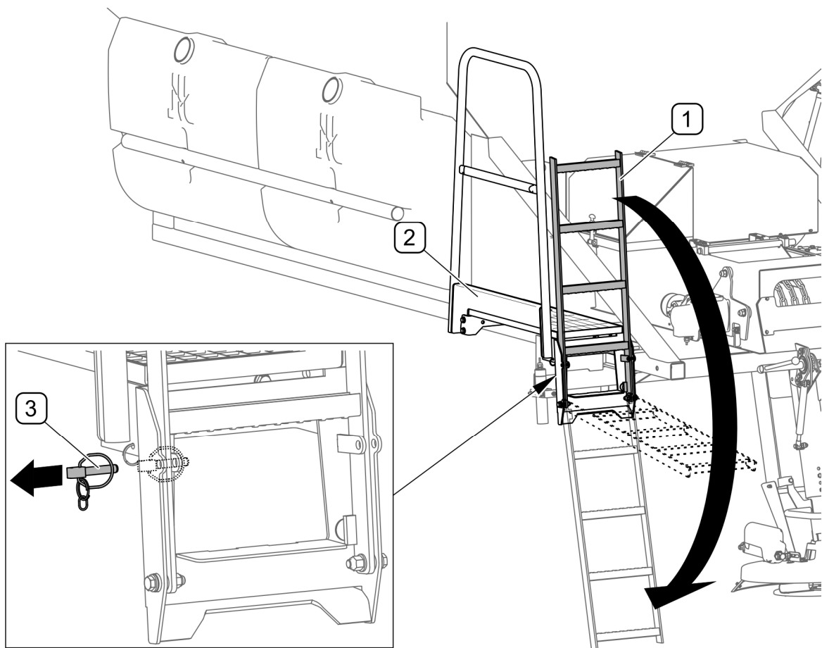
RYСУNEK 4.14 Drabinka i podest
