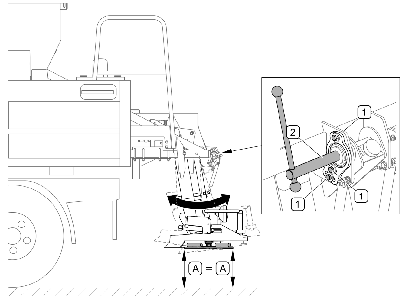
RYSUNEK 4.12 Poziomowanie tarczy rozsiewającej
