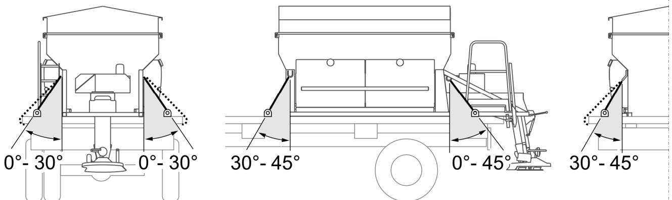
RYSUNEK 4.9 Mocowanie 5
