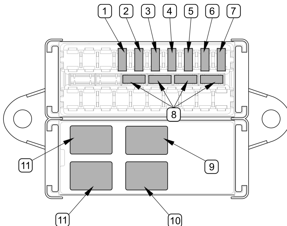
RYSUNEK 5.3 Bezpieczniki i przekaźniki
