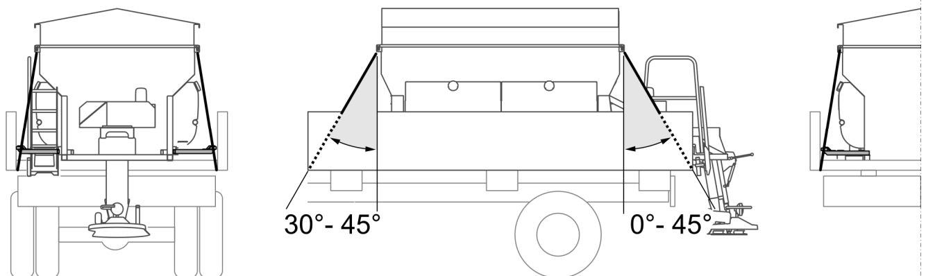
RYSUNEK 4.6 Mocowanie 2
