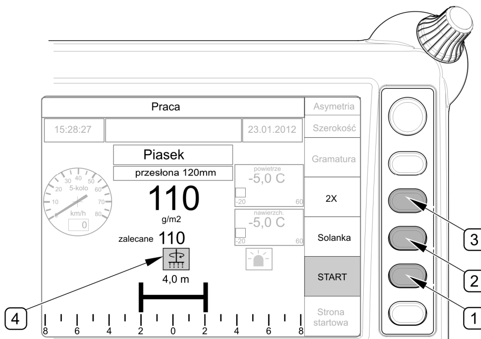
RYСУNEK 4.28 Uruchomienie posypywania
