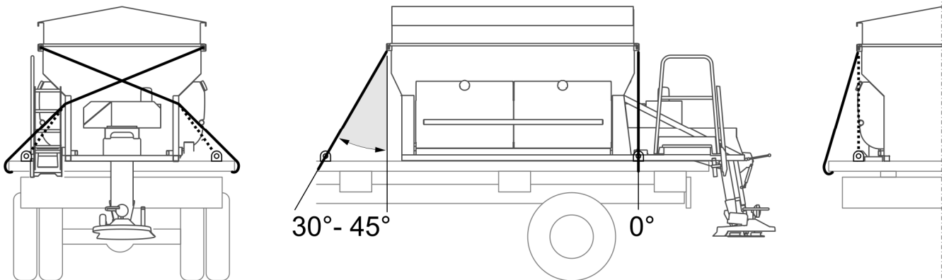
RYSUNEK 4.5 Mocowanie 1
