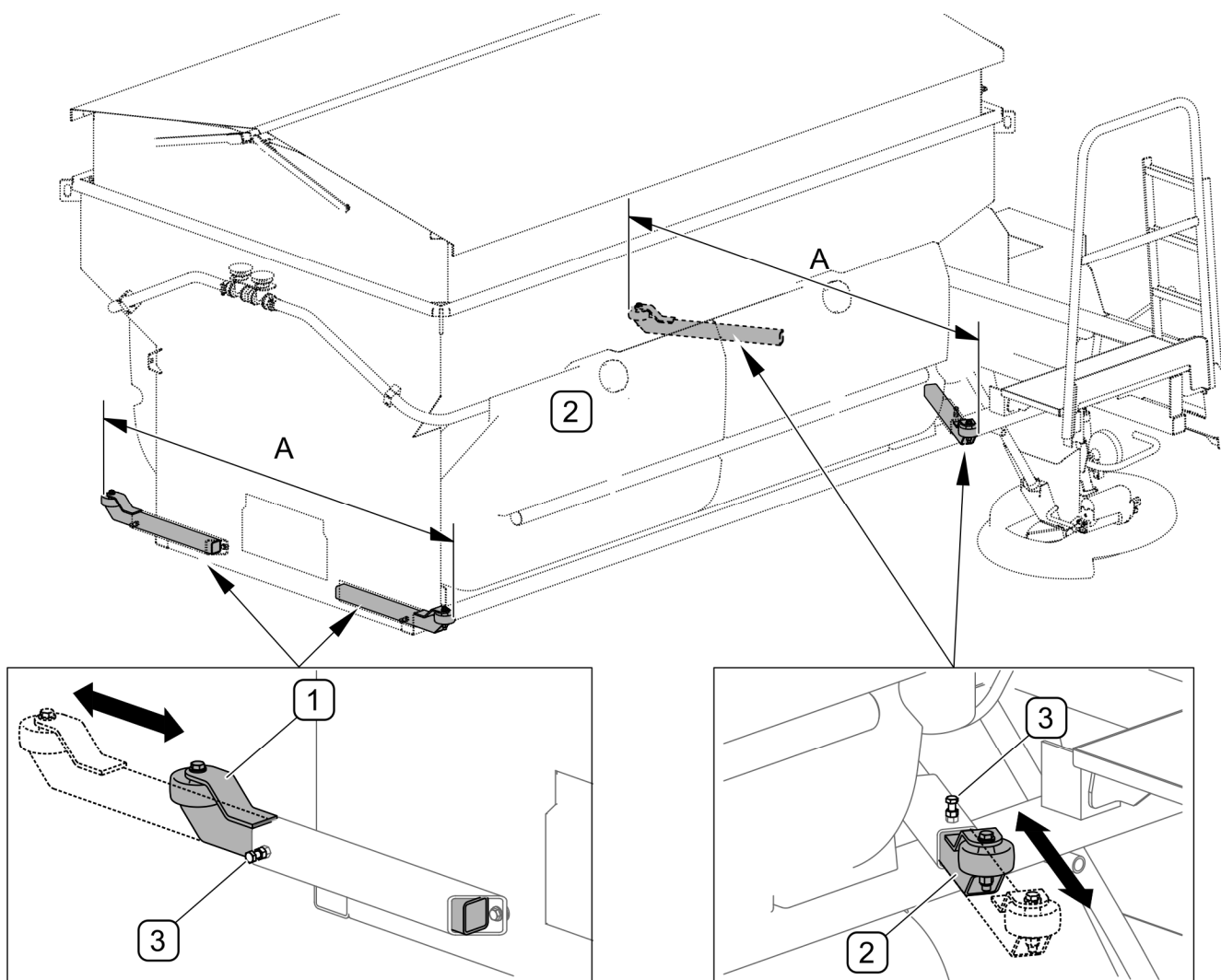
RYSUNEK 4.2 Prowadnice
