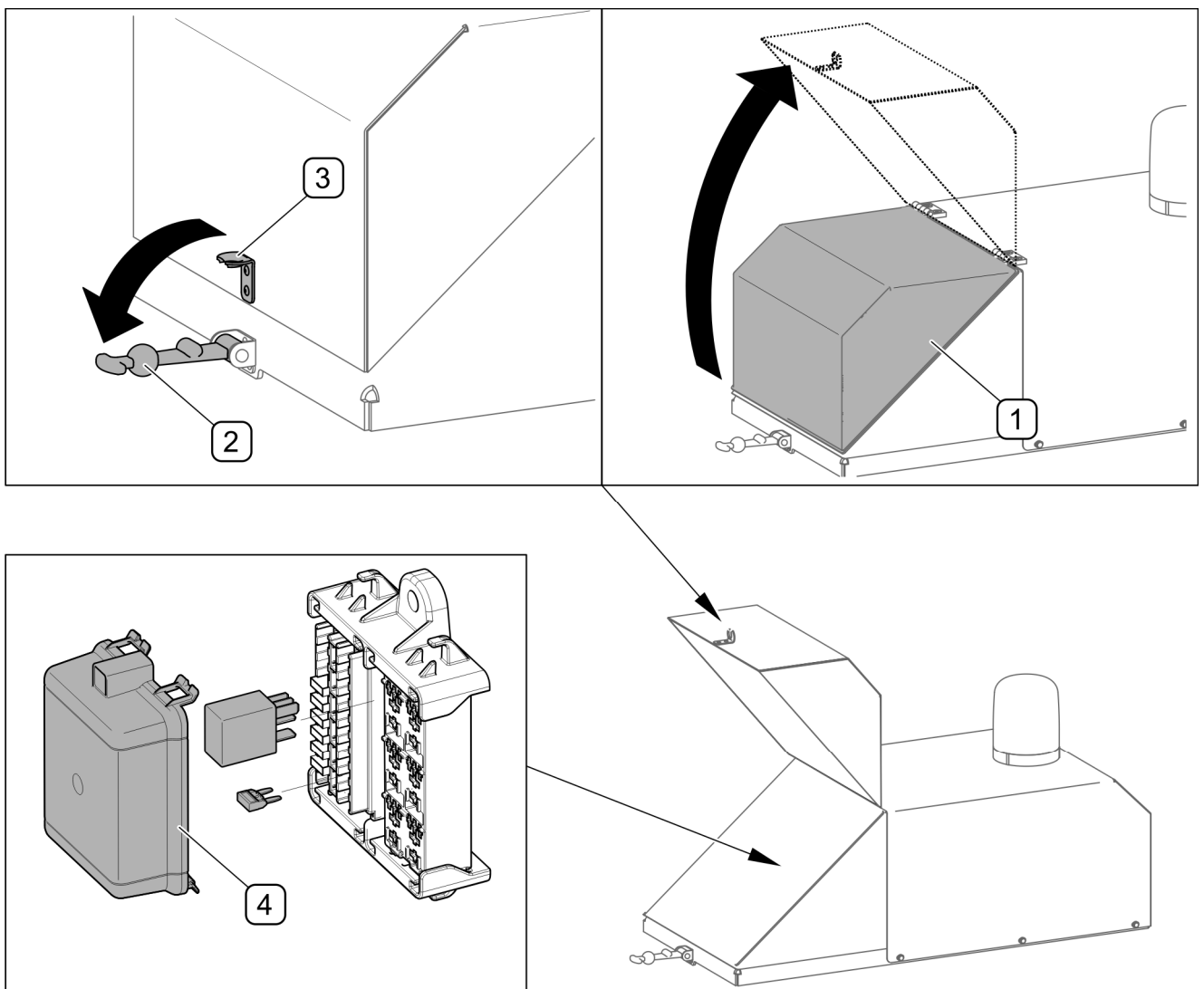
RYSUNEK 5.2 Umieszczenie skrzynki bezpiecznikowej
