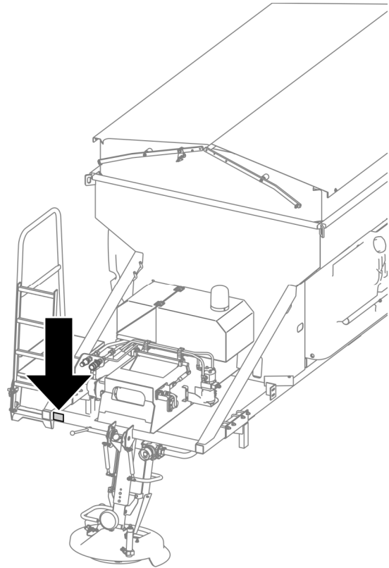
RYSUNEK 1.1 Miejsce umieszczenia tabliczki znamionowej
