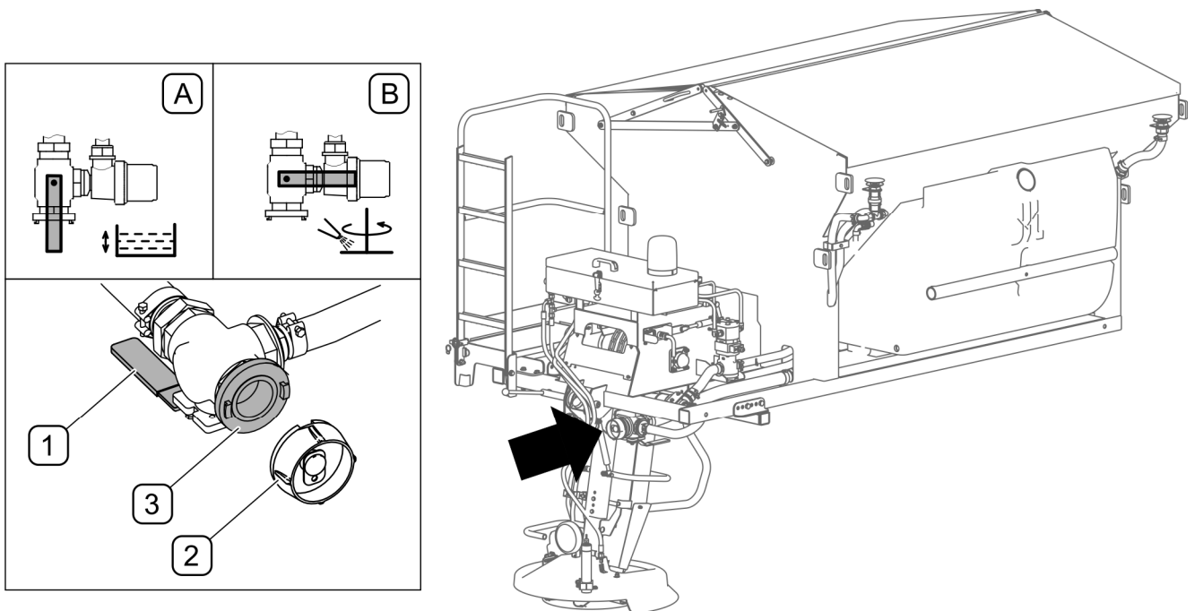
RYSUNEK 4.34 Opróżnianie zbiorników solanki
