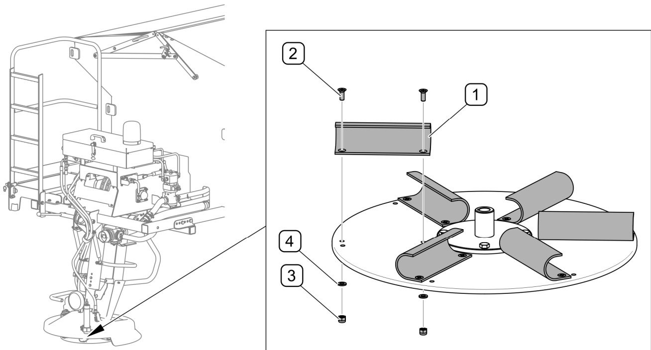
RYСУNEK 5.9 Wymiana łopatek tarczy mechanizmu wysiewającego
