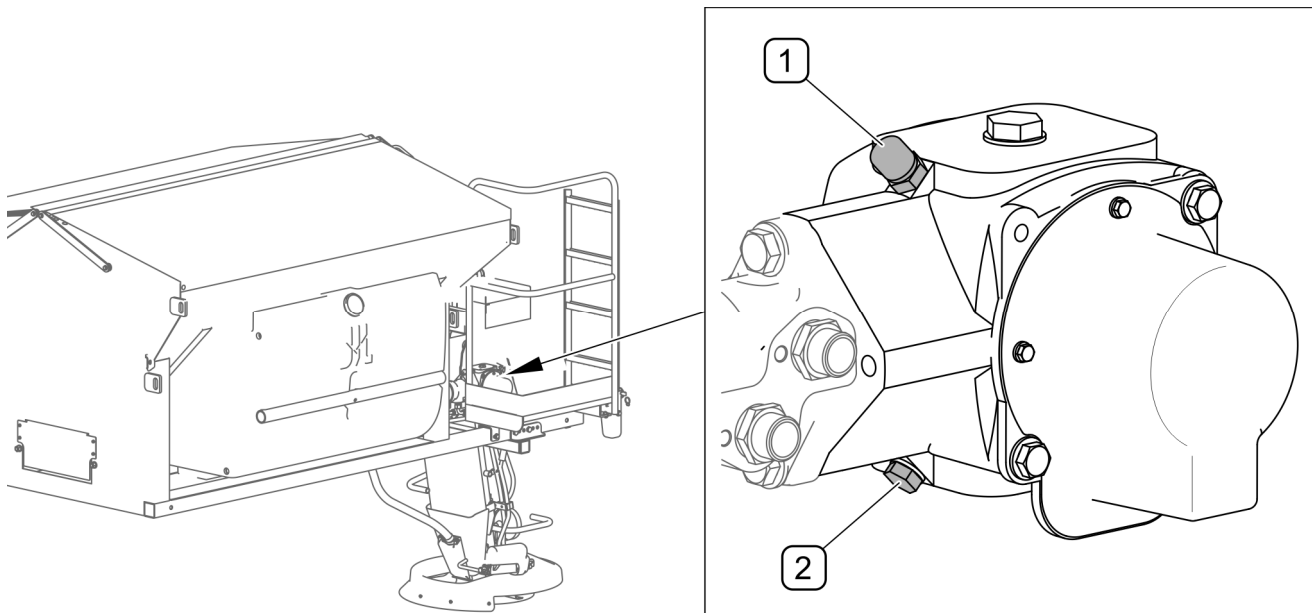
RYSUNEK 5.3 Wymiana oleju w przekładni napędu przenośnika taśmowego
