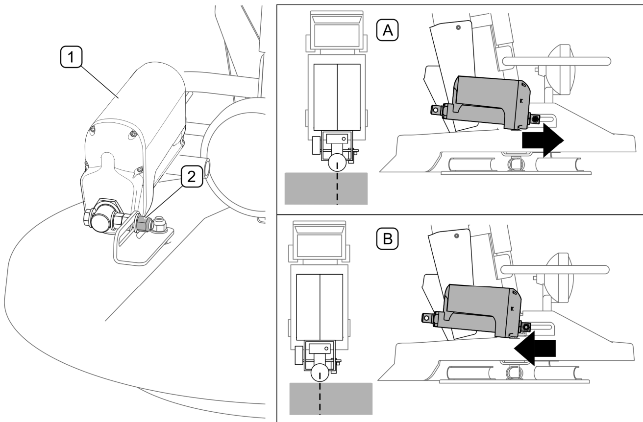
RYСУNEK 5.8 Regulacja mechanizmu wysiewającego
