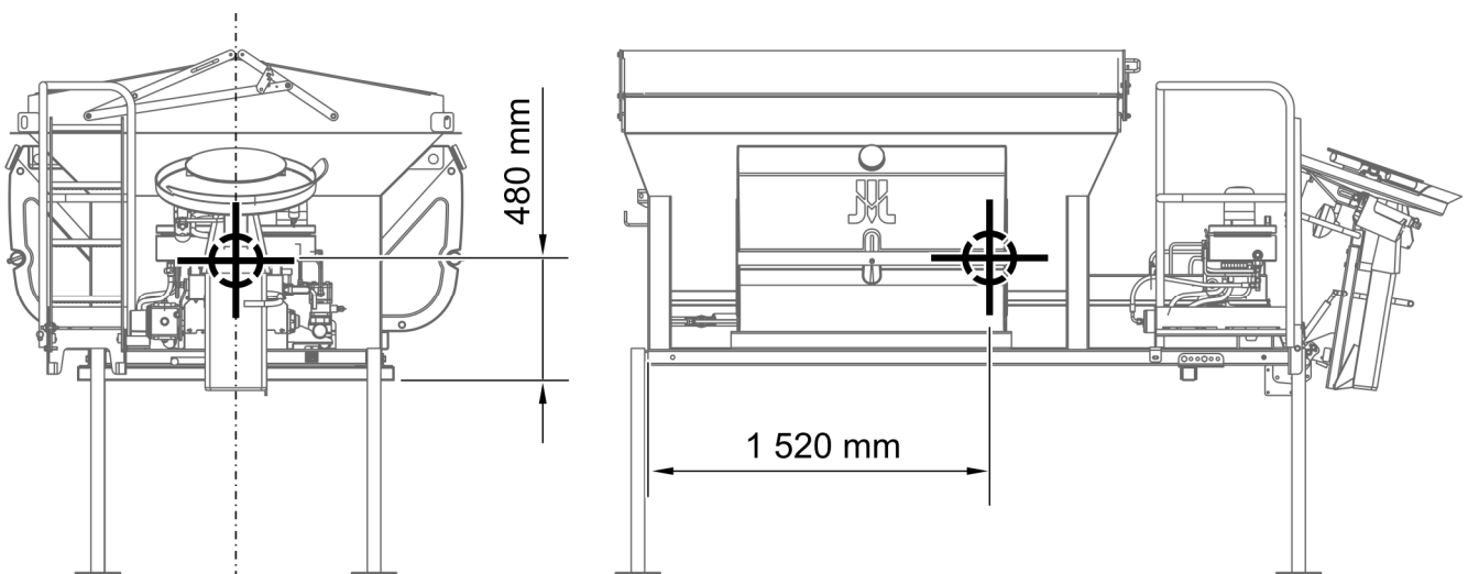
RYSUNEK 1.3 Położenie środka ciężkości (puste zbiorniki)
