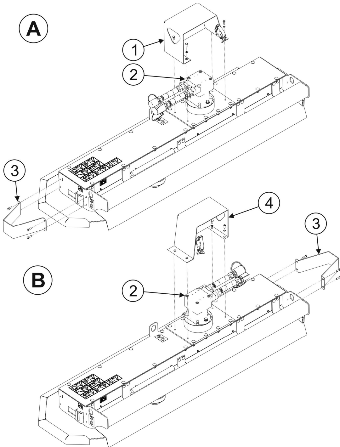
RYSUNEK 4.2 Dostosowanie budowy piły do pracy z lewej strony wyciągnika wielofunkcyjnego.
