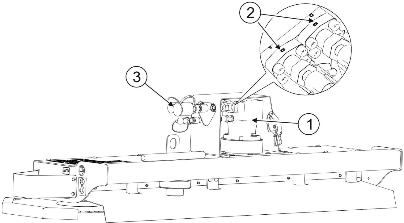
RYSUNEK 5.6 Kontrola połączeń szybkozłączy przewodów hydraulicznych silnika hydraulicznego.
