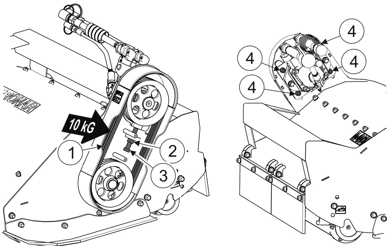
RYSUNEK 5.4 Kontrola i regulacja napięcia pasów klinowych
