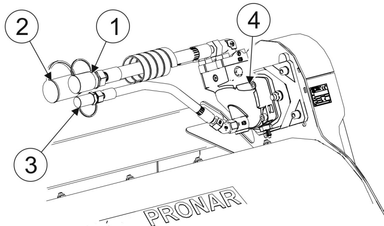
RYSUNEK 5.5 Kontrola połączeń szybkozłączy przewodów hydraulicznych silnika hydraulicznego.
