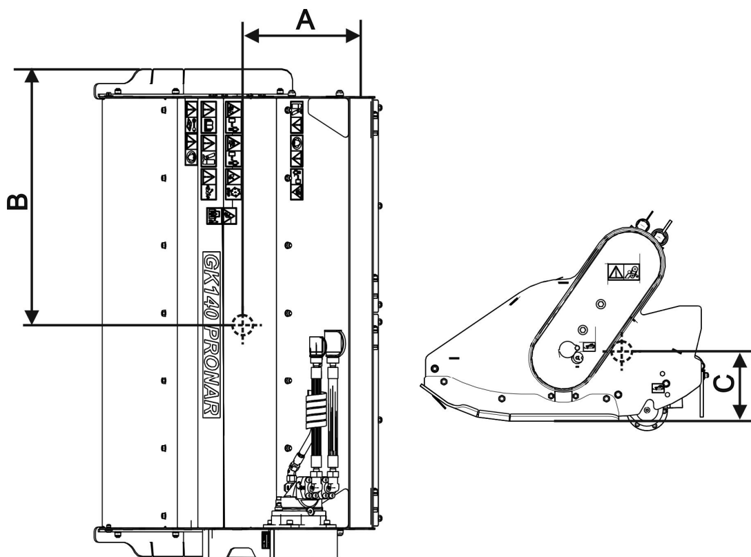
RYСУNEK 1.2 Położenie środka ciężkości głowicy koszącej.
