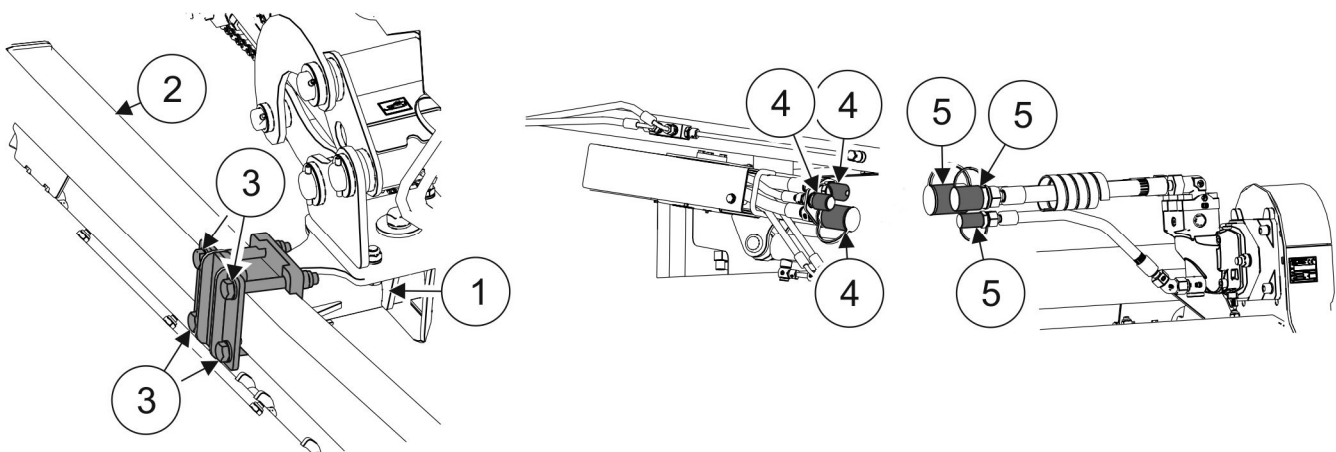
RYСУNEK 4.2 Łączenie z wysięgnikiem wielofunkcyjnym
