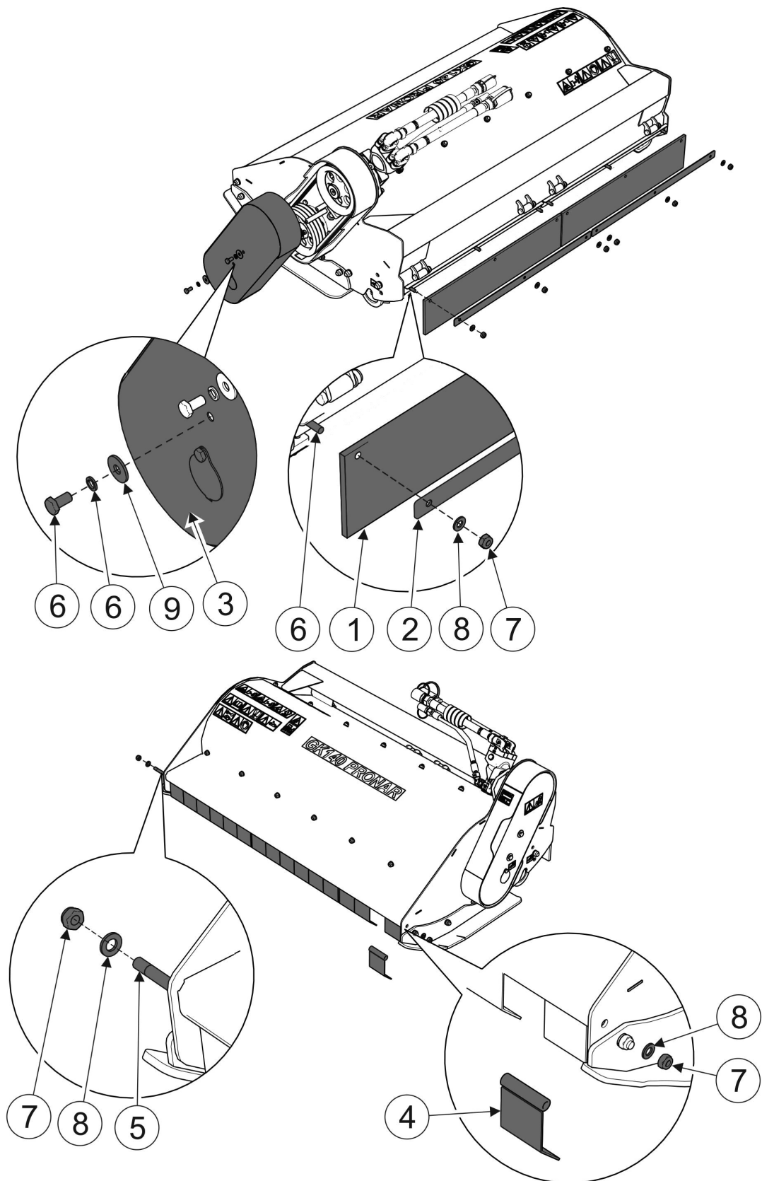
RYSUNEK 5.1 Demontaż osłon
