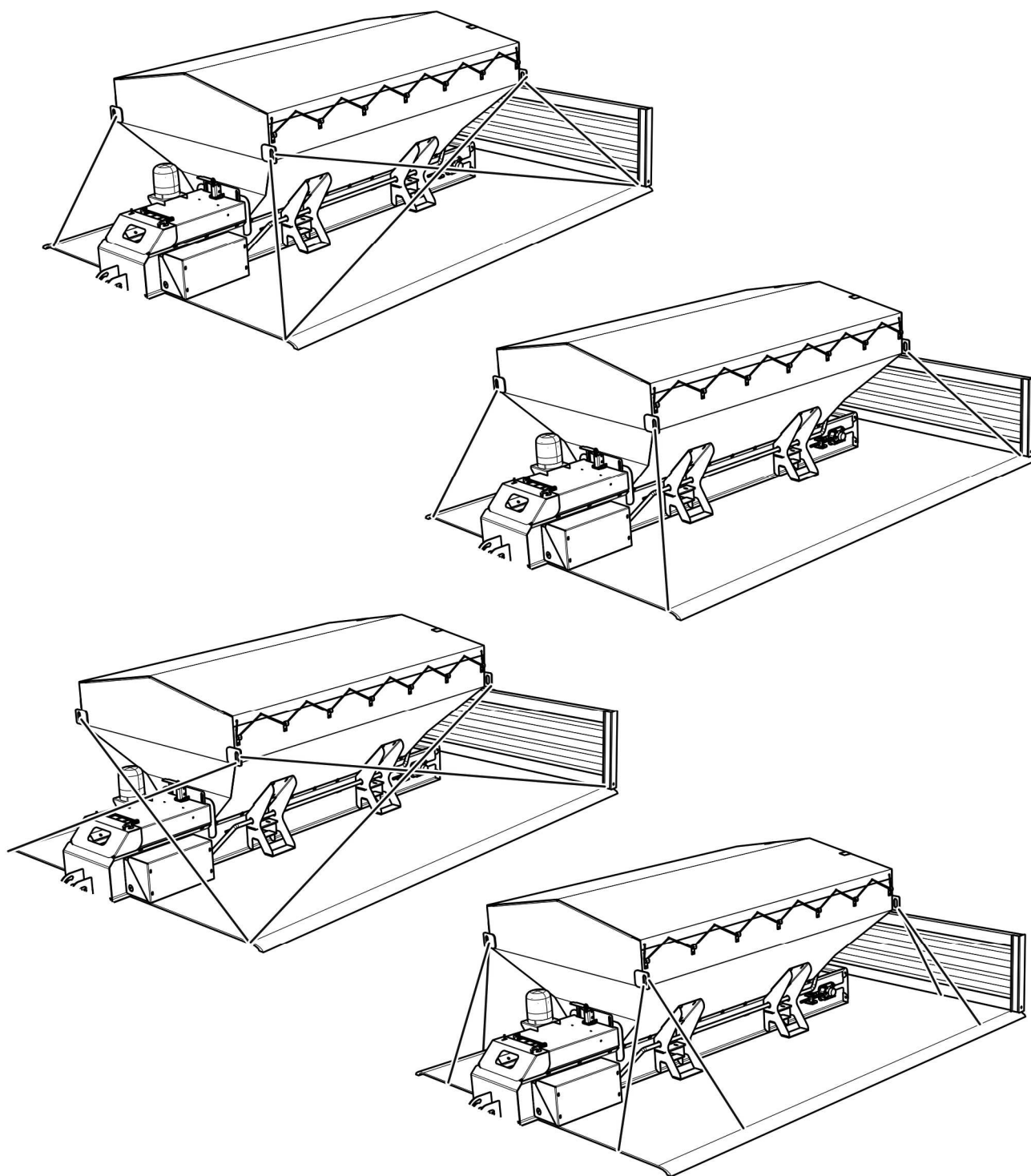
RYSUNEK 4.3 Warianty mocowania posypywarki
