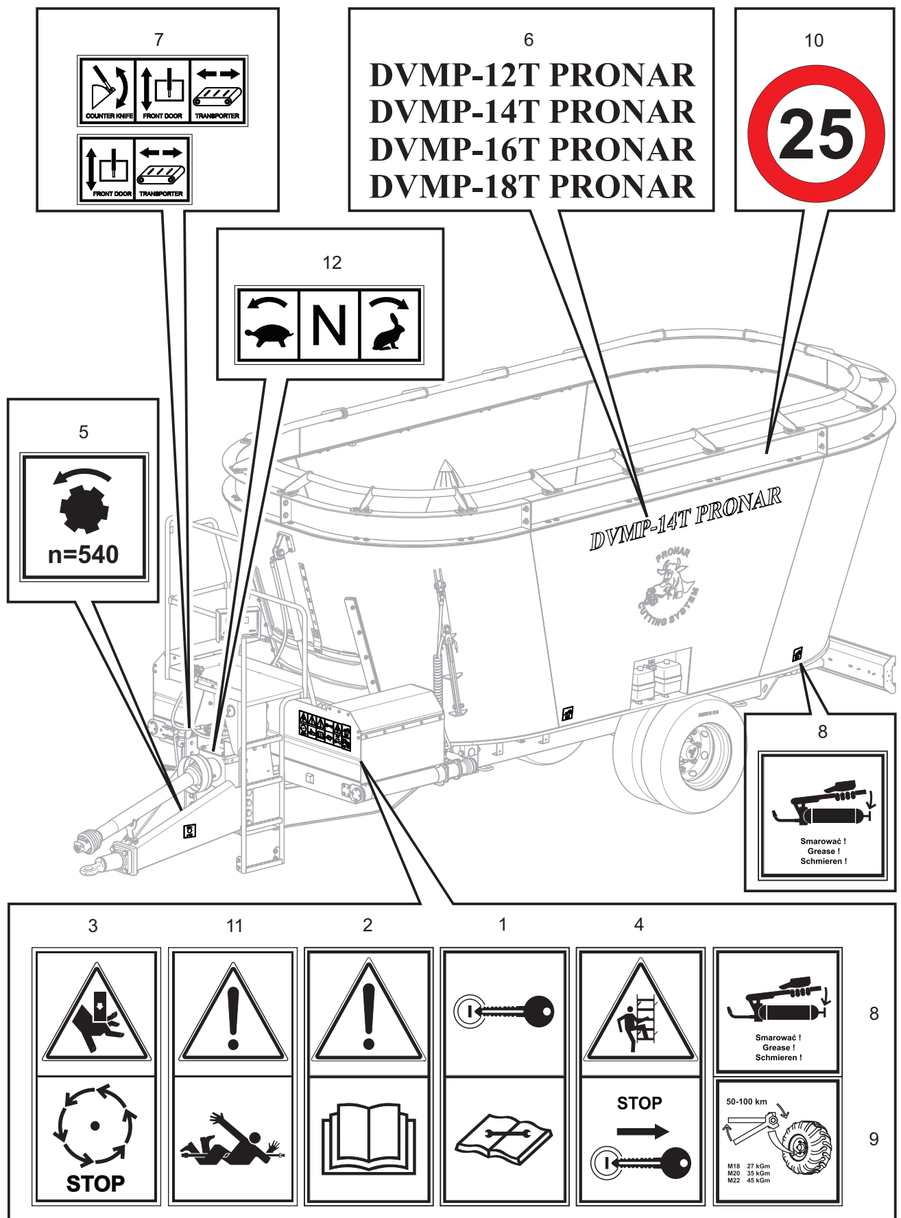
Rysunek 2.2 Rozmieszczenie naklejek informacyjnych i ostrzegawczych.
