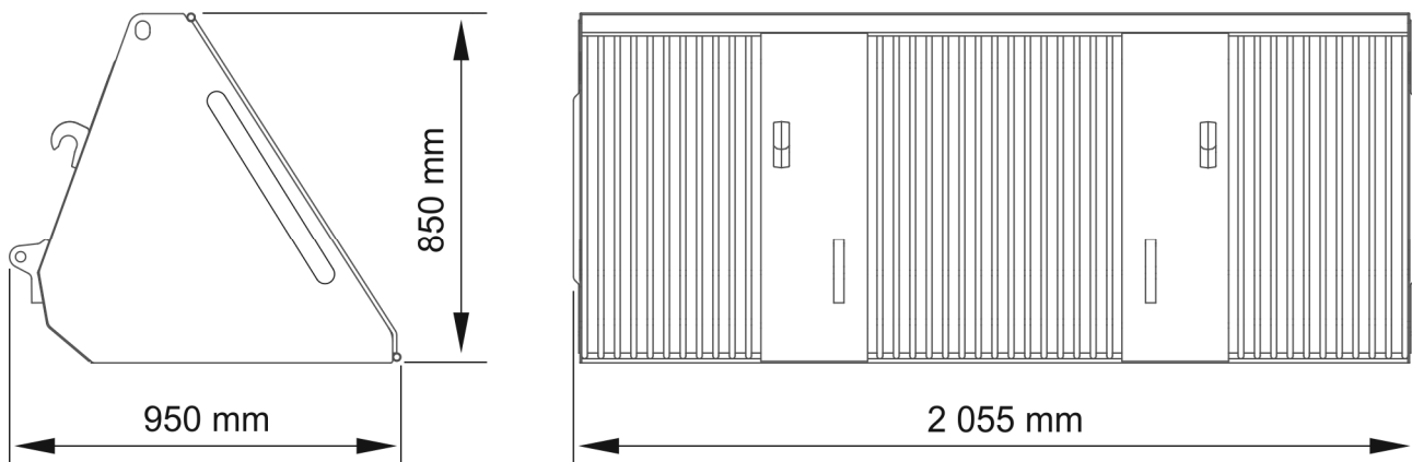
RYSUNEK 3.1 Wymiary zewnętrzne
