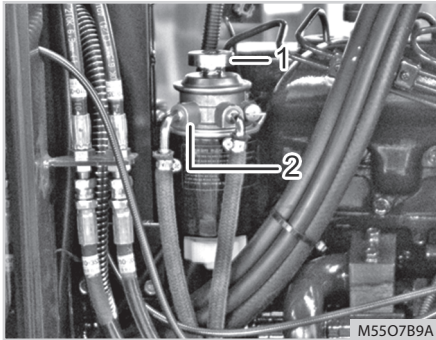
(1) Pompka odpowietrzająca (2) Korek odpowietrzający
