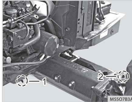
(1) Wspornika osi przedniej (tylny) (2) Podpora obudowy osi przedniej (prawa)
