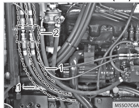
(1) Przewód płynu do wspomagania kierownicy (2) Połączyć
