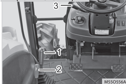
(1) Główna dźwignia zmiany biegów (2) Dźwignia przełączania inwersora (3) Dźwignia zmiany zakresu przełożeń przekładni
