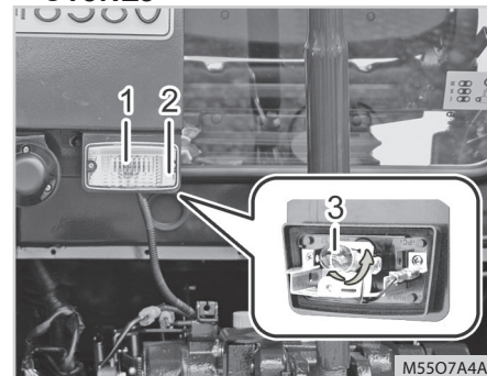
(1) Lampka tablicy rejestracyjnej (2) Śruba mocująca (3) Żarówka lampki tablicy rejestracyjnej
