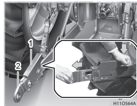
(1) Zatrzask (2) Końcówka cięgła dolnego
