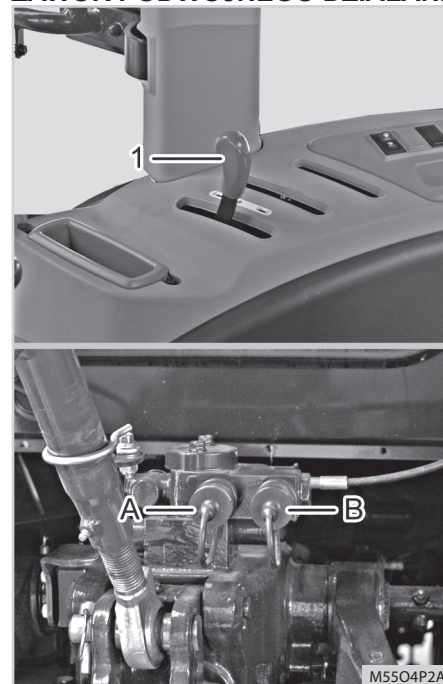
(1) Zawór podwójnego działania Dźwignia 1 (A) Przyłącze A (B) Przyłącze B
