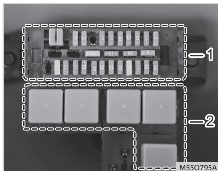
(1) Skrzynka bezpiecznikowa (2) Skrzynka przełącznikowa
