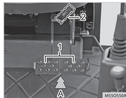
(1) pedał hamulca (lewy / prawy) (2) Zapadka do zblokowania pedałów
