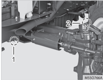
(1) Wspornika osi przedniej (przedni) (2) Podpora obudowy osi przedniej (lewa)
