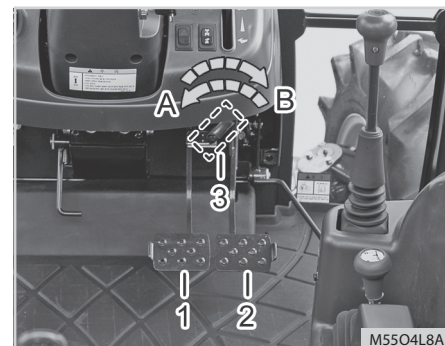
(1) Pedal hamulca (lewy) (2) Pedal hamulca (prawy) (3) Zapadka służąca do zblokowania pedałów hamulca
