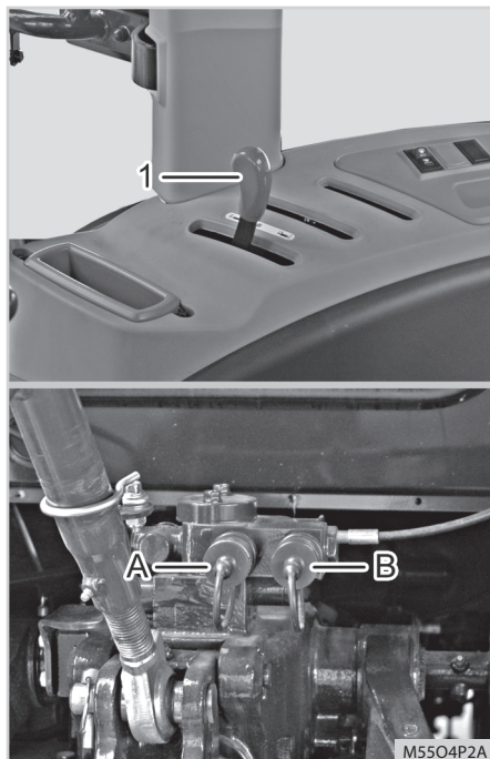
(1) Zawór podwójnego działania 1 i dźwignia 1 (A) Przyłącze A (B) Przyłącze B
