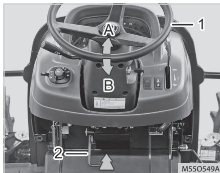
(1) Kierownica (2) Pedał przechylenia kierownicy
