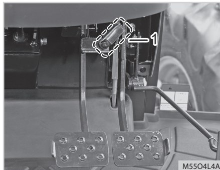
(1) Zapadka sprzęgająca pedały hamulca (hamowanie obustronne)
