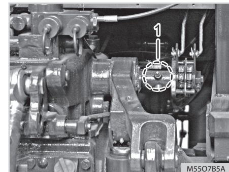
(1) Wspornik ramienia przekładni kierowniczej
