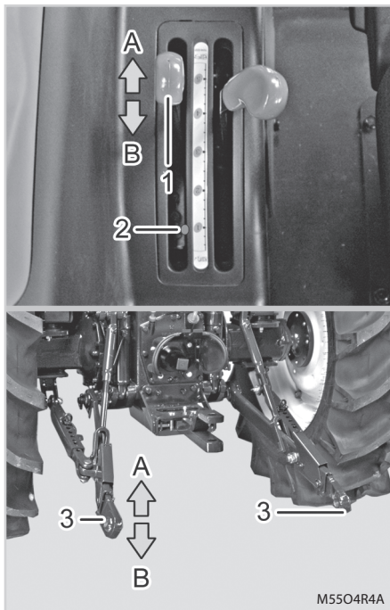
(1) Dźwignia regulacji pozycyjnej (2) Sworzni blokujący (3) Dolne cięgło (A) Podnoszenie (B) Opuszczanie
