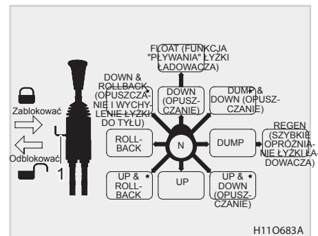
(1) Dźwignia blokowania joysticka
