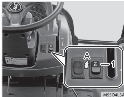
(1) Przełącznik wyboru trybu jazdy (A) Napęd na cztery koła (4WD)
