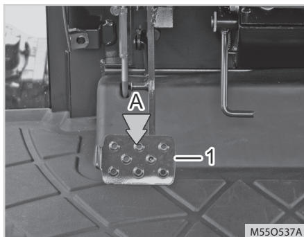
(1) Pedał sprzęgła (A) Wcisnąć
