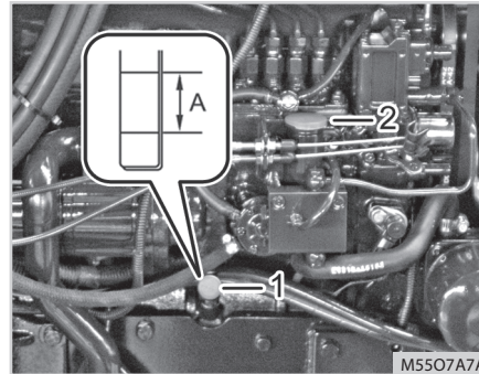
(1) Wskaźnik prętowy poziomu oleju (2) Wlew oleju silnikowego
