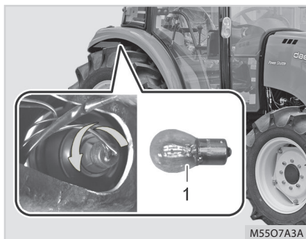
(1) Żarówka lampy kierunkowskazu (tylnej)
