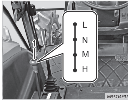
(1) Dźwignia zmiany zakresu przełożeń przekładni
