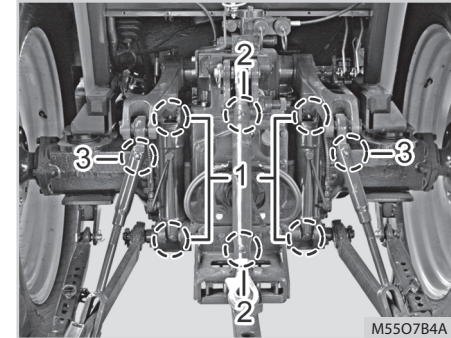
(1) Siłownik hydrauliczny (górny/dolny) (2) Ciężko górne (górne/dolne) (3) Ciężko podnoszące (lewe/prawe)
