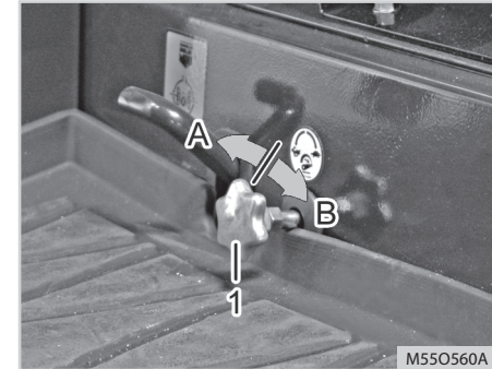
(1) Pokrętło regulacji prędkości opuszczania TUZ
