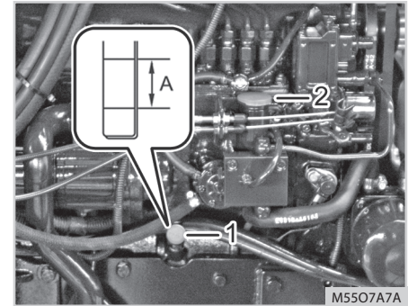
(1) Wskaźnik prętowy poziomu oleju (2) Korek wlewowy oleju silnikowego (A) Poziom oleju powinien mieścić się w tym zakresie
