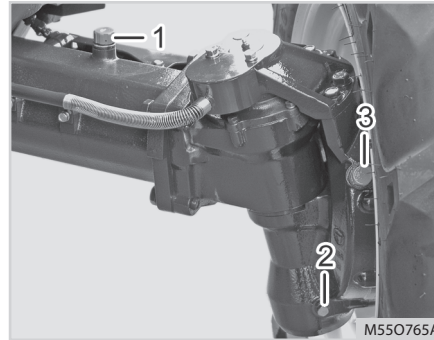
(1) Korek wlewowy oleju (2) Korek spustowy (3) Korek odpowietrzający
