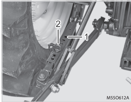
(1) Ciężko kontrolne (2) Sworzeń
