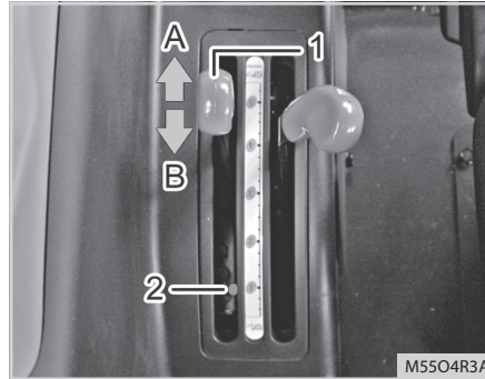
(1) Dźwignia regulacji pozycyjnej (2) Śruba (A) Podnoszenie (B) Opuszczanie
