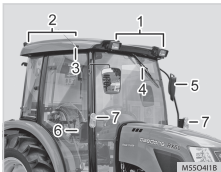
(1) Światło robocze (przednie) (2) Światło robocze (tylne) (3) Antena (4) Wycieraczka (5) Zewnętrzne lustro wsteczne (6) Klamka
