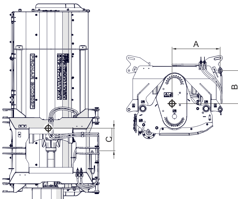
Rysunek 1.3 Położenie środka ciężkości
