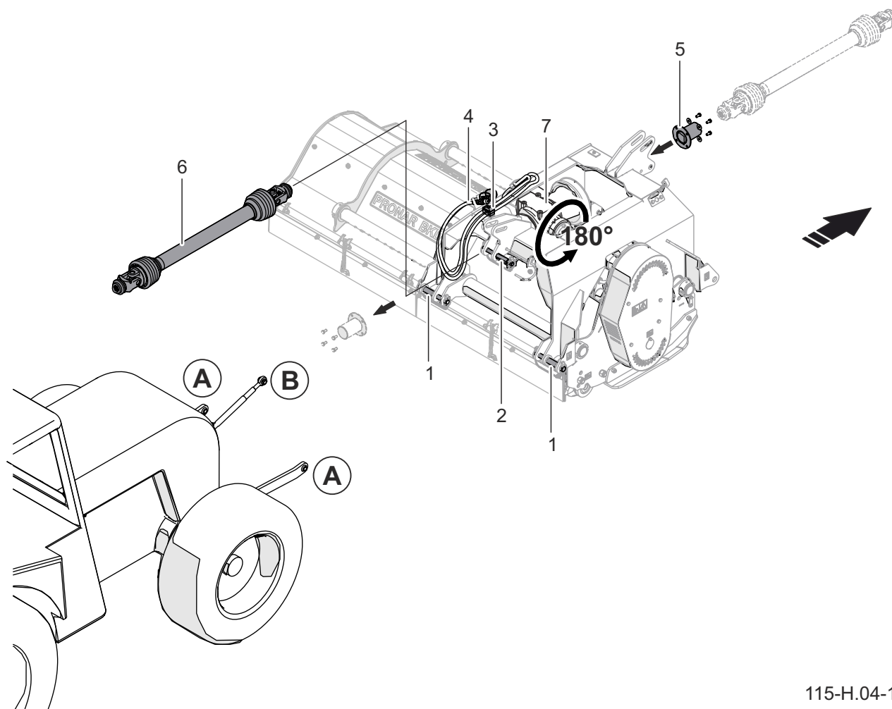
Rysunek 4.5 Łączenie z przednim TUZ nośnika
