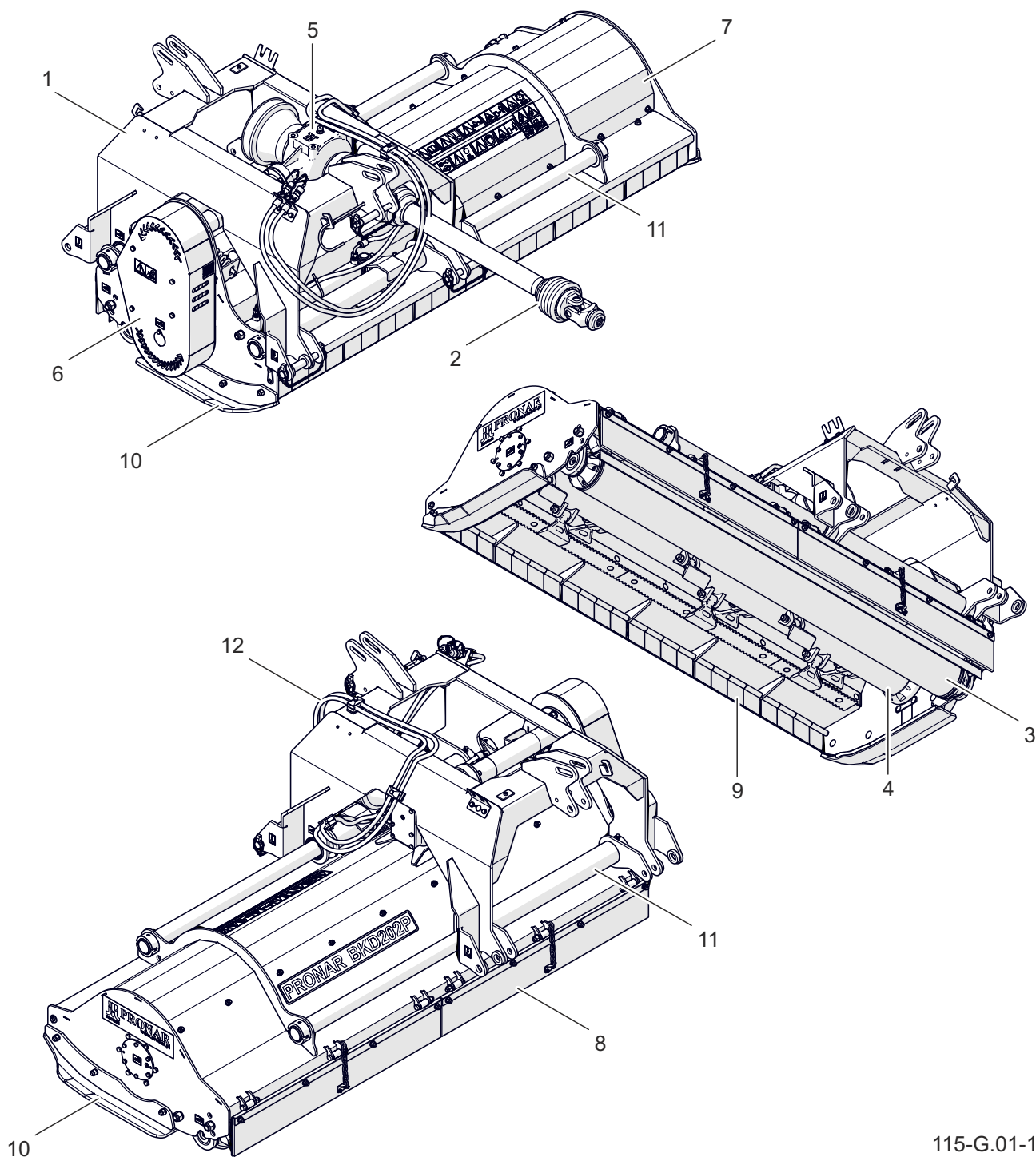
Rysunek 3.1 Budowa ogólna
