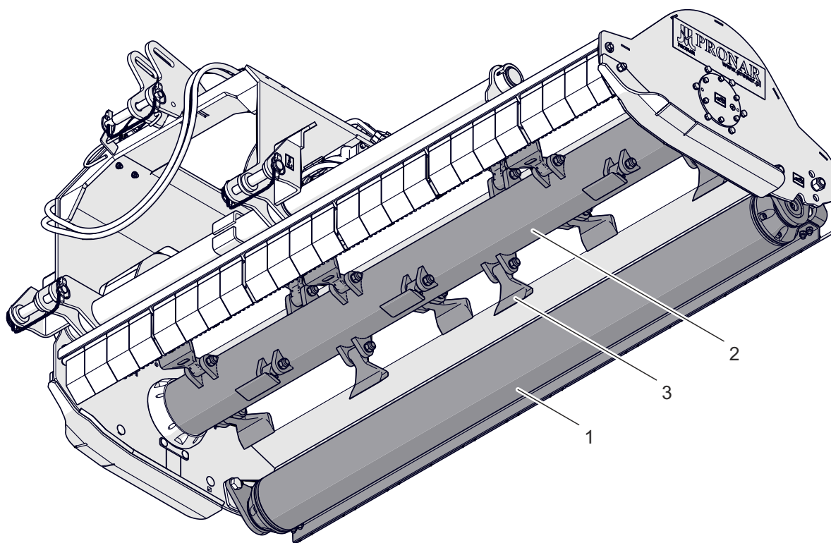
Rysunek 3.5 Zespół tnący
