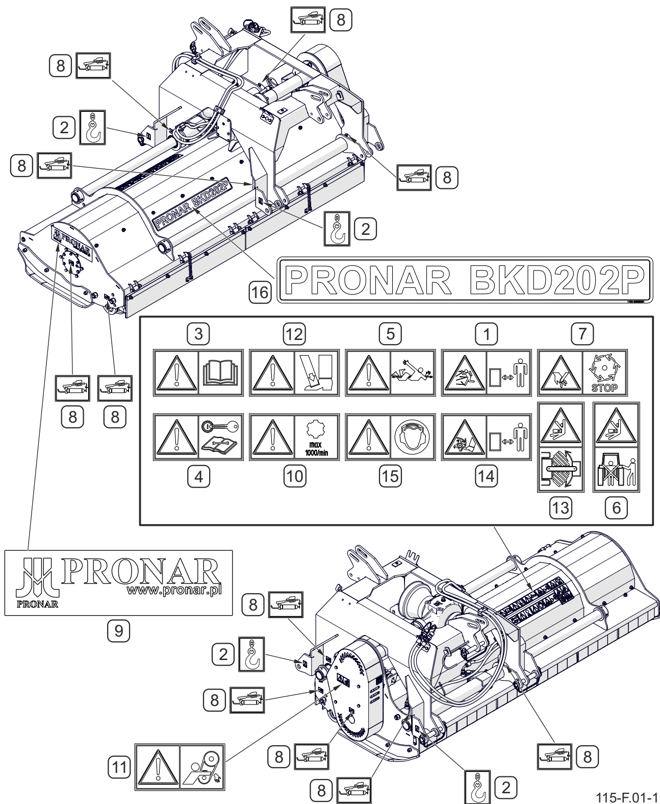
Rysunek 2.1 Rozmieszczenie naklejek informacyjnych i ostrzegawczych. Opis znaczenia symboli (TABELA 2.1)
