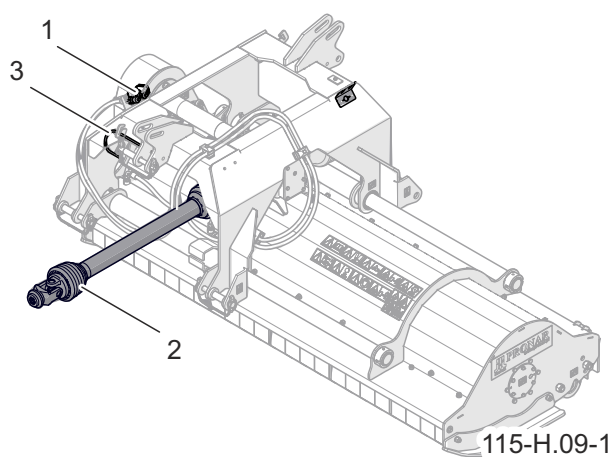
Rysunek 4.10 Odłączanie kosiarki od nośnika (1) wtyki przewodów hydraulicznych (2) wał przegubowo-teleskopowy (3) wieszak
