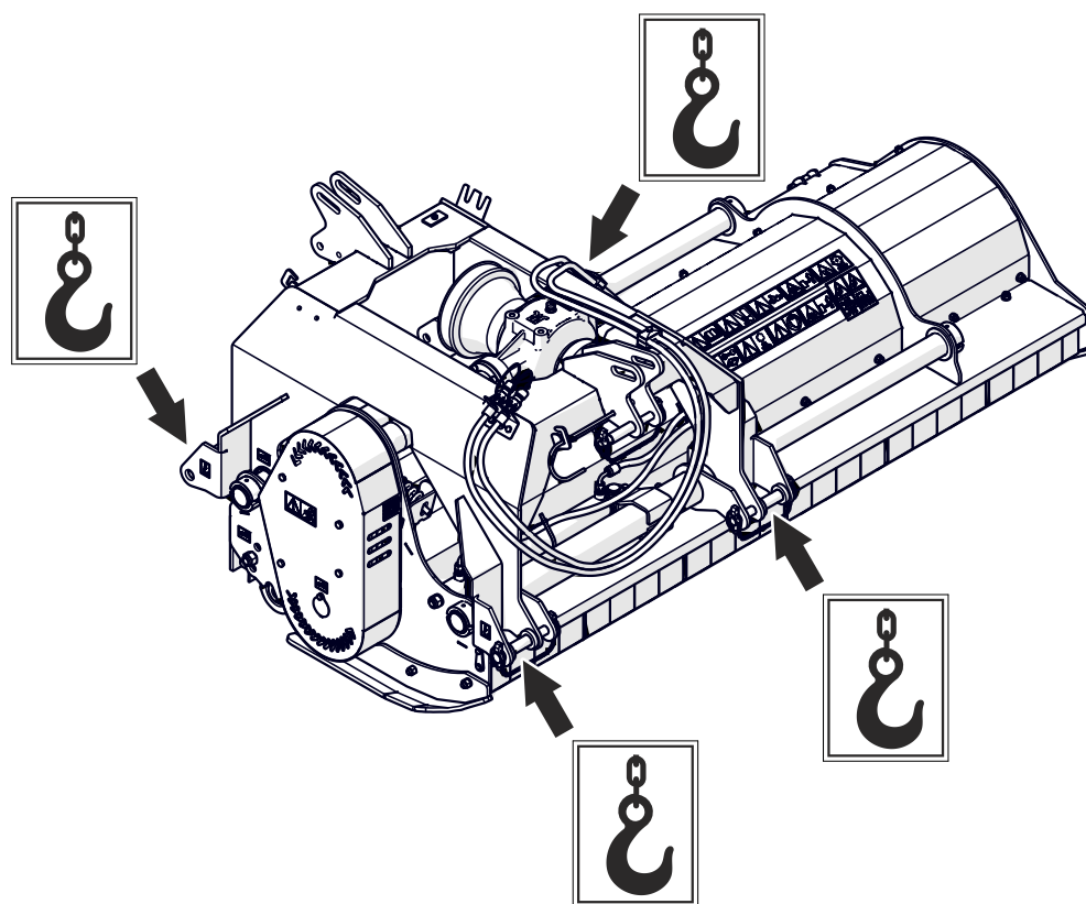
Rysunek 1.2 Uchwyty transportowe
