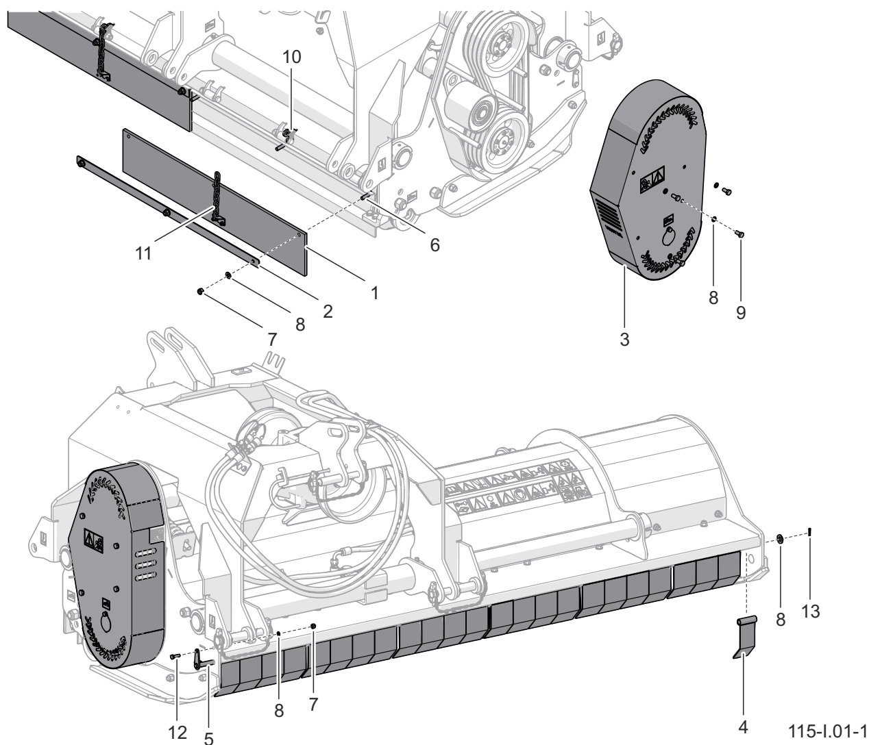
Rysunek 5.1 Demontaż osłon
