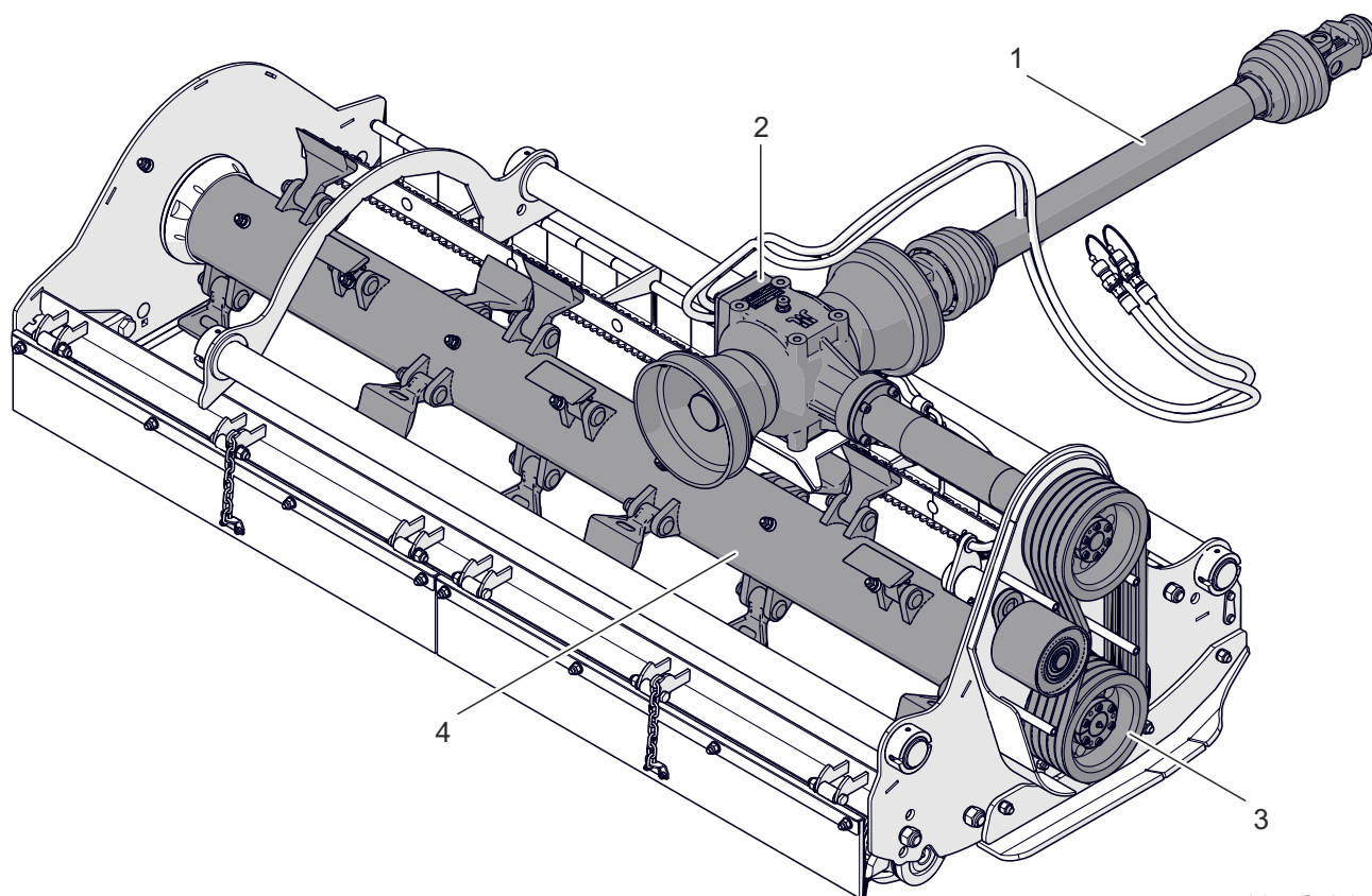
Rysunek 3.4 Układ przeniesienia napędu
