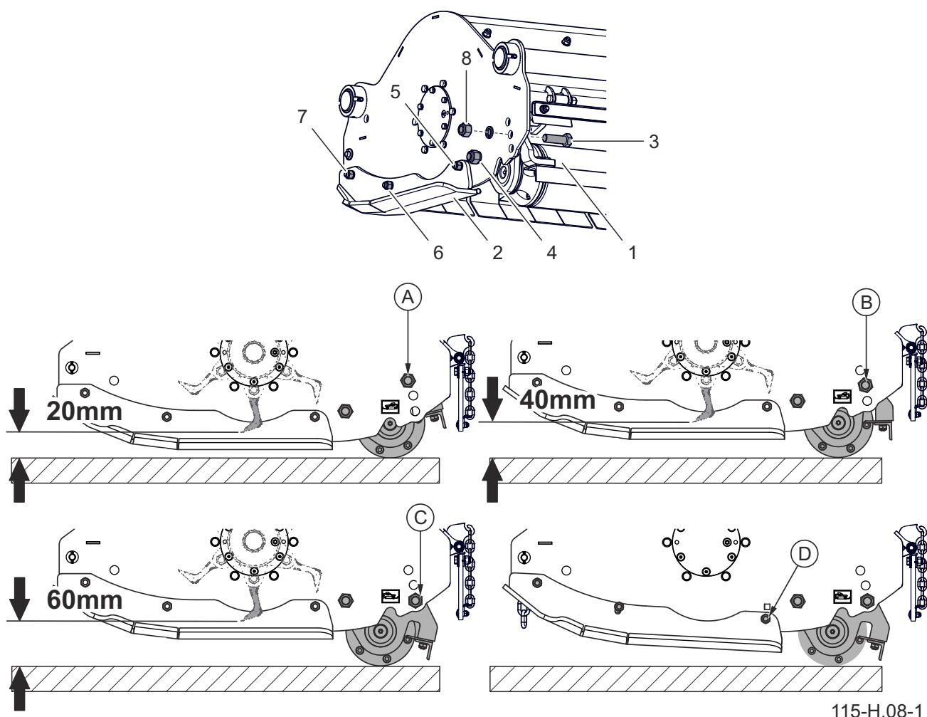
Rysunek 4.9 Ustawienie wysokości koszenia kosiarki
