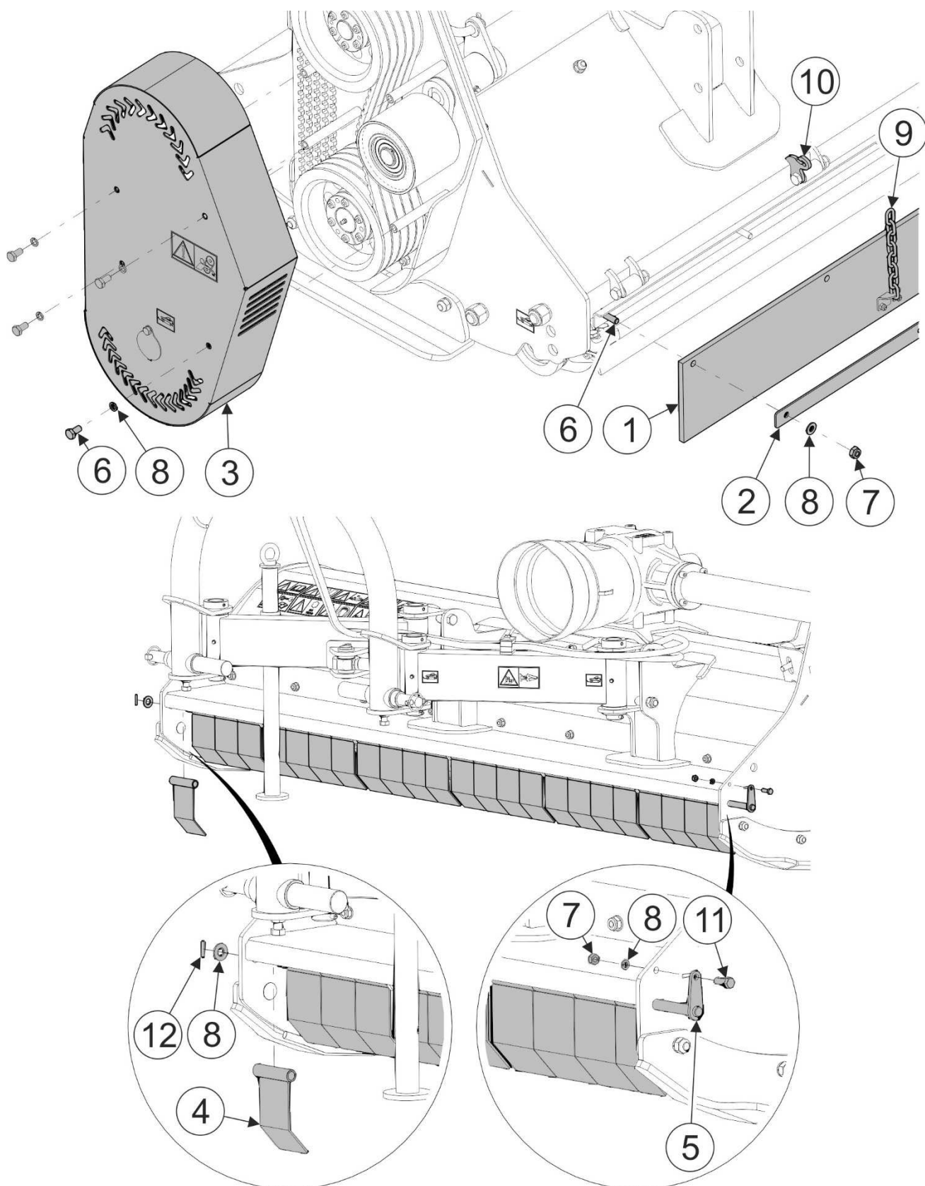
РИСУНОК 5.1 Демонтаж защитных приспособлений
