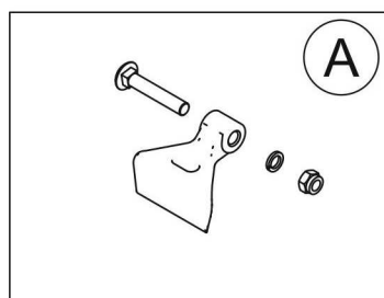
РИСУНОК 5.2 Замена ножей
