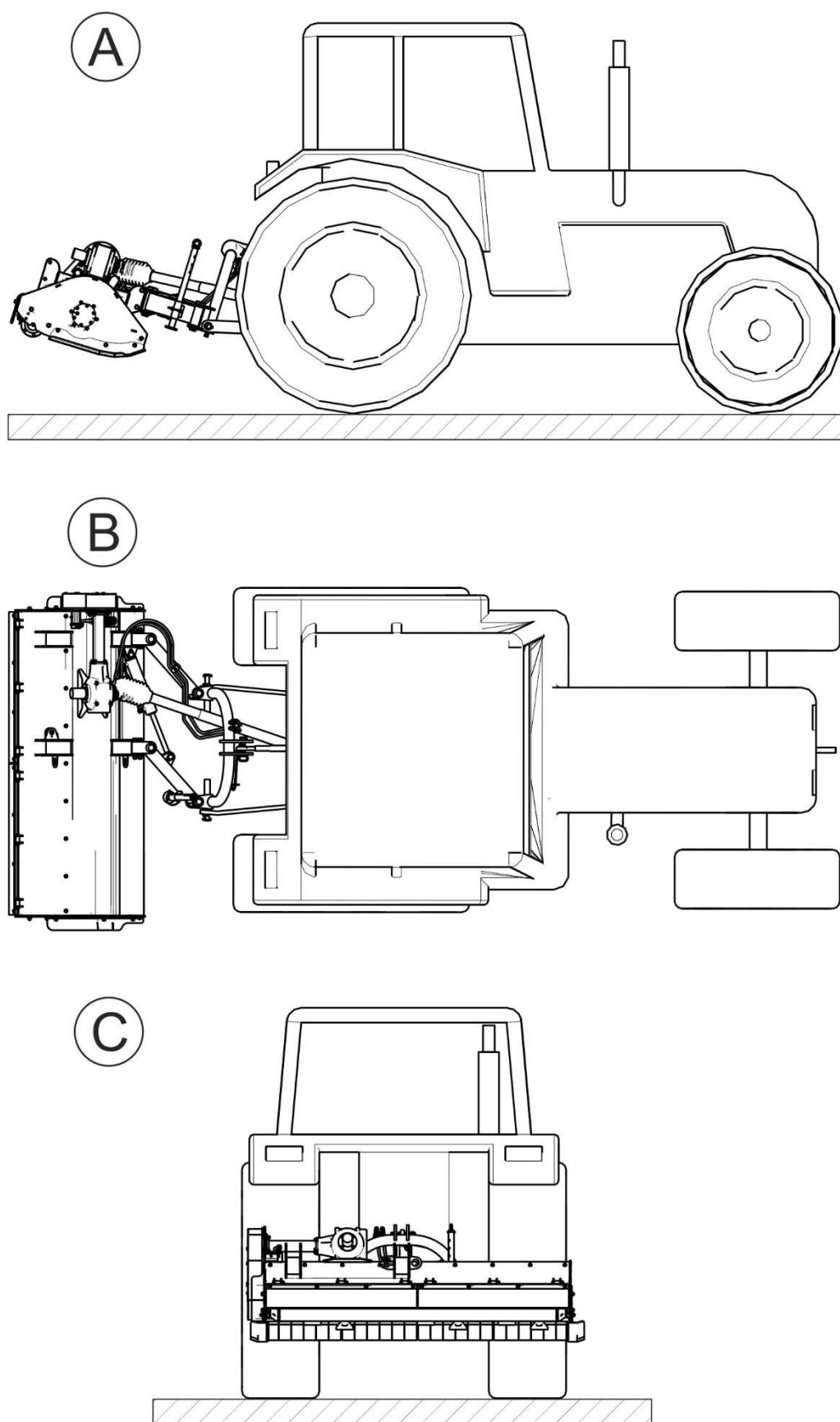
РИСУНОК 4.6 Транспортное положение
