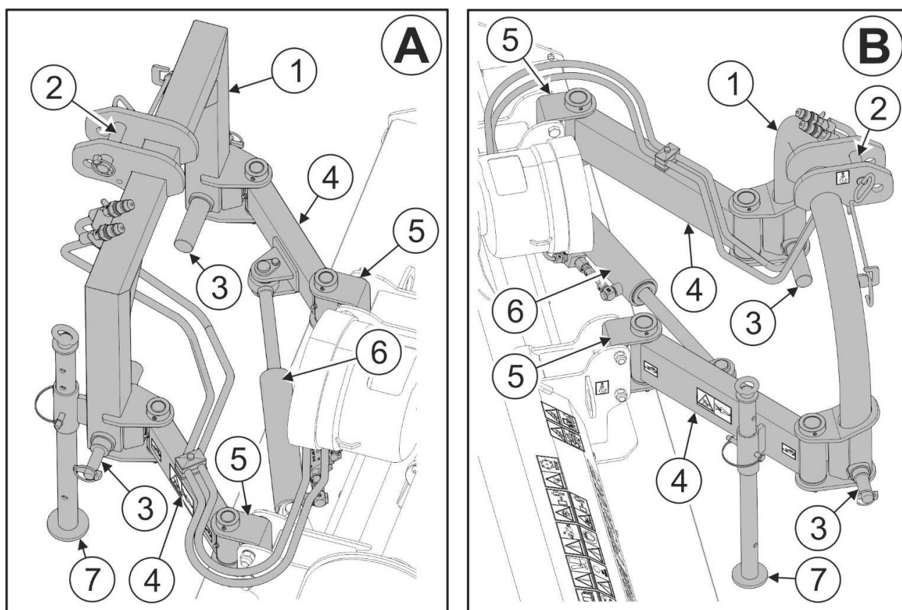
РИСУНОК 3.2 Система навески
