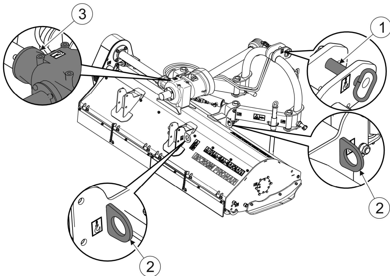
РИСУНОК 1.2 Транспортные захваты.
