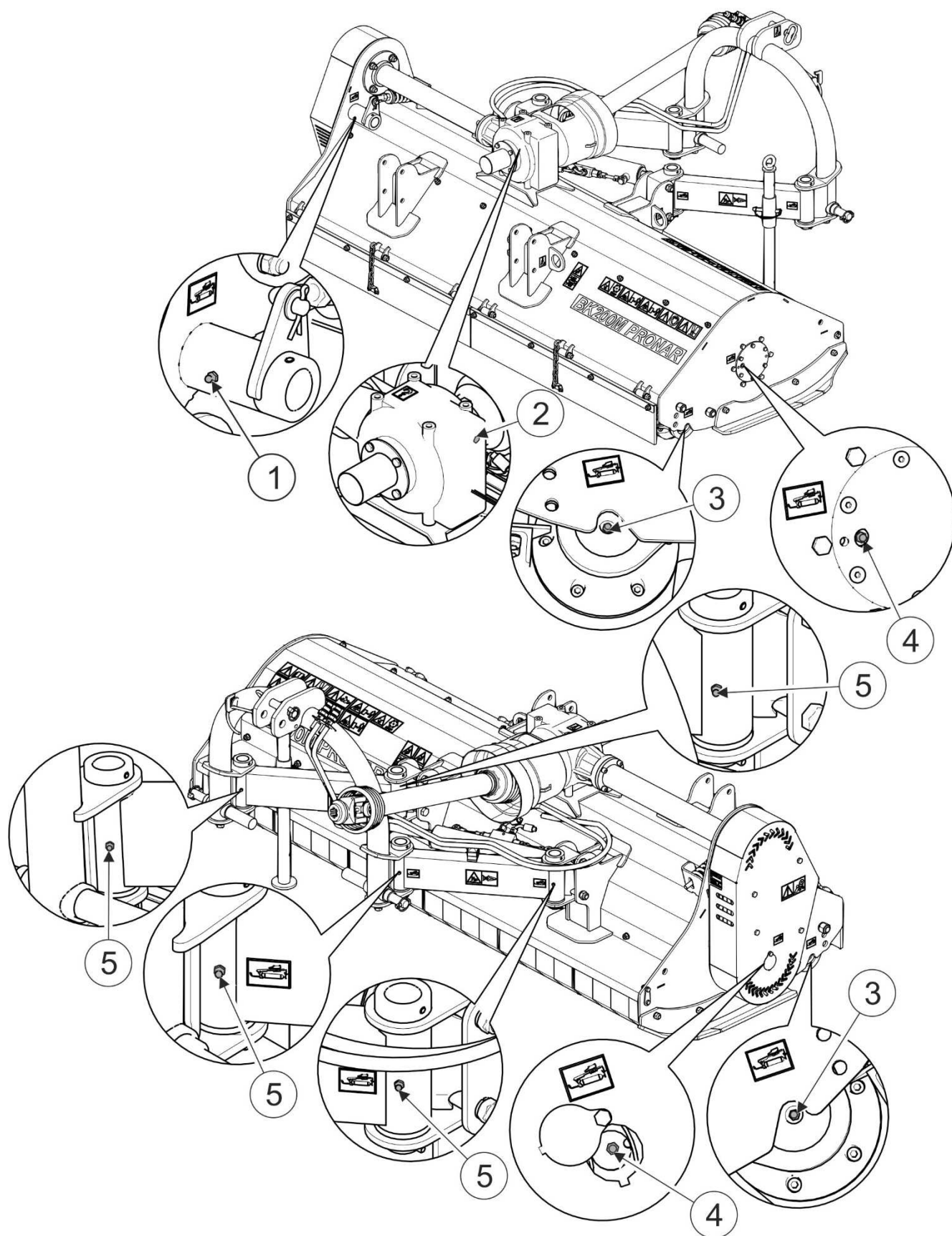
РИСУНОК 5.6 Точки смазки
