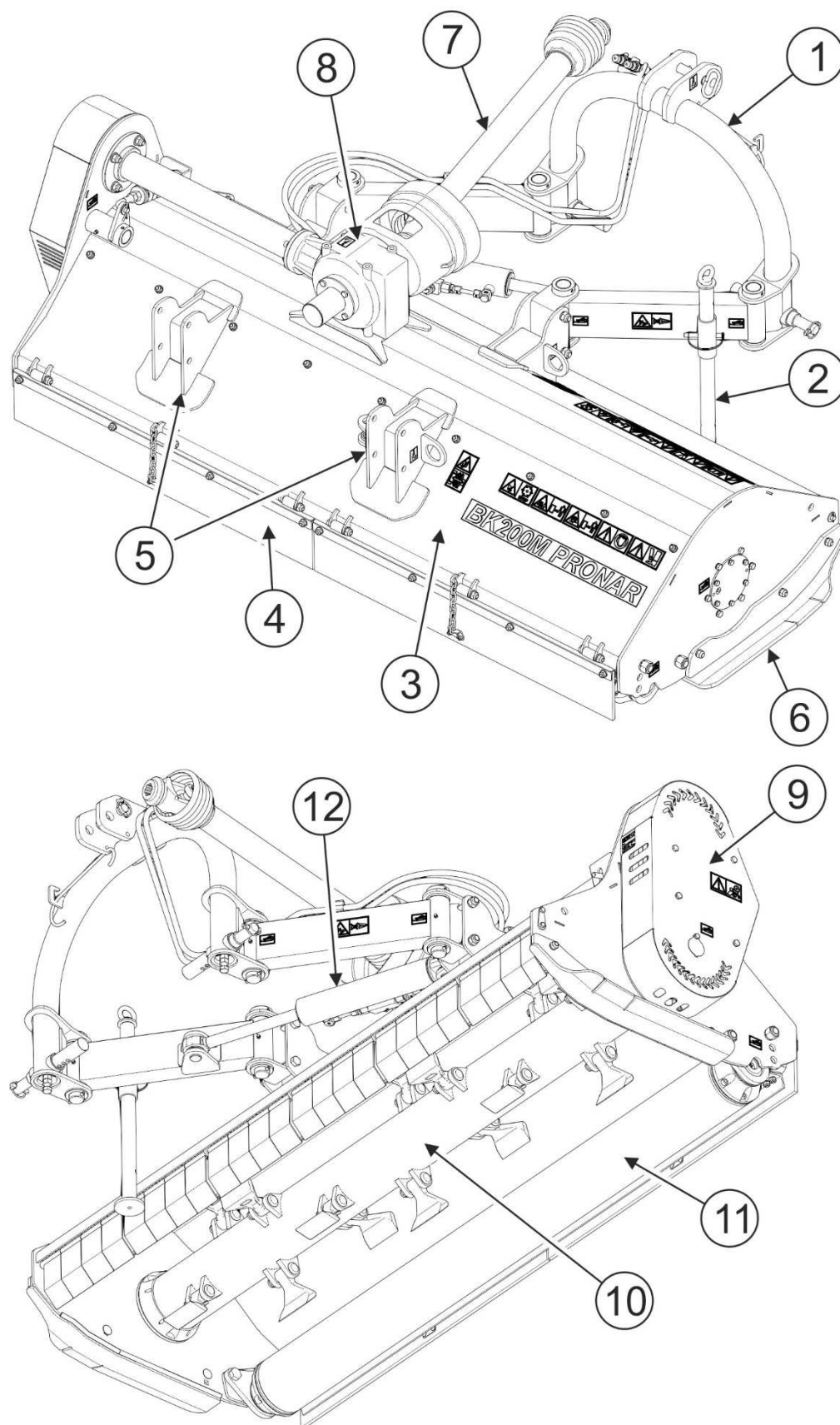
РИСУНОК 3.1 Общее устройство
