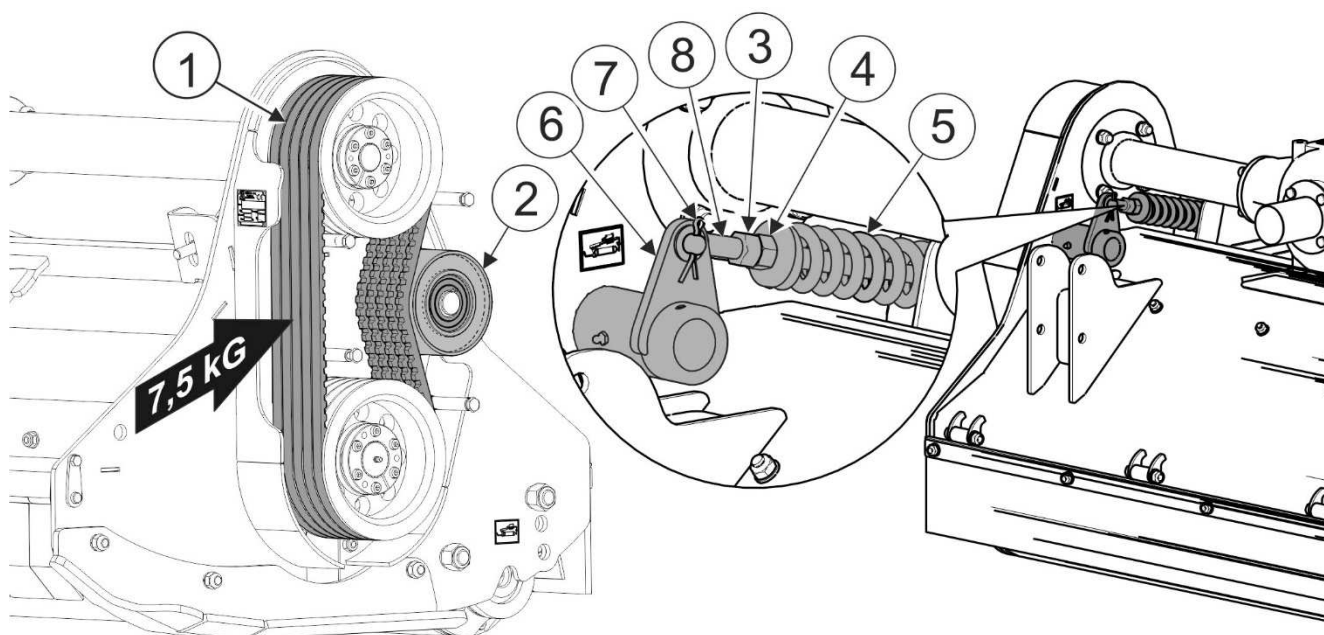
РИСУНОК 5.4 Контроль и регулирование натяжения клиновых ремней
